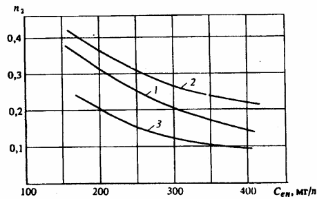
Черт. 2. Зависимость показателя степени n_2 от исходной концентрации взвешенных веществ в городских сточных водах при эффекте отстаивания 1 — \eta = 50\% ; 2 — \eta = 60\% ; 3 — \eta = 70\%
