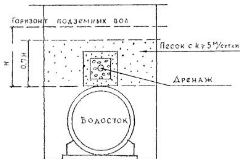
Рис. 9 Схема пластового дренажа
