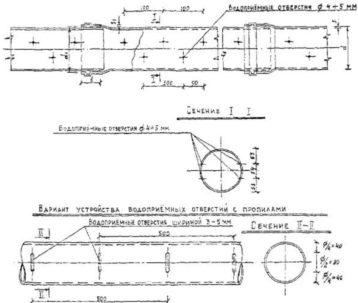
Рис. 11 Труба асбестоцементная с водоприемными отверстиями и с заделкой стыков
