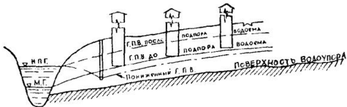
Рис. 5 Комбинированный дренаж с вертикальным самоизливающимся колодцем
