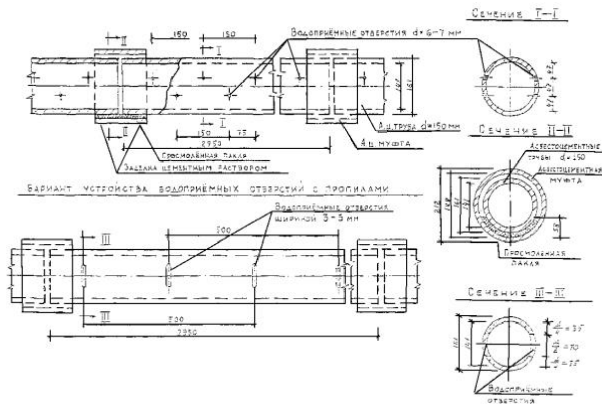
Рис. 10 Схема прокладки дренажа над водостоком
