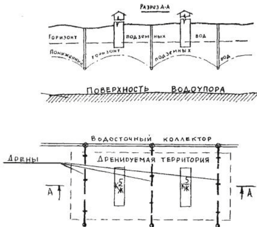
Рис. 7 Схема систематического дренажа
