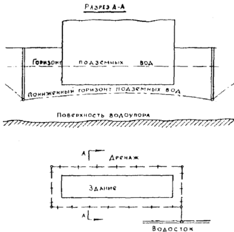
Рис. 7 Схема систематического дренажа
