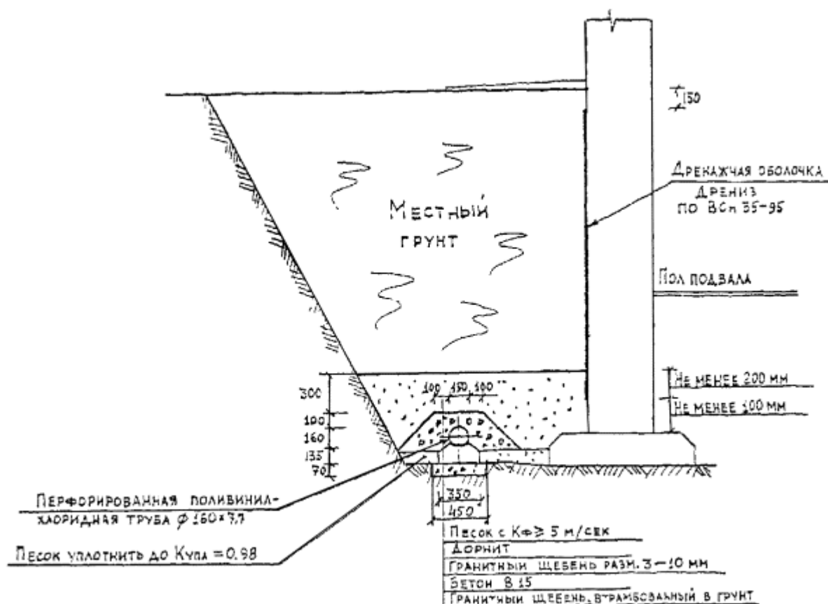
Рис. 14 Пристенный дренаж с применением поливинилхлоридных труб на бетонном основании и дренажной оболочки «Дренаж»
