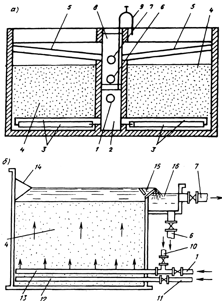
Рис. 5.23. Контактные осветители КО-1 (а) и КО-3 (б):
