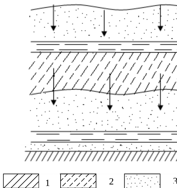
Рис. 1. Схема залегания верховодки на слабопроницаемом водоупоре: 1-песок; 2-супесь; 3-суглинок плотный
