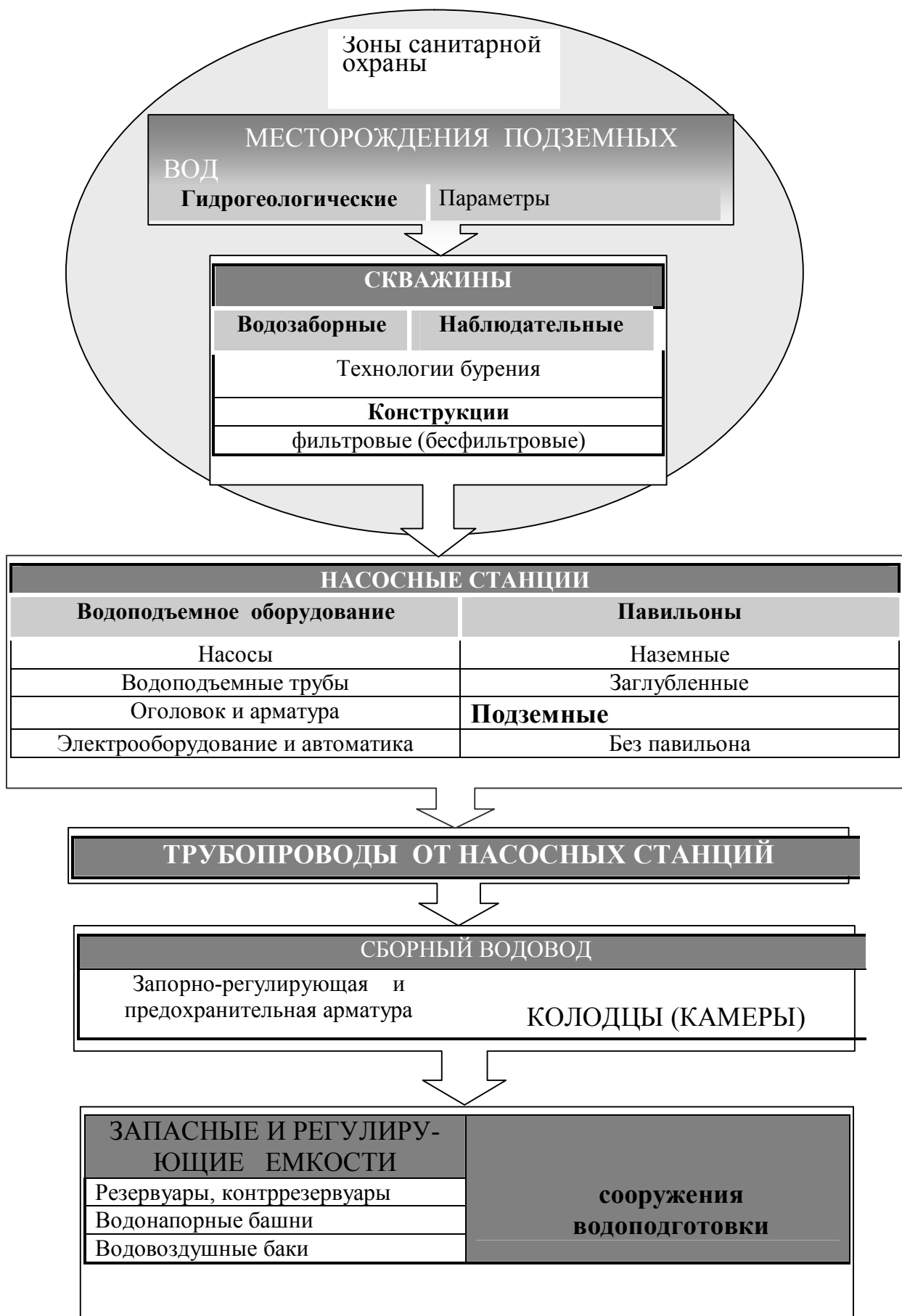
Рис. 3.3 Схема проектирования объектов и элементов скважинного водозабора
