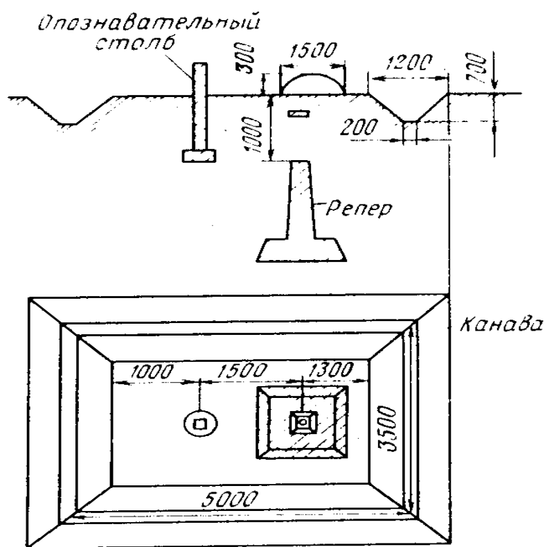
Рис. 15. Внешнее оформление фундаментальных реперов в области сезонного промерзания грунта
