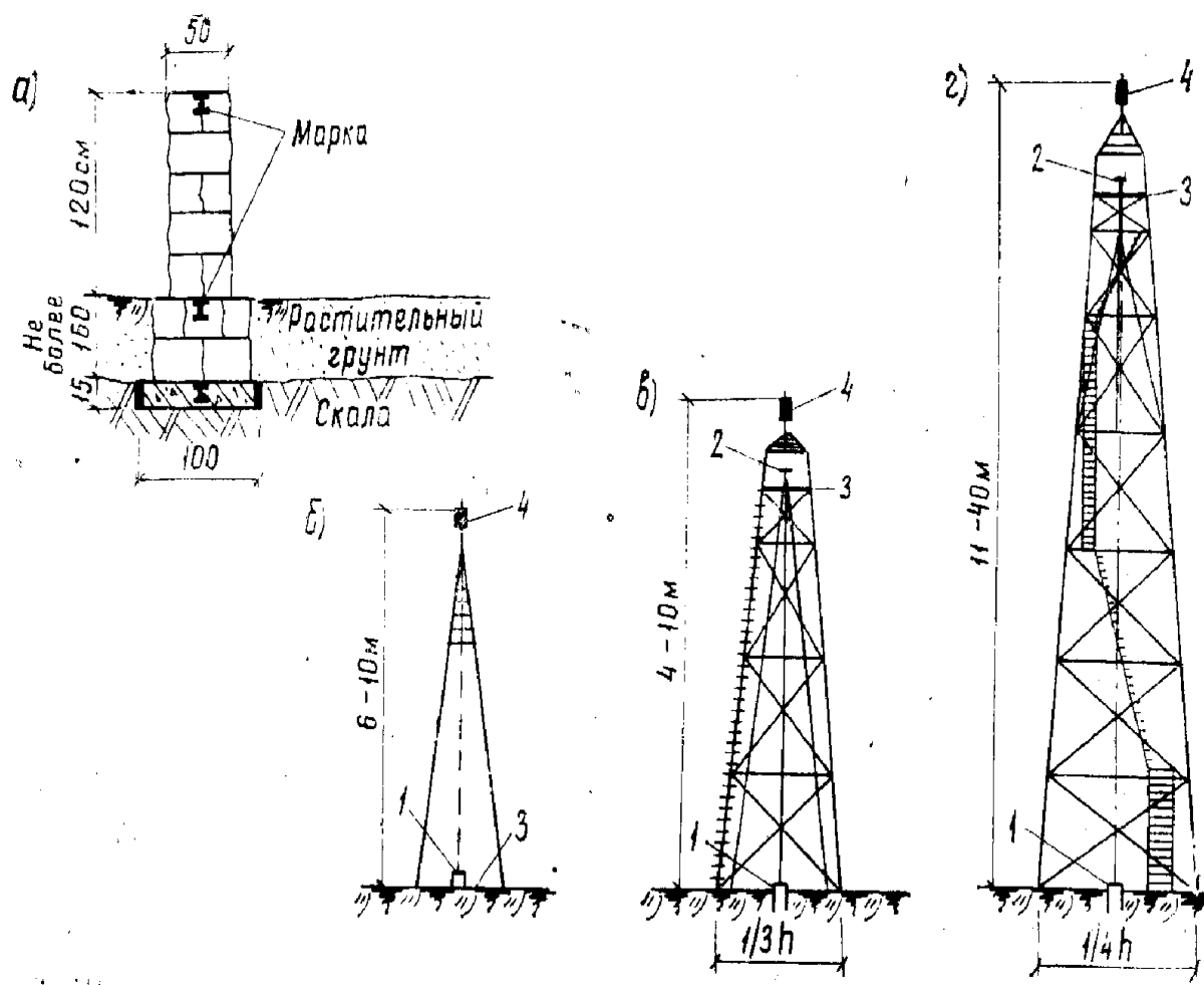
Рис. 7. Геодезические знаки:
