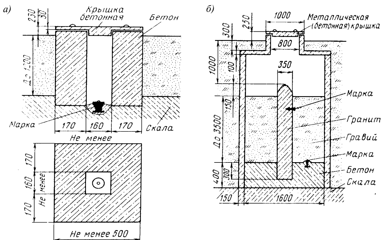
Рис. 10. Вековые реперы для скальных грунтов: а – тип 173; б – тип 174
