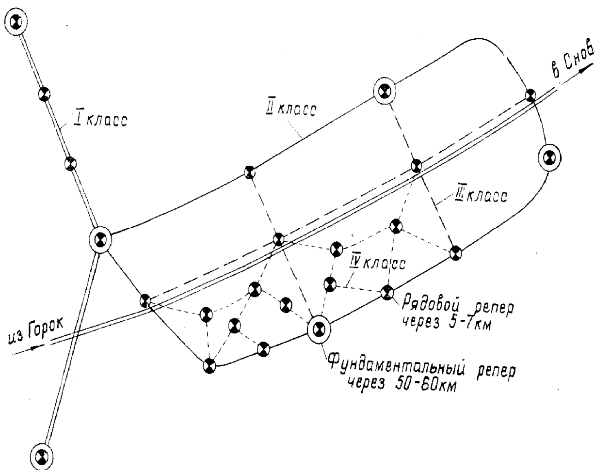
Рис. 9. Схема построения государственной нивелирной сети
