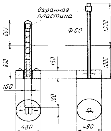
Рис. 16. Оповестительные столбы для сезонного промерзания грунтов
