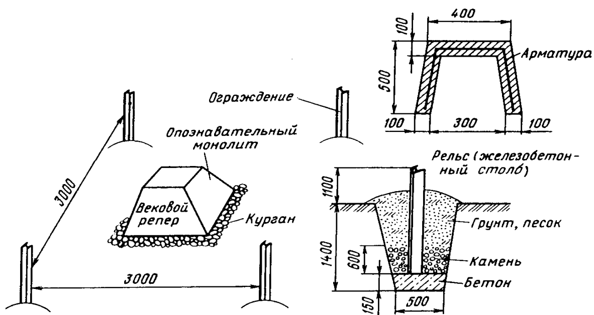
Рис. 14. Внешнее оформление вековых реперов
