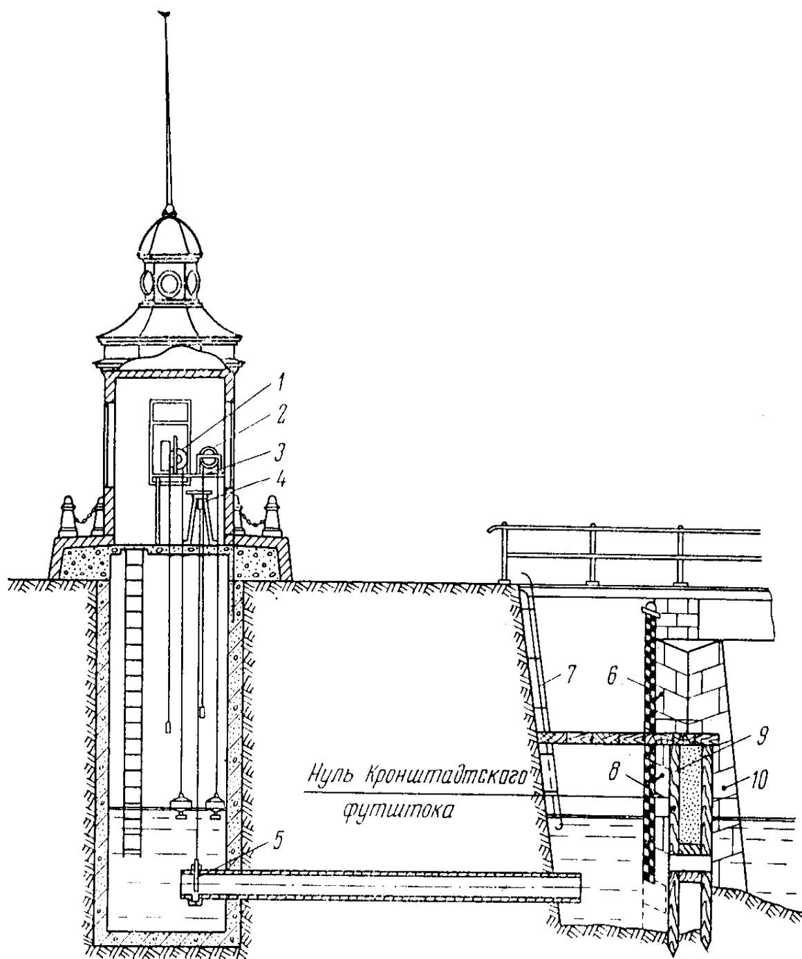
Рис. 4. Устройство Кронштадтского футштока
