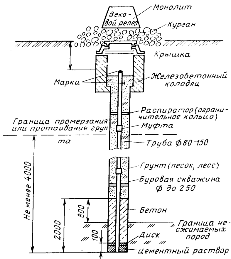
Рис. 11. Вековой трубчатый репер. Тип 175
