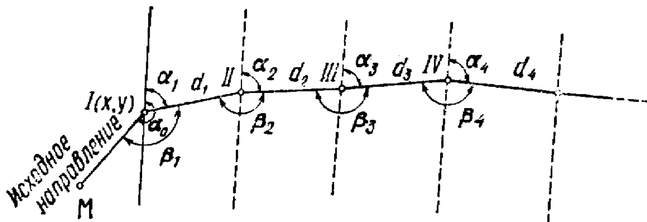
Рис. 2. Полигонометрия
