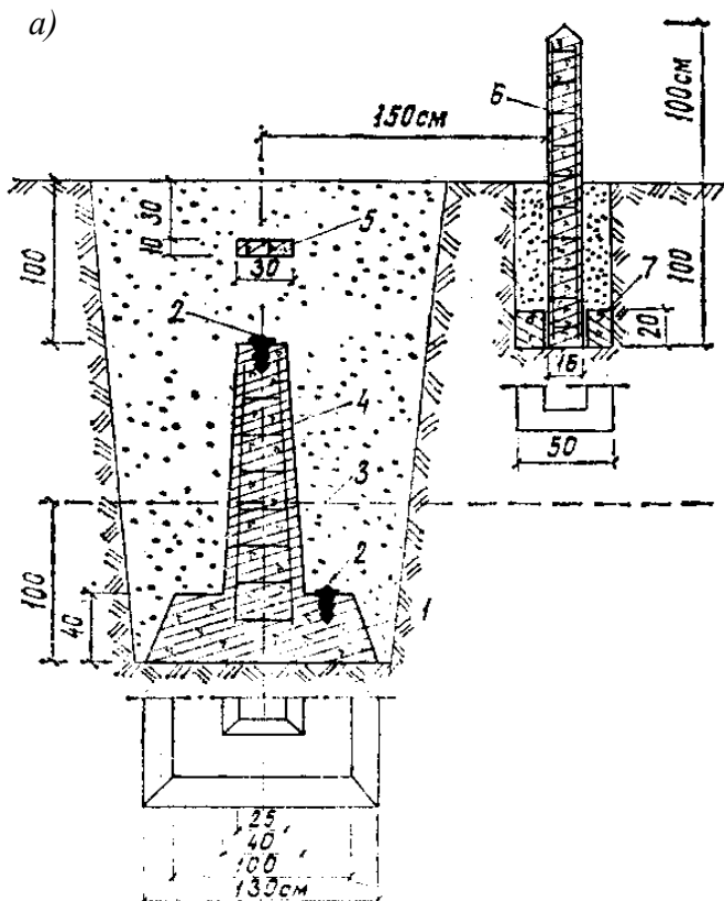
a – фундаментальный репер:
