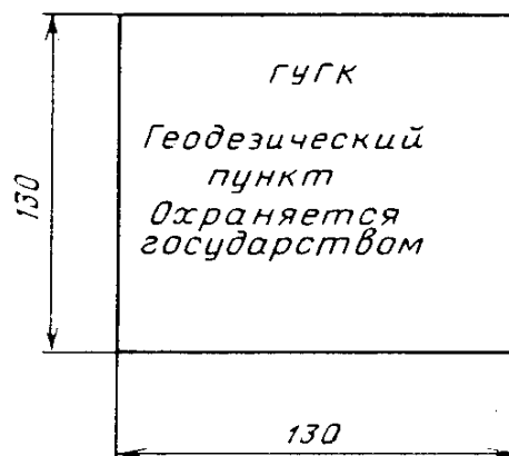
Рис. 17. Охранная пластина
