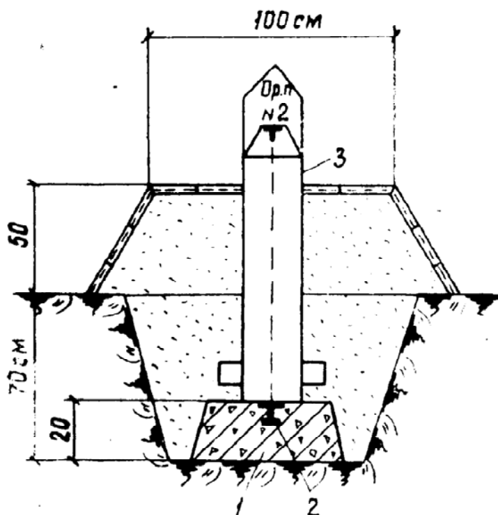
Рис. 8. Ориентирный пункт:
