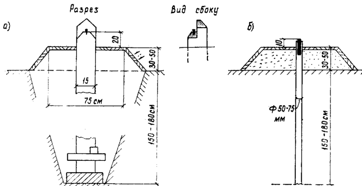
Рис. 20. Конструкция временного репера:
