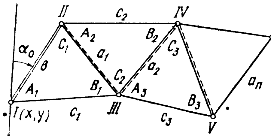
Рис. 1. Триангуляция
