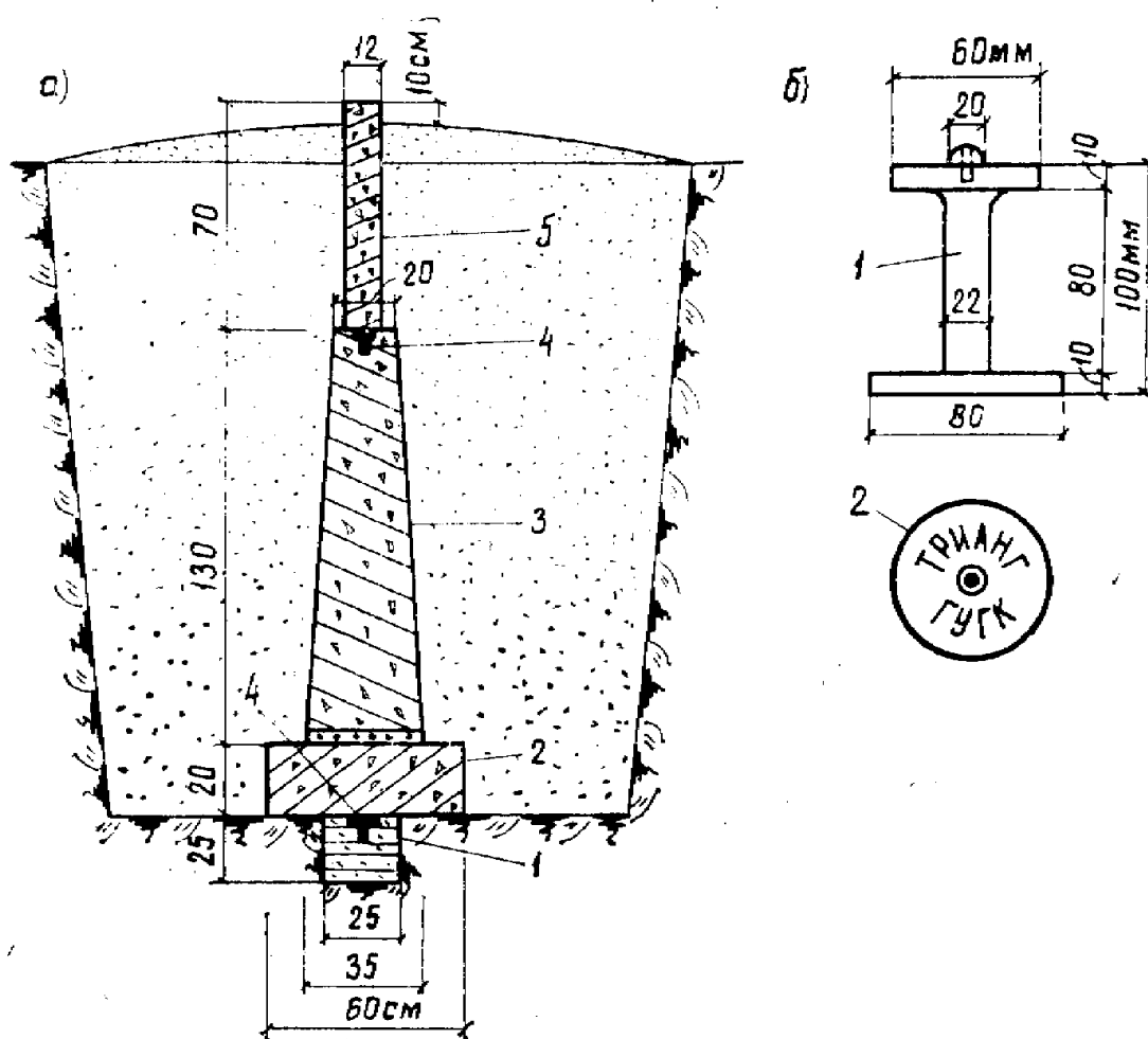
Рис. 6. Центр плановой геодезической сети:
