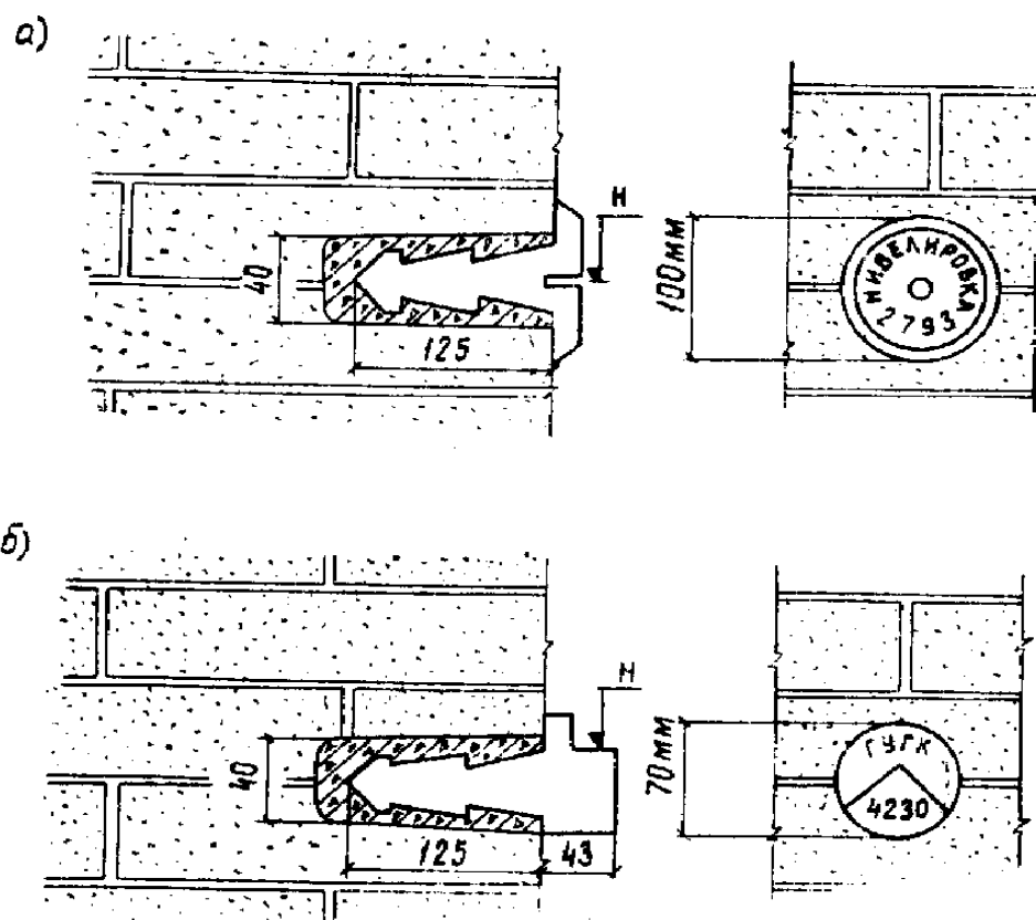
Рис. 13. Марка и репер, закладываемые в стены: а – разрез и вид на стене марки; б – разрез и вид на стене репера
