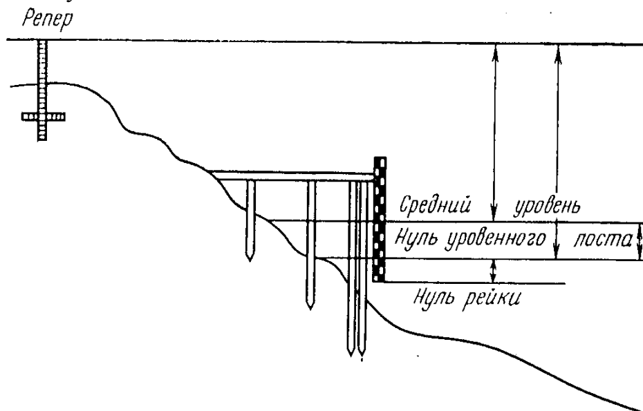
Рис. 3. Устройство уровня поста
