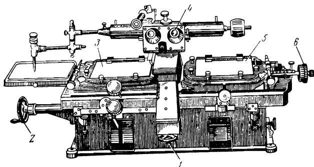
Рис. 108. Стереокомпаратор
