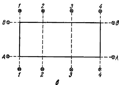
Рис. 145. Типы обноски
