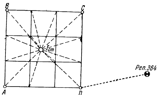
Рис. 86. Схема нивелирования участка с одной станцией
