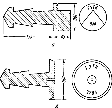
Рис. 41. Типы стенных нивелирных знаков
