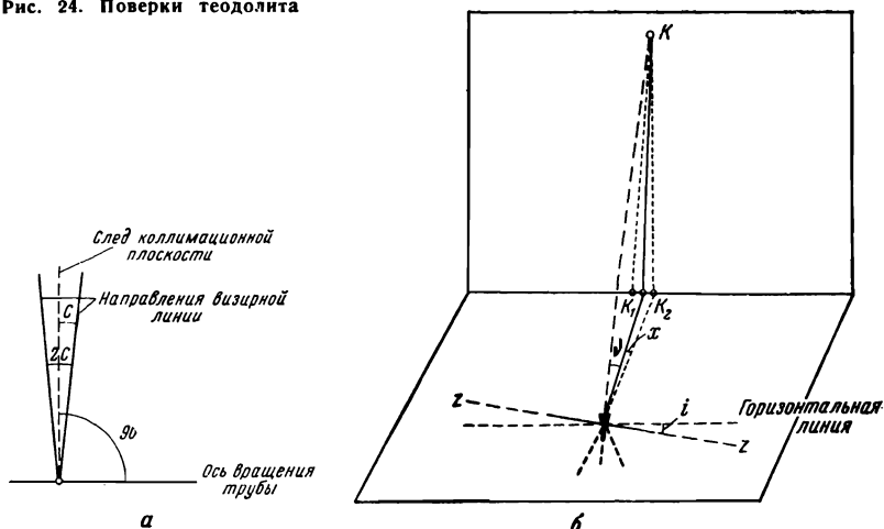
Рис. 24. Поверки теодолита
