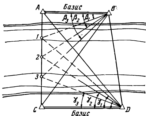
Рис. 189. Схема разбивки моста
