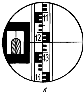
Рис. 73. Глухой нивелир НВ-1 ( a ) и поле зрения ( б )
