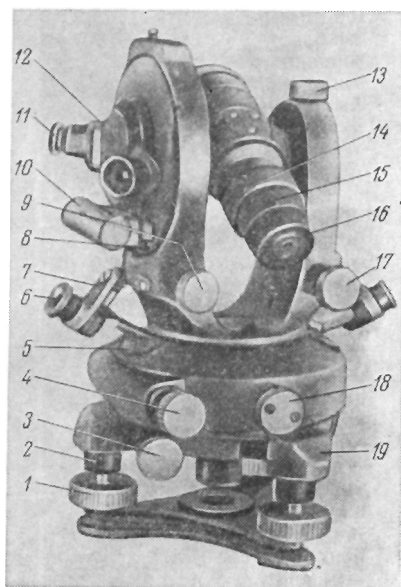
Рис. 15. Теодолит ТМ-1
