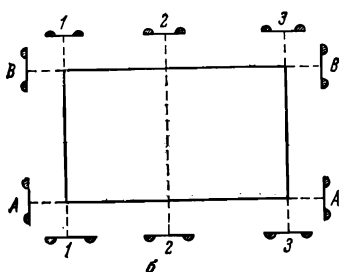
Рис. 145. Типы обноски
