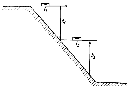
Рис. 93. Ватерпасовка кру- тых склонов
