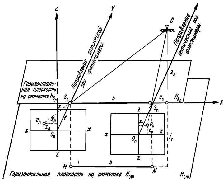
Рис. 107. Схема фототеодолитной съемки
