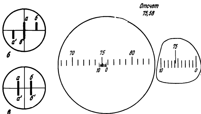
Рис. 7. Часть отсчетной шкалы микроскопа насадки ДНТ
