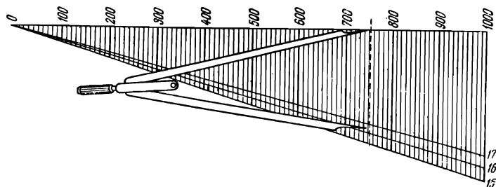
Рис. 113. Клиновой масштаб
