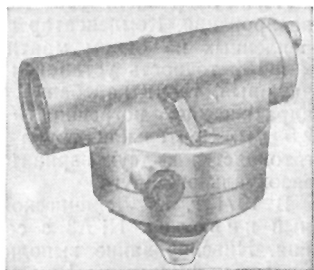
Рис. 76. Нивелир НС4
