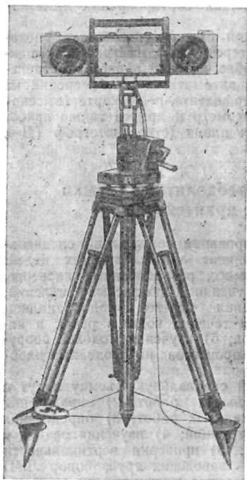
Рис. 110. Стереокamera
