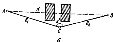
Рис. 48. Схема определения расстояния, недоступного для непосредственных измерений
