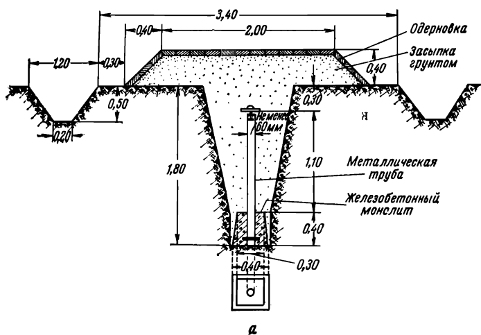
Рис. 40. Типы грунтовых реперов а — фундаментальный грубчатый грунтовый репер; б — рельсовый грунтовый репер.
