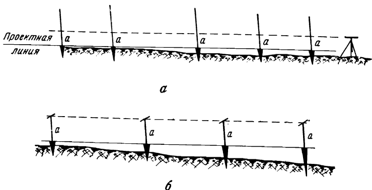
Рис. 157. Схема разбивки наклонной проектной линии при помощи наклонного луча визиринга в нивелир и по визиркам
