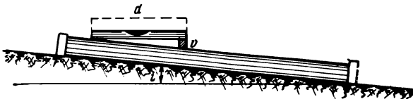
Рис. 155. Схема укладки труб по уровню
