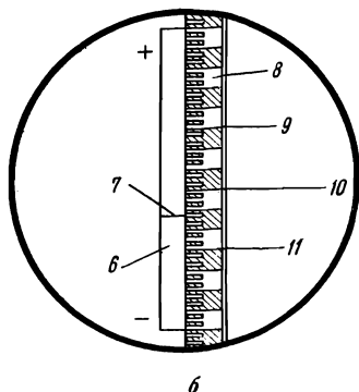
Рис. 75. Нивелир НЛ-3 (а) — оптический высотомер с прямолинейным высотным штрихом и поле зрения (б)
