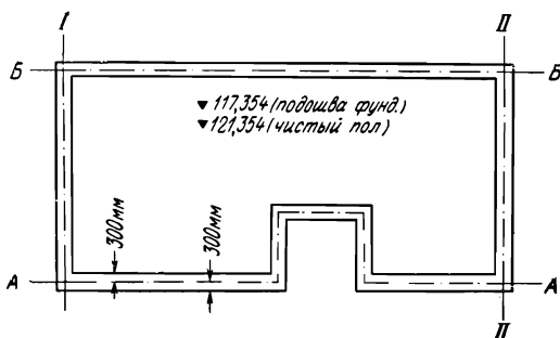
Рис. 174. Разбивочный чертеж фундамента наружных стен
