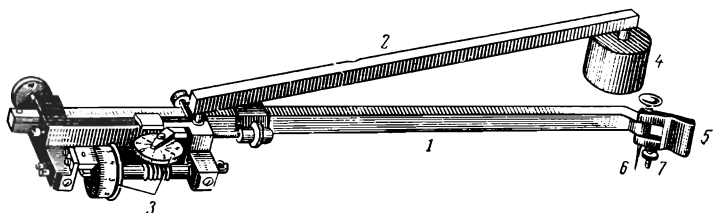
Рис. 62. Полярный планиметр
