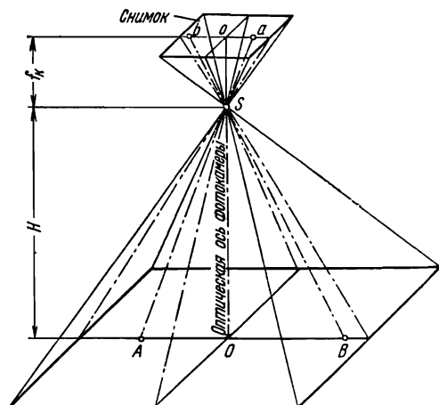
Рис. 111. Схема фото- графирования с са- молета
