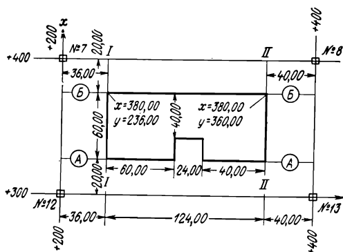
Рис. 173. Разбивочный чертеж основных осей цеха завода от строительной сетки (точки 7, 8, 12, 13)
