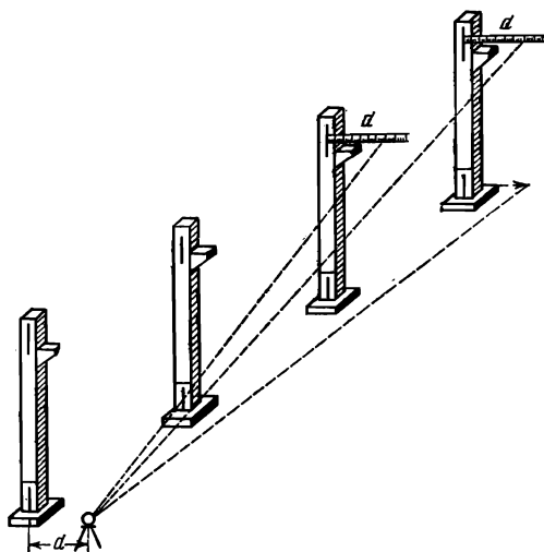
Рис. 152. Проверка установки ряда колонн
