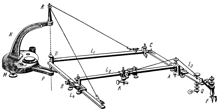
Рис. 65. Пантограф
