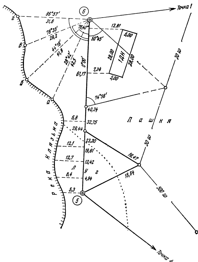
Рис. 56. Абрис съемки
