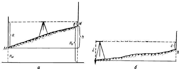
Рис. 67. Два способа геометрического нивелирования
