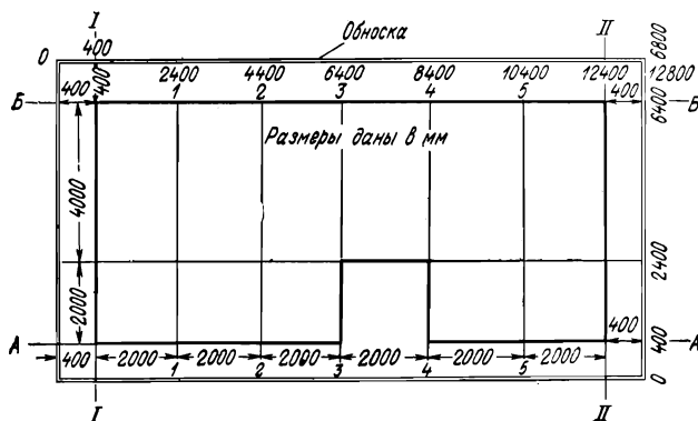
Рис. 175. Разбивочный чертеж обноска и внутренних осей фундамента
