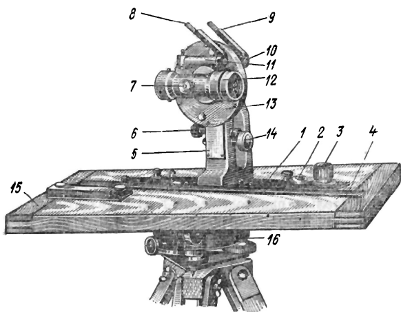
Рис. 101. Мензула и кипрегель КБ-1
