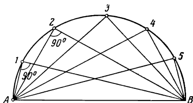
Рис. 166. Схема разбивки окружности при помощи эккера
