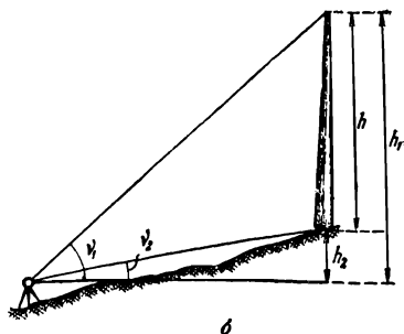
Рис. 138. Схема определения теодолитом высоты соору- жения
