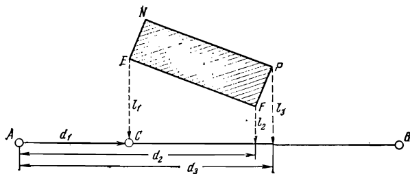
Рис. 49. Съёмка здания по способу перпендикуляров
