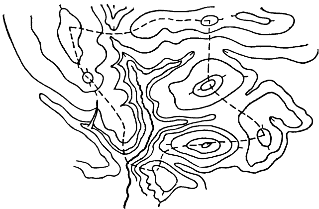
Рис. 127. Площадь водосбора
