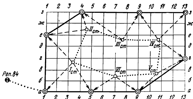
Рис. 87. Схема нивелирования связующих точек
