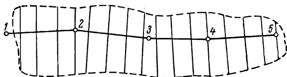
Рис. 88. Схема нивелирования теодолитно-нивелирной магистральной с поперечниками
