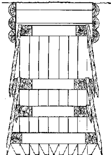
Рис. 8. Изоляция плавбуна косым шпунтом
