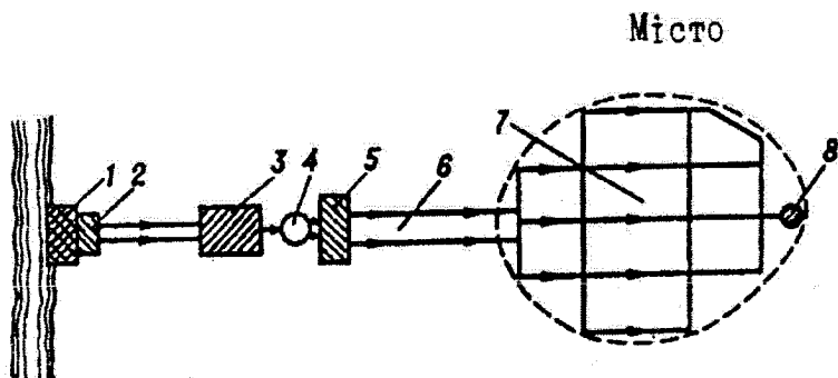
Рис. 3.2. Загальна схема системи водопостачання: 1 - водоприймальна споруда (водозабір); 2 - насосна станція першого підйому; 3 - водоочисні споруди; 4 - резервуар чистої води; 5 - насосна станція другого підйому; 6 - водоводи; 7 - водопровідна мережа; 8 - водонапірна вежа
