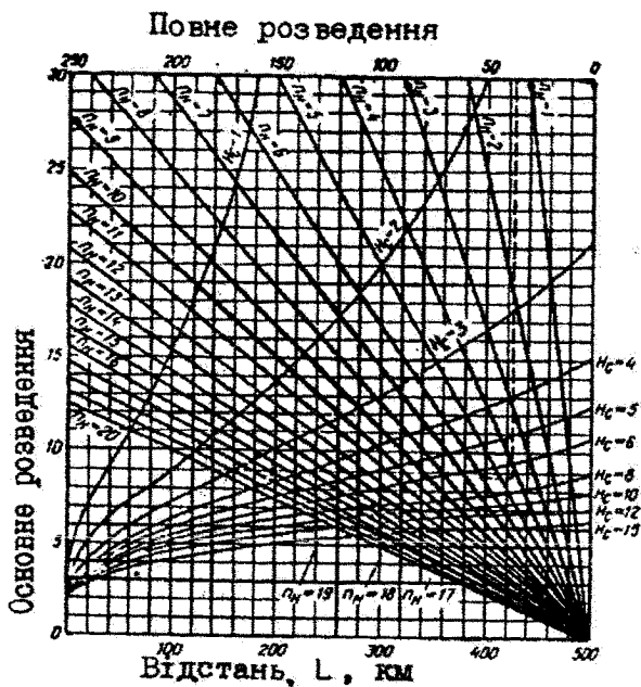
Рис. 11.2. Номограма для визначення повного розведення стічних вод при випуску в глибокі шарі водосховища
