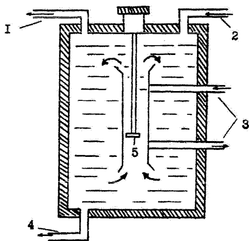
Рис. 9.6. Спрощена схема метантенка: 1 - збирання газу; 2 - свіжий осад; 3 - гаряча вода; 4 - зброджений осад; 5 - змішувач
