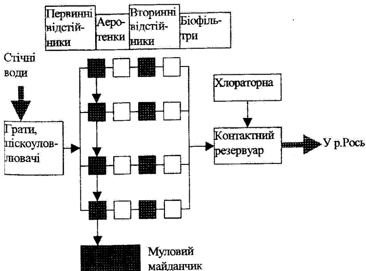
Рис. 3.16. Загальна схема станції очистки стічних вод м.Богуслава Київської області
