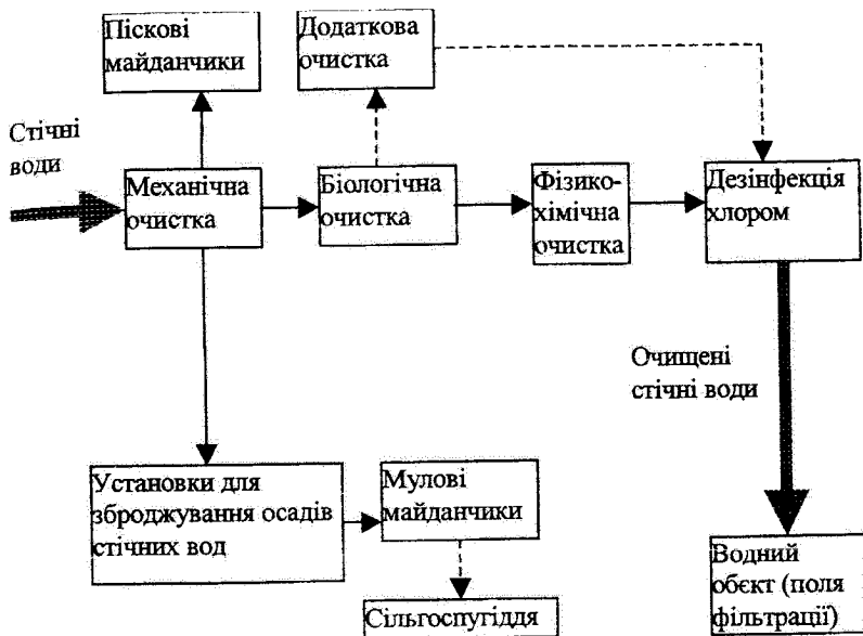
Рис. 3.15. Загальна схема видів очистки стічних вод на очисних спорудах
