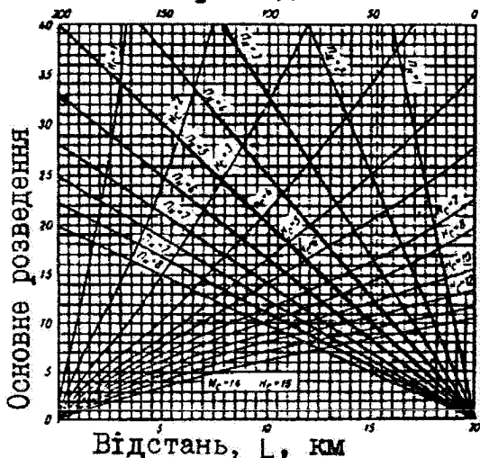
Рис. 11.1 Номограма для визначення повного розведення стічних вод при випуску в поверхневий шарі водосховища
