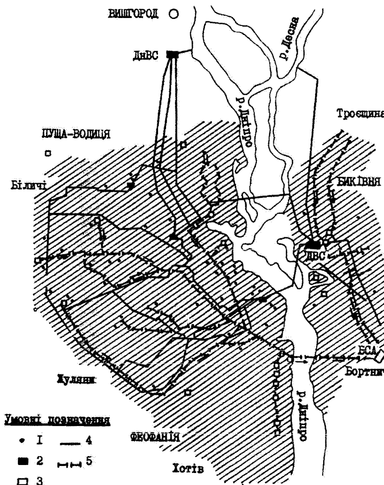
Рис. 3.1. Схема водопостачання і водовідведення м. Києва: 1 - артезіанська свердловина; 2 - водопровідна насосна станція; 3 - каналізаційна насосна станція; 4 - водовод; 5 - каналізаційний колектор; ДнВС - Дніпровська водопровідна станція; ДВС - Деснянська водопровідна станція; БСА - Бортницька станція аерації
