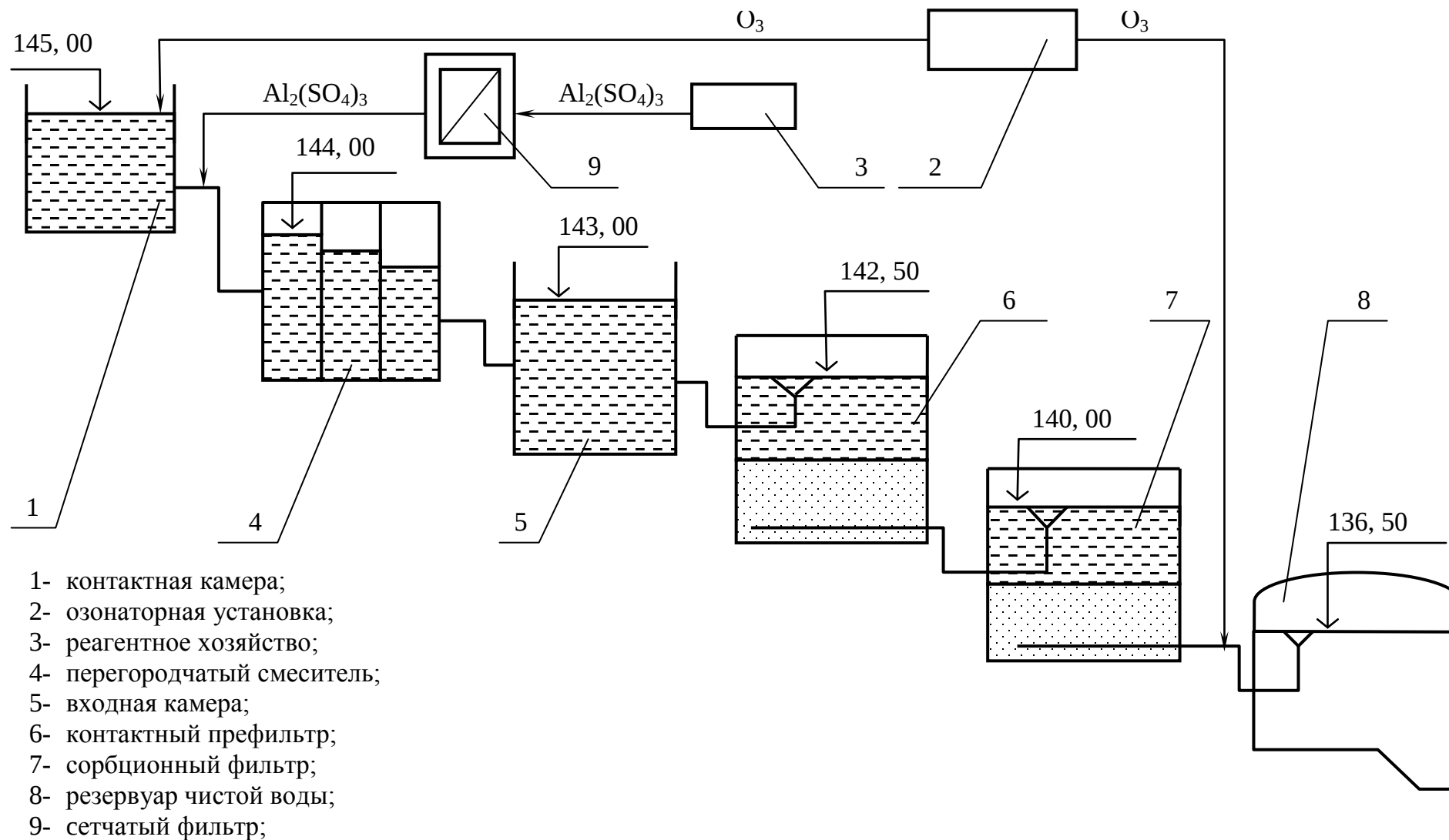
Рисунок 7.... – Высотная схема технологических сооружений водоочистой станции с контактными префильтрами-фильтрами
