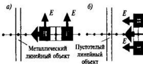
Рисунок 4.1. Оптимальная ориентация антенного блока и направления дорожки (профиля) сканирования относительно тонкого линейного объекта, металлического или пустотелого, с диэлектрическими стенками
