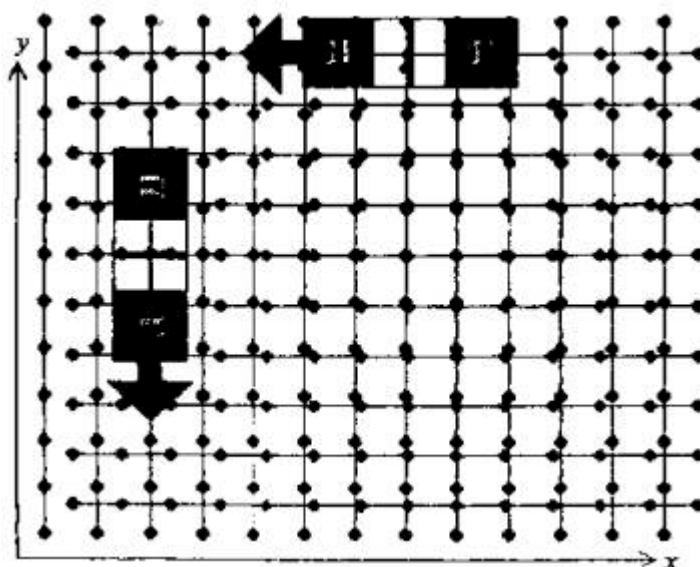
Рисунок 4.3. Схема сканирования при двух ортогональных направлениях прохождения профилей, каждое со своим направлением поля E , перпендикулярным профилю
