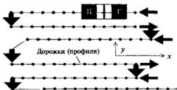
Рисунок 4.2. Схема сканирования вдоль параллельных профилей с одной поляризацией излучаемого и принимаемого полей
