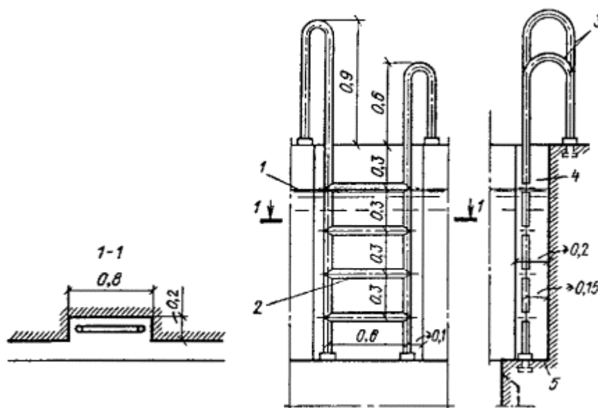
Рис. 9. Схемы лестницы для выхода из ванны
