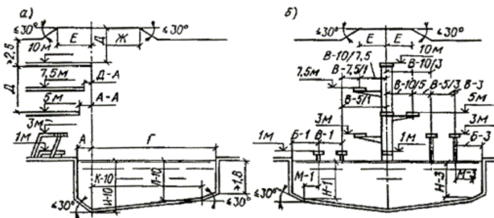
Рис. 3. Схема для определения размеров ванн для прыжков в воду и расстояний между устройствами для прыжков
