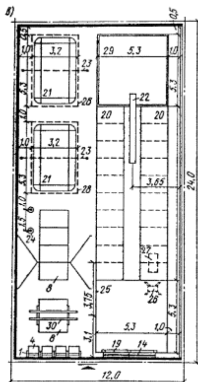
Рис. 11. Схематические планы расстановки оборудования в залах подготовительных занятий а - в зале 18×9 м при ванне для плавания длиной 25 м; б - в зале 24×12 м при ванне для плавания водного поло длиной 50 м; в - в зале 24 × 12 м при специализированной ванне для прыжков в воду или универсальной ванне длиной 50 м
