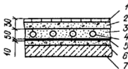
Рис. 10. Схема конструкции обходной дорожки крытых бассейнов
