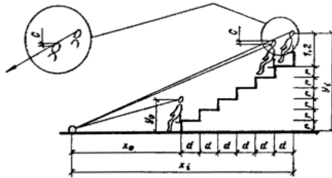
Рис. 14. Построение профиля трибуны по наклонной прямой аналитическим методом
