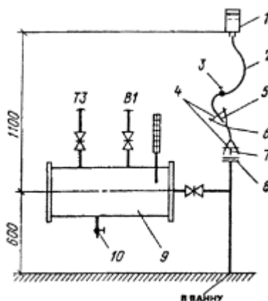
Рис. 22. Схема введения реагента с применением «Кружки Эсмарха» (расход раствора до 3 л/сут) 1 - ирригатор емкостью 1,5л (стеклянный); 2 - шланг; 3 - зажим; 4 - проволочная скрутка; 5 – наконечник; 6 - трубка резиновая \varnothing = 8 мм; 7 - штуцер \varnothing = 10 мм; 8 - глухой фланец \varnothing = 10 мм; 9 - смеситель; 10 - слив
