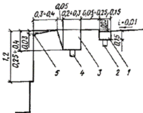
Рис. 23. Схема борта ванны с разделением воды: из ванны - на очистку с обходных дорожек - в канализацию
