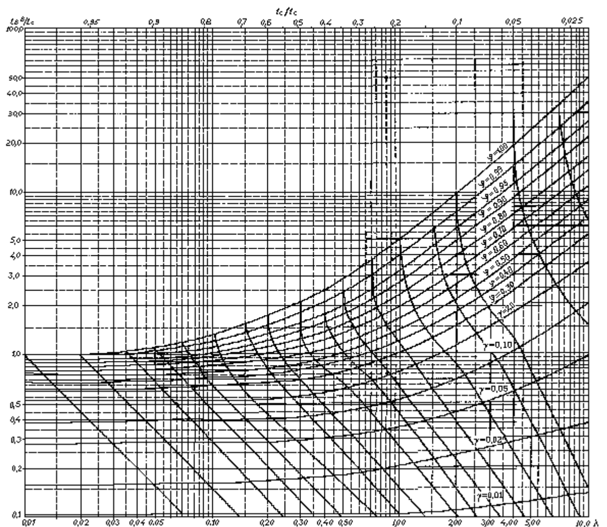
Рис. 2. Номограмма для определения полноты стока
