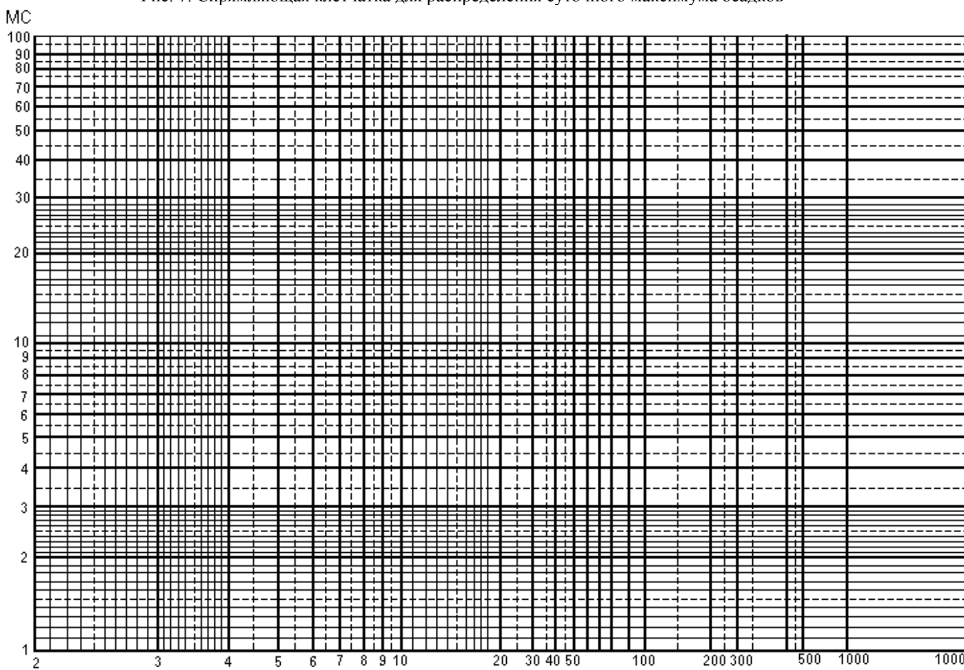
Рис. 8. Спрямяющая клетчатка для распределения месячных сумм осадков
