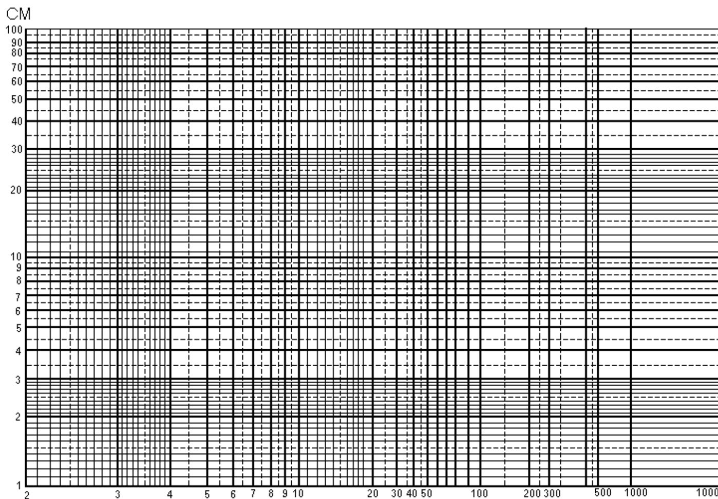
Рис. 7. Спрямяющая клетчатка для распределения суточного максимума осадков
