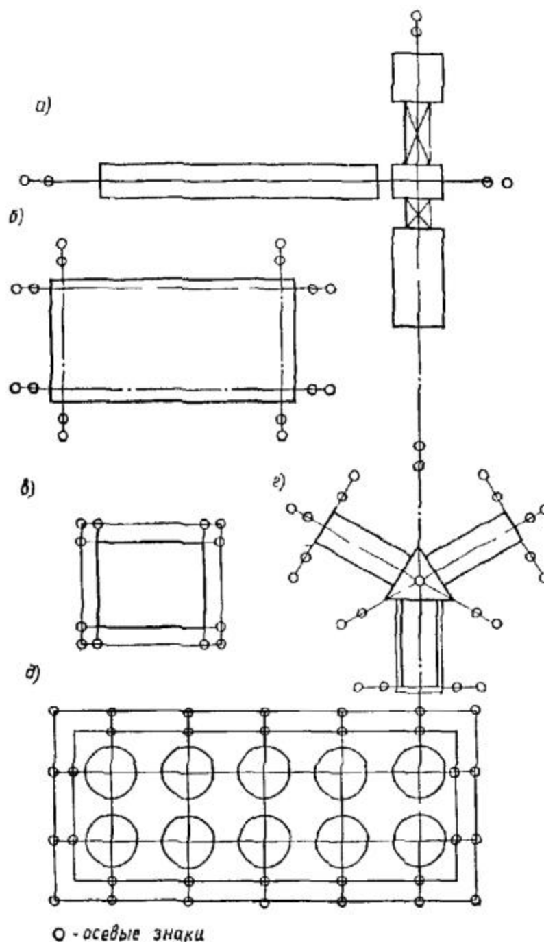
а - завод; б - жилое здание; в - цех; г - жилое здание типа «звездочка»; д - резервуарный парк
