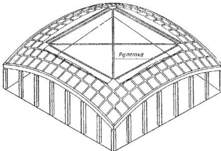
Рис. 25. Схема измерений при контроле планового положения сборных пят оболочки
