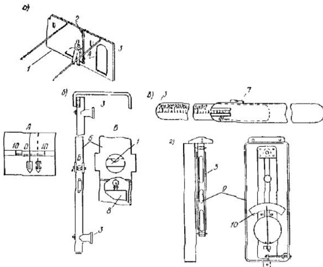
Рис. 22. Контроль вертикальности (а) и специальные рейки: с уровнем (б), телескопическая (в), маятниковый отвес (г)
