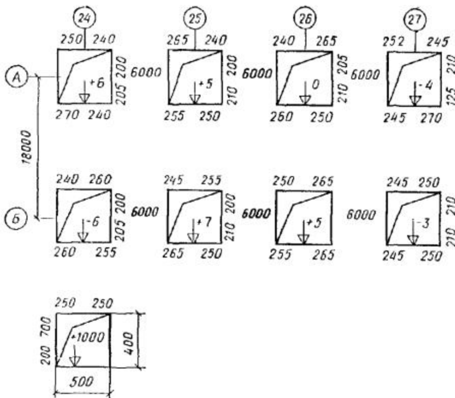
Рис. 27. Исполнительная схема плано-высотного положения стаканов фундаментов под железобетонные колонны. Проектные размеры приведены в миллиметрах; (+) завышенные, (-) заниженные от проектной отметки дна стакана
