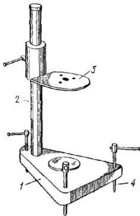
Рис. 6. Консольный штатив для установки геодезических приборов
