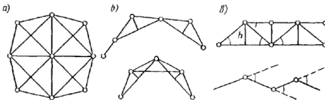
Рис. 13. Схемы внутренних разбивочных сетей зданий и сооружений
