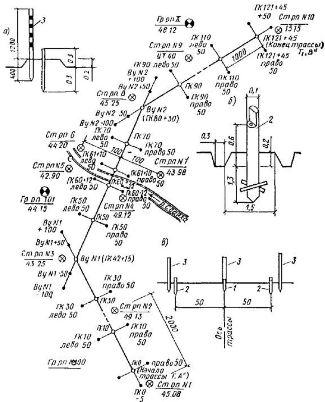
а - временный знак по трассе трубопровода (все размеры даны в метрах); б - постоянный знак по трассе; в - схема закрепления знаков по оси трассы; 1 - временные знаки; 2 - постоянные знаки; 3 - опознавательные вехи
