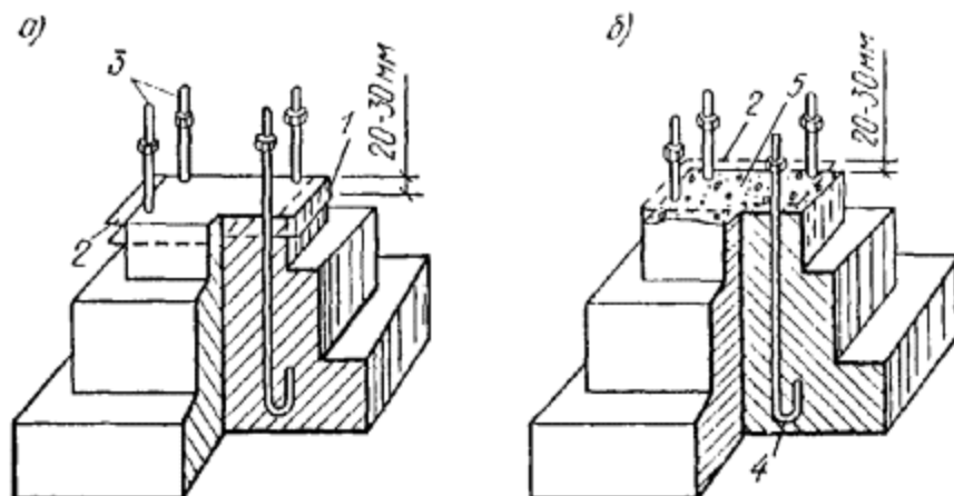
Рис. 11. Подготовка фундамента для монтажа стальных колонн
