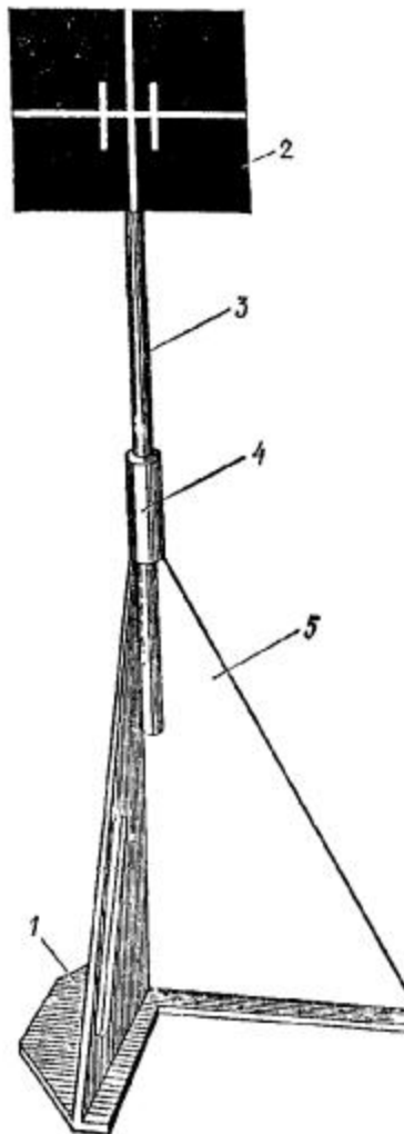
Рис. 12. Марка для нанесения рисок
