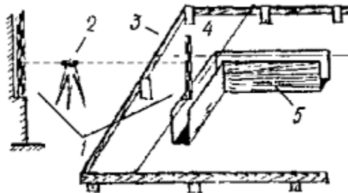
Рис. 10. Высотная разбивка опалубки монолитных фундаментов
