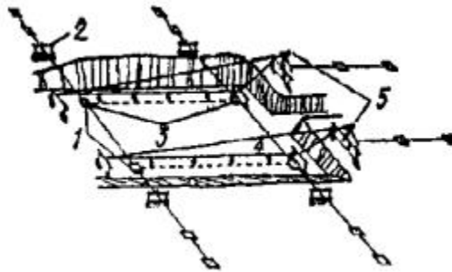
Рис. 8. Перенос разбивочных осей на дно котлована
