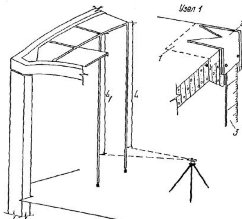
Рис. 23. Метод контрольно-монтажных измерений в процессе установки плит в проектное положение
