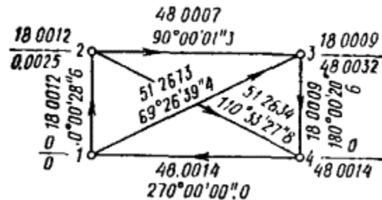
Рис. 19. Схема внутренней разбивочной сети на монтажном горизонте
