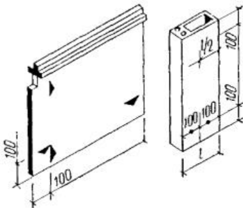
Рис. 31. Места съемки элементов конструкций зданий
