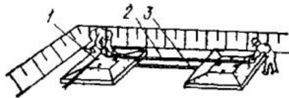
Рис. 21. Контроль укладки фундаментов в плане
