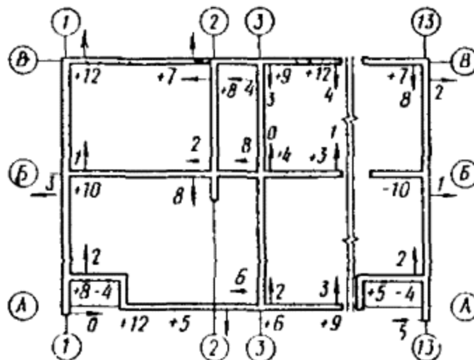
Рис. 28. Исполнительная схема положения блоков подвальной части здания. Стрелками показаны смещения блоков с осей; цифрами со знаком (+) или (-) обозначены отклонения от проектной отметки в миллиметрах
