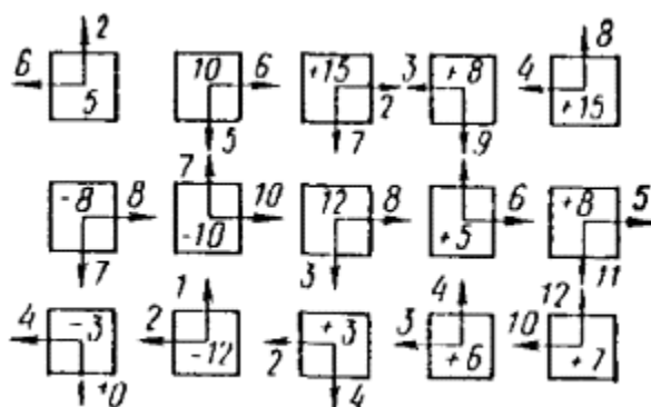
Рис. 28. Исполнительная схема положения блоков подвальной части здания. Стрелками показаны смещения блоков с осей; цифрами со знаком (+) или (-) обозначены отклонения от проектной отметки в миллиметрах
