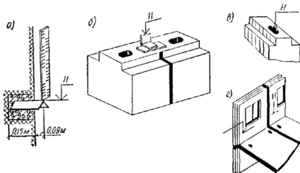
Рис. 17. Знаки закрепления высотной разбивочной сети
