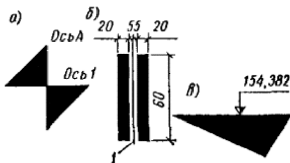
Рис. 15. Откраска осей (а, б) и отметок (в) на конструкциях зданий и сооружений
