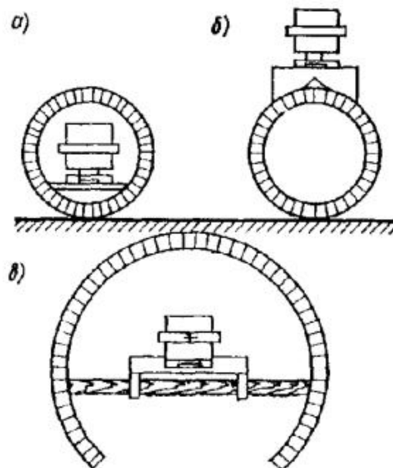
Рис. 5. Установка навесных контрольных марок на секции трубопровода
