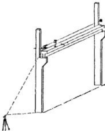
Рис. 33. Съемка подкрановых путей с помощью лазерного прибора
