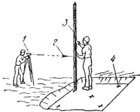
Рис. 20. Контроль после зачистки оснований для фундаментов
