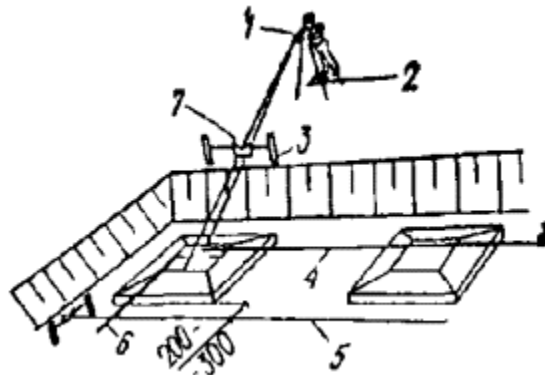
Рис. 9. Перенос разбивочных осей на фундаментные блоки с помощью теодолита
