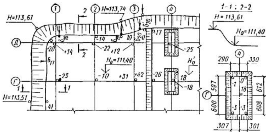
Рис. 26. Места исполнительной съемки котлована и примеры записи результатов. Размеры (кроме отметок) приведены в миллиметрах; -18, -26 - отклонение отметки дна котлована от проектной; \delta_{17} , \delta_{20} - отклонения верхней и нижней бровок от проектного положения
