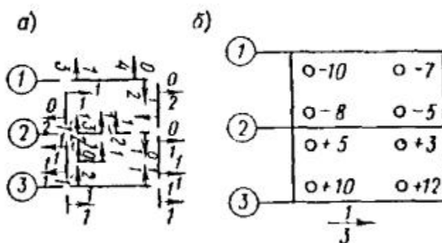
Рис. 30. Исполнительная схема планово-высотного положения конструкций цокольного этажа
