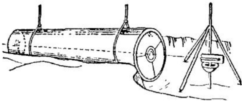
Рис. 4. Укладка секций трубопровода по лазерному лучу
