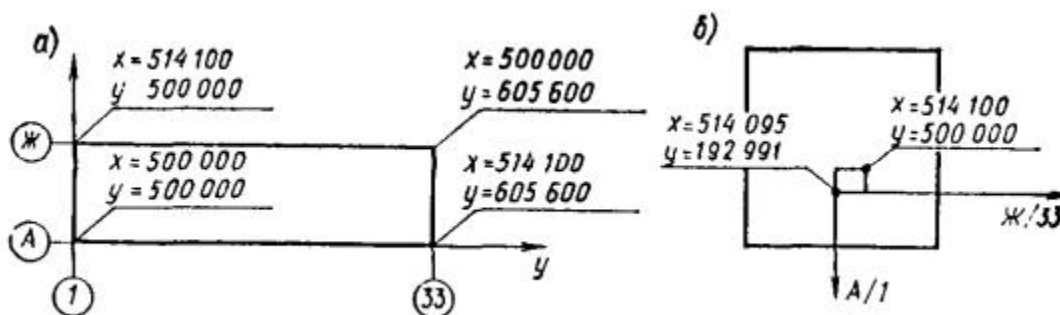
Рис. 14. Редуцирование точек разбивочной сети здания на исходном горизонте
