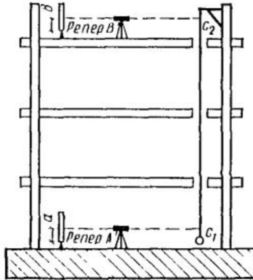
Рис. 18. Передача отметок на монтажный горизонт
