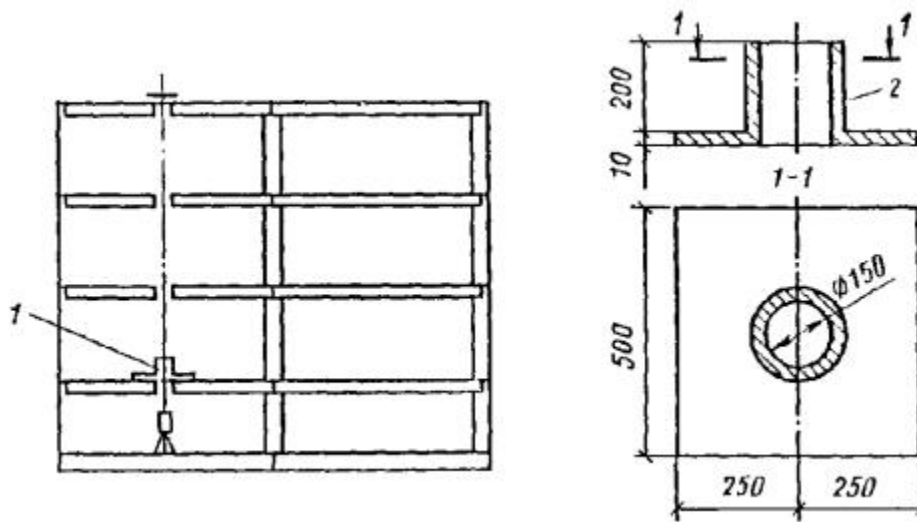
Рис. 16. Ловушка, схема ее установки
