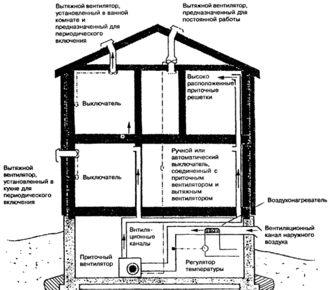
Рисунок 7.2 - Система воздушного отопления с принудительной циркуляцией воздуха, совмещенная с системой механической вентиляции, не присоединенной к системе теплоснабжения
