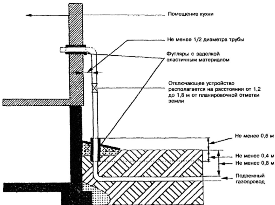
Рисунок 9.1 - Газовый ввод
