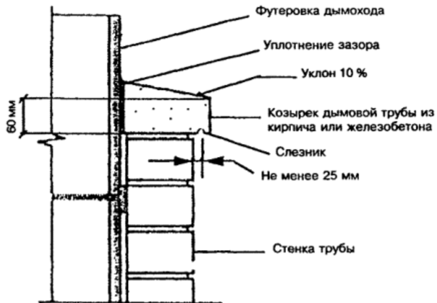
Рисунок 7.7 - Оголовок дымовой трубы
