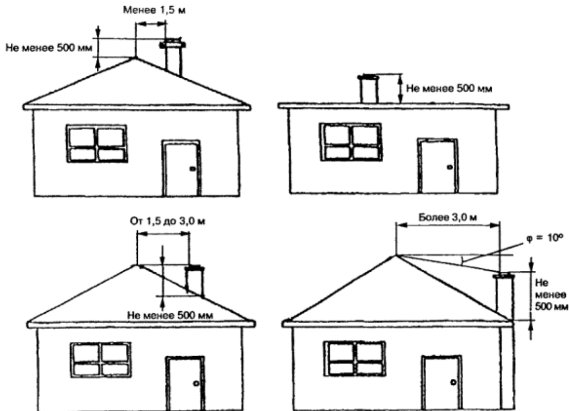
Рисунок 7.9 - Минимальная высота дымовой трубы
