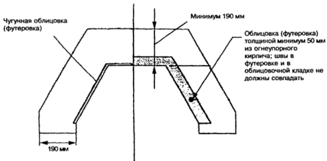
Рисунок 7.5 - Футеровка камина
