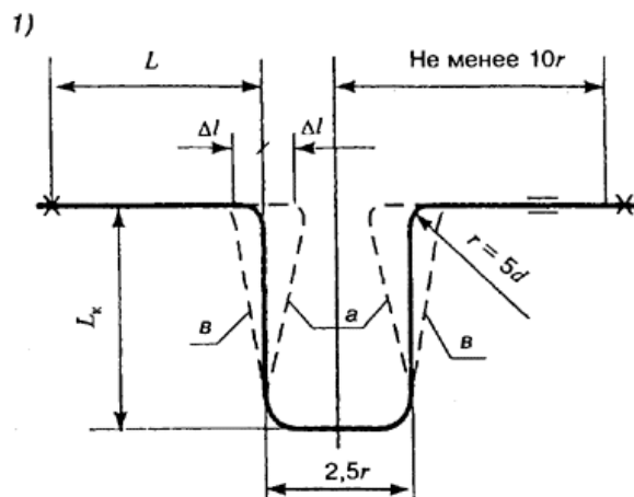
Рисунок 10 - Диаграмма для определения удлинения труб
