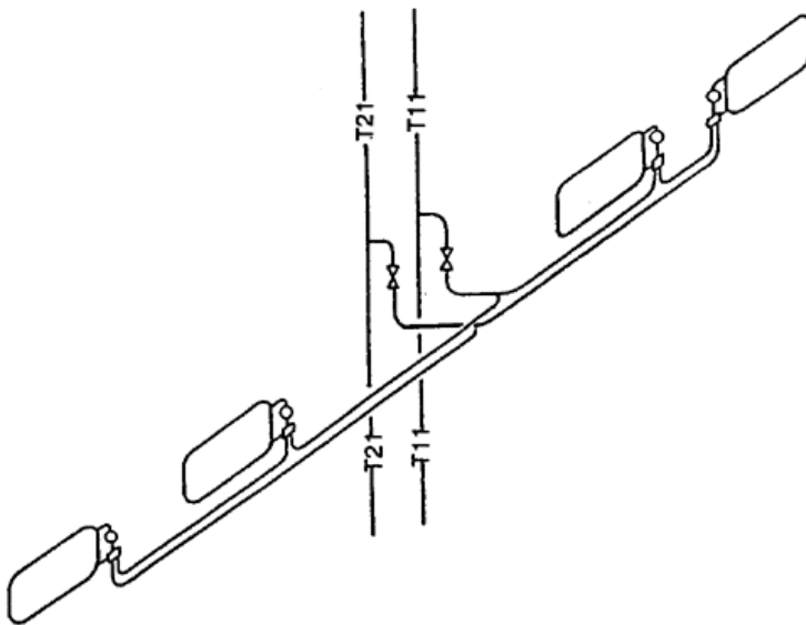
Рисунок 6 - Система отопления с горизонтальными однетрубными ветками для группы последовательно соединенных отопительных приборов
