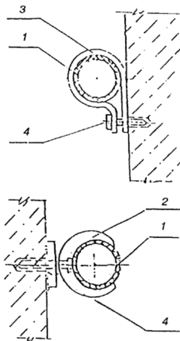
Рисунок 17 - Крепление труб к стенам и перегородкам
