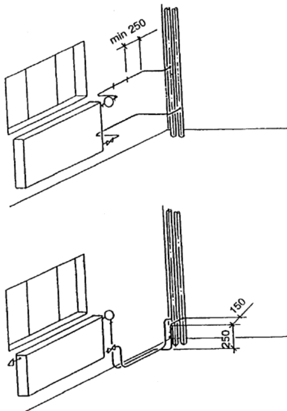
Рисунок 8 - Вариант подсоединения распределительных коллекторов к стоякам из металлополимерных труб
