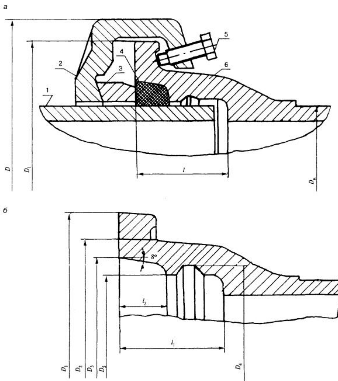
а - раструбное соединение с крепежной струбциной; б - раструб трубы
