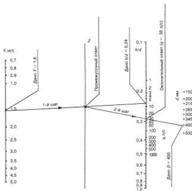
Рисунок В. 1 - Номограмма для выбора диаметра d стеклопластиковых труб в зависимости от расхода q , скорости V и наполнения \frac{d}{2} для самотечного канализационного трубопровода (Z - промежуточная шкала)
