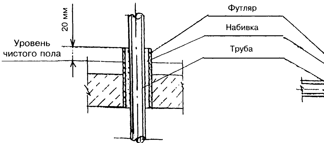
Рисунок 6 — Установка футляров для прохода труб через перекрытия
