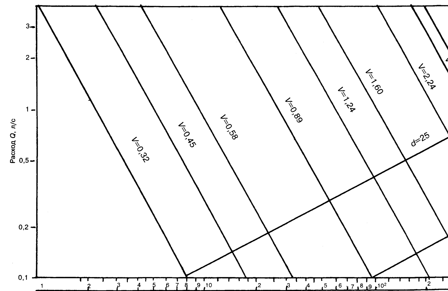
"Рисунок А.1 - Номограмма для приближенного гидравлического расчета водопровода холодной воды из металлополимерных труб по ТУ 2248-001-07629379-96"
