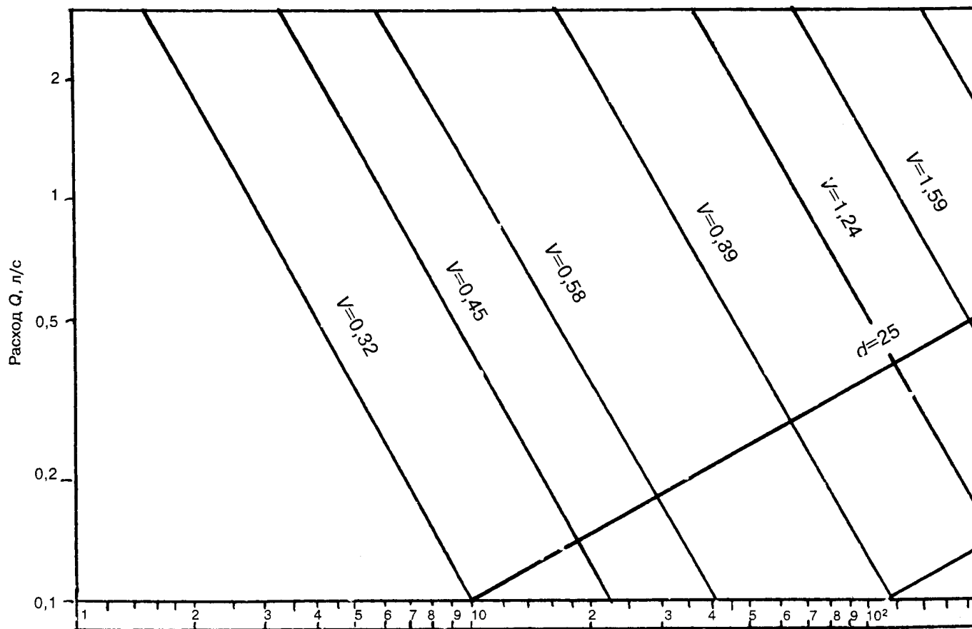
Рисунок А.1 — Номограмма для приближенного гидравлического расчета водопровода холодной воды ТУ 2248-001-076293/9-96
