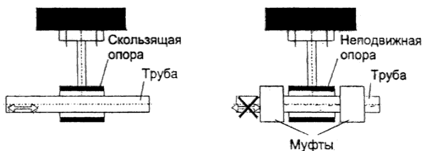
Рис. 4.1. Виды опор
