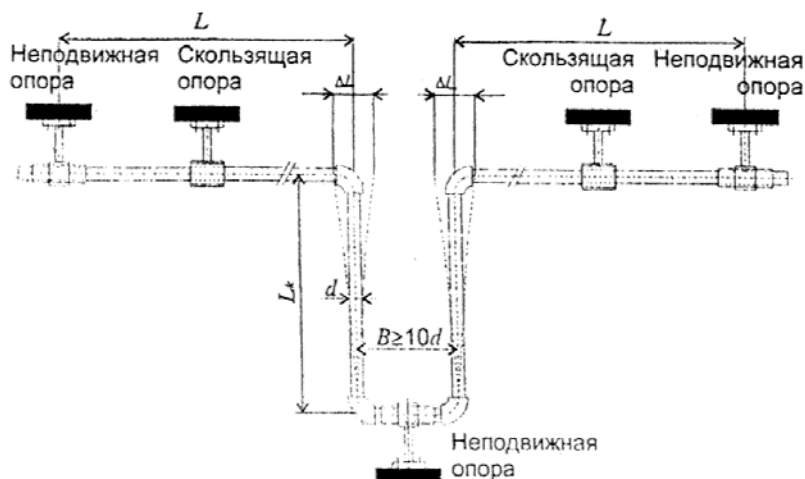
Рис. 2.5. П-образный компенсатор
