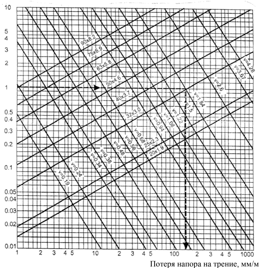
Рис. 2.1. Номограмма для инженерного гидравлического расчета холодного водопровода из труб PPRC (PN10)
