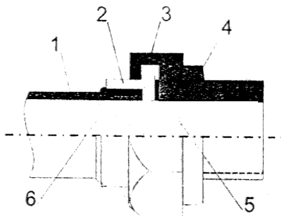
Рис. 5.4. Соединение с накладной гайкой
