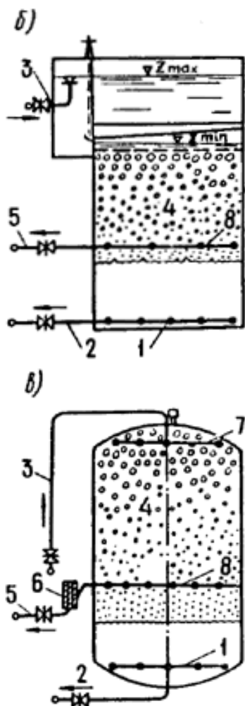
Черт. 30. Фильтры с плавающей пенополистирольной загрузкой
