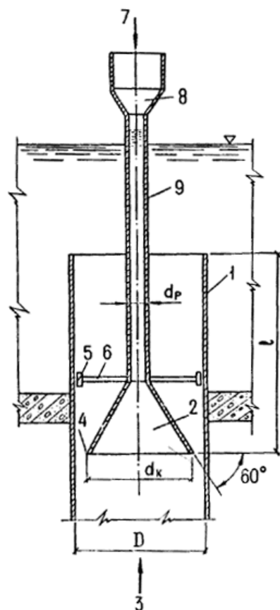
Черт. 5. Диффузорный распределитель (тип III)
