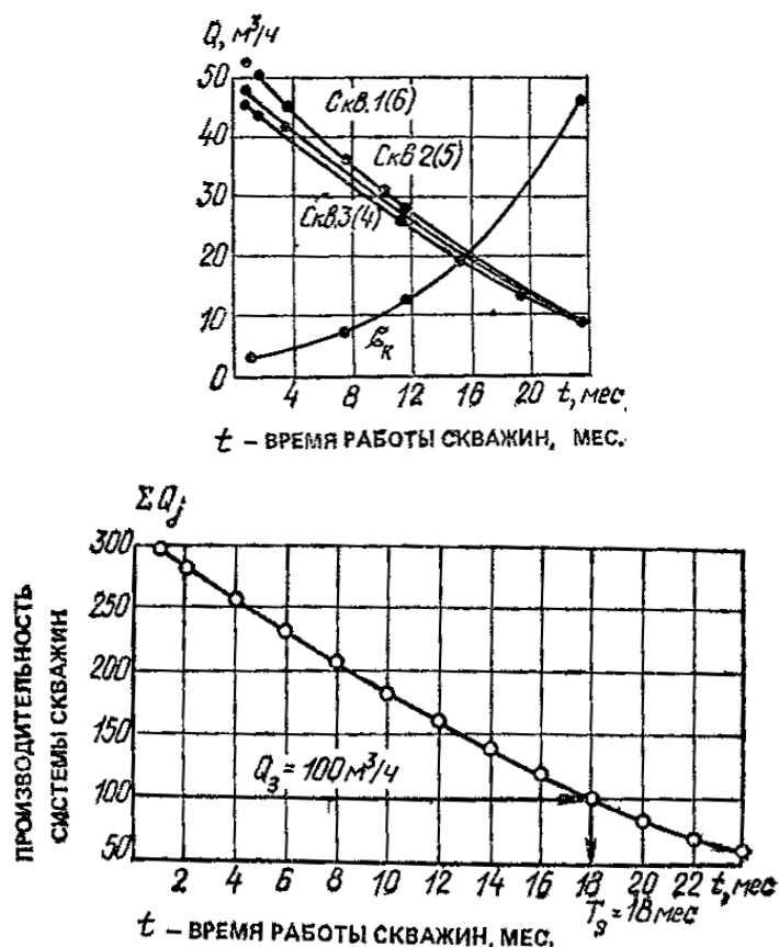
Рис. 107. Расчетные графики изменения во времени \zeta_k(t) , Q_j(t) и \Sigma Q(t) при действии скважин в режиме S_j = \text{const}
