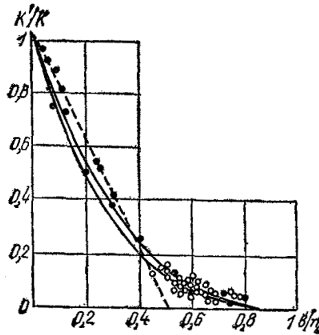
Рис. 58. Графики изменения k^1/k в функции b/n_0
