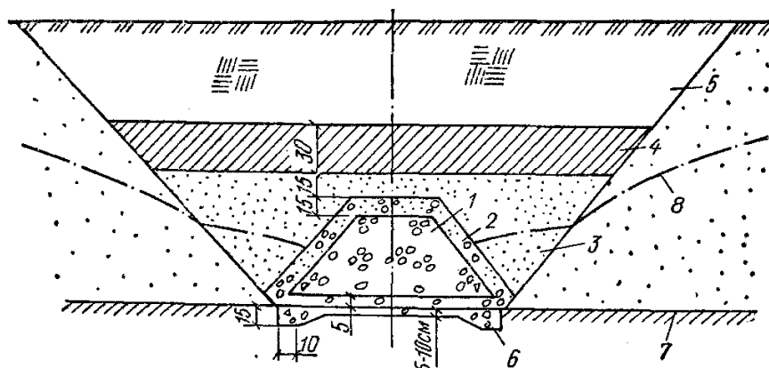
Рис. 15. Каменно-щебеночный водозабор
