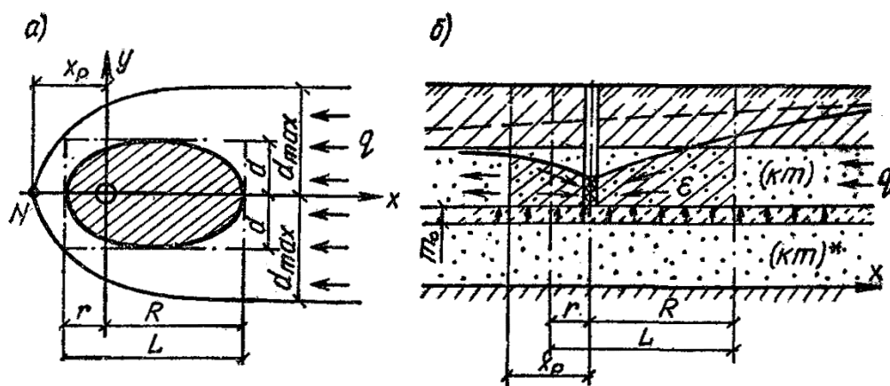
Рис. 85. График для определения протяженности ЗСО ( R и r ) при действии линейного водозабора в изолированном неограниченном пласте
