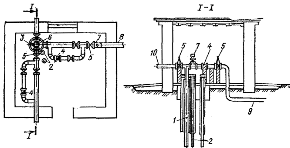
Рис. 57. Схема входного узла скважины двойного назначения (план и разрез I-I)
