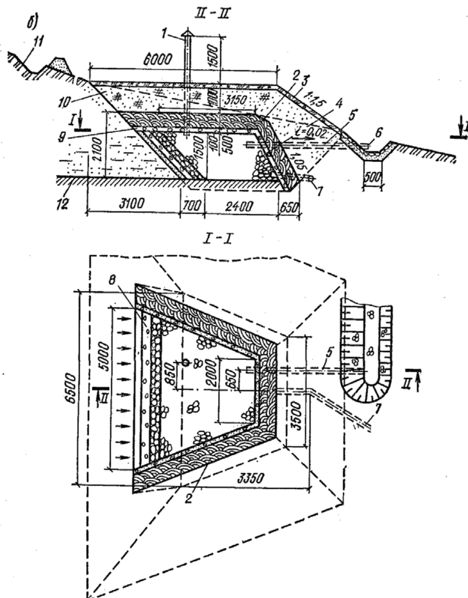
Рис. 45. Глиняно-каменная каптажная камера
