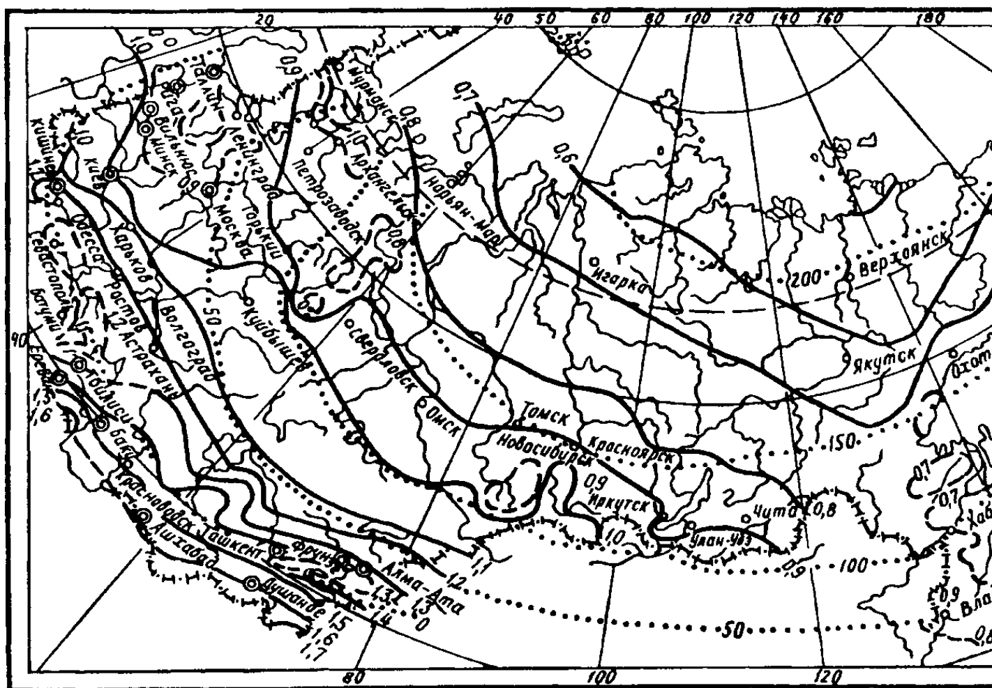
Черт. 3. Климатические коэффициенты для определения величины нагрузки на иловые площадки (сплошные линии) и продолжительности периода намораживания на иловых площадках, дни (точечные линии)
