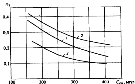
Черт. 2. Зависимость показателя степени n_2 от исходной концентрации взвешенных веществ в городских сточных водах при эффекте отстаивания 1 — 50 %; 2 — 60 %; 3 — 70 %
