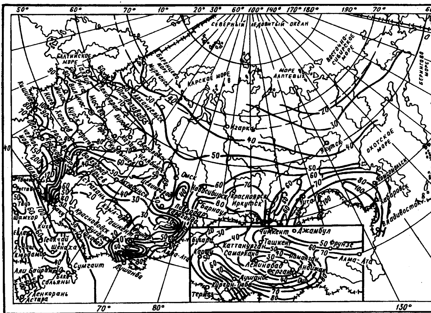
Черт. 1. Значения величин интенсивности дождя q_{20}
