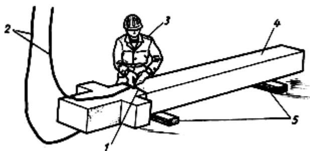
Рис.11. Схема строповки колонны:
