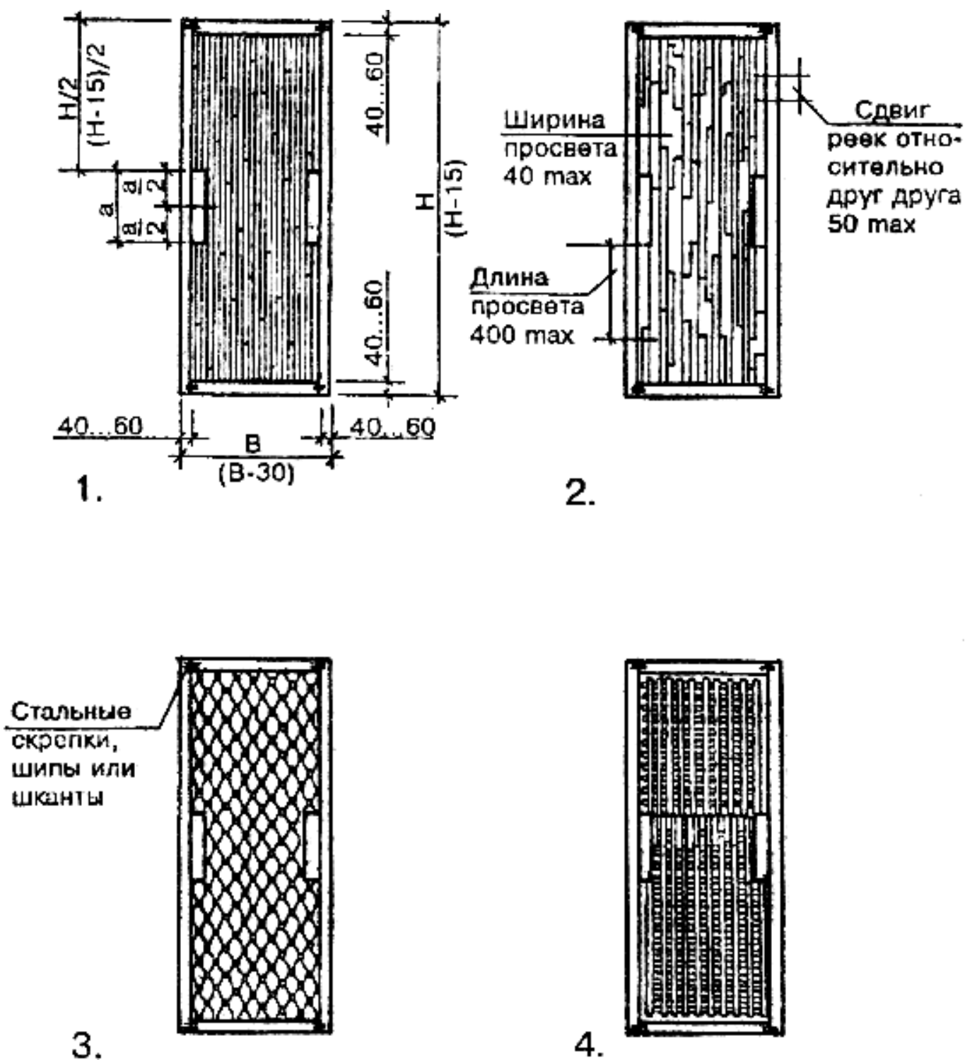
Рис.2. Примеры заполнения щитов дверных полотен:
