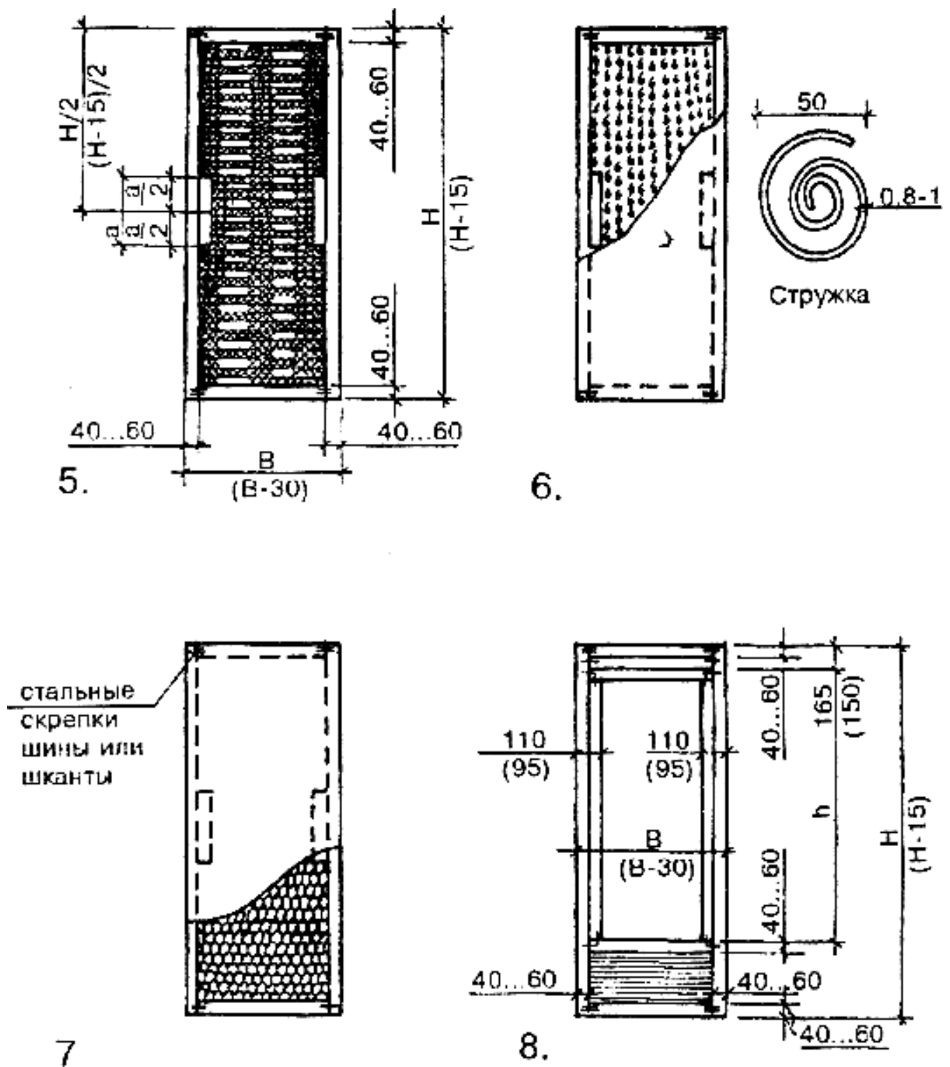
Рис.3. Примеры заполнения щитов дверных полотен (продолжение):
