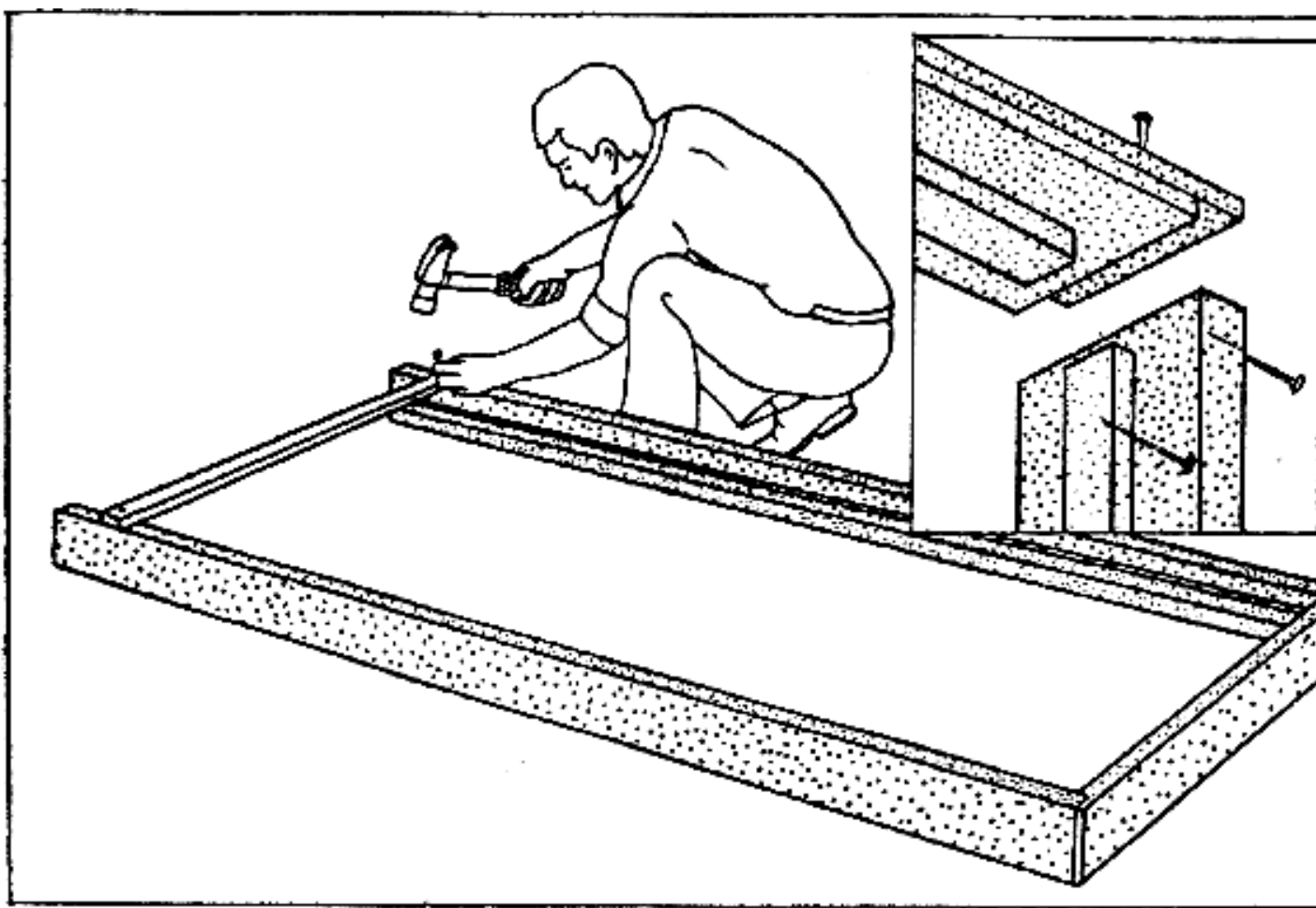
Рис.8. Сборка и установка дверной коробки
