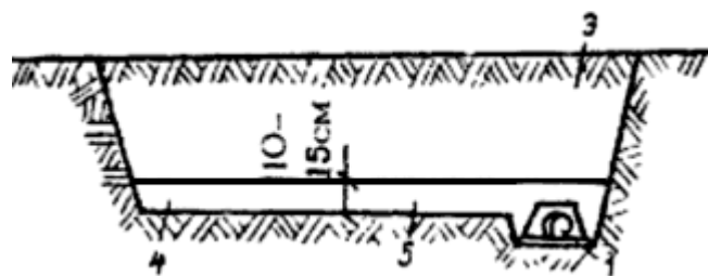
б) Отсыпка песка с трамбовкой пазух
