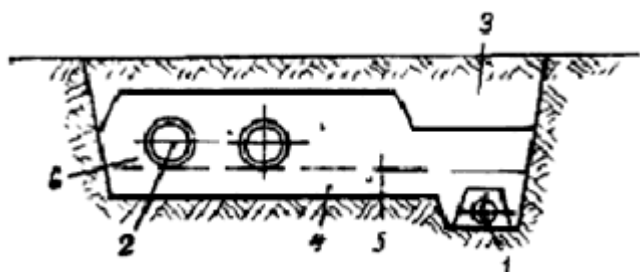
г) Засыпка траншеи
