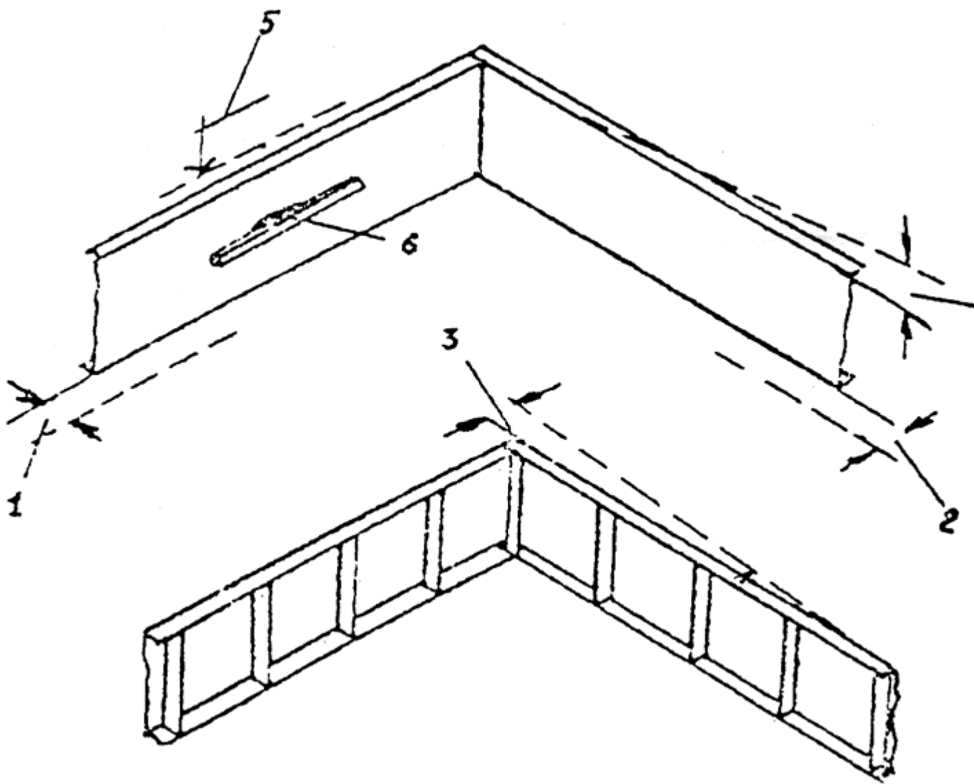
Рис.7. Допустимые отклонения геометрических размеров при установке опалубки:
