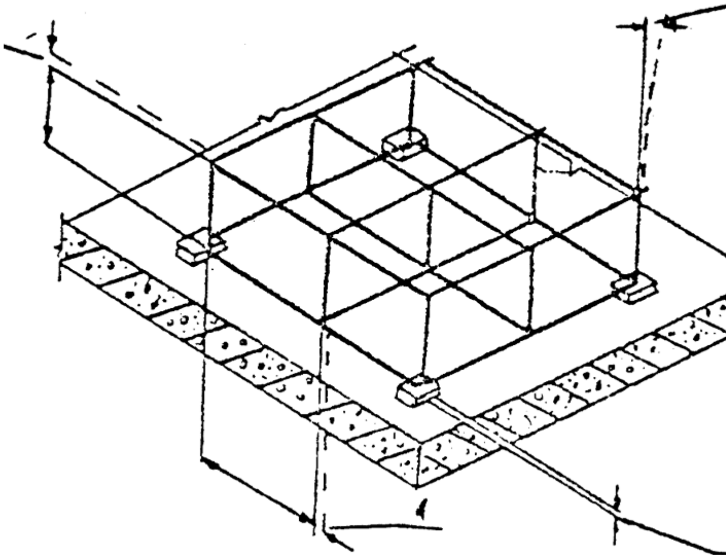
Рис.6. Отклонения геометрических размеров при установке арматуры:
