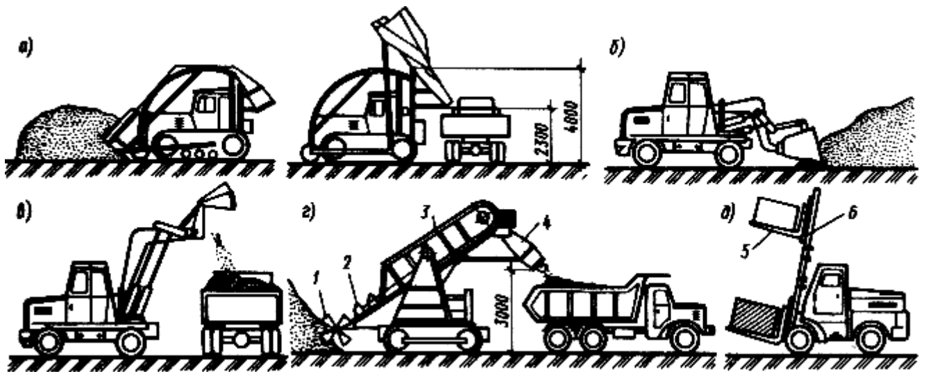
Рис.1. Погрузчики:
