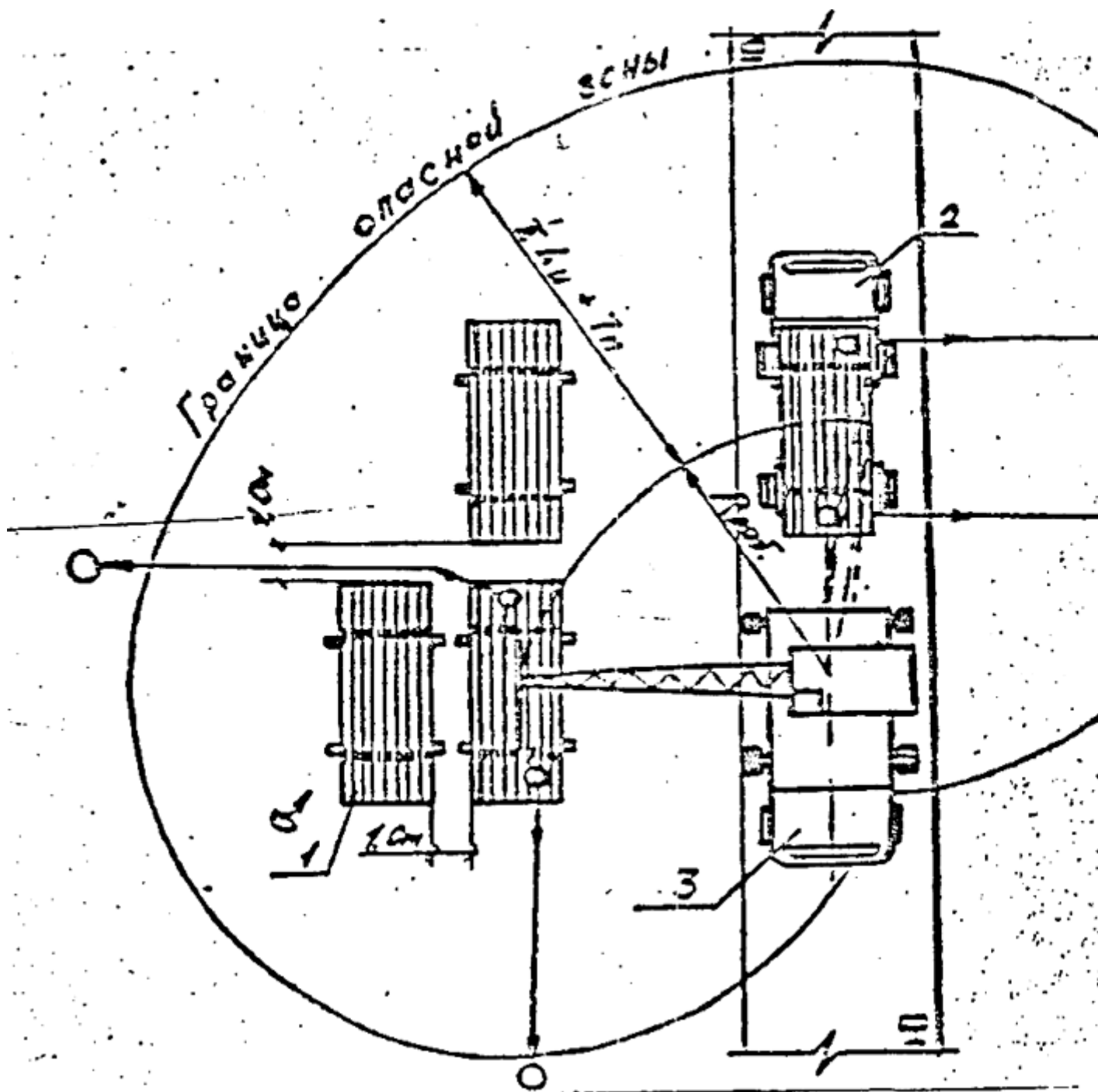
Рис.9. Схемы взаимного расположения грузоподъемного механизма и автомашины при производстве погрузочно-разгрузочных работ
