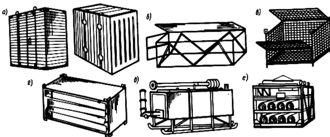
Рис.5. Контейнеры:
