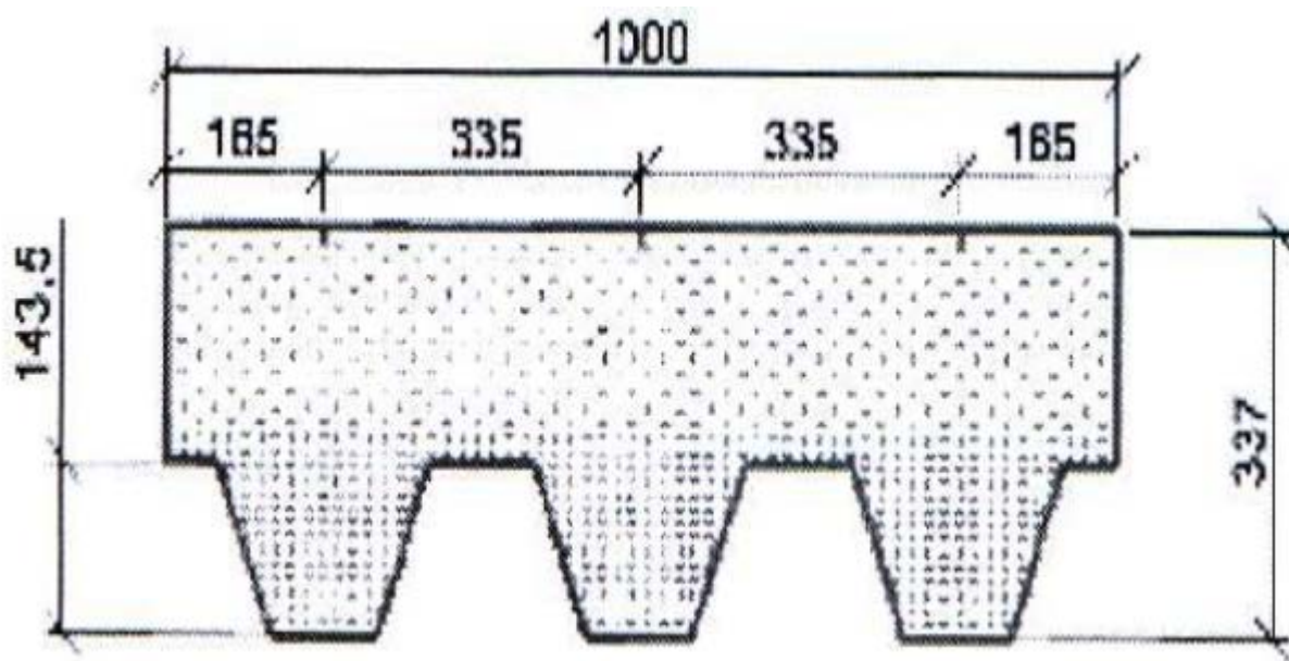
Рис. 2. Форма плитки мягкой кровли Tegola
