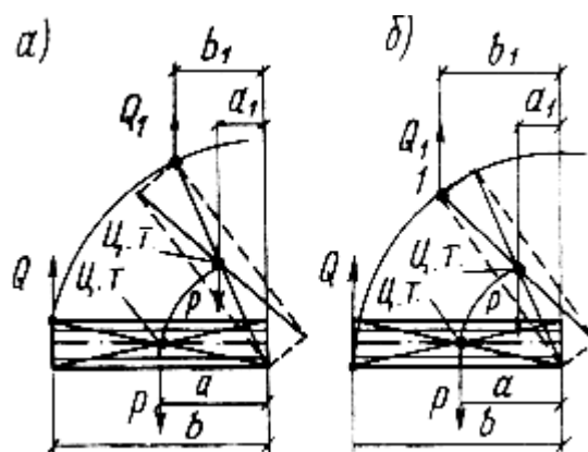
Рис.6. Усилия, приходящиеся на кран при подъеме рулона:
