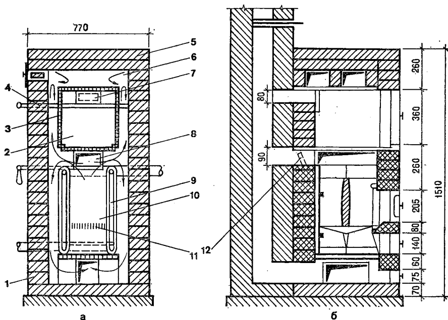
Рис. 5.38. Печь-котел:
