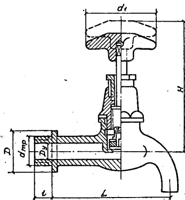
Рис. 9.33. Кран водоразборный настенный типа KB15Д и KB20Д.
