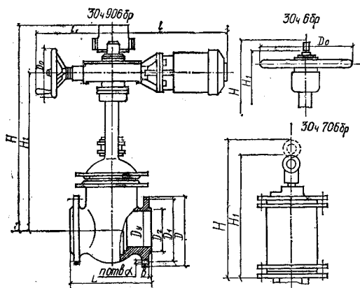
Рис. 9.1. Задвижки чугунные параллельные с выдвижным шпинделем фланцевые.
