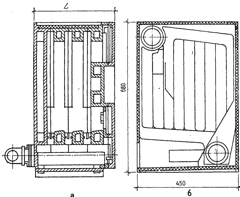
Рис. 5.32. Чугунный секционный водогрейный котел КЧММ-2: а — продольный разрез; б — поперечный разрез.
