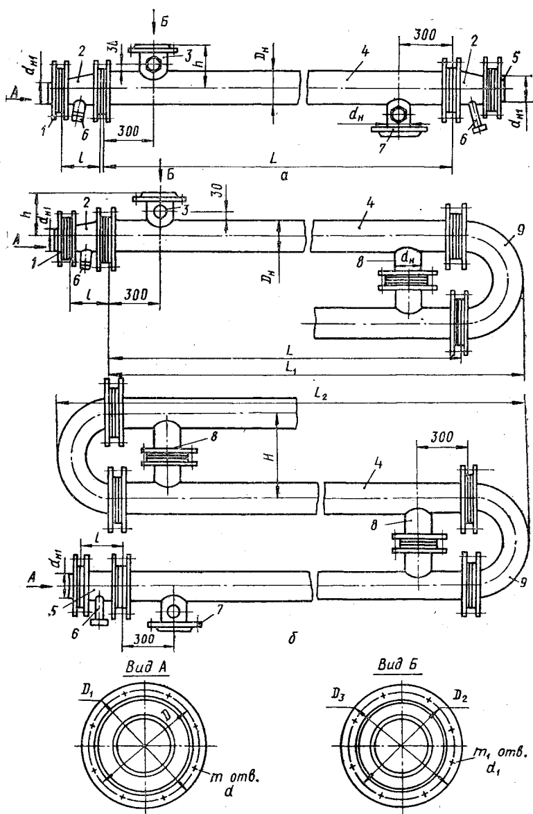
Рис. 4.9. Водно-водяные скоростные секционные подогреватели ОСТ 34-588-68: а — односекционный; б — многосекционные разъемные; 1 — патрубок входа нагретой воды; 2 — конфузор; 3 — патрубок входа греющей воды; 4 — секция; 5 — патрубок входа нагреваемой воды; 6 — штуцер; 7 — патрубок выхода гре- ющей воды; 8 — перемычка; 9 — колено.
