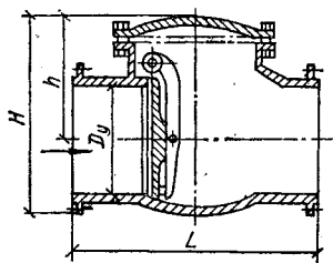
Рис. 9.4. Клапан обратный поворотный чугунный фланцевый.
