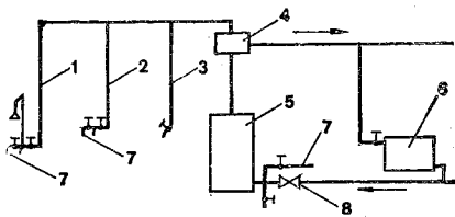
Рис. 5.39. Схема совмещенной системы водяного квартирного отопления и горячего водоснабжения в генераторе теплоты повышенной емкости:
