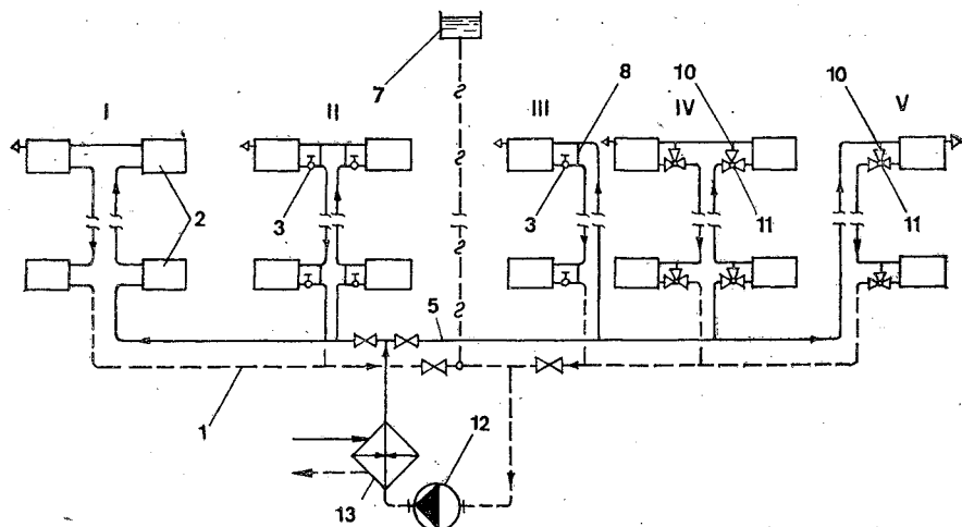
Рис. 5.2. Вертикальные однетрубные насосные системы водяного отопления с верхним расположением подающих магистралей:
