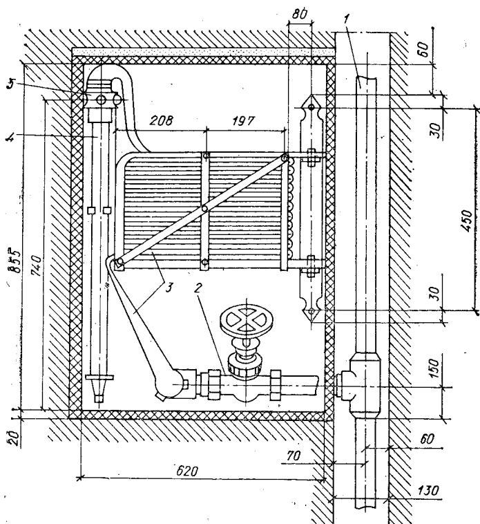
Рис. 2.21. Внутренний пожарный кран:
