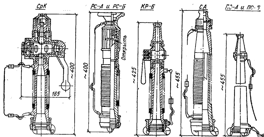
Рис. 2.22. Стволы пожарные ручные.
