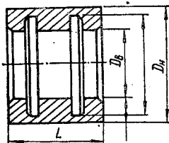
2.35. Размеры, мм, и масса, кг, асбестоцементных муфт типа САМ (ГОСТ 539—80)
