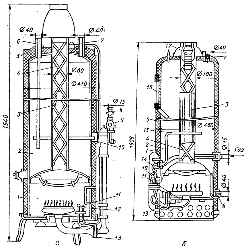
Рис. 4.15. Емкостные газовые водонагреватели:
