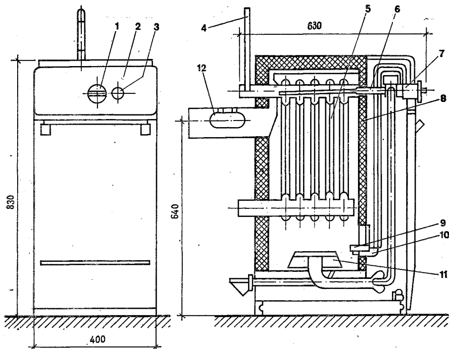
Рис. 5.36. Котел типа АОГВ, работающий на газообразном топливе:
