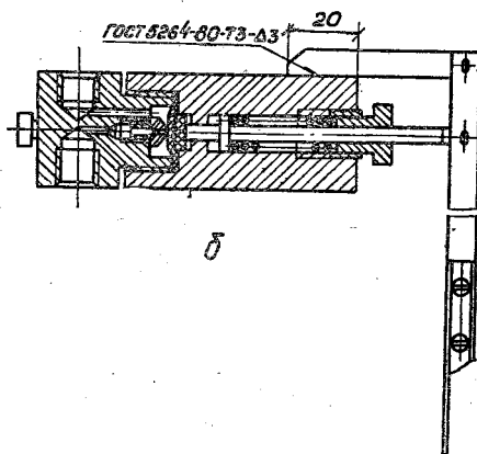
Рис. 9.24. Терморегулятор конструкции Башкирэнерго:
