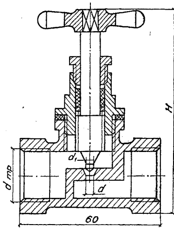
Рис. 9.11. Кран регулирующий дроссельный типа КРД.
