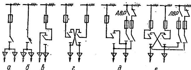
Рис. 8.6. Схемы вводно-распределительных устройств:
