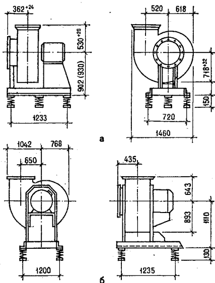
Рис. 6.3. Размеры центробежных вентиляторов Ц4-70 № 8 и 10 (исполнение 1):
