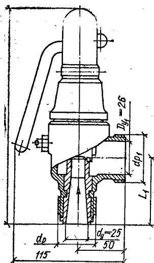
Рис. 9.31. Клапан предохранительный полноподъемный, пружинный, цапковый 17с42нж ( d_p = M39 \times 2 ; d_{p1} = M48 \times 2 ).
