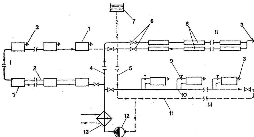
Рис. 5.5. Горизонтальные однотрубные насосные системы водяного отопления:
