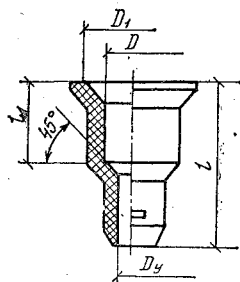
3.27. Размеры, мм, патрубков из ПВХ, ПНП, ПП и ПВХ для присоединения выпусков к унитадам, трапам и чугунным трубам
