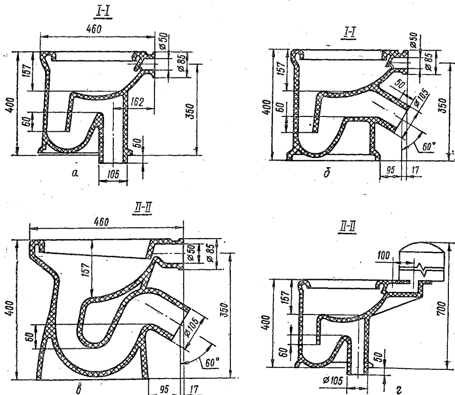
Рис. 3.2. Унитазы тарельчатые:
