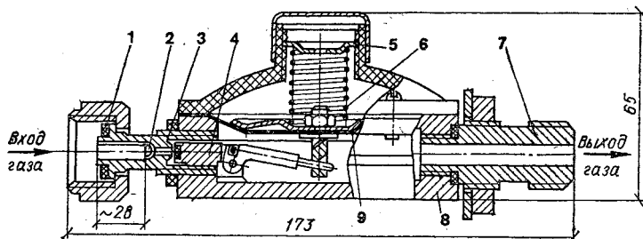
Рис. 9.27. Регулятор давления газа РДСГ-1.2:
