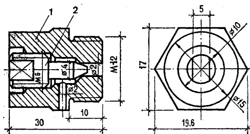
Рис. 5.29. Воздухоспускной кран: 1 — корпус; 2 — игла.
