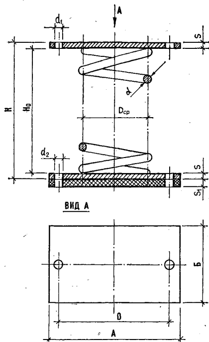
Рис. 6.14. Пружинные виброизоляторы типа ДО.
