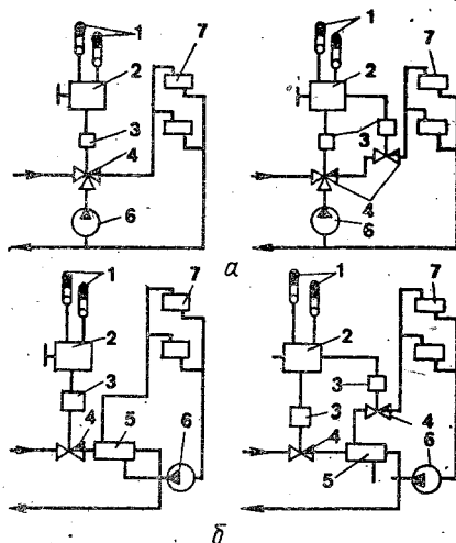
Рис. 9.23. Схема авторегулирования тепловых вводов термосистемой РТК-2216:
