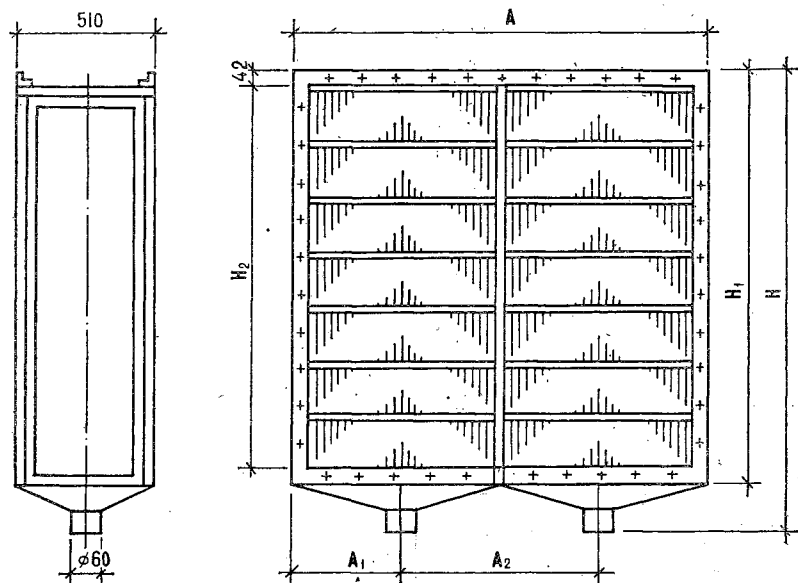
Рис. 6.12. Электрические фильтры типа ФЭ.
