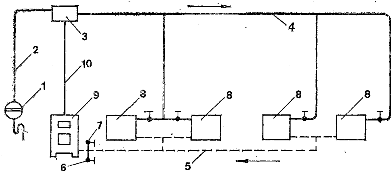
Рис. 5.30. Схема водяного квартирного отопления с прокладкой горячей линии сверху и обратной снизу приборов:
