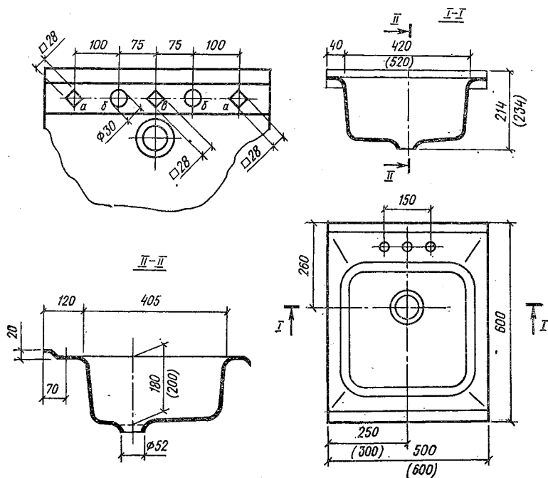
Рис. 3.10. Мойки чугунные эмалированные: без скобок даны размеры для типа МЧ-1-М; в скобках — для типа МЧ-1-Б.
