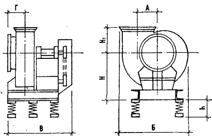
Рис. 6.4. Размеры центробежных вентиляторов Ц4-70 № 8, 10 и 16 (исполнение 6).
