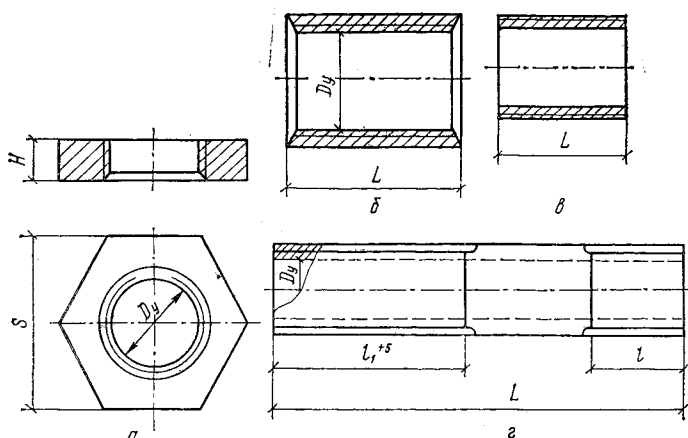
2.28. Стальные контргайки, муфты прямые, короткие, ниппели и стоны
