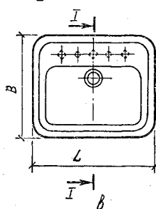
3.38. Размеры, мм, умывальников
