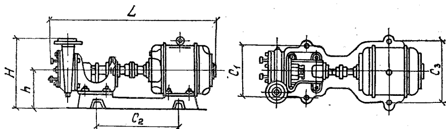
Рис. 2.20. Насос центробежный типа ЦНШ.
