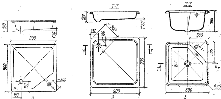
Рис. 3.12. Поддон душевой чугунный эмалированный типов: а — мелкий ПДЧМ 800; б — мелкий ПДЧМ 900; в — глубокий ПДЧГ 800.
