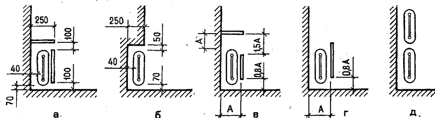
Рис. 5.23. Размещение отопительных приборов:
