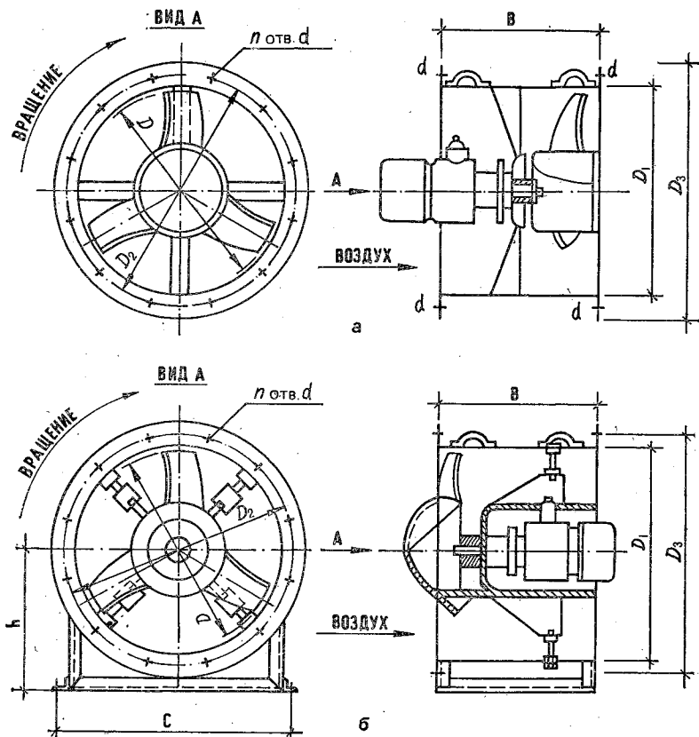
Рис. 6.7. Осевые вентиляторы 06-300 (см. табл. 6.9):
