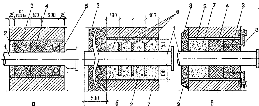
Рис. 2.5. Ввод водопровода через фундамент здания:
