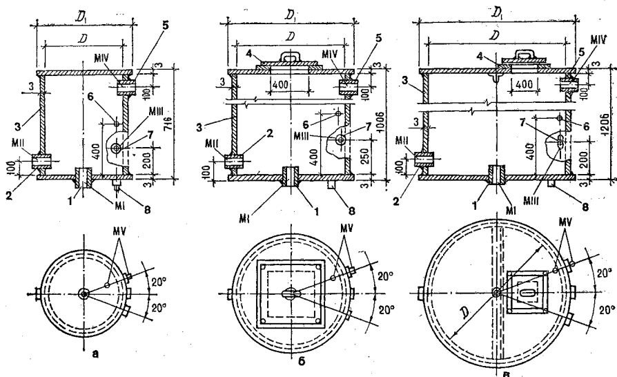
Рис. 5.10. Расширительные баки серии ЕО:
