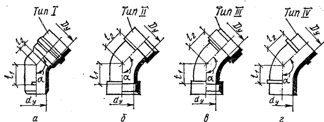
3.29. Размеры, мм, отводов по ГОСТ 22689.9—77 из ПВП, ПП и ПВХ (а), из ПВП ПНП и ПП (б и в), из ПВП (г)
