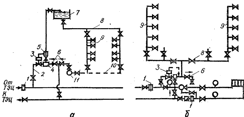
Рис. 4.3. Открытая система горячего водоснабжения:
