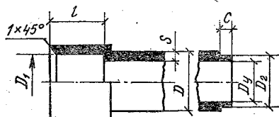
3.18. Размеры, мм, фасонных частей типа II с раструбами и гладкими концами
