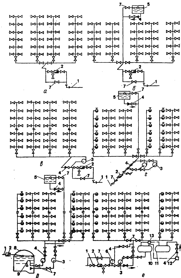
Рис. 2.2. Схемы внутренних водопроводов жилых и общественных зданий:
