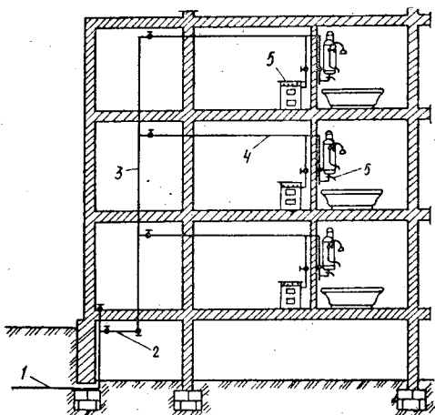
Рис. 7.4. Внутридомовая сеть газопровода:
