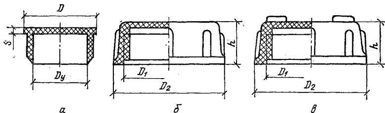
3.36. Размеры, мм, заглушек по ГОСТ 22689.16—77 из ПВХ, ПП и ПВХ при соединении по типу I (а) и по типу III (б и в)
