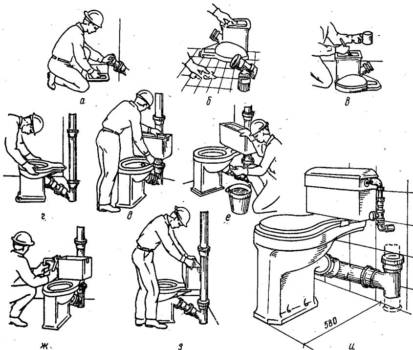
Рис. 3.24. Последовательность установки унитаза с косым выпуском — а...з и его монтажное положение — и.
