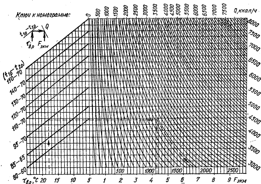
Рис. 5.14. Номограмма для определения теплоотдачи чугунных, колончатых стальных отопительных радиаторов, конвекторов типа КП, ребристых труб и регистров из стальных гладких труб.
