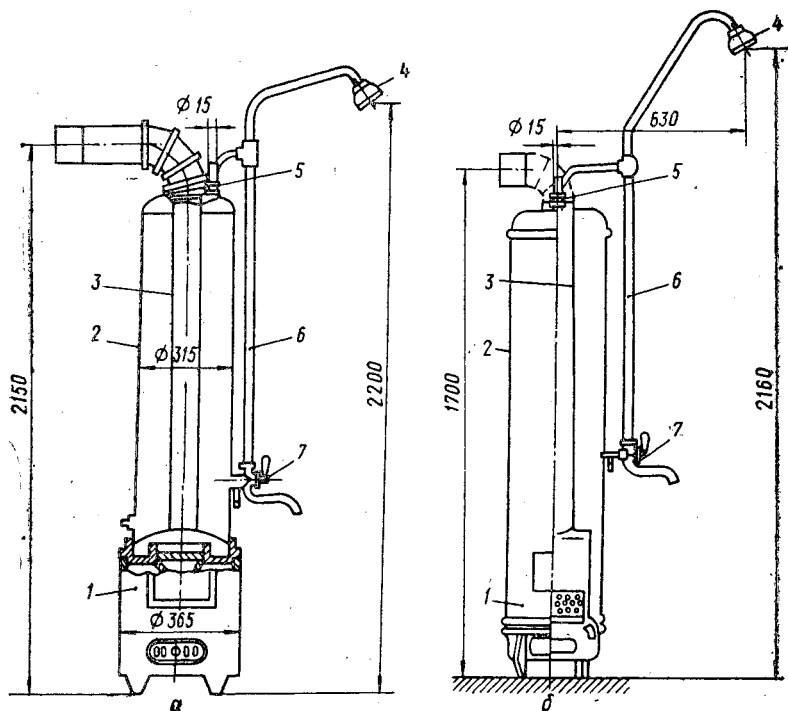
Рис. 4.13. Колонка водогрейная для ванн:
