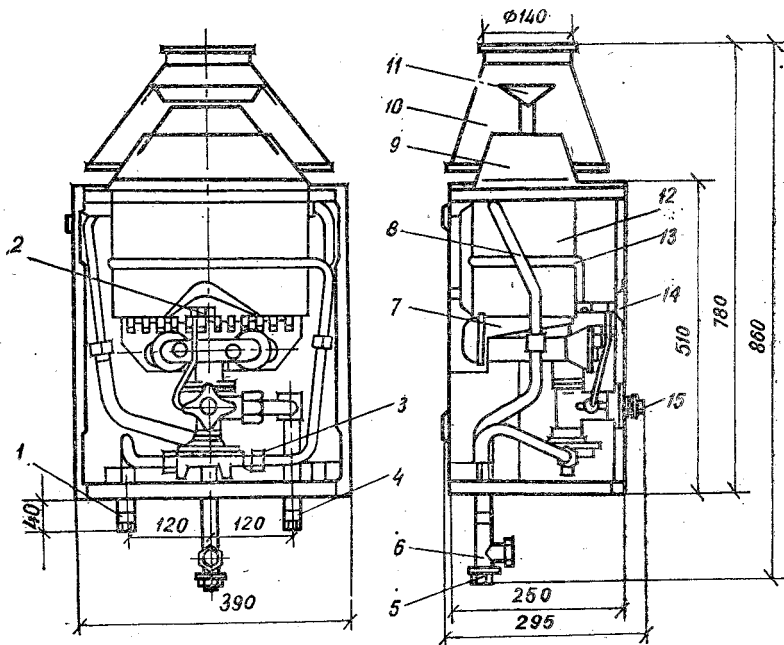
Рис. 4.14. Водонагреватель проточный газовый ВПГ-18-1-3-II:
