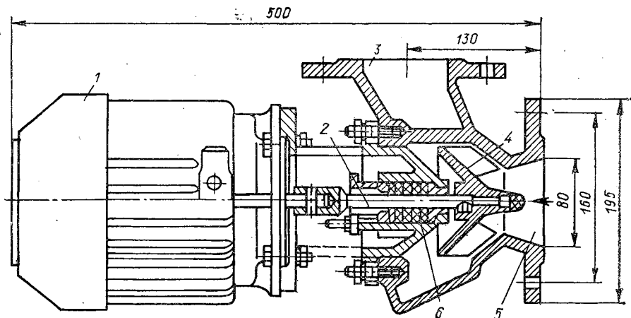
Рис. 2.19. Циркуляционные насосы типа ЦНИПС 20, 10:
