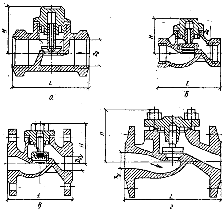
Рис. 9.3. Клапаны обратные подъемные:
