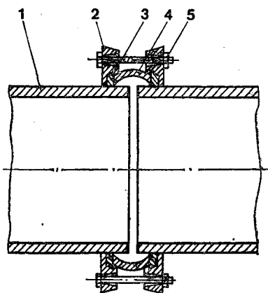
Рис. 2.8. Общий вид соединения асбестоцементных труб при помощи фланцев и чугунных муфт:
