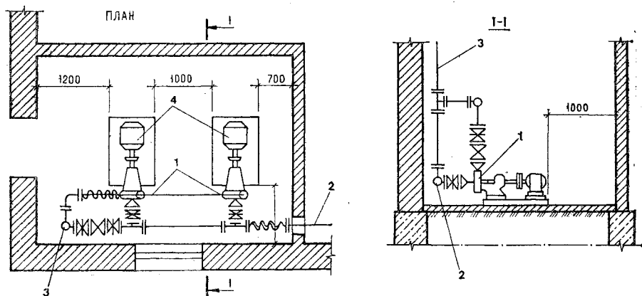
Рис. 2.13. Монтажные схемы насосных установок:
