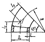
2.29. Размеры, мм, и масса, кг, стальных бесшовных приварных крутоизогнутых отводов (ГОСТ 17375—83)
