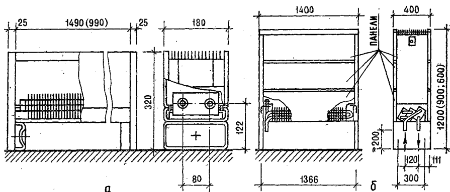
Рис. 5.20. Конвекторы напольные островные стальные с кожухом:
