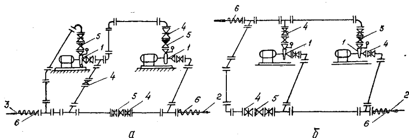
Рис. 2.12. Установка повысительных насосов:
