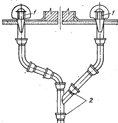
Рис. 3.29. Компенсирующий стык: 1 — водосточная воронка; 2 — компенсирующие стыки.
