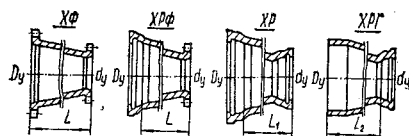
2.34. Размеры, мм, и масса, кг, чугунных водопроводных переходов (ГОСТ 5525—61)
