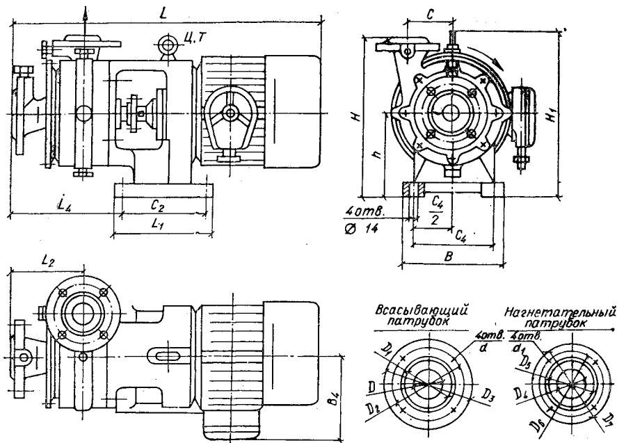
Рис. 2.15. Насосы центробежные консольные типа КМ ПО Архимедмаш.
