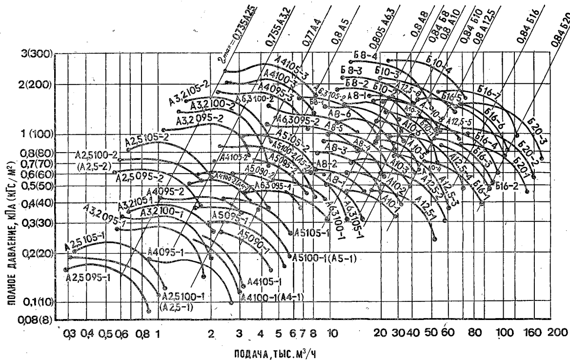
Рис. 6.8. Сводный график для подбора центробежных вентиляторов:
