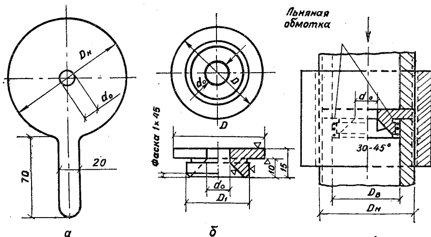
Рис. 4.8. Дроссельные шайба (а) и втулка (б).
