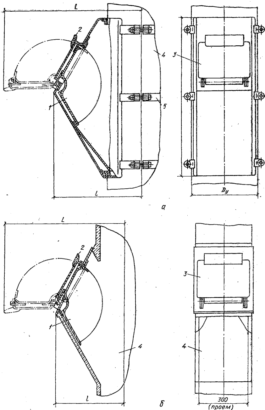
Рис. 3.32. Клапаны загрузочные: а — навесной типа КН, б — встраиваемый типа КВ; 1 — ковш; 2 — ручка; 3 — крышка; 4 — ствол мусоропровода; 5 — хомут.
