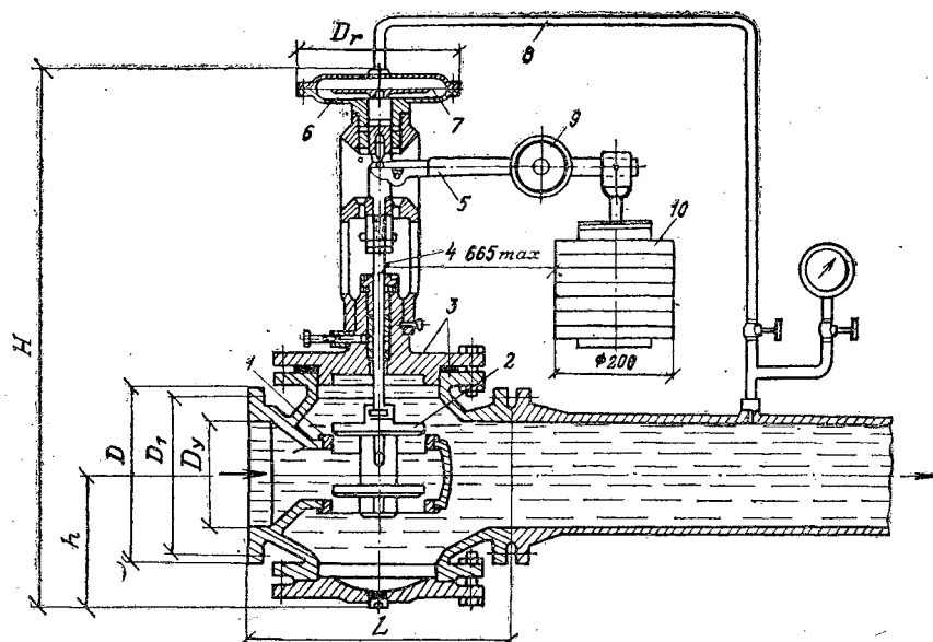
Рис. 9.6. Регулятор давления прямого действия:
