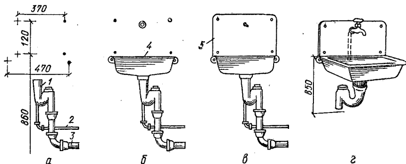
Рис. 3.22. Последовательность установки раковины — а...в и ее монтажное положение — г:
