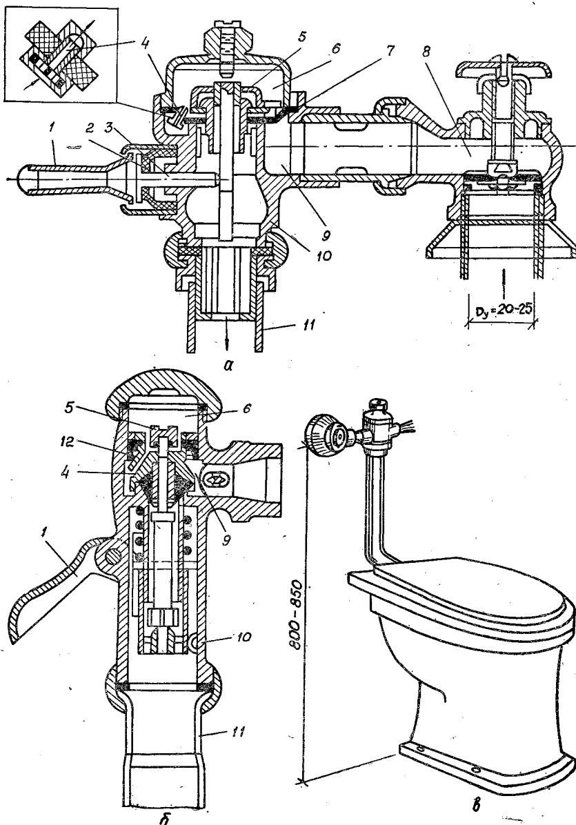
Рис. 9.35. Полуавтоматические смывные краны:
