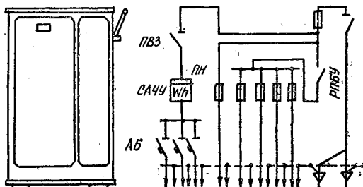
Рис. 8.9. Общий вид и схема ВРУ серии ШВ:
