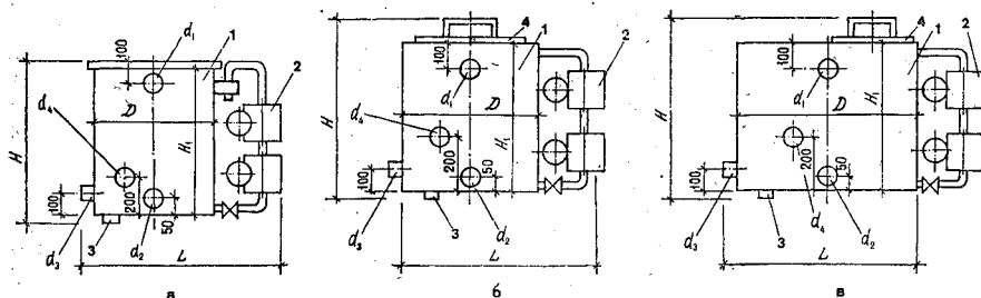
Рис. 5.9. Расширительные баки по серии 3.903—10 типов А16В041 (а), А16В042 (б) и А16В043 (в):
