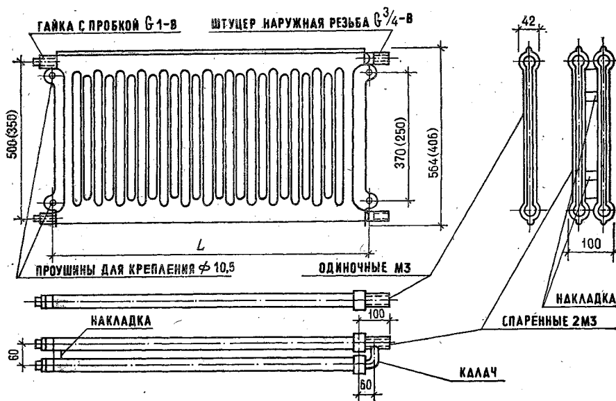
Рис. 5.15. Радиаторы стальные панельные типа РСВ.
