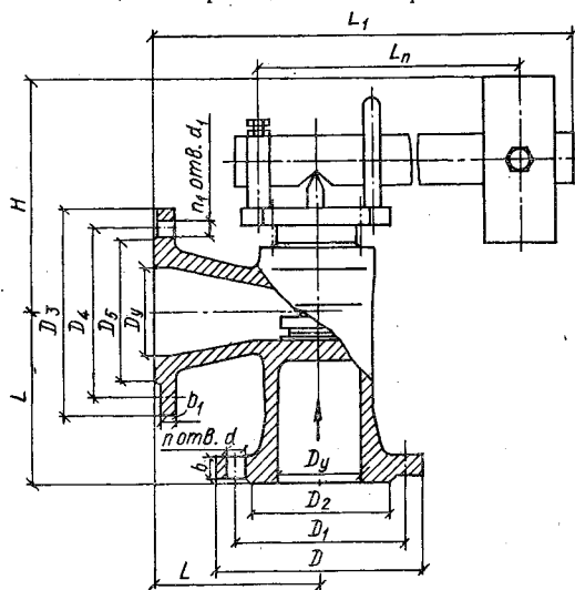
9.26. Размеры, мм, и масса, кг, одинарных предохранительных клапанов 17кч36р (см. рис. 9.29)
