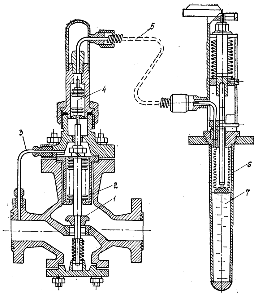
Рис. 9.19. Регулятор-температуры типа РТ:
