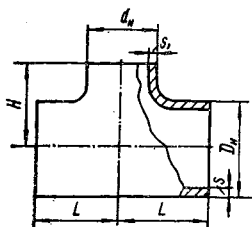
2.30. Размеры, мм, и масса, кг, стальных бесшовных приварных тройников (ГОСТ 17376—83)
