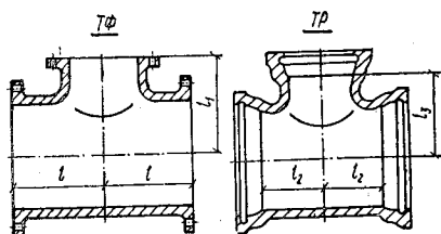
2.32. Размеры, мм, и масса, кг, чугунных тройников и крестов (ГОСТ 5525—61)
