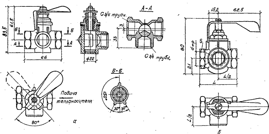
Рис. 9.12. Кран регулирующий трехходовой типа КРТ; а — из ковкого чугуна с D_y = 20 мм; б — латунный.
