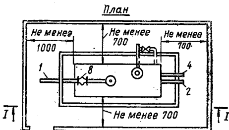
Рис. 2.9. Оборудование водонапорного бака:
