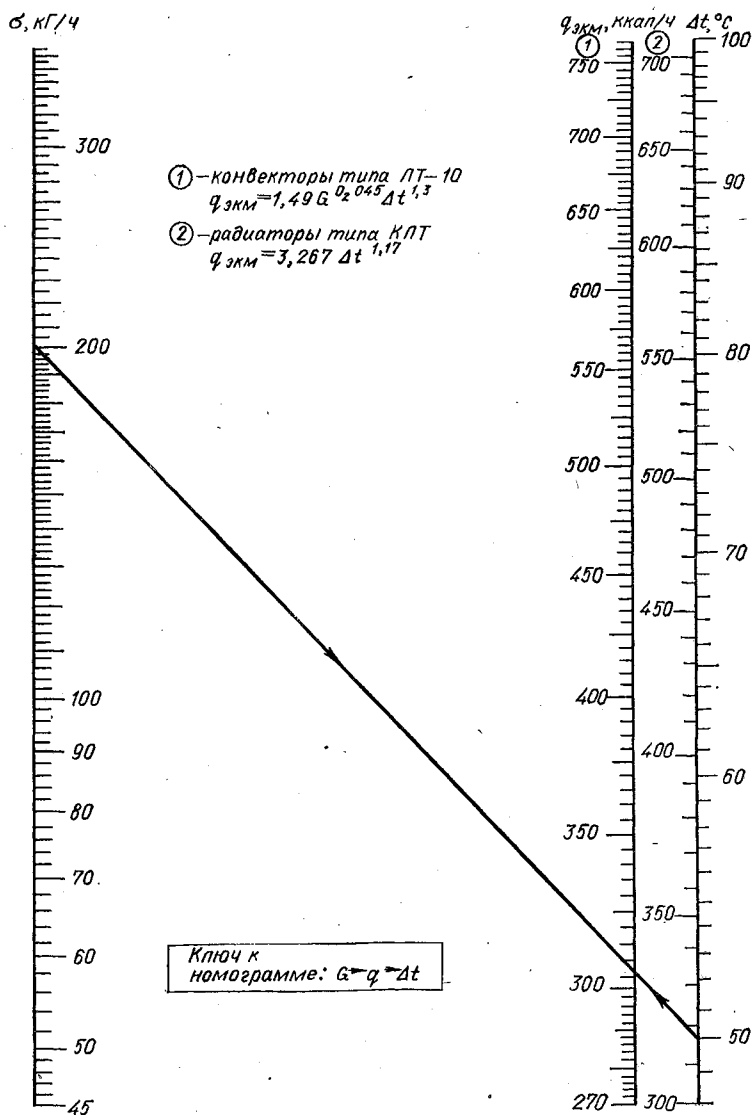
Рис. 5.18. Номограмма для определения теплоотдачи 1 экм стальных листотрубных радиаторов КЛТ и конвектора марки ЛТ-10.
