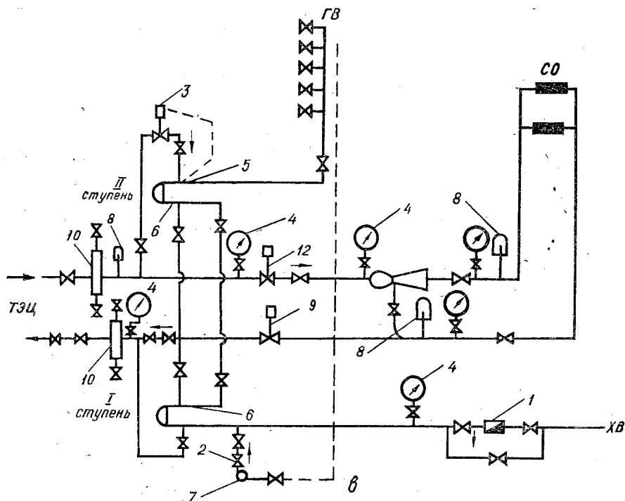
Рис. 4.4. Схемы присоединения водонагревателей к тепловым сетям, устраиваемые в тепловых пунктах:
