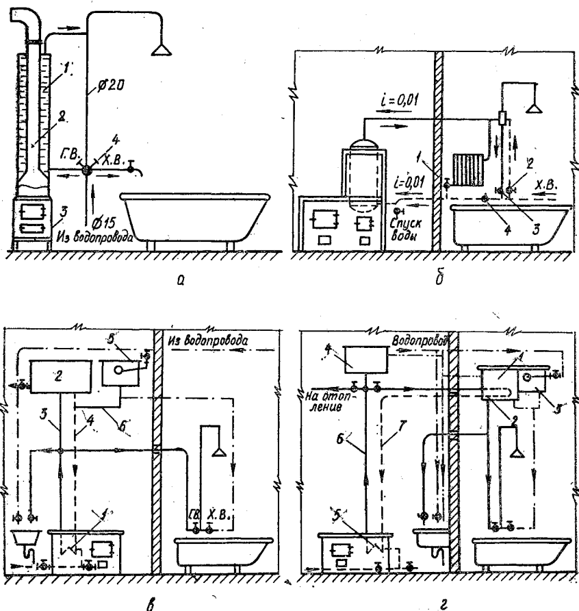
Рис. 4.12. Местные системы горячего водоснабжения:
