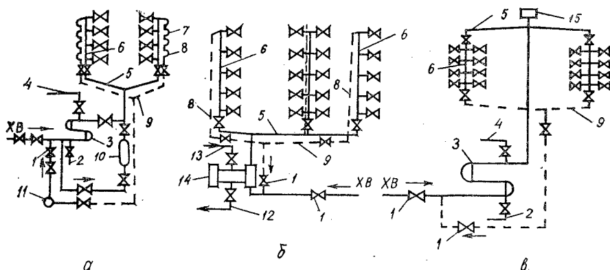
Рис. 4.2. Закрытая система горячего водоснабжения:
