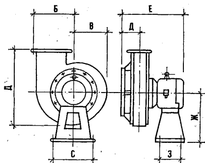
6.7. Центробежные вентиляторы высокого давления Ц10-28
