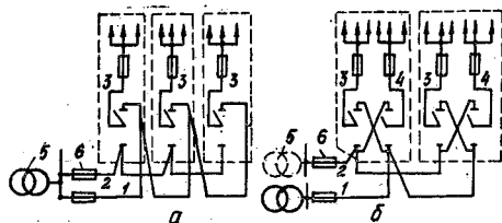
Рис. 8.2. Схемы электроснабжения жилых домов до пяти этажей с электроплитами:
