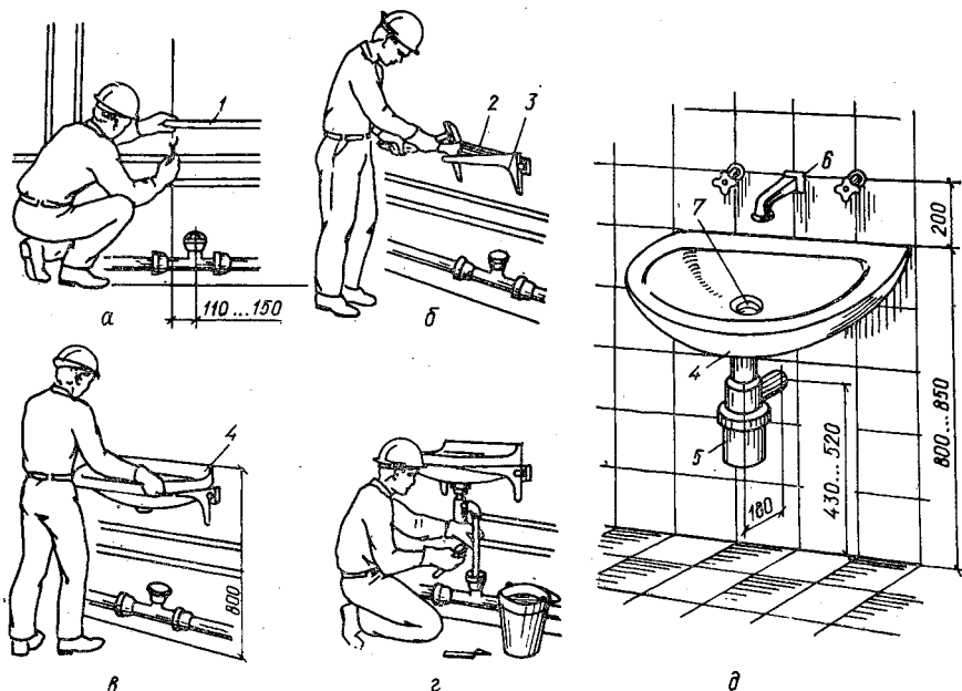
Рис. 3.18. Последовательность установки умывальника — а...г и его монтажное положение д:
