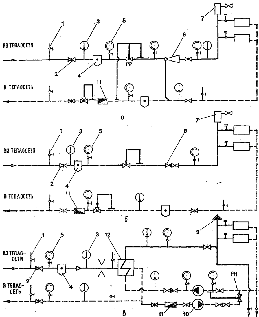
Рис. 5.7. Схемы узлов присоединения систем водяного отопления к тепловым сетям: а — с элеватором; б — непосредственно, без подмешивания; в — независимое через подогреватель; 1 — штуцер с краном для манометра; 2 — задвижка; 3 — термометр; 4 — грязевик; 5 — манометр; 6 — элеватор; 7 — воздухоотборник; 8 — обратный клапан; 9 — кран воздушный; 10 — насос; 11 — водомер; 12 — подогреватель; PP — регулятор расхода; РД — регулятор давления; РН — регулятор напора прямого действия; РДН — регулятор давления непрямого действия.
