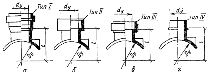
3.28. Размеры, мм, седельчатых патрубков по ГОСТ 22689.8—77 из ПВХ, ПП и ПВХ(а), из ПВХ, ПНП и ПП (б и в), из ПВХ (г)
