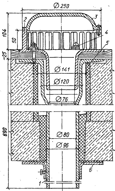
Рис. 3.29. Компенсирующий стык: 1 — водосточная воронка; 2 — компенсирующие стыки.
