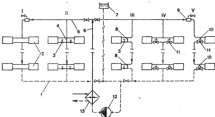
Рис. 5.3. Вертикальные однотрубные насосные системы водяного отопления с нижним расположением обеих магистралей и П-образными стояками:
