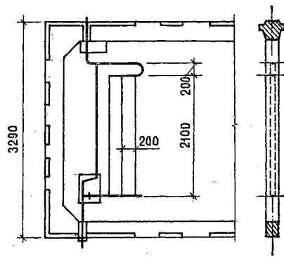
ПЕРЕГОРОДОЧНАЯ ПАНЕЛЬ
