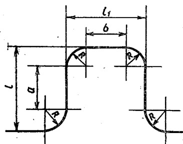
Рис. 4.5. П-образный компенсатор.
