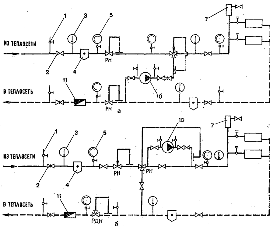
Рис. 5.8. Схемы узлов присоединения систем водяного отопления к тепловым сетям с насосом на перемычке (а) и с насосом на подающем трубопроводе (б) (обозначения 1—11, РР, РД, РН и РДН см. рис. 5.7).
