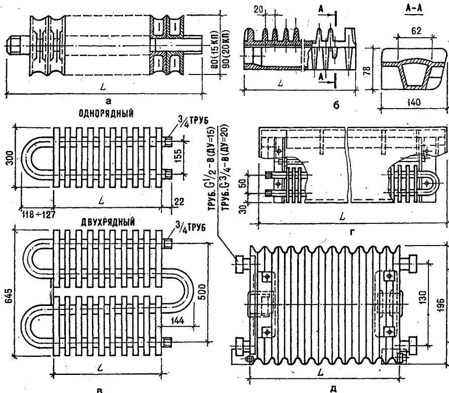
Рис. 5.19. Конвекторы:
