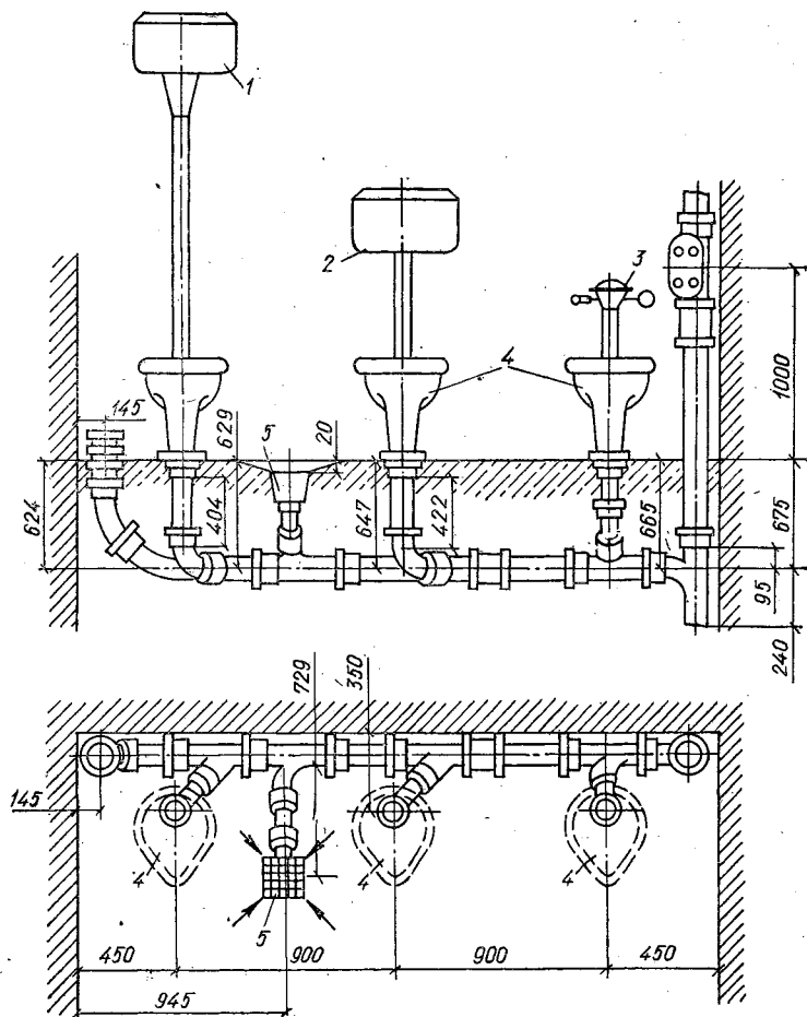
Рис. 3.25. Установка унитаза с прямым выпуском:
