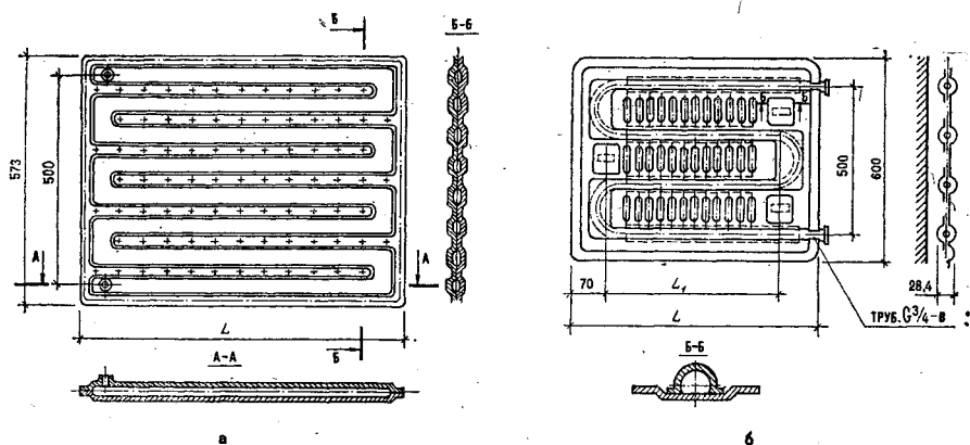
Рис. 5.16. Радиаторы стальные панельные типа РСГ (а) и листотрубные марки КЛТ (б).
