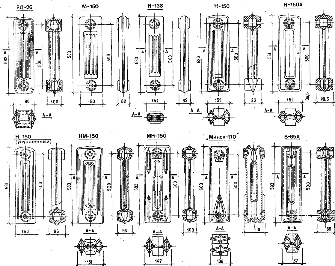
Рис. 5.13. Радиаторы отопительные чугунные.
