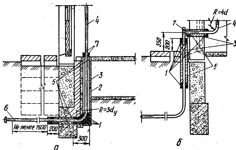
Рис. 7.5. Ввод газопровода в здание:
