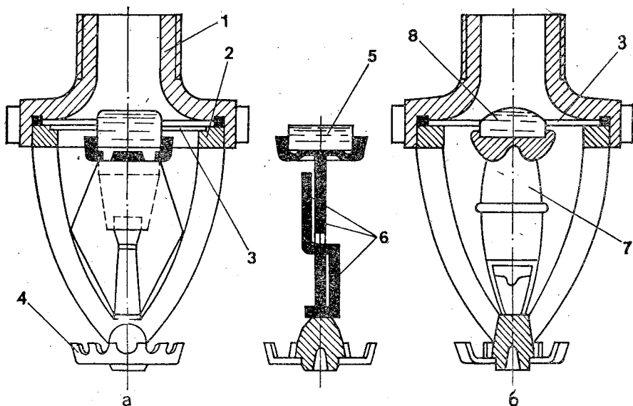
Рис. 2.23. Спринклеры:
