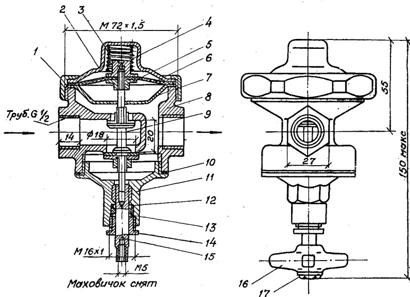
Рис. 9.8. Квартирный регулятор давления:
