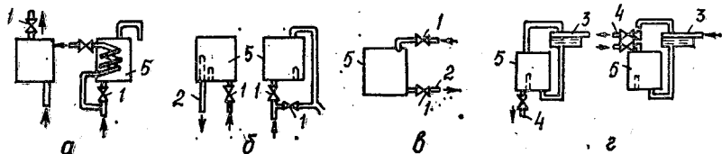
Рис. 8.4. Типы электроводонагревателей:
