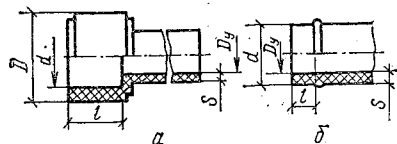
3.20. Размеры, мм, фасонных частей типа IV с гладкими концами
