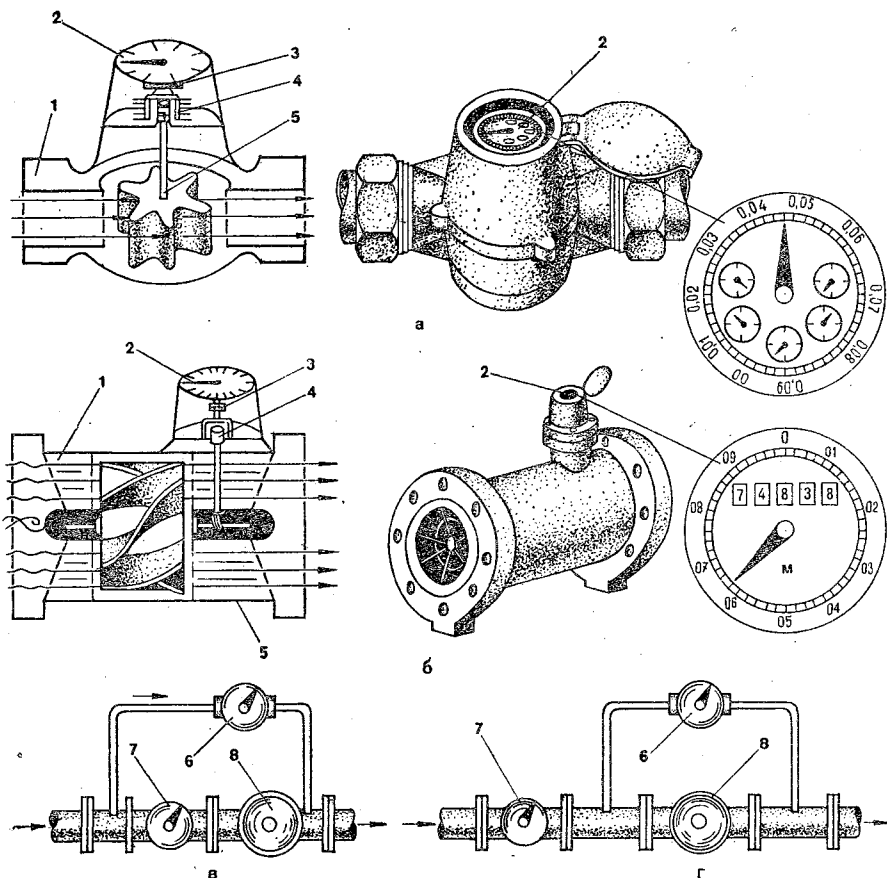
Рис. 2.7. Счетчики воды:
