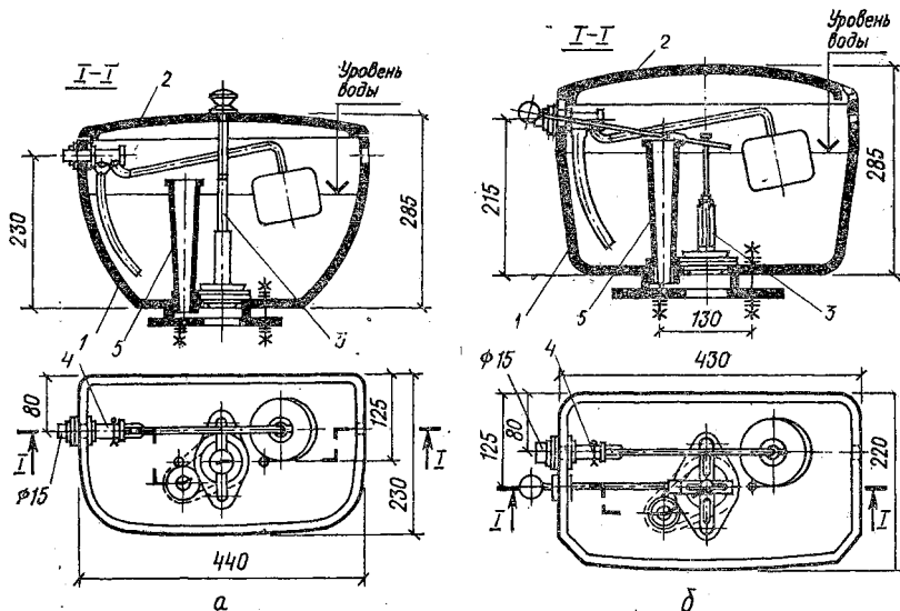
Рис. 3.6. Бачки смывные керамические:
