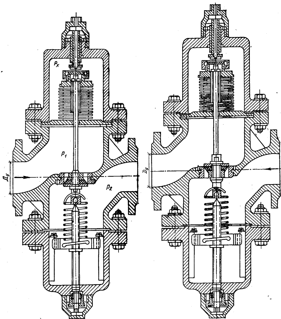
Рис. 9.14. Регулятор расхода типа РР. Рис. 9.15. Регулятор давления типа РД.
