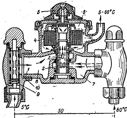
Рис. 9.37. Термостатический смеситель:
