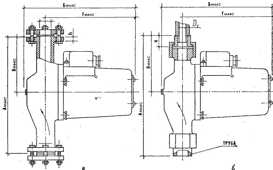
Рис. 2.18. Электронасос ЦВЦ:
