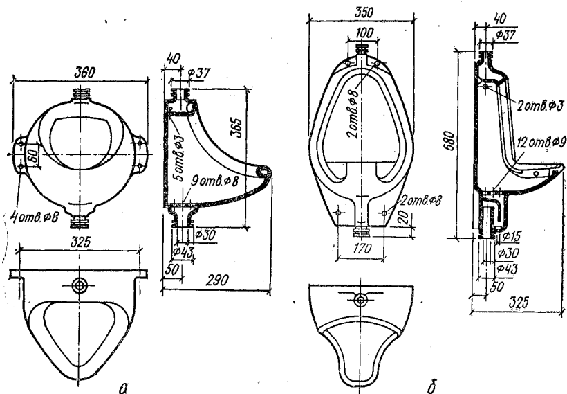
Рис. 3.5. Писсуары:
