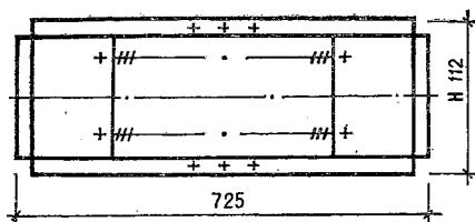
6.12. Размеры, мм, электрокалориферов СФО
