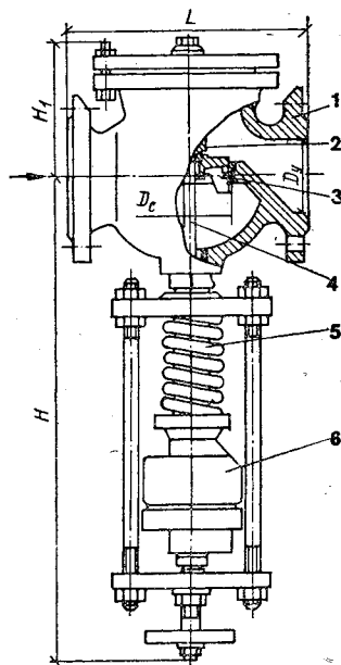
Рис. 9.7. Пружинный регулятор давления «после себя» типа 18ч26р:
