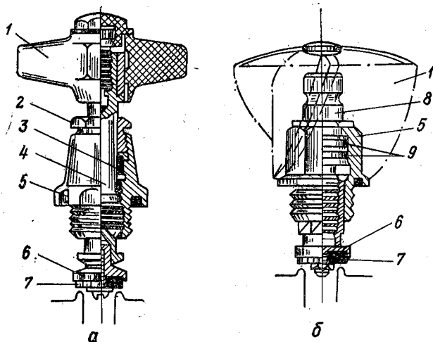
Рис. 9.32. Вентильные головки:
