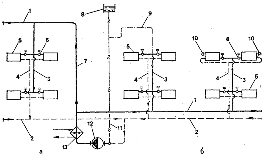
Рис. 5.6. Двухтрубная насосная система водяного отопления с верхней (а) и с нижней (б) разводкой:
