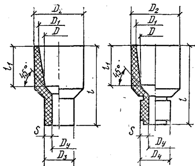
3.26. Размеры, мм, патрубков из ПВХ, ПНП и ПП по ГОСТ 22689.7—77 для присоединения к выпускам раковин
