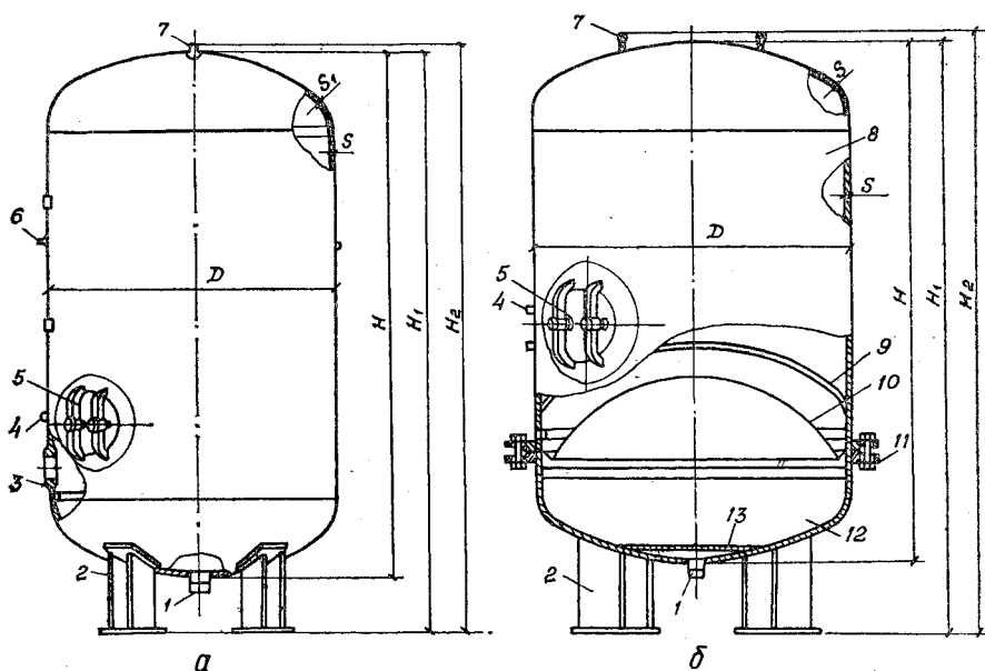
Рис. 2.11. Гидропневматические баки:
