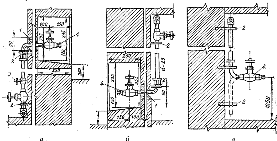
Рис. 2.24. Поливочные краны:
