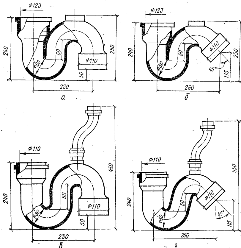
Рис. 3.16. Сифоны для напольных чугунных чаш типов:
