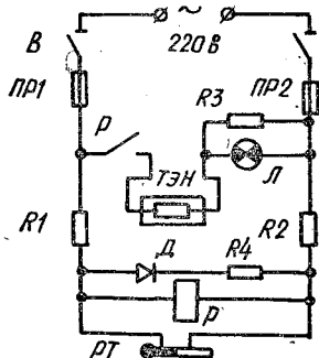
Рис. 8.5. Электрическая схема электроводонагревателя типа УНС-100:
