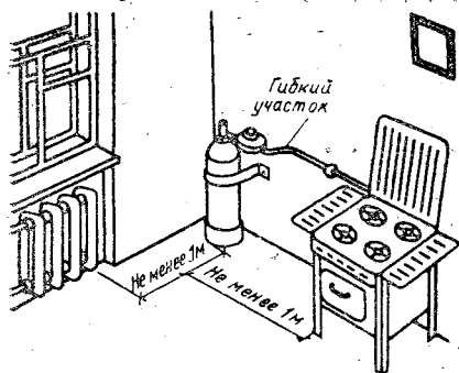
Рис. 7.10. Однобаллонная установка сжиженного газа.
