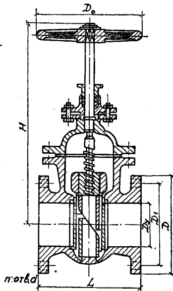
Рис. 9.1. Задвижки чугунные параллельные с выдвижным шпинделем фланцевые.
