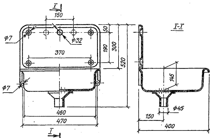
Рис. 3.9. Раковины стальные эмалированные.
