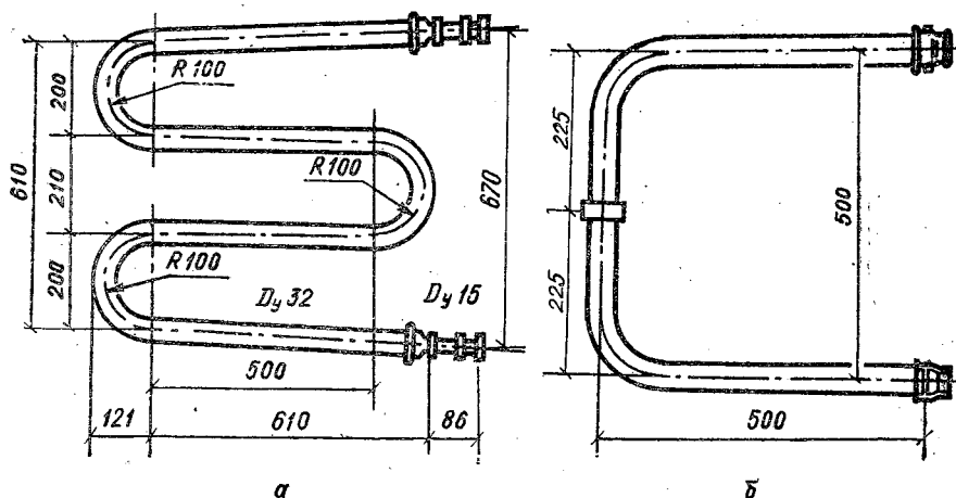
Рис. 4.7. Полотенцесушители из водогазопроводных труб под окраску (а) и эмалированный (б).
