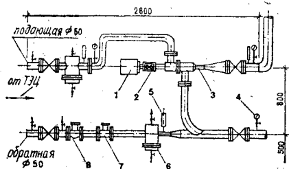
Рис. 5.12. Электронный элеватор с регулируемым соплом типа «Электроника Р-1»: 1 — синхронный электродвигатель; 2 — трехступенчатый цилиндрический редуктор; 3 — элеватор; 4 — манометр; 5 — термометр; 6 — грязевик; 7 — водомер; 8 — реле давления.
