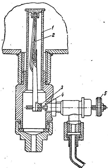
Рис. 9.16. Термореле ТРБ-2:
