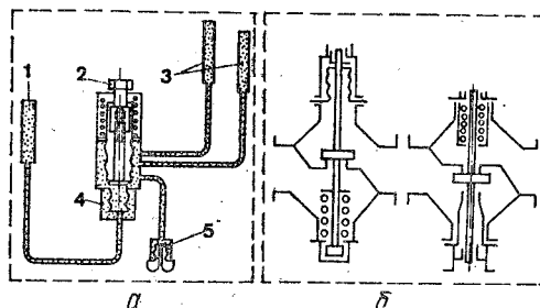
Рис. 9.22. Регулятор температуры прямого действия для систем отопления (термосистема РТК-2216):
