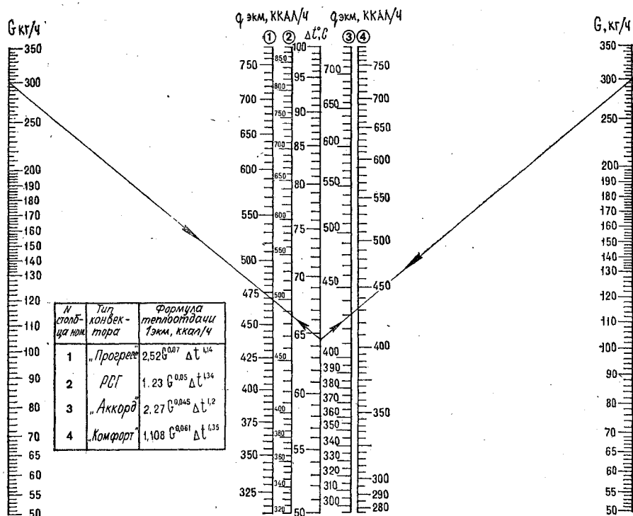
Рис. 5.17. Номограмма для определения теплоотдачи 1 экм стальных панельных радиаторов РСГ и конвекторов «Аккорд», «Комфорт» и «Прогресс».
