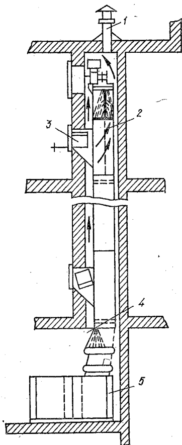
Рис. 3.31. Общая схема мусоропровода:
