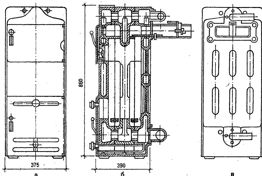
Рис. 5.31. Чугунный секционный водогрейный котел КЧММ: а — вид с фронта; б — разрез; в — вид со стороны задней секции.
