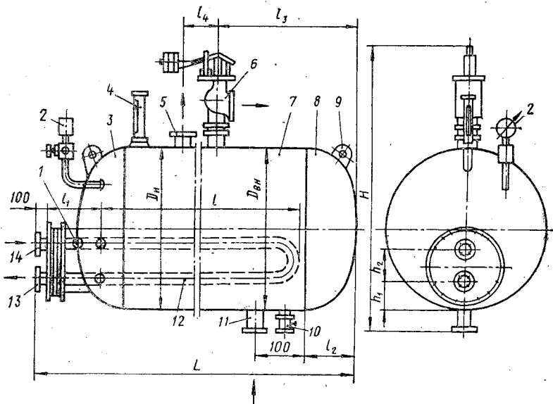
Рис. 4.11. Пароводяной емкий подогреватель:
