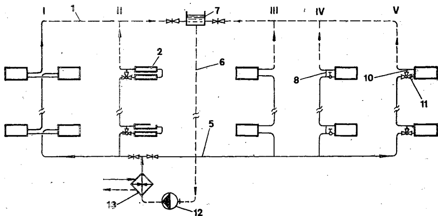
Рис. 5.4. Вертикальные однотрубные насосные системы водяного отопления с нижним расположением подающих магистралей, верхней прокладкой обратных и проточным расширительным баком:
