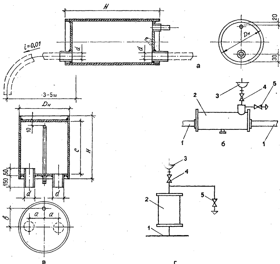
Рис. 5.27. Проточные воздухооборники:
