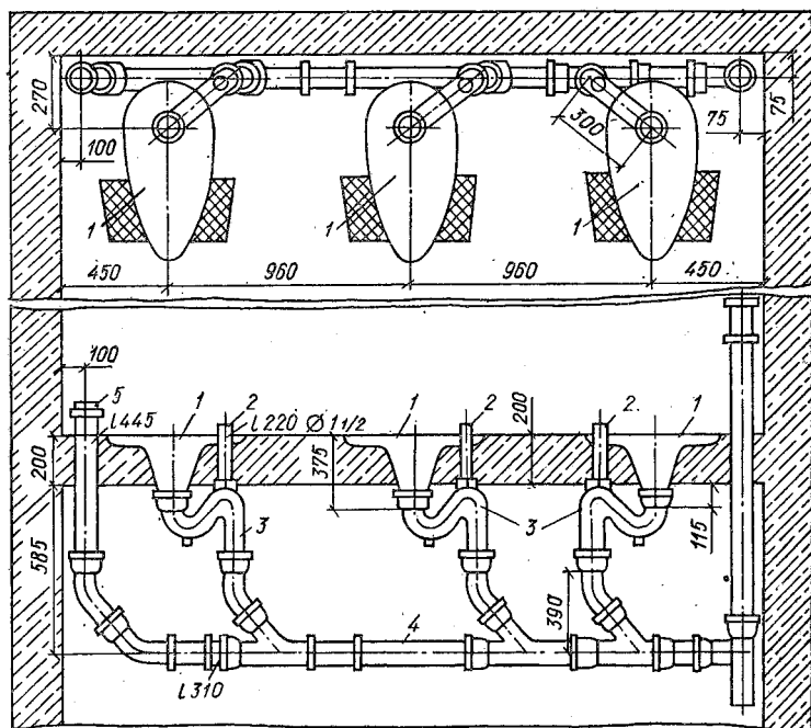
Рис. 3.26. Монтажное положение напольных чаш:
