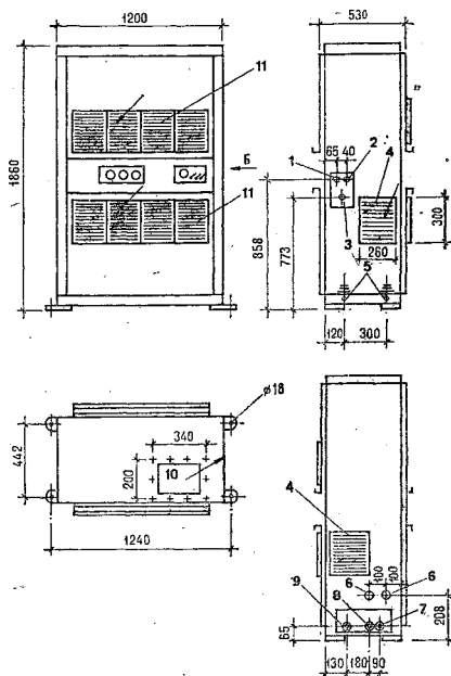
Рис. 6.9. Автономный кондиционер КТА1-4-01:
