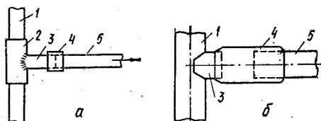
Рис. 7.3. Присоединение отвления к газопроводу:
