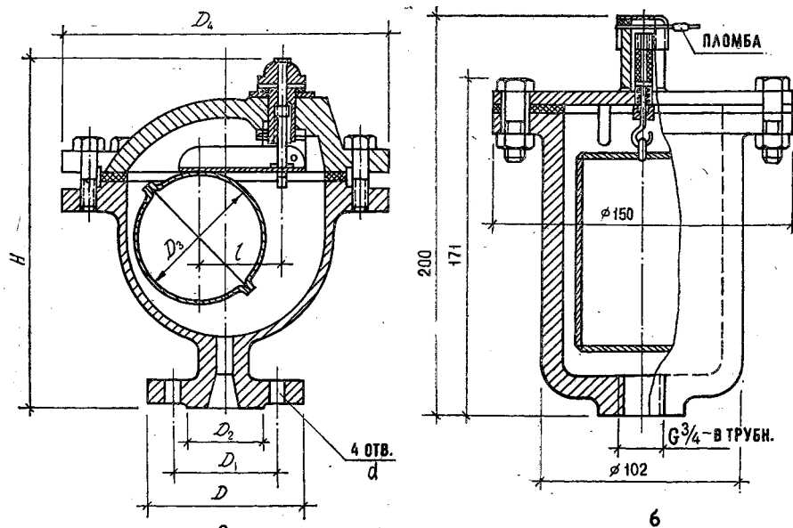
Рис. 5.28. Воздухоотводчики автоматические: а — конструкции ВНИИСТО; б — конструкции ВНИИГС,
