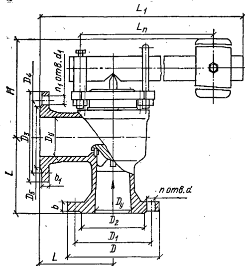
Рис. 9.29. Клапан предохранительный малоподъемный однорычажный фланцевый 17кч36р.
