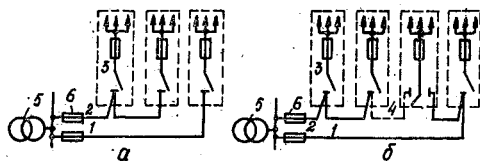
Рис. 8.1. Схемы электроснабжения жилых домов:
