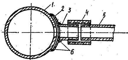
Рис. 7.2. Приварка штуцера с седелькой к газопроводу:
