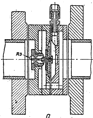
Рис. 9.24. Терморегулятор конструкции Башкирэнерго:
