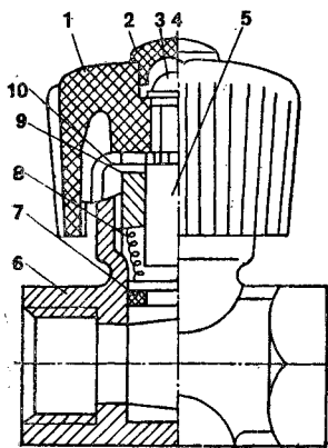
Рис. 9.9. Кран двойной регулировки типа КРДП:
