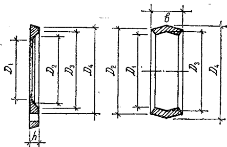
2.36. Размеры, мм, и масса, кг, деталей чугунных соединительных муфт для асбестоцементных труб (ГОСТ 17584—72*)
