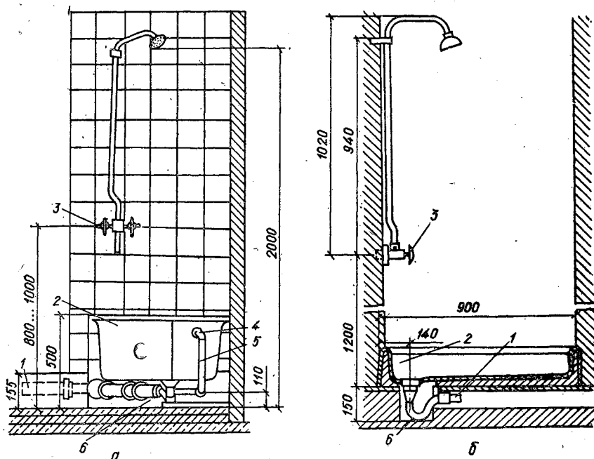
Рис. 3.20. Установка поддонов:
