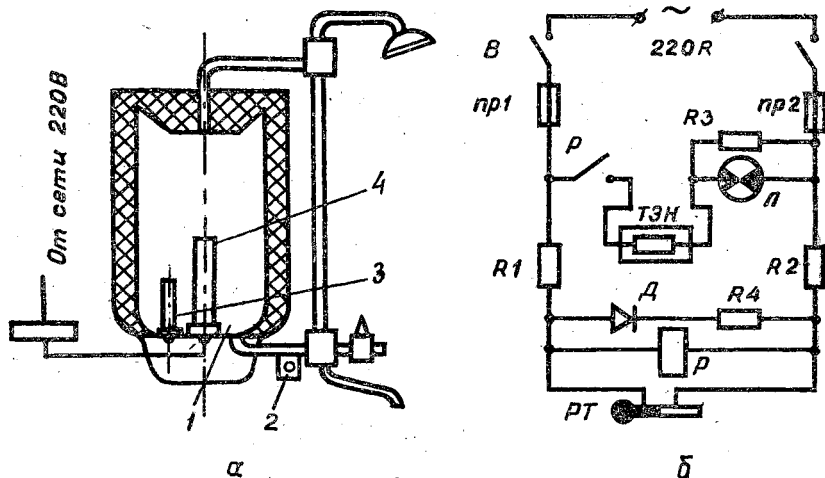
Рис. 4.16. Электронагреватель типа УНС-100:
