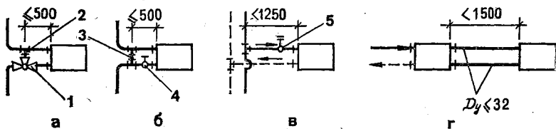
Рис. 5.24. Одностороннее присоединение нагревательных приборов к теплопроводам:
