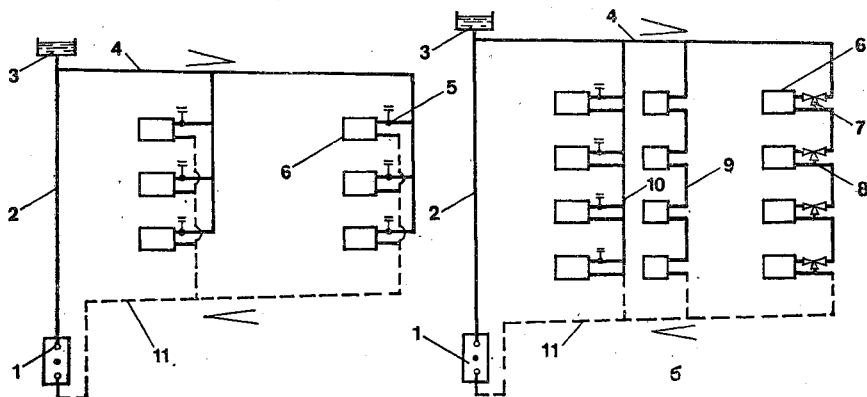
Рис. 5.1. Системы водяного отопления с естественной циркуляцией с двухтрубными (а) и (б) однотрубными отопительными стояками:
