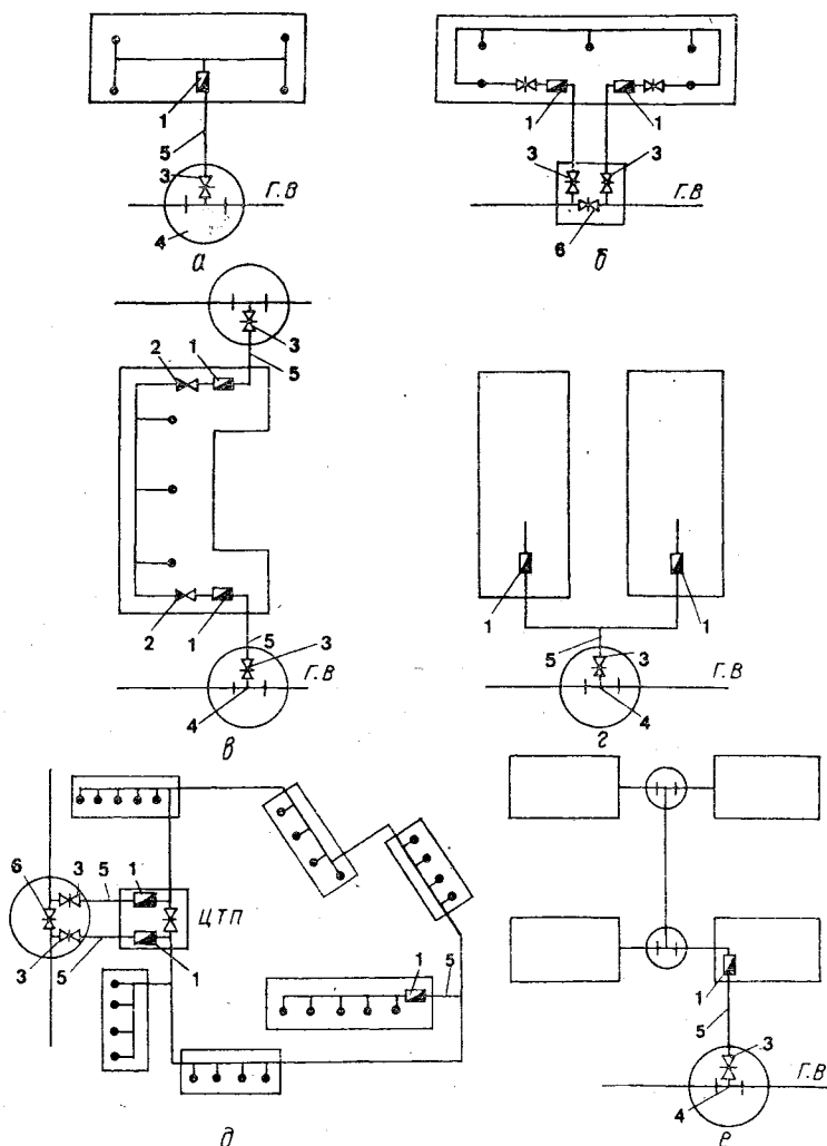
Рис. 2.4. Схемы водопроводных вводов:
