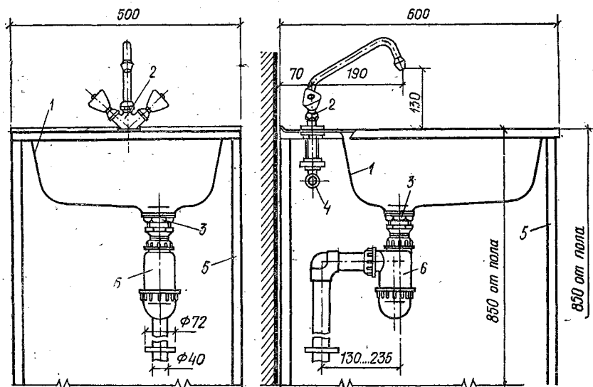
Рис. 3.21. Монтажная схема установки мойки типа МСУ:
