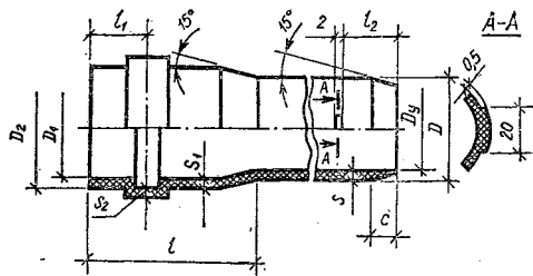
3.17. Размеры, мм, фасонных частей типа I с раструбами и гладкими концами
