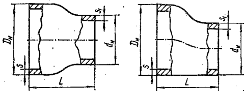
2.31. Размеры, мм, и масса, кг, стальных бесшовных приварных переходов (ГОСТ 17378—83)
