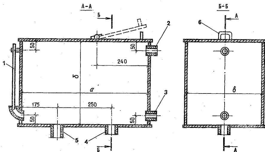
Рис. 5.41. Расширительный бак увеличенной емкости:
