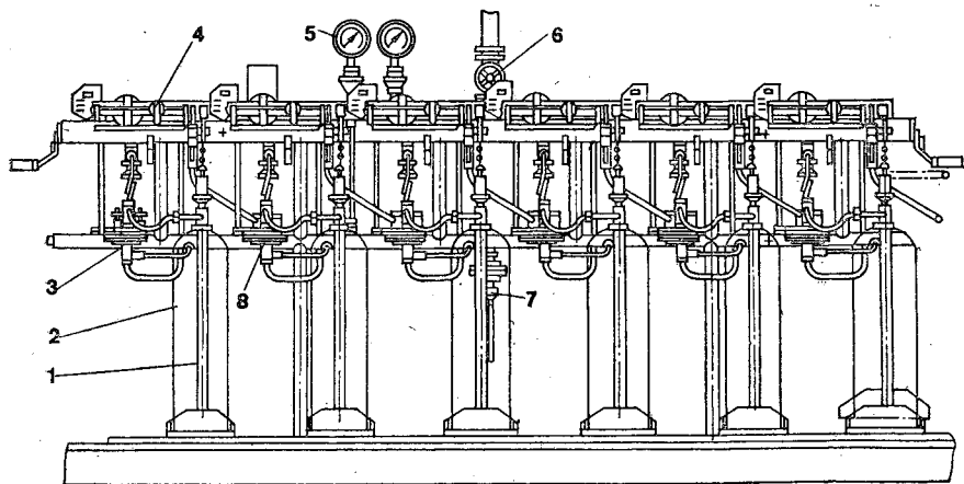
Рис. 7.9. Установка для наполнения баллонов сжиженным газом с неподвижной рамой УНБН-04:
