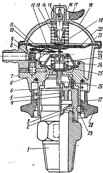
Рис. 9.27. Регулятор давления газа РДСГ-1.2:
