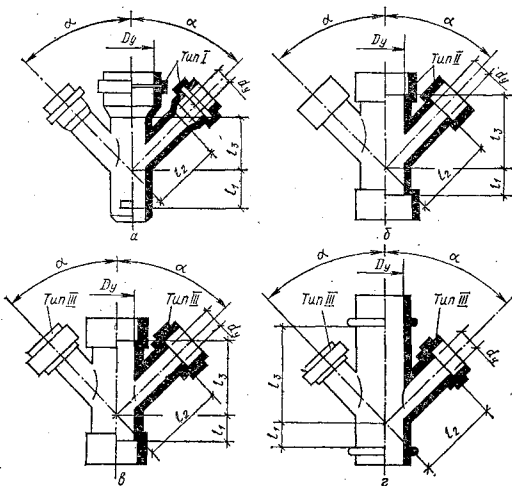
3.31. Размеры, мм, крестовин по ГОСТ 22689.11—77 из ПВХ, ПП и ПВХ (а), из ПВХ, ПНП и ПП (б и в), из ПВХ (г)
