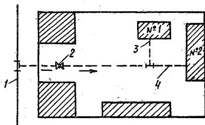
Рис. 7.1. Дворовая сеть газопроводов: 1 — газовая магистраль, d = 150 мм; 2 — задвижка; 3 — газовый ввод в здание №1; 4 — то же, в здание №2.
