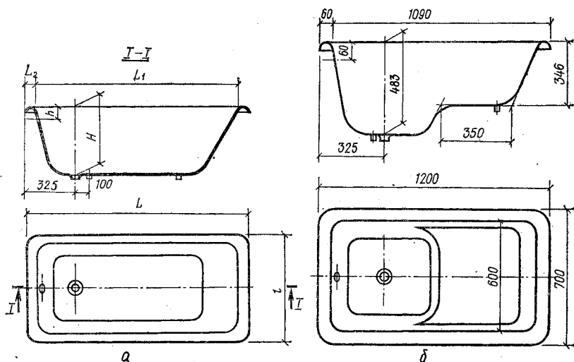
Рис. 3.11. Ванны чугунные эмалированные типов: а — ВЧ-1500, ВЧ-1700, ВЧ-1800; б — ВЧСд-1200.
