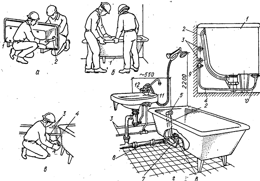
Рис. 3.19. Последовательность установки ванны — а...в и ее монтажное положение — г:
