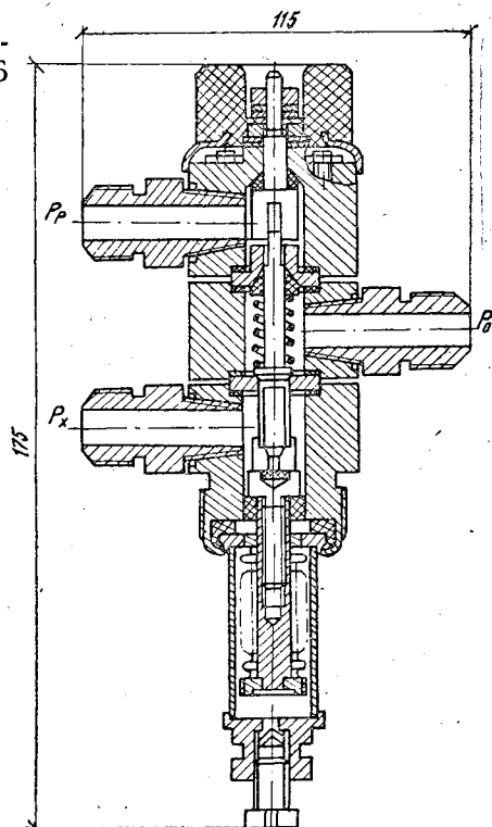
Рис. 9.17. Термодатчик типа ТМП:
