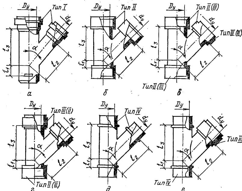
3.30. Размеры, мм, тройников по ГОСТ 22689.10—77 из ПВП, ПП и ПВХ (а), из ПВП, ПНП, и ПП (б, в, г,), из ПВП (д, е)
