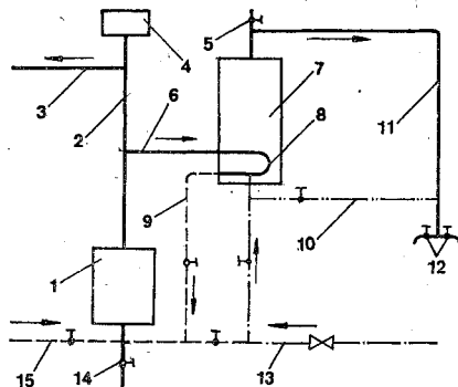
Рис. 5.44. Схема напорного горячего водоснабжения, совмещенного с квартирным отоплением:
