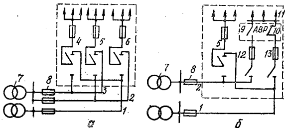
Рис. 8.3. Схемы электроснабжения жилых домов повышенной этажности:
