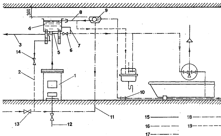
Рис. 5.40. Схема горячего водоснабжения, совмещенного с водяным квартирным отоплением при непосредственном подогреве воды в генераторе теплоты и увеличенной емкости расширительного бака:
