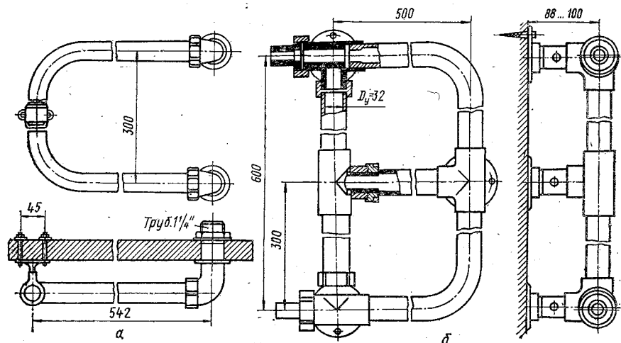
Рис. 4.6. Полотенцесушители латунные типа ПО-30 (а) и ПО-20 (б).
