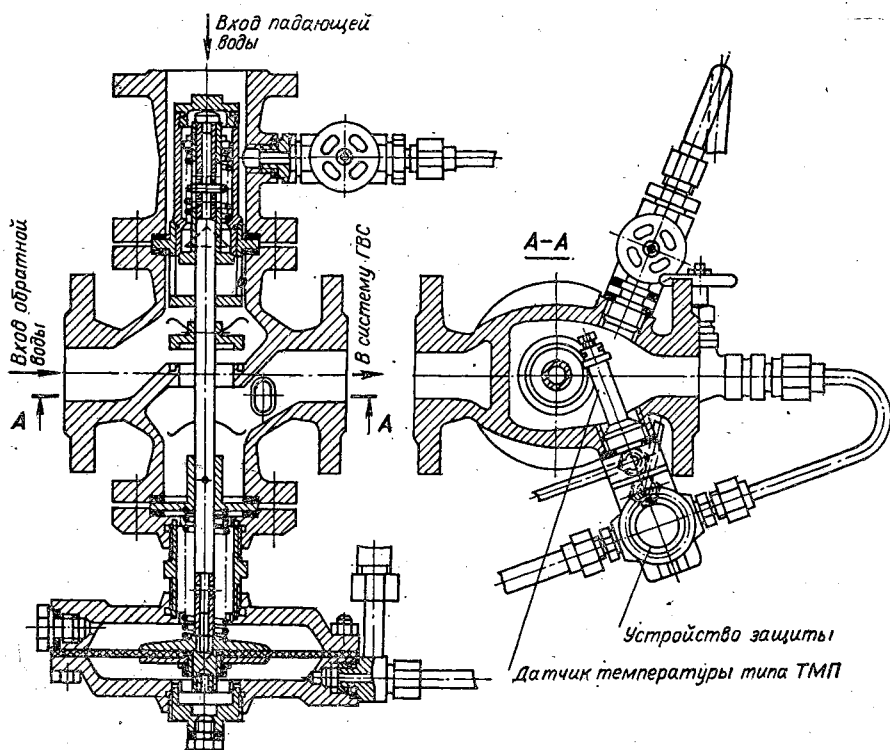
Рис. 9.18. Регулятор температуры РТБ конструкции Союзтехэнерго.
