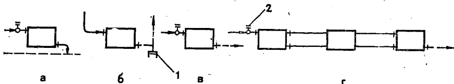
Рис. 5.25. Разностороннее присоединение нагревательных приборов к теплопроводам при движении воды в приборах сверху вниз:
