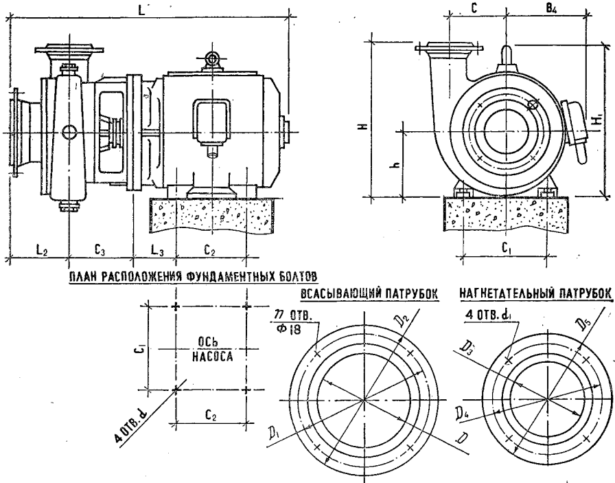
Рис. 2.17. Насосы центробежные консольные типа КМ Китайского завода.
