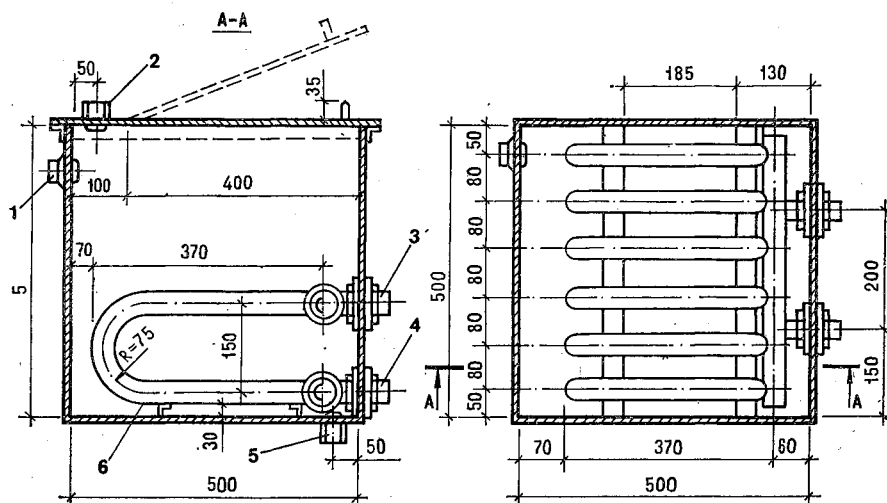
Рис. 5.43. Водоподогреватель:
