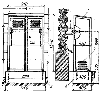
Рис. 7.11. Установка шкафа для двух баллонов у деревянной стены дома:
