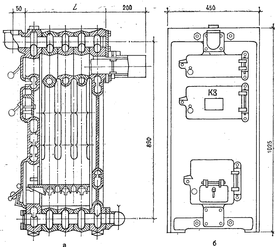
Рис. 5.33. Чугунный секционный водогрейный котел КЧМ-1: а — продольный разрез; б — вид с фронта.
