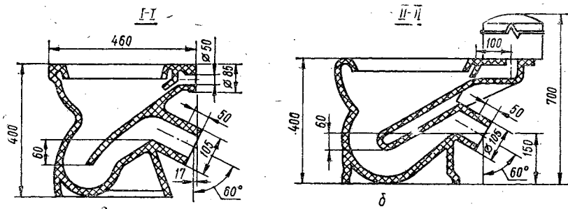
Рис. 3.3. Унитазы:
