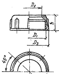
3.37. Размеры, мм, гаек накидных по ГОСТ 22689.17—77
