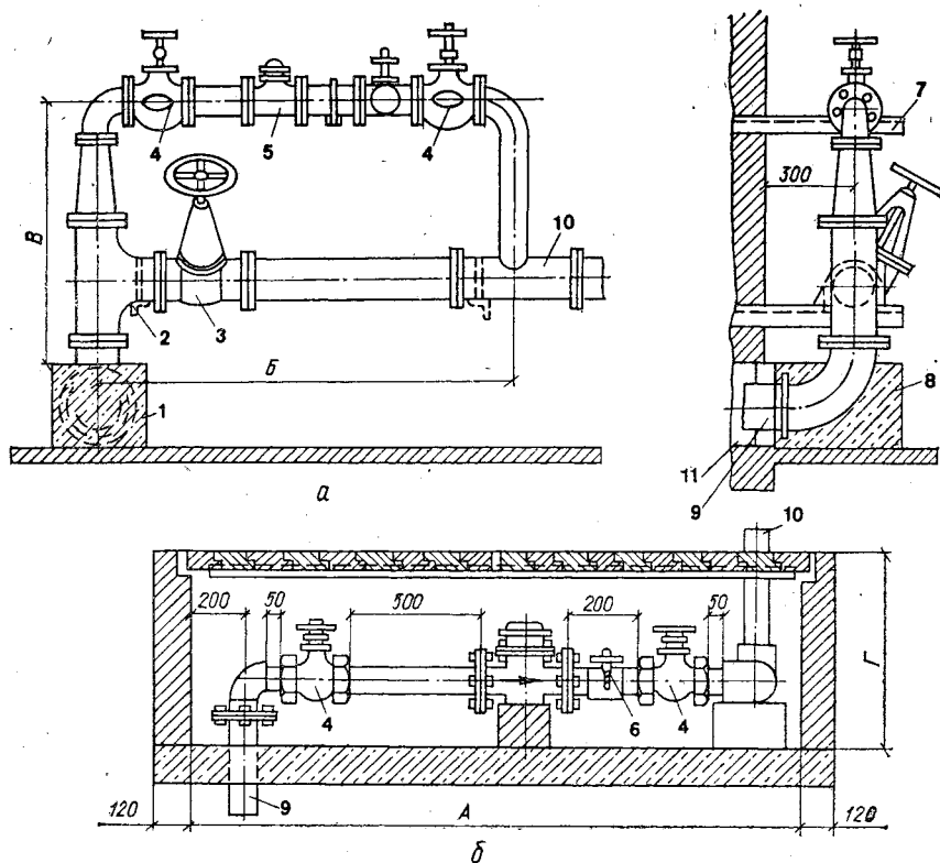
Рис. 2.6. Водомерные узлы:
