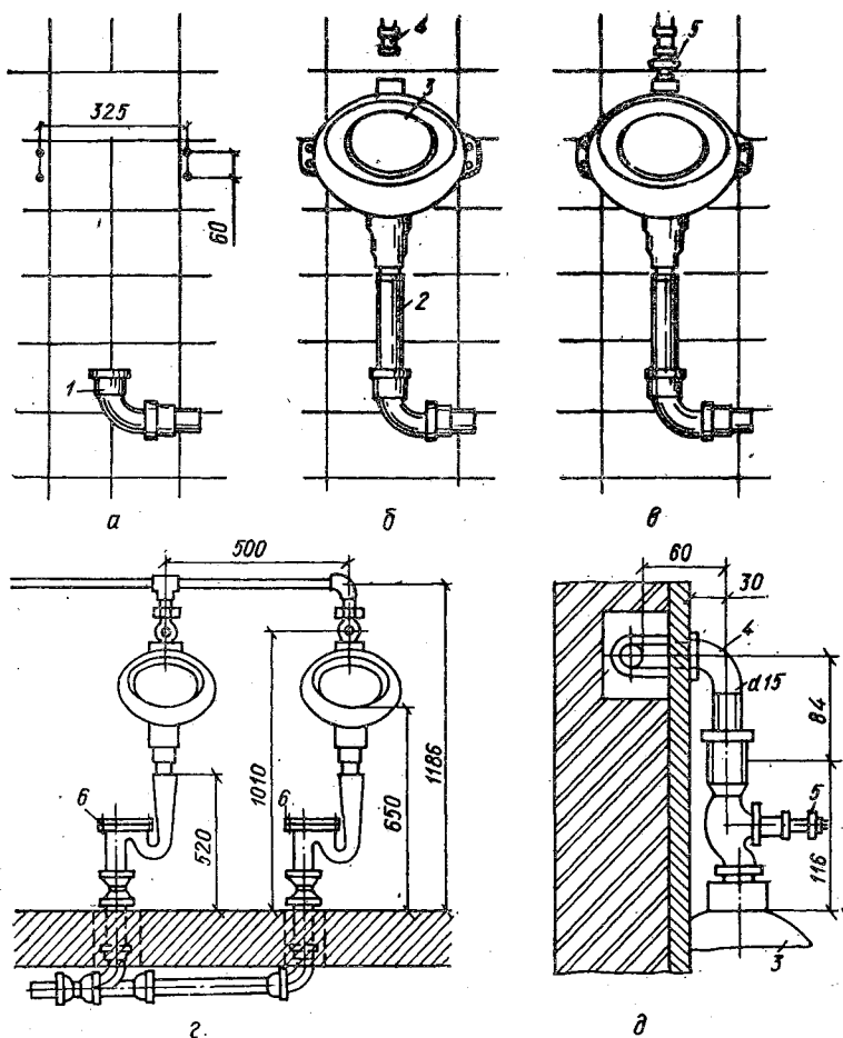
Рис. 3.27. Последовательность установки писсуаров — а...в и их монтажное положение — г и д:
