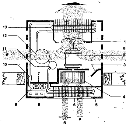
Рис. 6.10. Принципиальная схема кондиционера типа БК:
