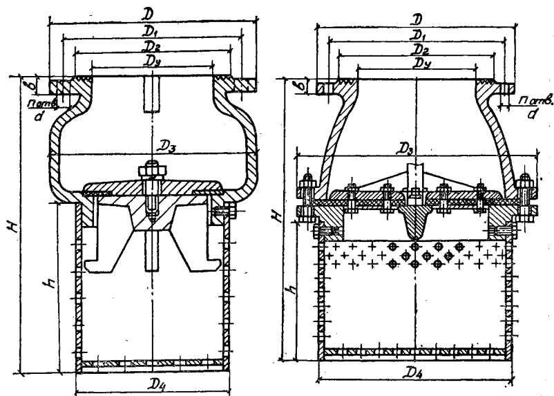
Рис. 9.5. Клапан обратный приемный фланцевый чугунный: а — с одной тарелкой; б — с двумя тарелками.
