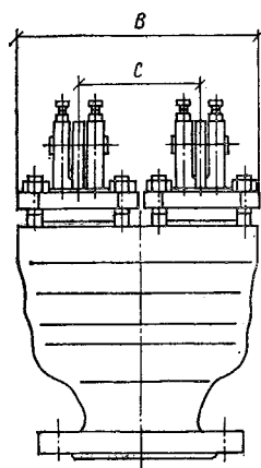
9.26. Размеры, мм, и масса, кг, одинарных предохранительных клапанов 17кч36р (см. рис. 9.29)
