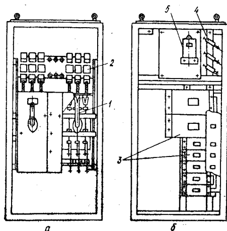
Рис. 8.7. Шкафы ВРУ (двери сняты):
