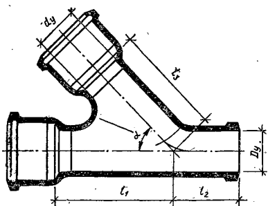
3.10. Размеры, мм, и масса, кг, тройников по ГОСТ 6942.17—80
