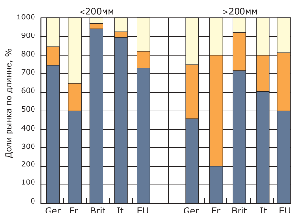
Рис. 1. Структура рынка труб для напорного водоснабжения в странах Евросоюза (по данным AMI)
