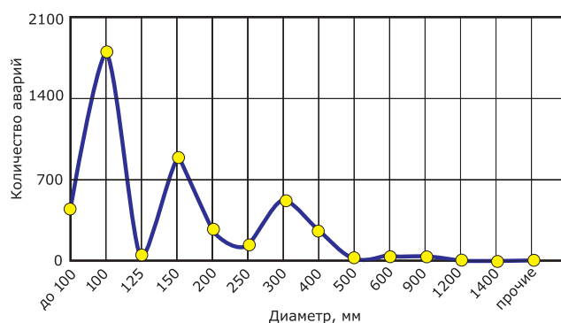
Рис. 2. Динамика аварийности в земле трубопроводов различных диаметров
