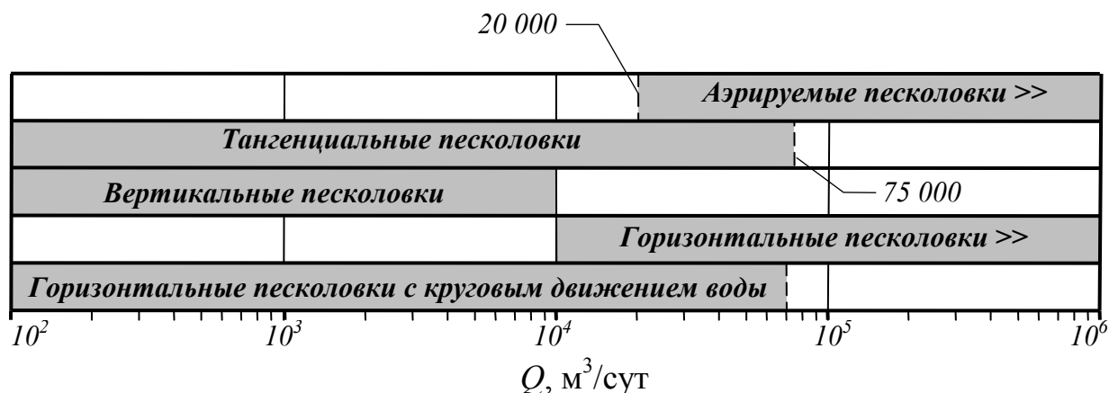
Рис. 3.8. Область применения различных типов песколовок
