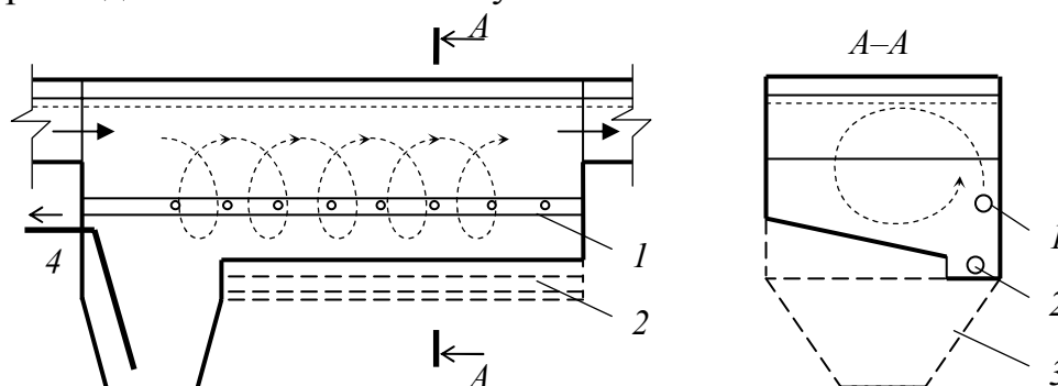
Рис. 3.5. Аэрируемая песколовка
