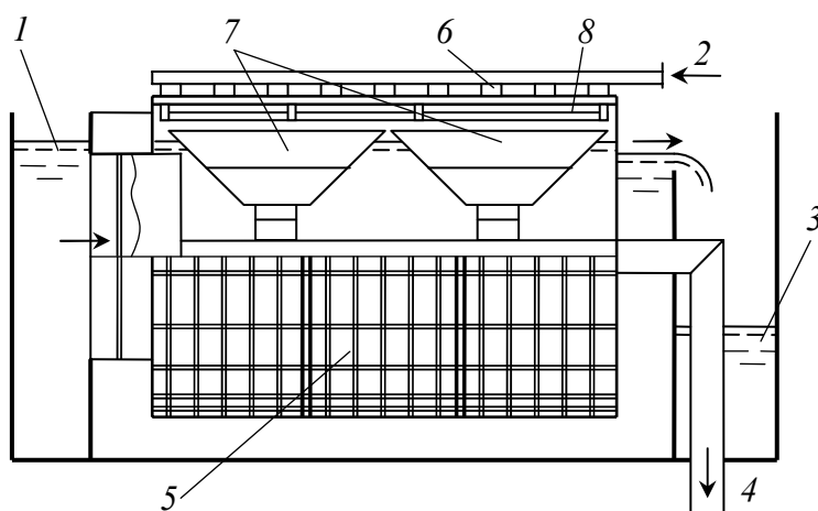
Рис. 7.8. Сетчатый барабанный фильтр (верхняя часть барабана показана в разрезе)
