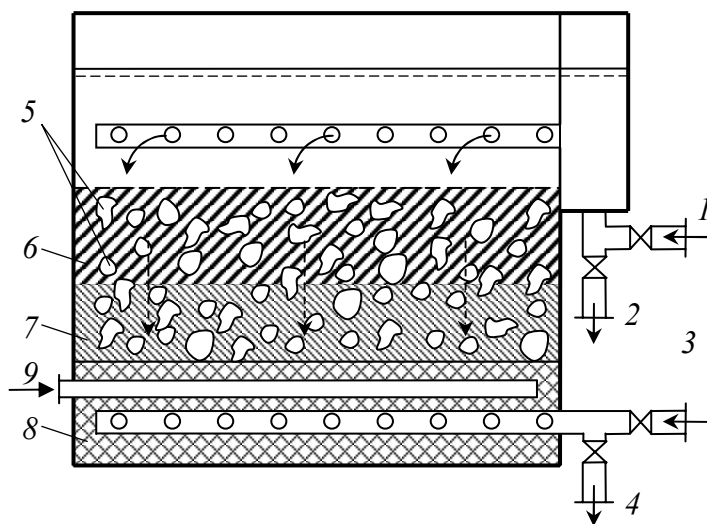
Рис. 7.6. Каркасно-засыпной фильтр
