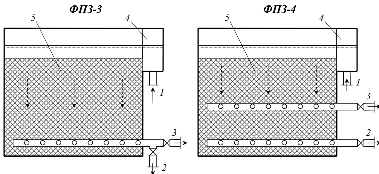
Рис. 7.7. Фильтры с плавающей загрузкой
