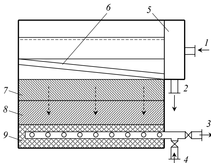
Рис. 7.4. Двухслойный фильтр
