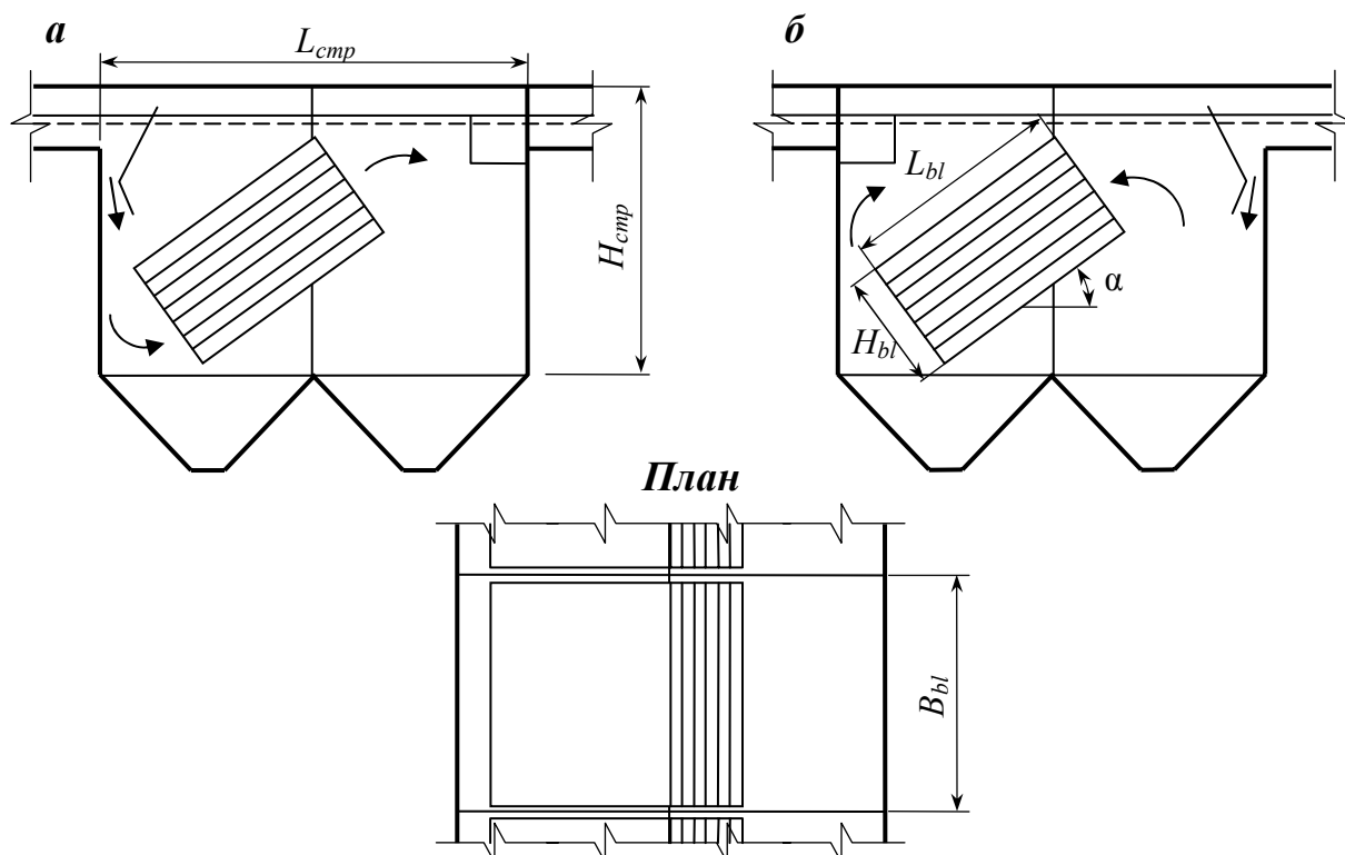
Рис. 4.16. Расчетная схема тонкослойного отстойника с противоточной схемой работы № 1 а – для удаления тяжелых примесей; б – для удаления легких примесей (масло, нефтепродукты и т.д.)
