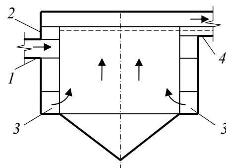
Рис. 3.3 Вертикальная песколовка с вращательным движением
