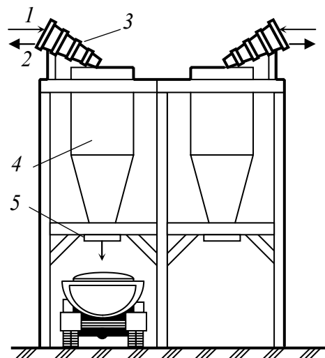
Рис. 3.7. Бункеры для обезвоживания и хранения песка 1 – подача пескопульпы; 2 – отвод воды; 3 – гидроциклон; 4 – бункер; 5 – задвижка для выгрузки песка
