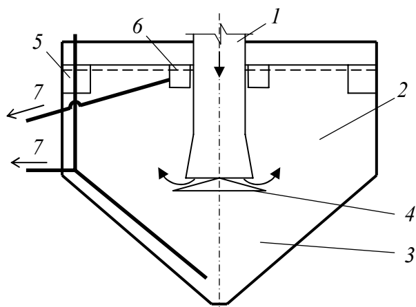
Рис. 4.3. Вертикальный отстойник с центральным впуском
