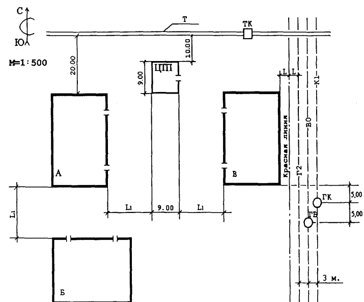
Рис. 1. Генплан
