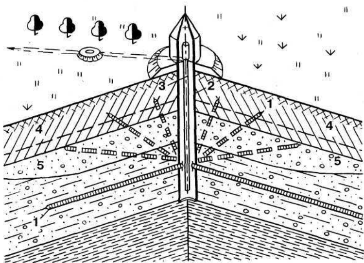
Рис. 3. Лучевой водозабор:
