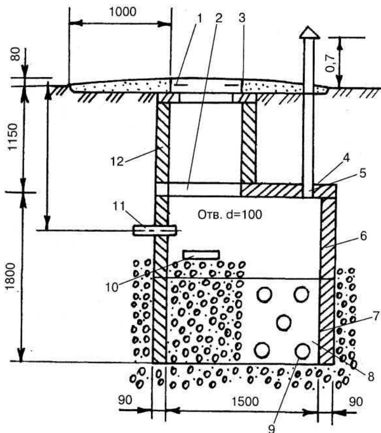
Рис. 20. Фильтрующий колодец (из железобетонных колец):
