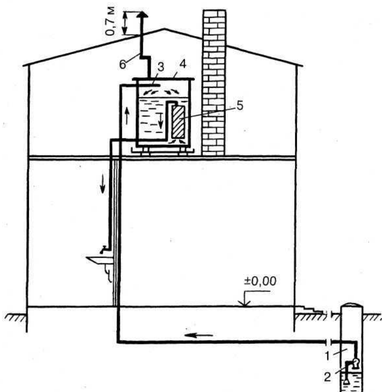
Рис.1. Автономная система водоснабжения сельского усадьбного дома с фильтром водоочистки:
