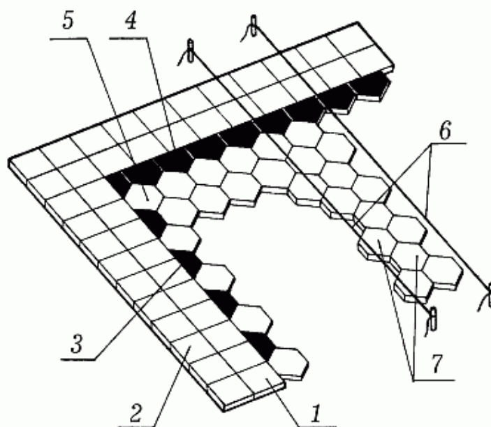
Рис. 90. Облицовка пола шестигранными плитками: 1 – начальный ряд; 2 – заделочный ряд; 3 – четырехгранные половинки; 4 – пятигранные половинки; 5 – шестигранные половинки; 6 – шнуры-причалки; 7 – маячные ряды
