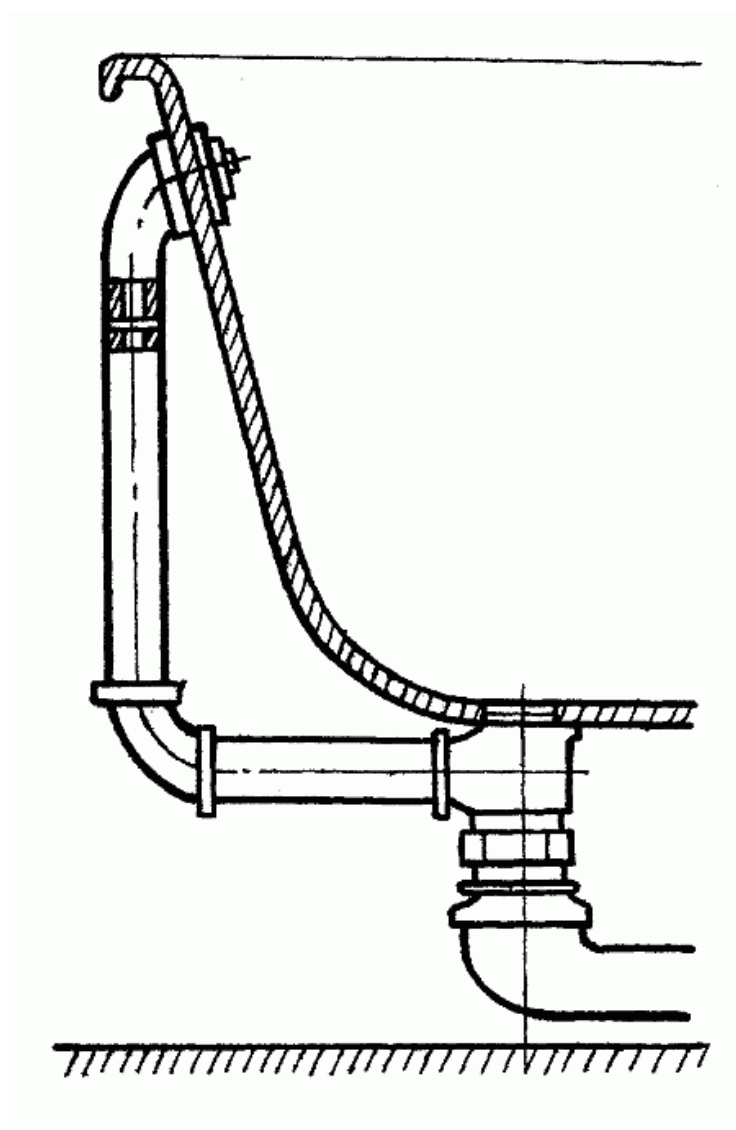
Рис. 32. Сообщение перелива с сифоном
