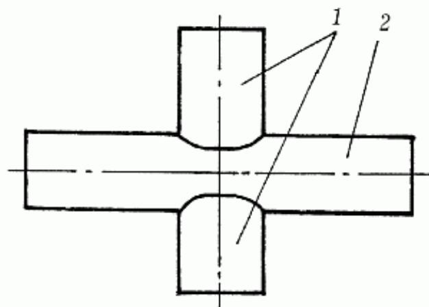
Рис. 18. Крест: 1 — штуцер; 2 — ствол
