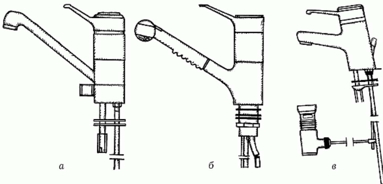
Рис. 21. Некоторые конструкции смесителей: а – смеситель для кухни; б – смеситель для кухни с душевой сеткой; в – смеситель для умывальника с управляемым выпуском
