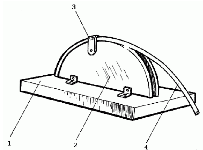
Рис. 46. Плоскопараллельная пластина: 1 – плита; 2 – пластина; 3 – хомут; 4 – труба
