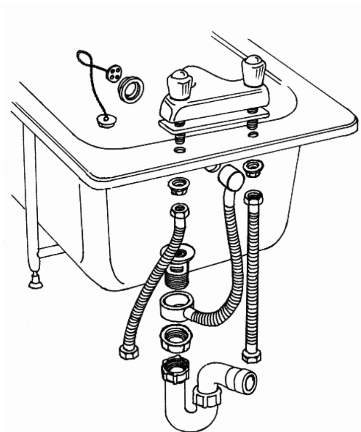
Рис. 34. Присоединение ванны к водопроводу
