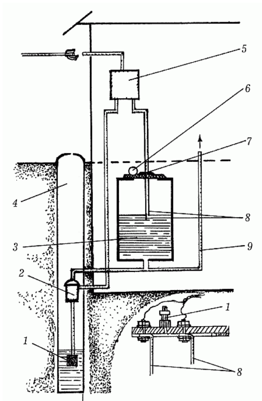
Рис. 58. Водопровод с пневмонапором: 1 – водоприемник с обратным клапаном; 2 – электронасос; 3 – напорный бак; 4 – колодец; 5 – блок управления; 6 – манометр; 7 – вентиль; 8 – датчики уровня; 8 – расходная труба
