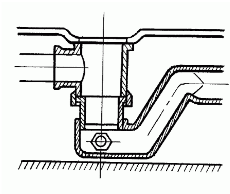
Рис. 33. Сифон для ванны
