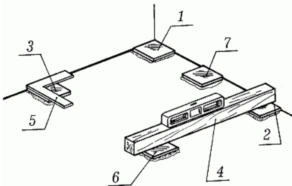
Рис. 88. Разметка горизонтальной поверхности и установка маячных плиток: 1–3 – угловые маячные плитки; 4 – деревянная рейка; 5 – угольник; 6–7 – промежуточные маячные плитки
