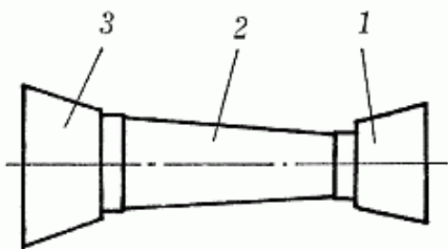
Рис. 15. Переход: 1 — втулка; 2 — переход; 3 — раструб
