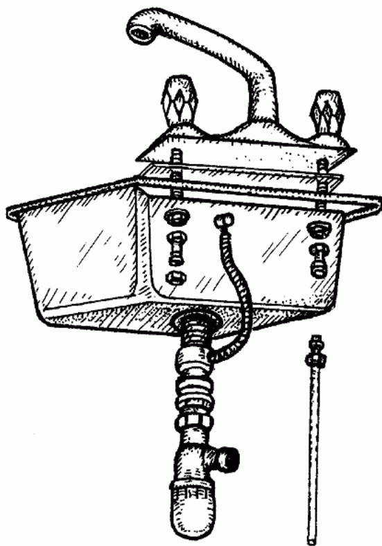
Рис. 31. Присоединение мойки к водопроводу
