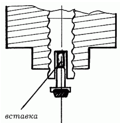
Рис. 113. Вставка между штоком и клапаном
