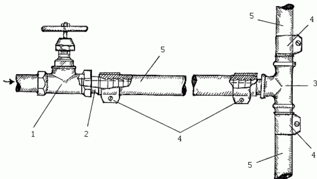
Рис. 63. Соединение резинового водопровода: 1 – вентиль; 2 – переходник; 3 – тройник; 4 – хомут; 5 – шланг
