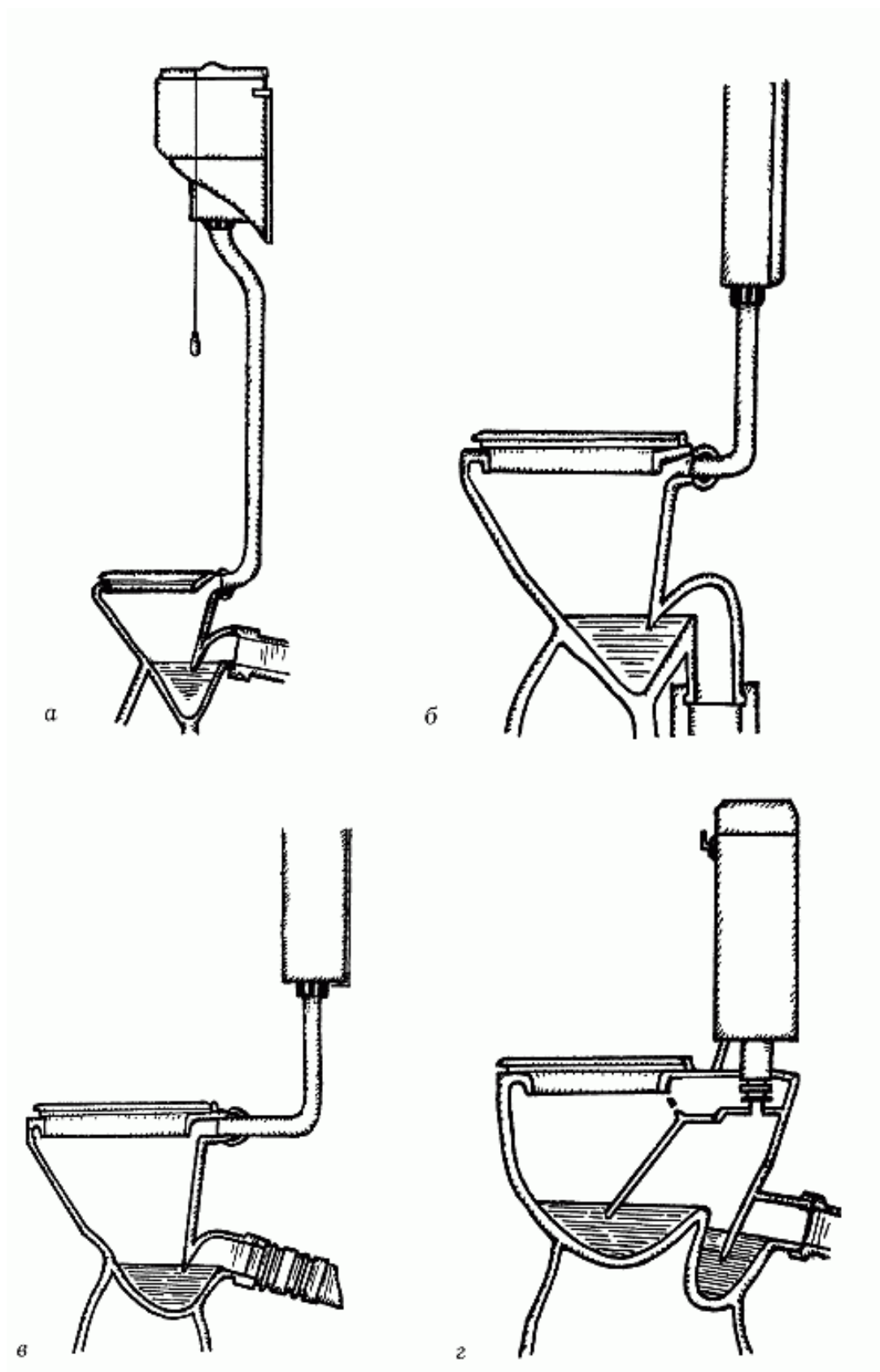
Рис. 35. Виды унитазов: а – с высокорасположенным бачком; б – с низко укрепленным плоским бачком и s-образным сифоном (косой выпуск); в – с низко укрепленным плоским бачком и р-образным сифоном
