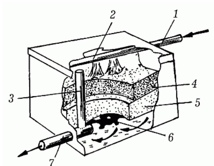
Рис. 103. Внешний фильтр: 1 – вход; 2 – труба с отверстиями; 3 – трубка для излишков воды; 4 – фильтр предварительной очистки; 5 – пористый материал; 6 – перфорированная основа; 7 – выход
