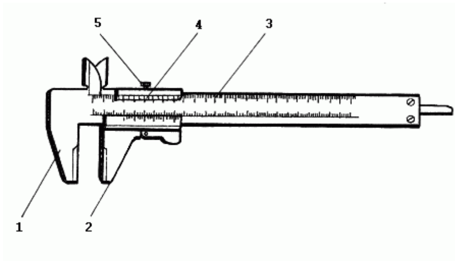
Рис. 13. Штангенциркуль: 1 – измерительные губки; 2 – рамка; 3 – штанга; 4 – нониус; 5 – стопорный винт
