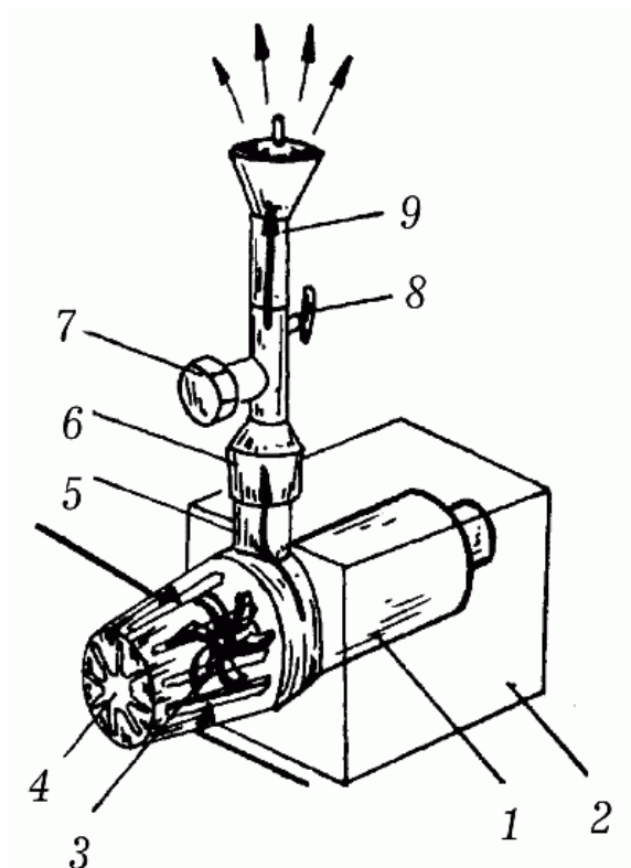
Рис. 100. Устройство насоса: 1 – мотор; 2 – корпус мотора; 3 – крыльчатка насоса; 4 – сетка; 5 – выходная труба; 6 – тройник; 7 – кран для подключения водопада; 8 – регулятор производительности; 9 – форсунка
