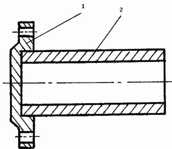
Рис. 19. Патрубок: 1 — фланец; 2 — патрубок
