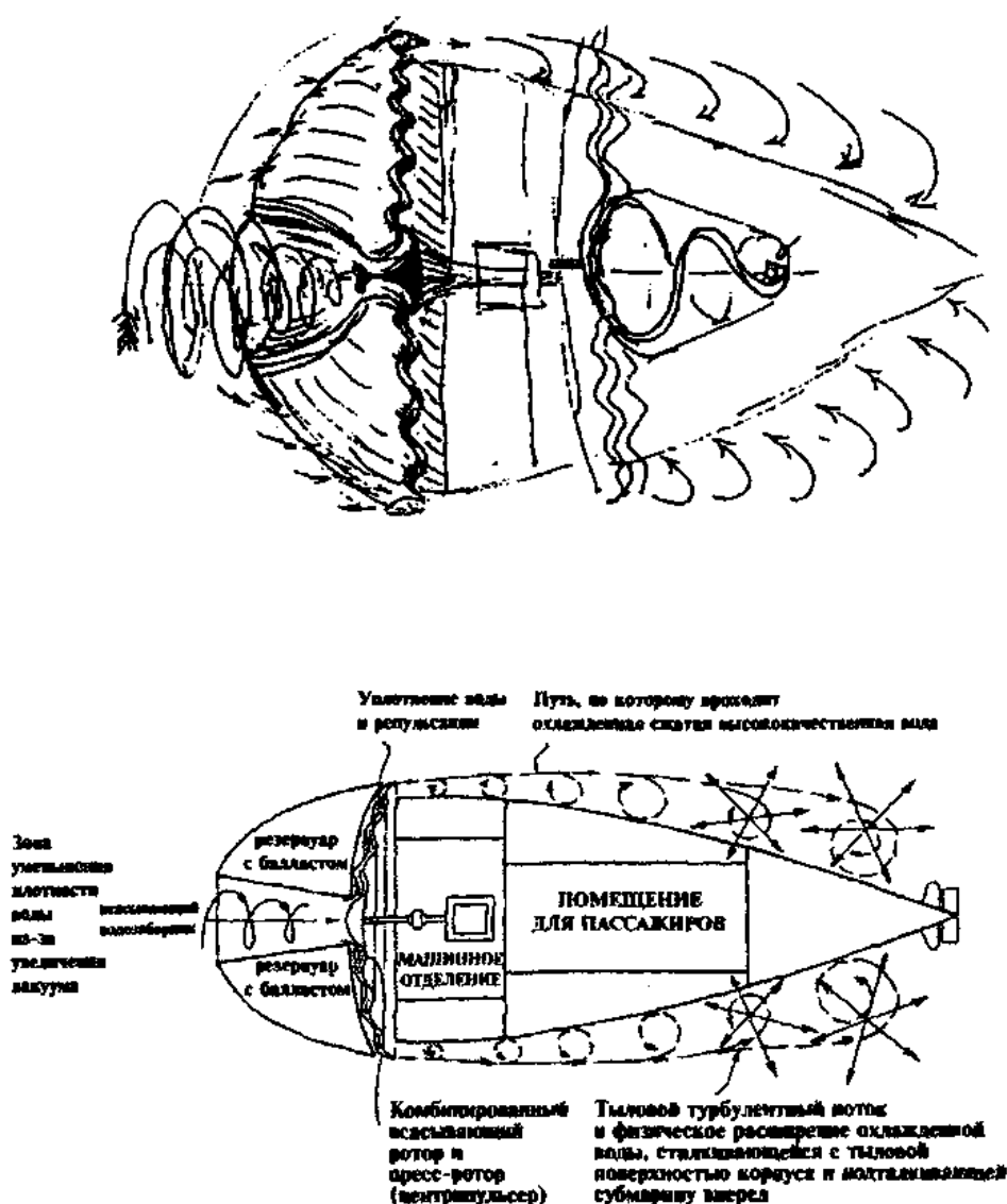
Рис. 22. Биотехническая субмарина (принцип устройства)
