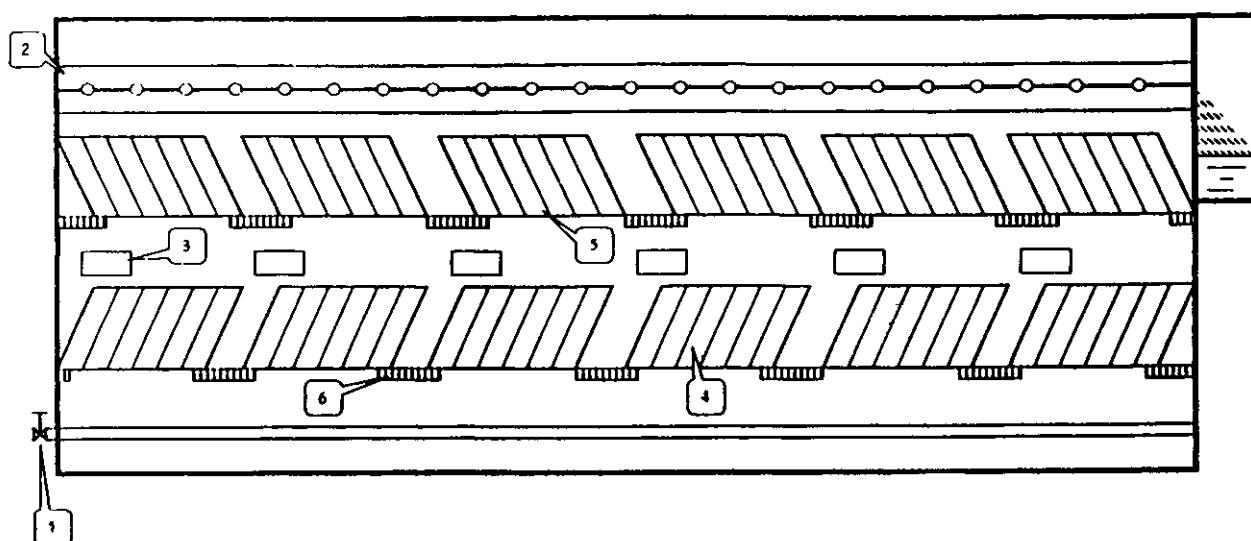
Рис. 2. Тонкослойный осветлитель, оборудованный тонкослойной камерой хлопьеобразования:
