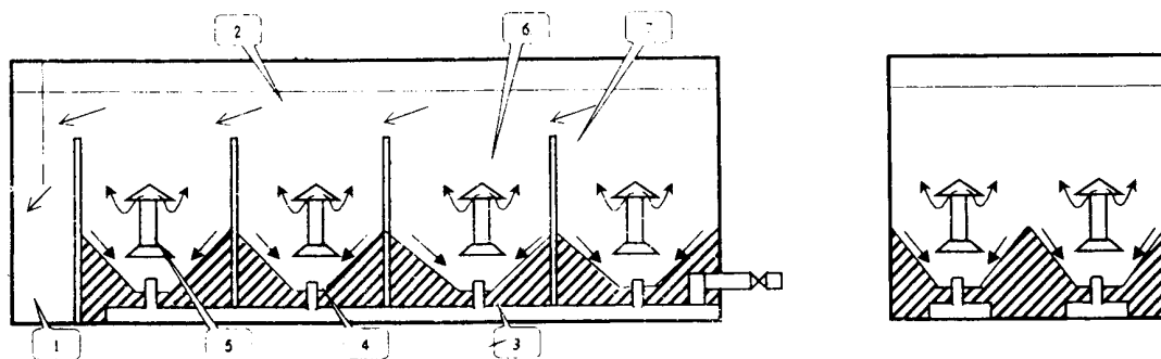
Рис. 4. Камера хлопьеобразования с малозабаритными аппаратами для рециркуляции осадка: 1 — отстойник; 2 — камера хлопьеобразования; 3 — канал исходной воды; 4 — патрубок с соплом; 5 — смеситель; 6 — направляющий аппарат; 7 — перегородки
