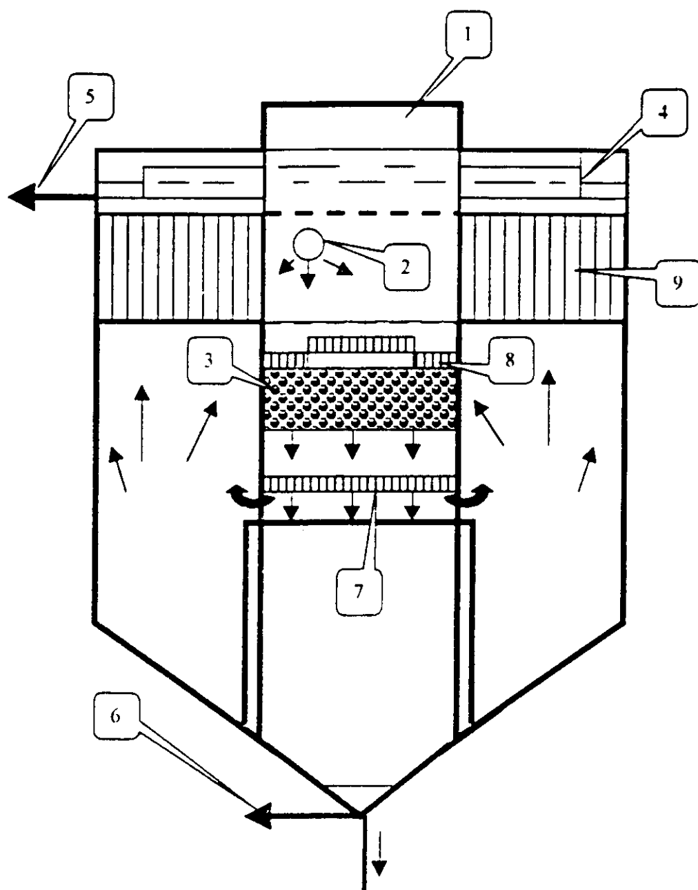
Рис. 1. Вертикальный тонкослойный отстойник с контактной камерой хлопьеобразования:
