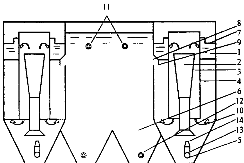
Рис. 8. Осветлитель-рециркулятор:
