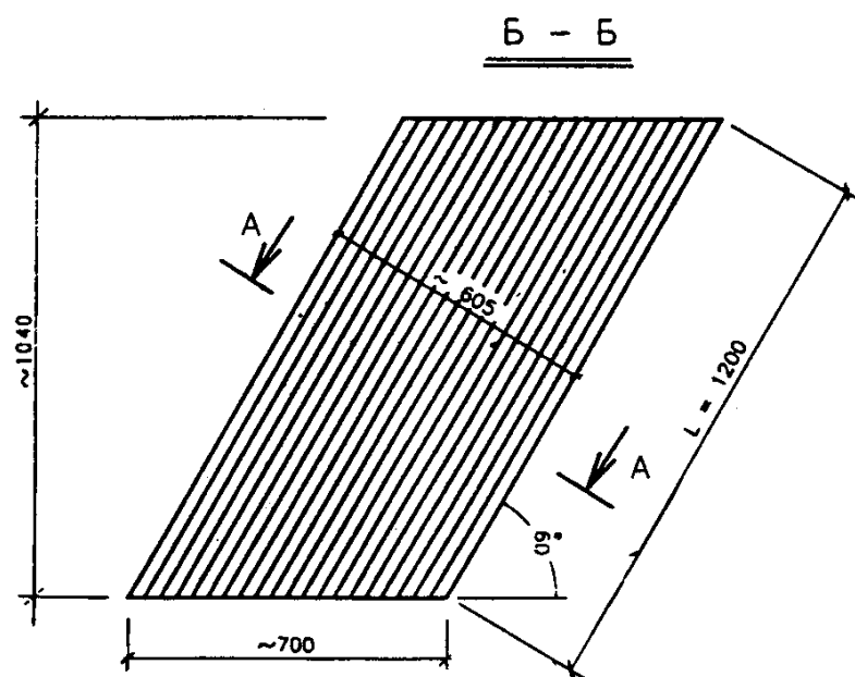
Рис. 7. Тонкослойные модули сотового типа из рулонного материала ПВХ
