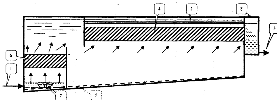
Рис. 5. Тонкослойный горизонтальный отстойник с тонкослойно-эжекционной камерой хлопьеобразования:
