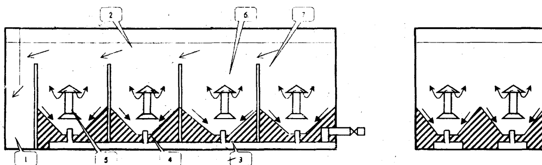
Рис. 4. Камера хлопьеобразования с малогабаритными аппаратами для рециркуляции осадка:
