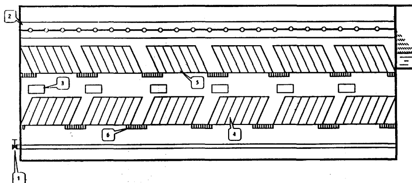
Рис. 2. Тонкослойный осветлитель, оборудованный тонкослойной камерой хлопьеобразования:
