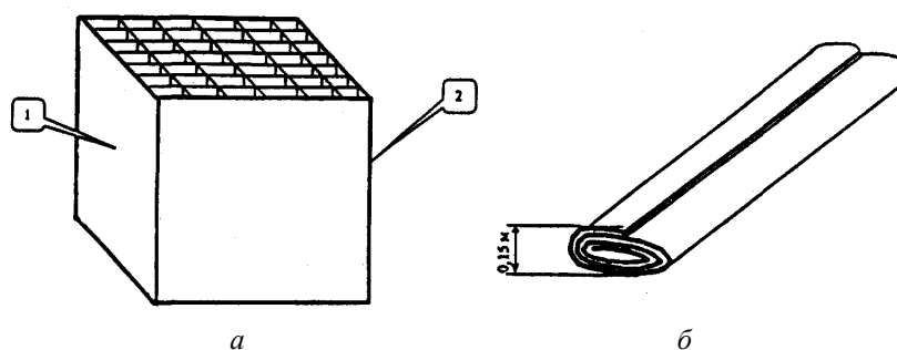
Рис. 6. Тонкослойный сотовый блок из полиэтиленовой пленки:
