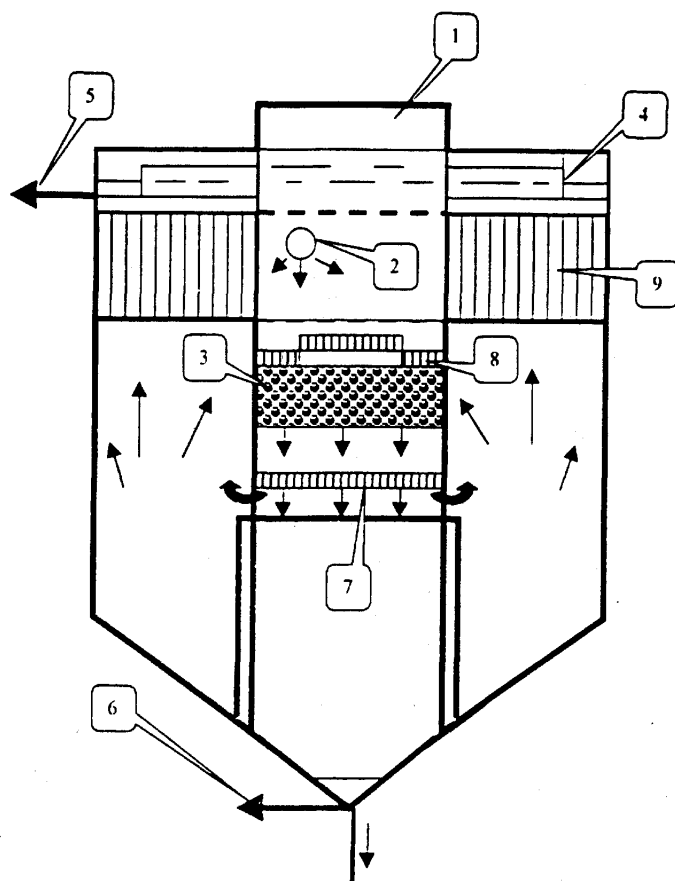
Рис. 1. Вертикальный тонкослойный отстойник с контактной камерой хлопьеобразования:
