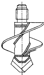
Рис. 5.21. Долото змеевикового типа
