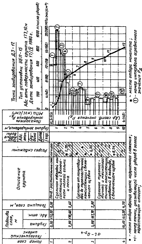
Рис. 2.5.5. График изменения условного динамического сопротивления пород ( R_D ) по результатам динамического зондирования: 1 — место отбора пробы горных пород нарушенного сложения; 2 — кривая изменения количества ударов нарастающим итогом; 3 — место отбора проб горных пород естественного сложения; 4 — значения R_D осредненные по интервалам
