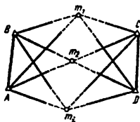
Рис. 1.4. Схема динамической триангуляции
