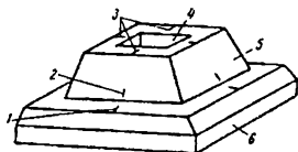
Рис. 1.56. Схема ориентирных и установочных рисков на фундаменте и опорных башмаках колонны:
