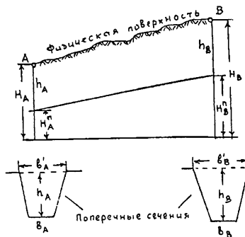
Рис. 1.38. Определение объема траншеи
