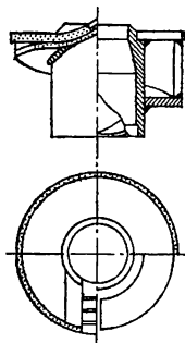
Рис. 5.25. Ограничитель подачи долота
