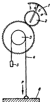
Рис. 2.2.5. Схема боты прогибомера для измерения осадки штампа при пробных статических нагрузках: 1 — циферблат; 2 — зубчатые колеса — редуктор; 3 — барабан; 4 — струна (стальная проволока); 5 — противовес; 6 — штамп
