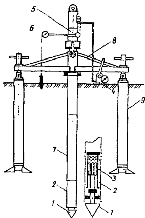
Рис. 2.6.22. Свая-зонд
