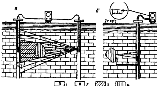
Рис. 6.3. Акустические методы просвечивания — теневой (а) и отражения (б) — для изучения скальных пород: 1 — датчик; 2 — приемник; 3 — акустическая тень; 4 — пустота в породе
