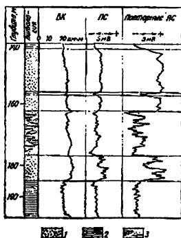
Рис. 6.1. Выделение водоносных пластов по данным метода повторных ПС: 1 — песок; 2 — глины; 3 — чередование песчаных и глинистых отложений
