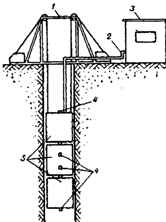
Рис. 2.3.6. Схема прессиометра марки ЦГШ конструкции Института гидротехники им. Введенеева:
