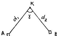
Рис. 1.51. Линейная засечка
