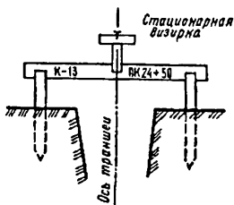
Рис. 1.59. Обноска при разбивке траншеи
