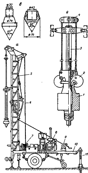
Рис. 2.5.3. Установка УБ-18 конструкции Гидропроекта для производства динамического зондирования: а — установка в рабочем положении; б — конические наконечники инвентарный и съемный; в — навесное устройство для подъема и сбрасывания ударного молота; 1 — ударный молот; 2 — кулачки для захвата и сбрасывания молота; 3 — направляющая штанга; 4 — траверса для подъема молота; 5 — мачта; 6 — трос; 7 — лебедка; 8 — двигатель; 9 — ручная лебедка; 10 — рама; 11 — опоры
