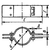
Рис. 5.13. Хомут для обсадных труб
