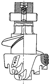
Рис. 5.20. Трехлопастное долото
