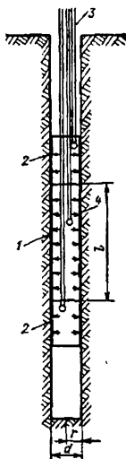
Рис. 2.3.1. Принципиальная схема работы прибора бокового давления — прессиометра:
