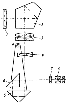
Рис. 1.96. Оптическая схема нивелира Ni-007:
