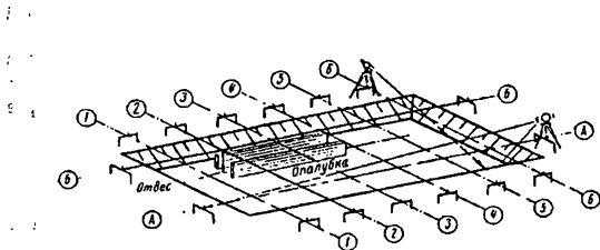
Рис. 1.55. Схема детальной разбивки фундамента
