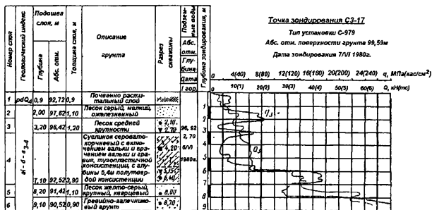
Рис. 2.5.4. График изменения удельных сопротивлений горных пород погружения конуса ( R_{уд.кон} ) и сопротивления горных пород трению по боковой поверхности зонда ( R_{тр} ) с глубиной по результатам статического зондирования: 1–3 — места отбора проб; 1 — горных пород нарушенного сложения; 2 — горных пород естественного сложения; 3 — грунтовой воды
