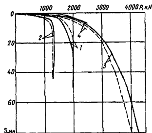
Рис. 2.6.27. Сопоставление экспериментальных графиков «осадка — нагрузка» для свай НС с рассчитанными по предлагаемой методике на производственных площадках:
