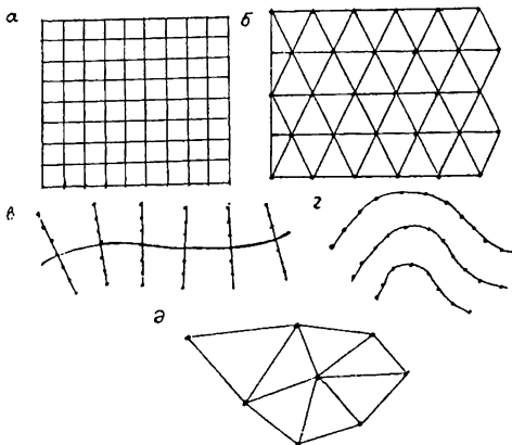
Рис. 1.28. Схемы цифровых моделей местности
