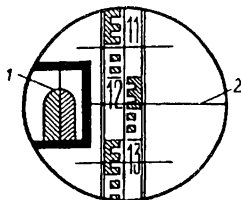
Рис. 1.94. Поле зрения нивелира Н-3:
