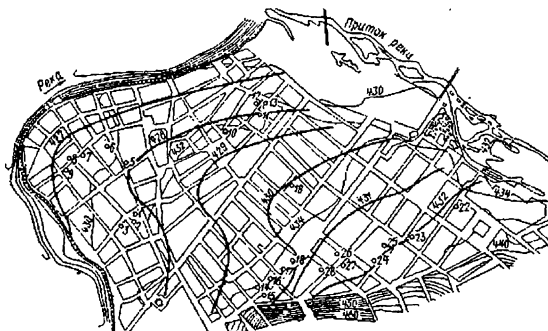
Рис. 6.5б. План участка с гидроизогипсами, характеризующими положение уровня грунтовых вод на 22.01.1975 г. (зимний максимум).
