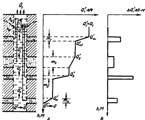
Рис. 3.28. Схема расходометрического исследования скважины при откачке:
