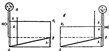
Рис. 1.111. Схемы определения превышения:
