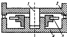
Рис. 1.70. Вертикальная ось теодолита ДКМ-3 с разнесенной шариковой опорой: 1 — ось алидады; 2 — шарикоподшипник; 3 — лимб; 4 — подставка
