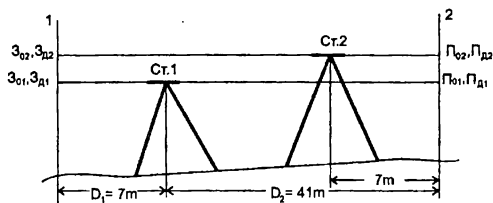
Рис. 1.102. Проверка главного условия нивелира
