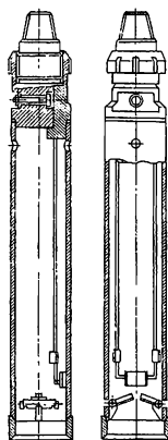
Рис. 5.18. Разъемный вибронд для бурения слабосвязных пород
