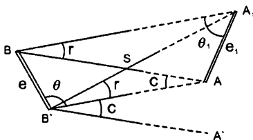
Рис. 1.87. Элементы центрировки и редукции и вызываемые ими поправки
