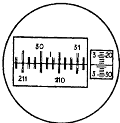
Рис. 1.74. Поле зрения отсчетного микроскопа теодолита Т05
