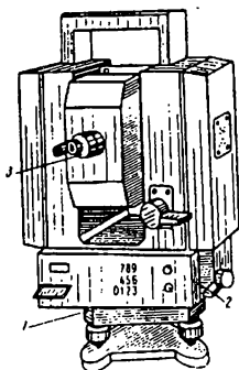
Рис. 1.107. Внешний вид тахеометра Та5:
