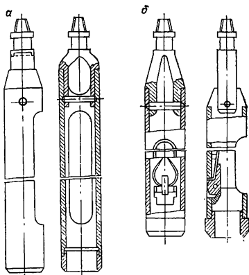
Рис. 5.17. Виброзонды: а — для бурения связных пород; б — с клапаном
