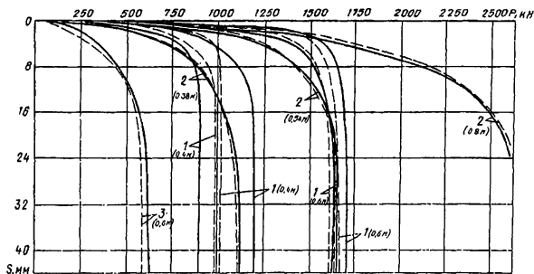
Рис. 2.6.28. Сопоставление экспериментальных графиков «осадка — нагрузка» для свай НС с рассчитанными по предлагаемой методике на опытных площадках:
