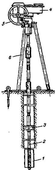
Рис. 2.4.4. Установка СП-52 для испытания горных пород на сдвиг в скважинах, конструкции ГПН «Фундамент-проект»: 1 — крыльчатка; 2 — штанга; 3 — центрирующие муфты; 4 — измерительное и вращательное устройство; 5 — штурвал; 6 — штатив
