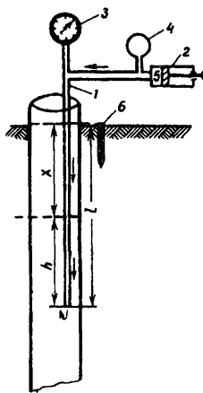
Рис. 3.11. Схема пневматического уровнемера: 1 — трубка; 2 — воздушный насос; 3 — манометр; 4 — баллон; 5 — клапан; 6 — репер
