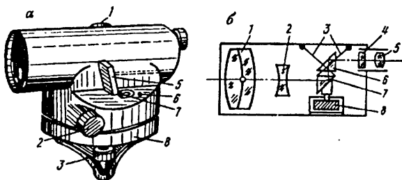
Рис. 1.97. Нивелир Н-3К: а — общий вид: 1 — головка фокусирующего устройства; 2 — головка наводящего винта; 3 — подъемный винт; 4 — окуляр; 5 — зеркало круглого уровня; 6 — исправительный винт круглого уровня; 7 — круглый уровень; 8 — подставка; б — оптическая схема компенсатора: 1 — объектив; 2 — фокусирующая линза; 3 — нити подвески; 4 — пластина сетки нитей; 5 — окуляр; 6 — неподвижная призма; 7 — подвешенная призма; 8 — успокоитель колебаний
