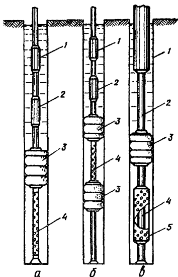
Рис. 3.14. Схемы применения снаряда ИСВ: а — с одним пакером; б — с двумя пакерами (1 — поплавковый клапан, 2 — узел с манометром, 3 — пакер, 4 — фильтр), в — упрощенная компоновка узлов снаряда для откачки из-под пакерной зоны (1 — обсадные трубы, 2 — бурильные трубы, 3 — пакер, 4 — манометр, 5 — хвостовик)
