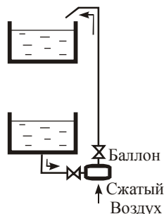
Рис. 1.10. Пневмо-подъемник
