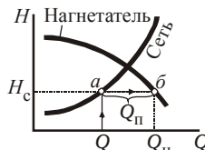
Рис. 4.20. Расчет перепуска
