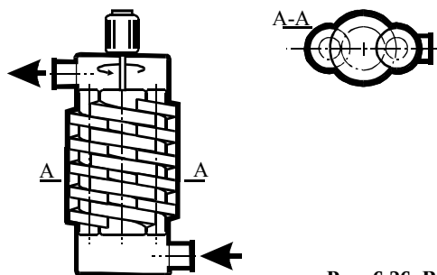
Рис. 6.26. Винтовой насос
