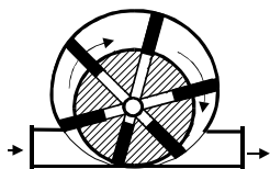
Рис. 6.24. Пластиновый роторный насос с внешней подачей
