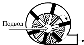
Рис. 6.25. Пластиновый роторный насос с внутренней подачей
