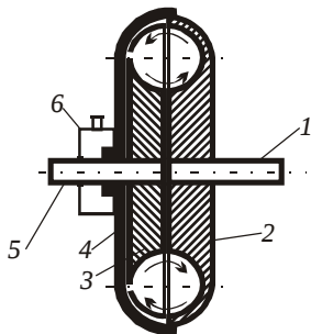
Рис. 4.21. Гидромufта:
