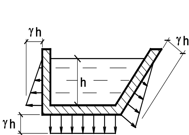
Рис. 3. Эпюры давления жидкости на плоские поверхности
