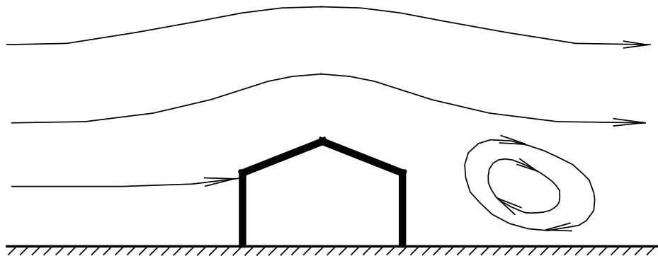
Рис. 30. Обтекание здания воздушным потоком
