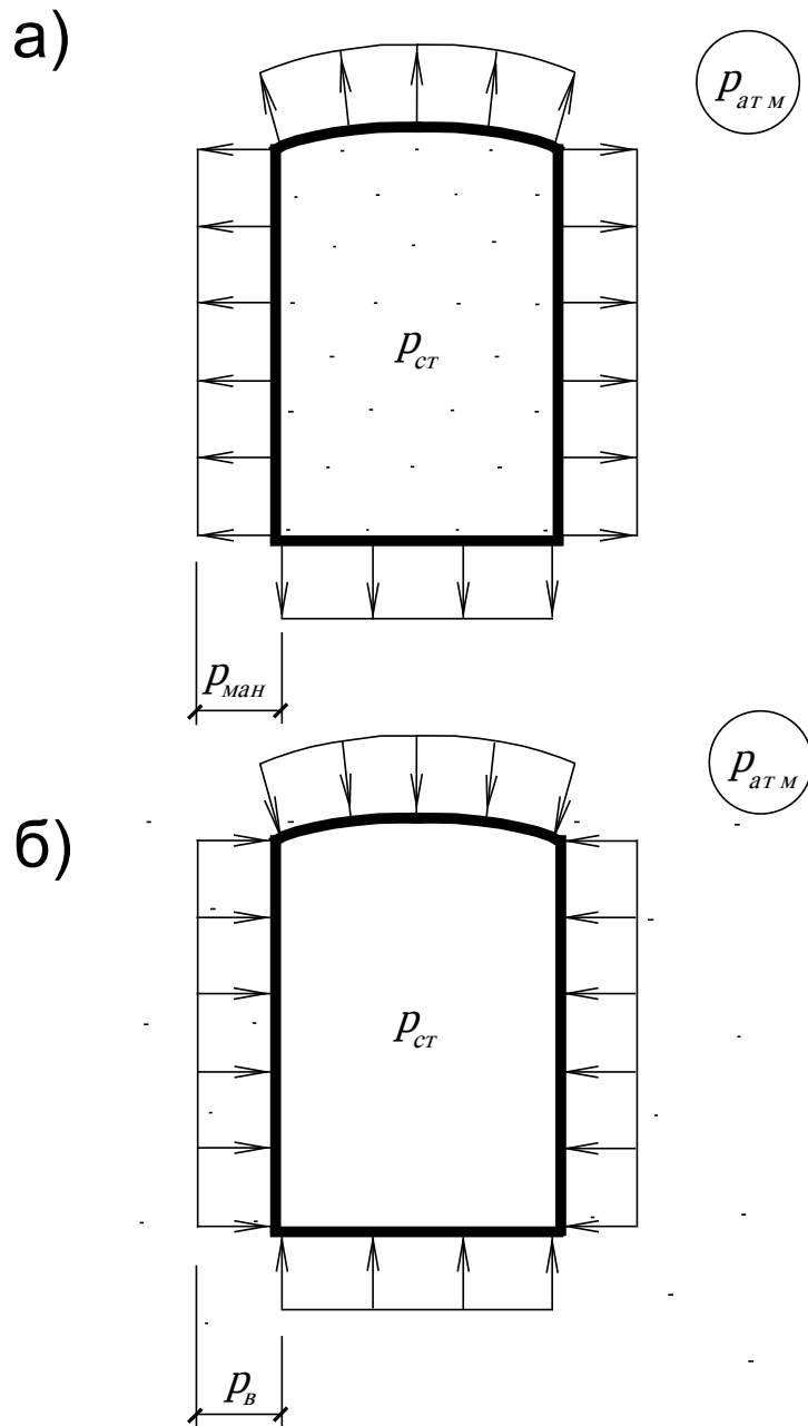
Рис. 23. Эпюры давления на поверхность резервуара: а - p_{ст} > p_{атм} ; б - p_{ст} < p_{атм}
