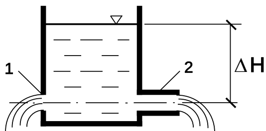
Рис 15. Истечение из отверстий и насадков : 1 - отверстие; 2 - насадок
