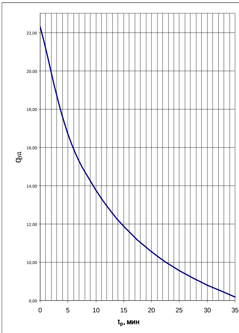
Рис. 2.2. График зависимость q_{уд} = f(t_p)
