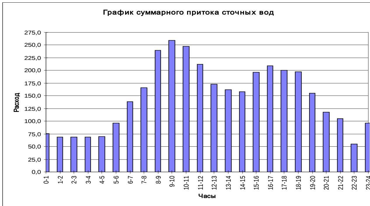
Рис. Ступенчатый график притока сточных вод на ГНС
