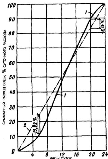
Рис. 2.10. Интегральный график водопотребления (1) и подачи воды насосами (2)
