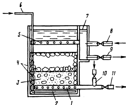
Рис. 5.21. Схема устройства каркасно-засыпного скорого фильтра: 1, 2 — водо- и воздухоподразделительные системы; 3 — песчаная засыпка в межгравийном пространстве; 4 — гравийный каркас; 5 — трубчатая перфорированная система распределения исходной и сбора промывной воды; 6 — подача воздуха; 7 — боковой карман; 8, 11 — подача исходной и отвод фильтрованной воды; 9, 10 — отвод и подача промывной воды
