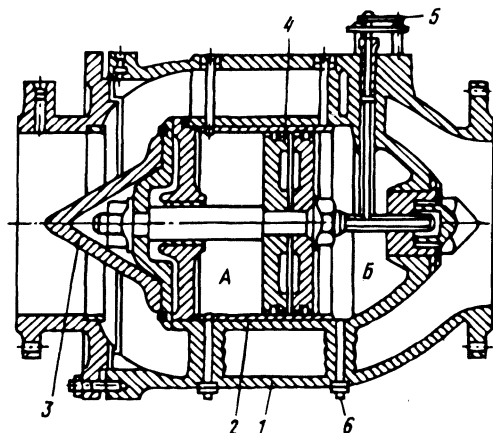
Рис. 3.17. Кольцевая задвижка:
