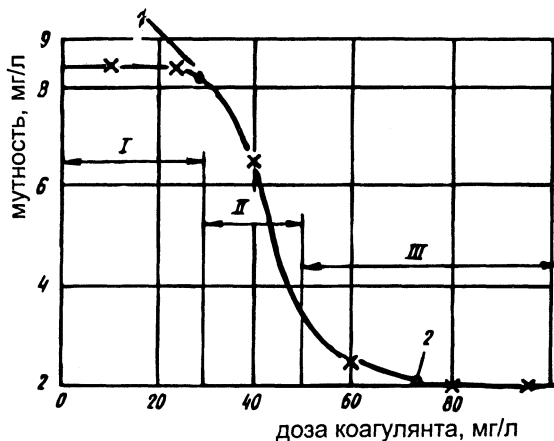
Рис. 5.3. Коагуляционная кривая:
