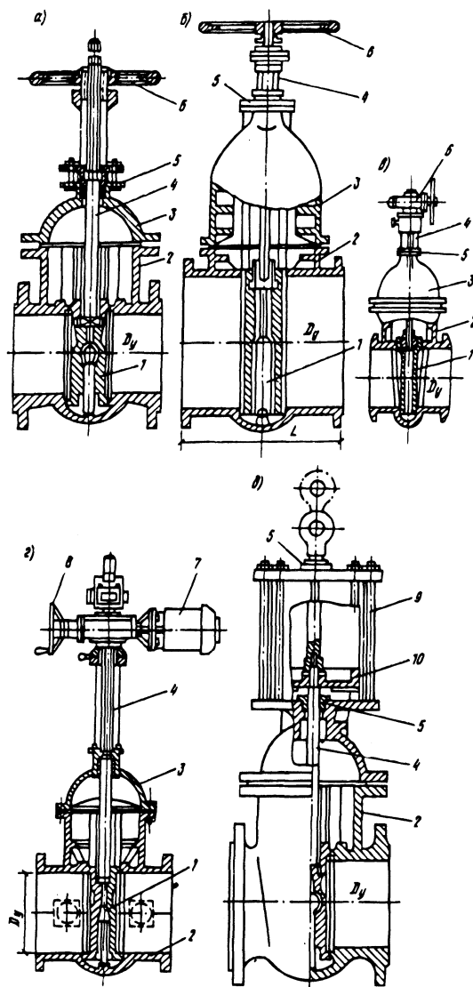
Рис. 3.16. Схемы затворек:
