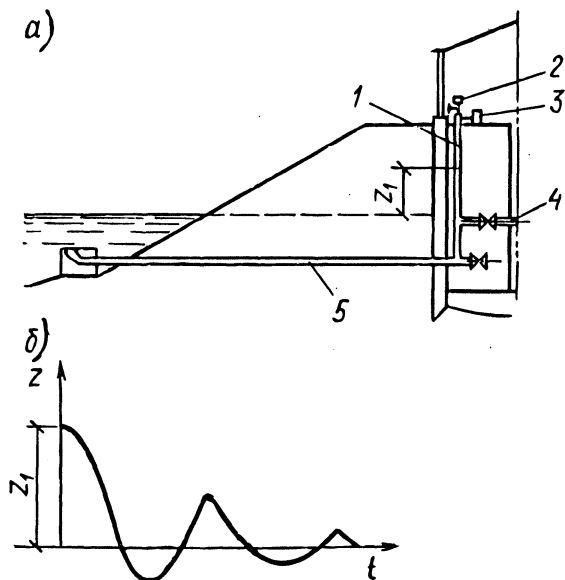
Рис. 4.23. Схема импульсной промывки сороудерживающих решеток (а) и график изменения уровня воды в колонне (б): 1 — колонна на самотечном водоводе; 2 — патрубок с затвором для впуска воздуха; 3 — вакуум-насос; 4 — трубопровод для промывки решеток обратным током воды; 5 — самотечный водовод; z_1 — столб воды, поднятый вакуумом
