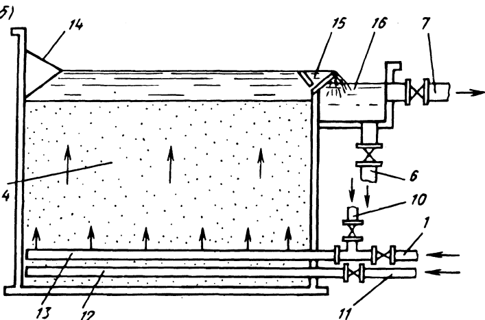
Рис. 5.23. Контактные осветители КО-1 (а) и КО-3 (б):
