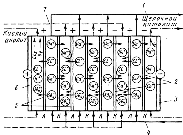
Рис. 5.31. Схема многокамерного электродиализного аппарата: 1, 4 — отвод обессоленной и подача исходной воды; 2, 5 — ионо-селективные катионитовые и анионитовые мембраны; 3 — катод; 6 — анод; 7 — отвод концентрата
