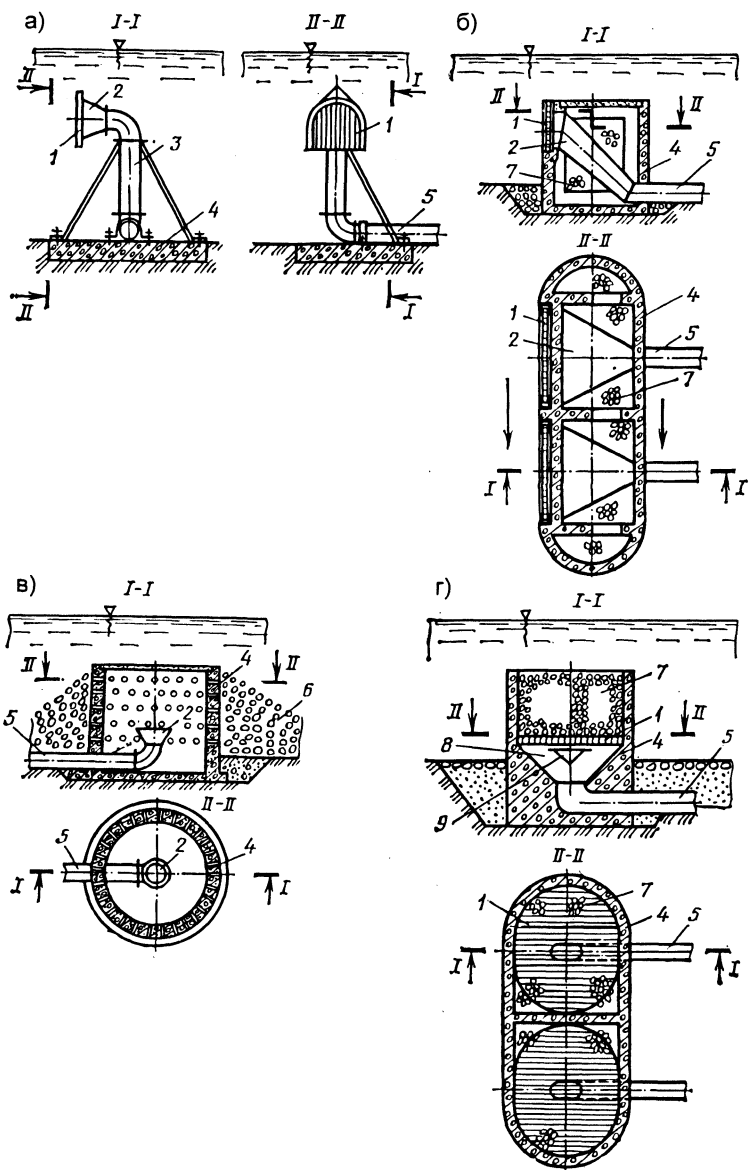
Рис. 4.20. Типы оголовков:
