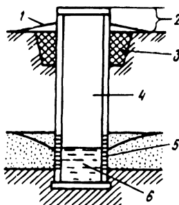
Рис. 4.5. Схема шахтного колодца:
