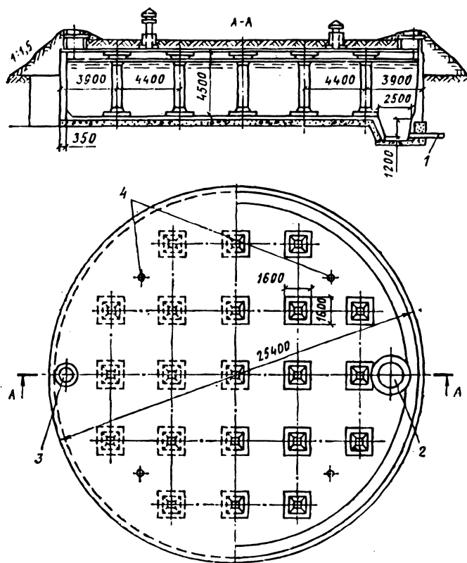
Рис. 2.15. Конструкция резервуара цилиндрической формы: 1 — грязевая труба; 2 — прямок; 3 — лаз; 4 — вентиляционные трубопроводы
