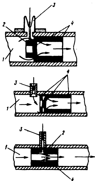
Рис. 5.7. Трубчатые смесители:
