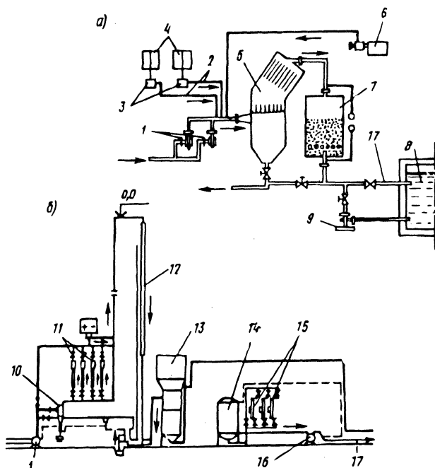
Рис. 5.34. Схема установки АзНИИ ВП «Струя» (а) и ВНИИГиМ (б): 1 — насос I подъема; 2 — подача реагентов; 3 — насос-дозатор; 4 — реакгентное хозяйство; 5 — тонкослойный отстойник; 6 — электролизер для обеззараживания воды; 7 — напорный скорый фильтр; 8 — резервуар чистой воды; 9 — промывной насос; 10 — гидроциклон; 11 — электрокоагулятор; 12 — воздухоохладитель; 13 — самопромывающийся скорый фильтр; 14 — пневматический бак; 15 — бактерицидная установка; 16 — электронасос; 17 — отвод обработанной воды
