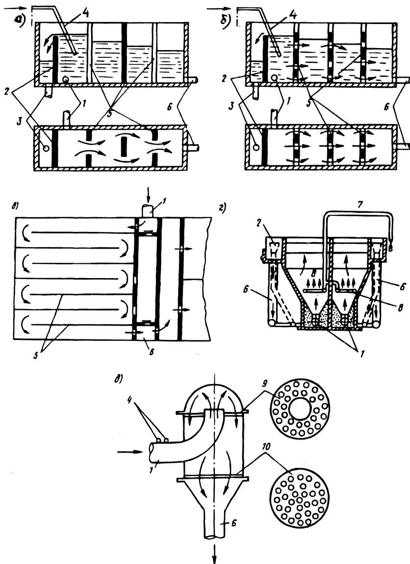
Рис. 5.6. Смесители гидравлического типа с разделением потока (а), дырчатый (б), перегородчатый (в), вихревой (г):
