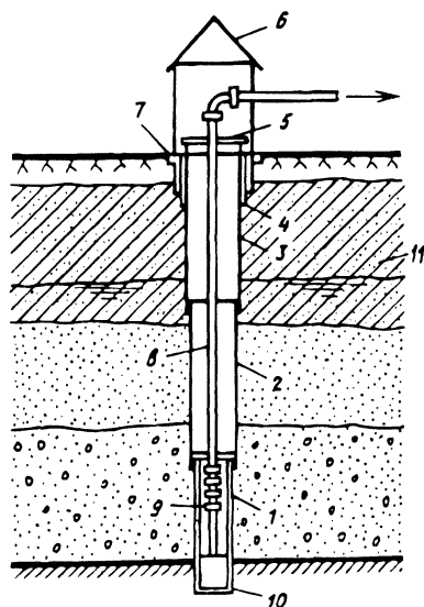
Рис. 4.2. Водозаборная скважина:
