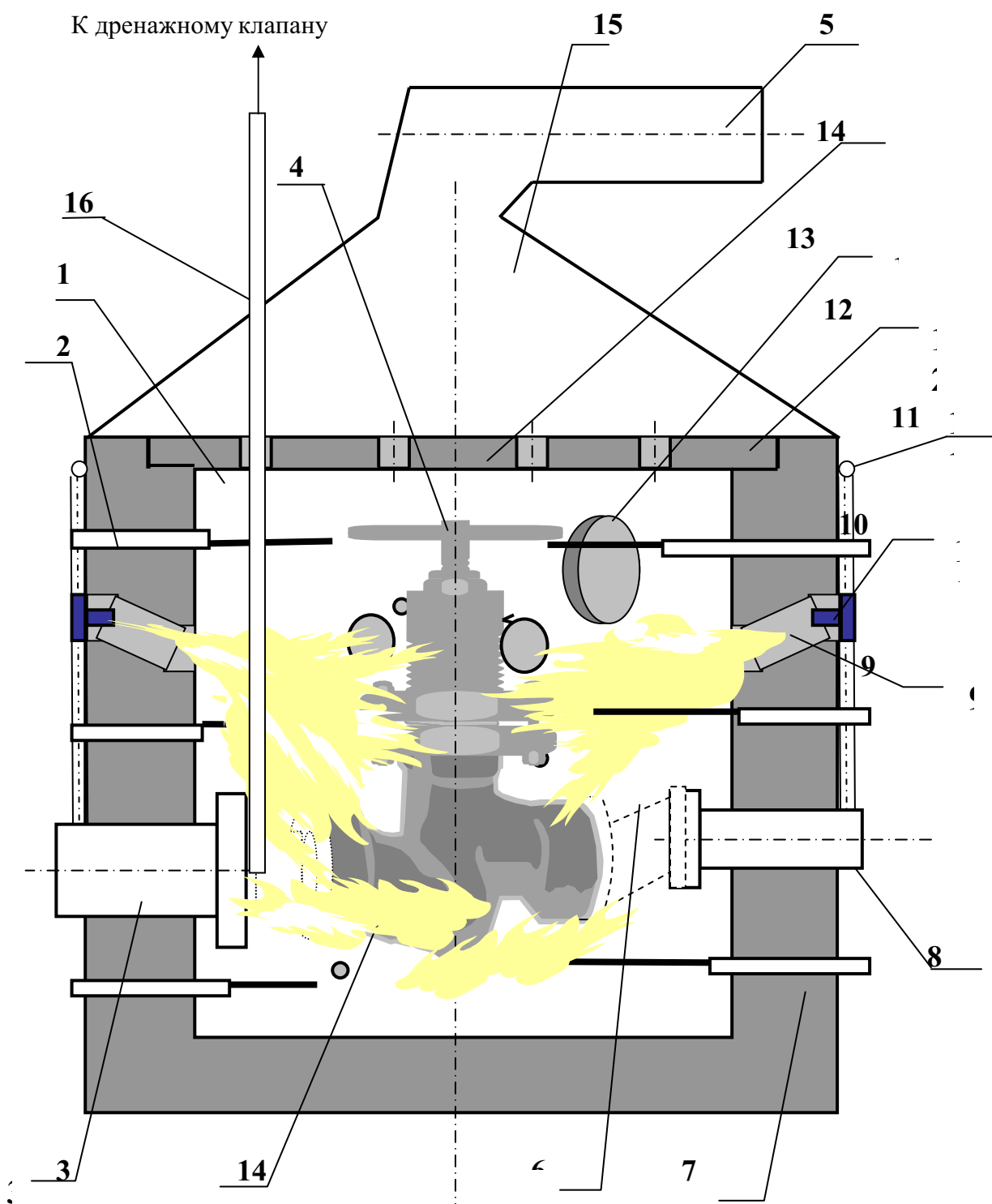
Рисунок 2 - Установка для огневых испытаний трубопроводной арматуры:
