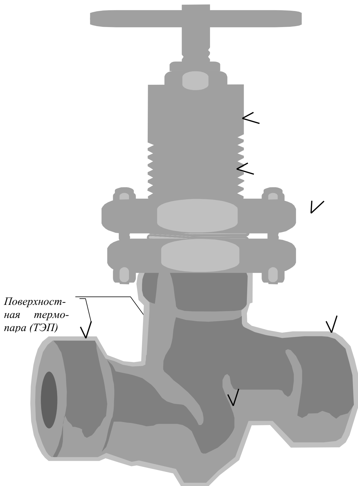
Рисунок 3- Принципиальная схема расстановки ТЭП на поверхности ИА.
