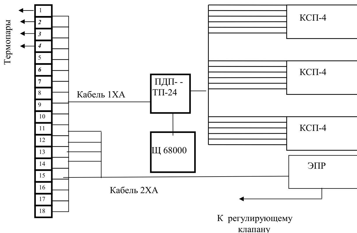
Рисунок 4 - Измерительная схема стенда
