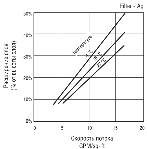
Рис. 2.5. Расширение слоя во время обратной промывки
