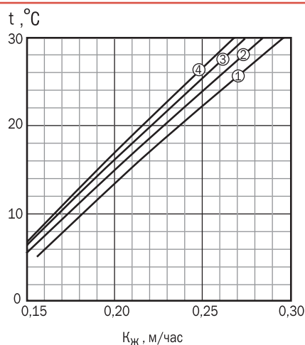
Рис. 1.6. График для определения K_{ж} при удалении углекислоты в процессе обезжелезивания воды аэрацией. Площадь орошения насадки 90 \text{ м}^3 / (\text{м}^2 \cdot \text{ч}) :
