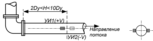
Установка ПП-1 после "колена"
