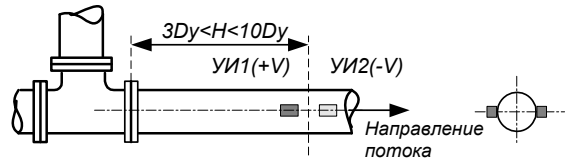
Установка ПП-1 после "тройника"
