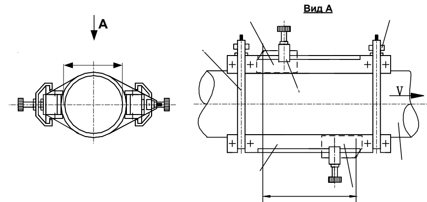
Вариант крепления с помощью зажима
