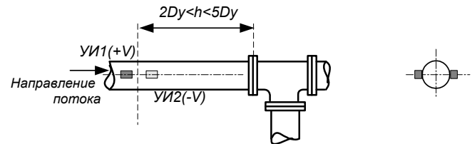
Установка ПП-1 до "тройника"
