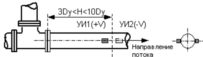
Установка ПП-1 после "тройника"
