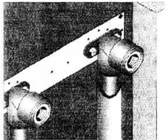
Настенные пластины для двойного подключения арматуры с монтажной платой.
