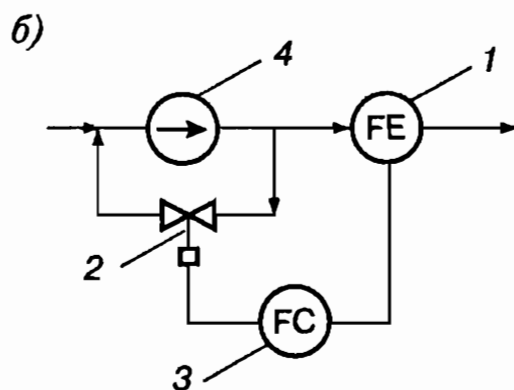
Рис. 53. Схема регулирования расхода после центробежного (а) и поршневого (б) насосов:
