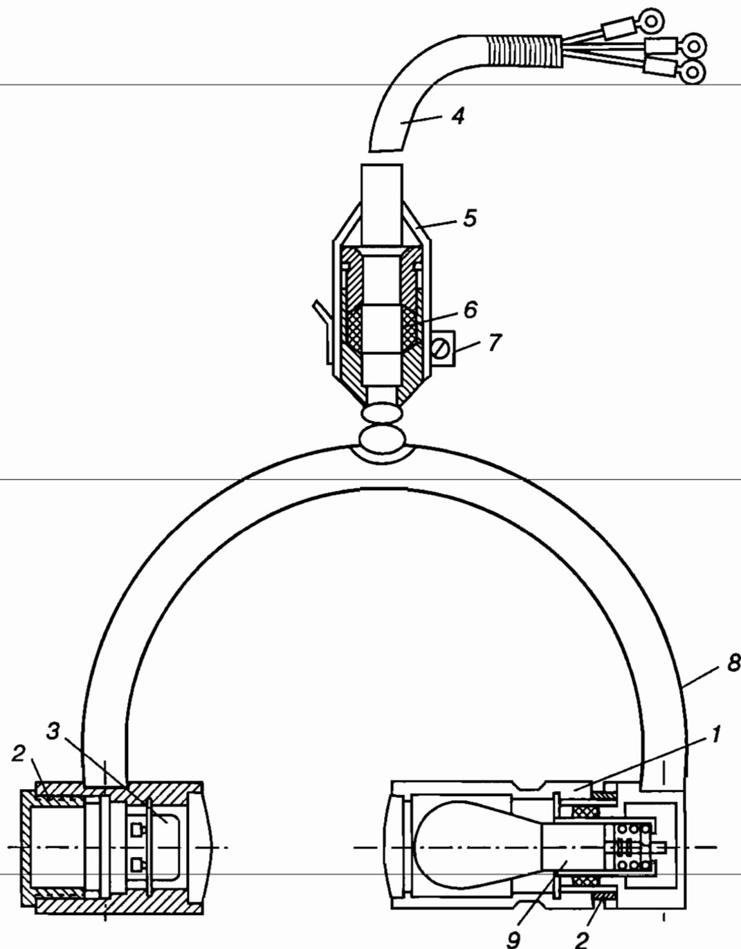
Рис. 105. Автоматический сигнализатор уровня осадка:
