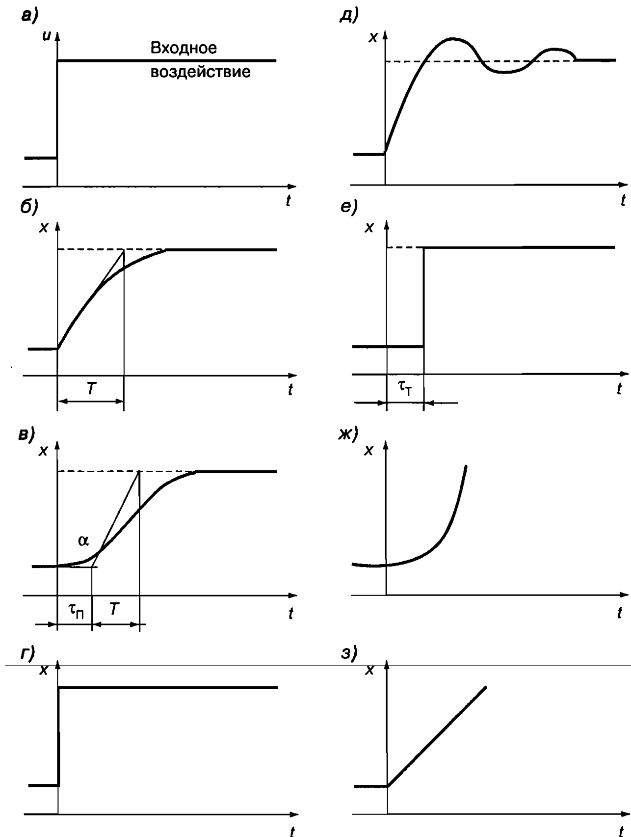
Рис. 33. Типичные переходные процессы в объектах регулирования при скачкообразном входном воздействии:
