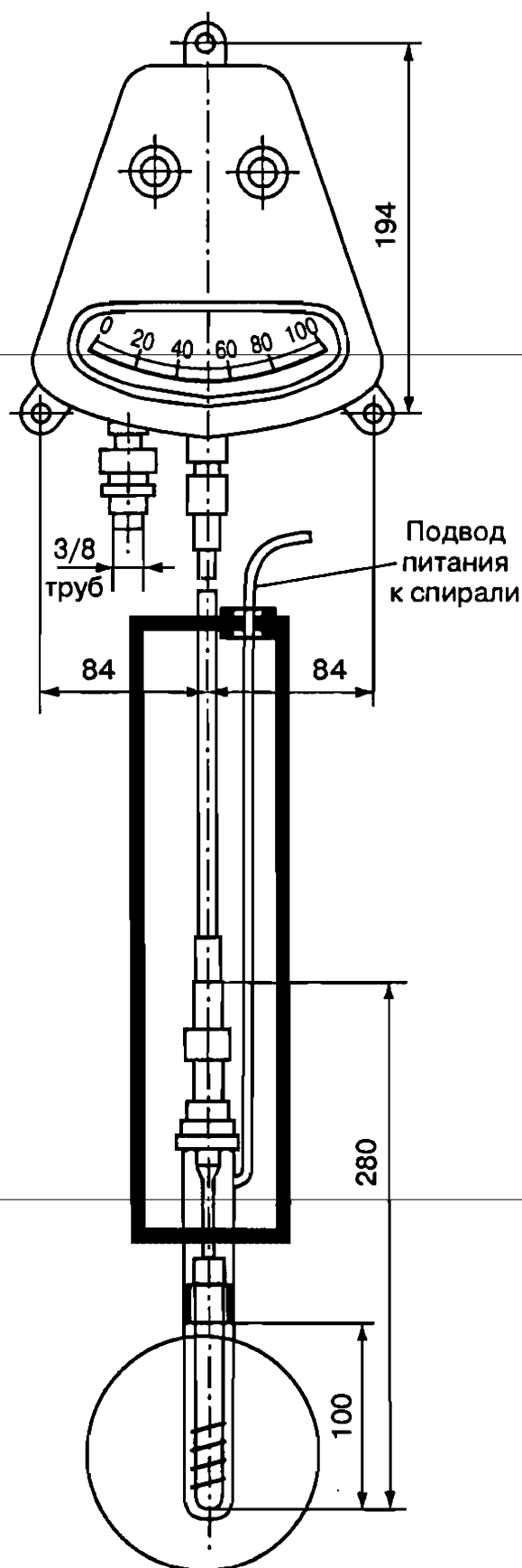
Рис. 104. Прибор для контроля уровня песка в песколовках
