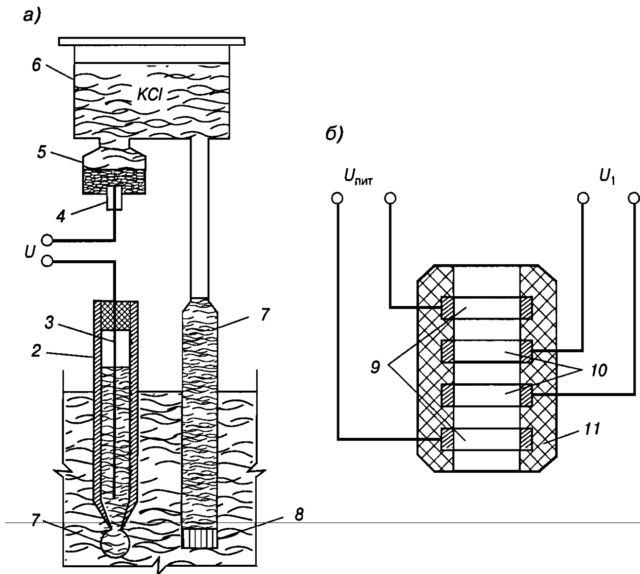
Рис. 25. Измерительные преобразователи анализаторов жидкости:
