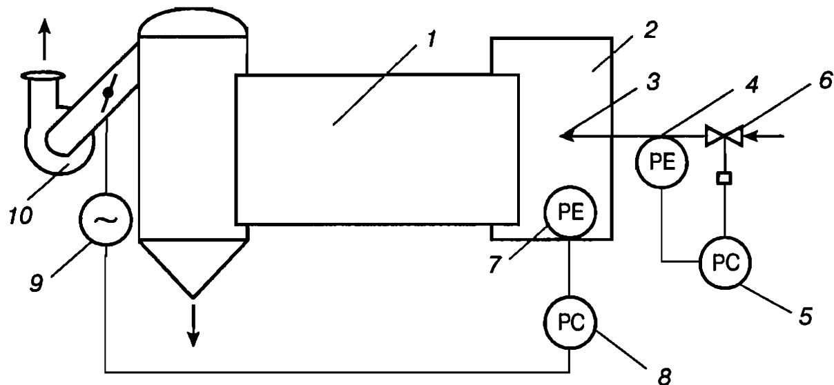
Рис. 61. Схема регулирования давления (разрежения) в барабанной сушилке:
