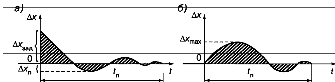
Рис. 35. Переходные процессы в АСР при скачкообразных входных воздействиях:
