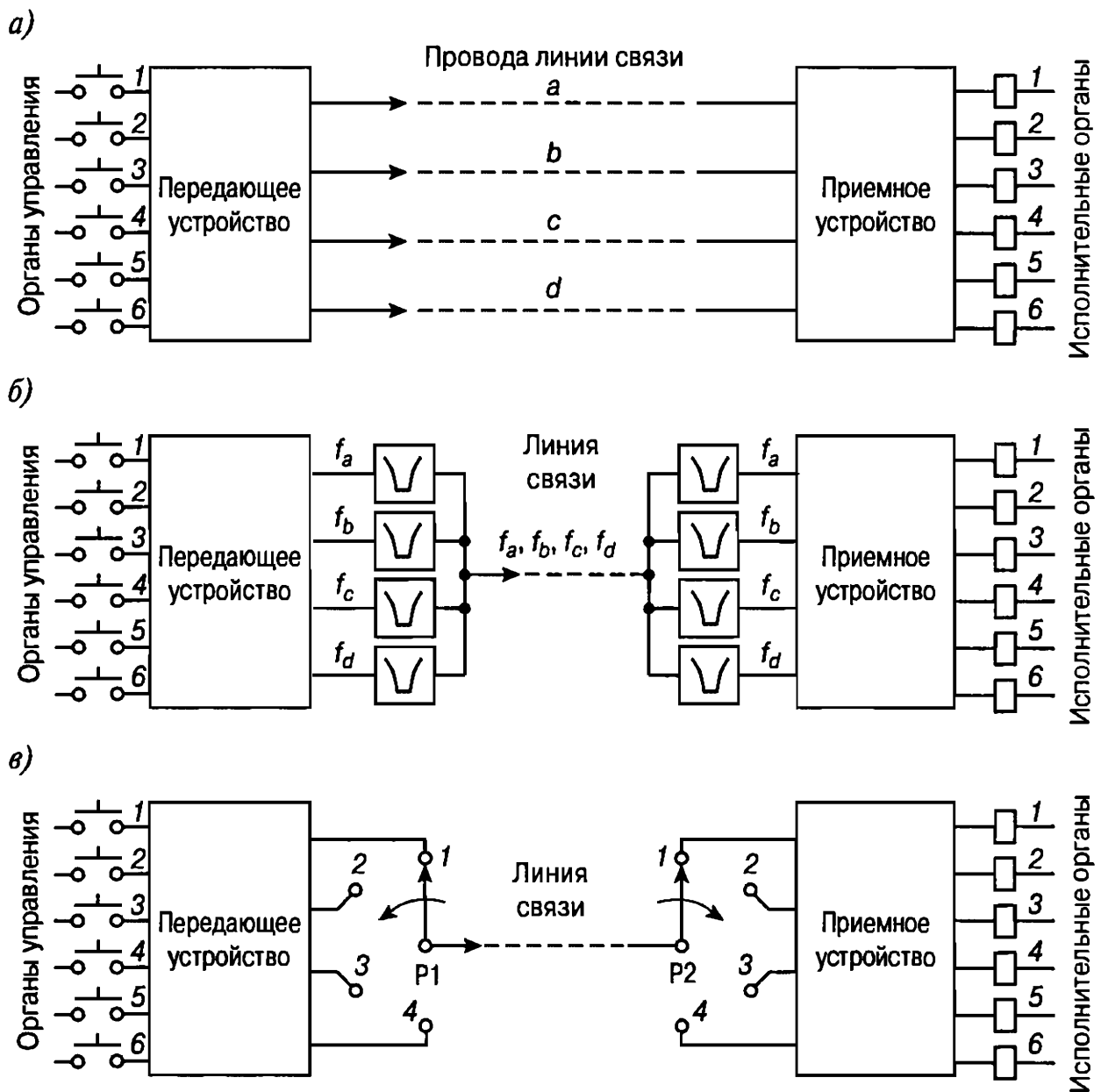
Рис. 79. Принципиальная схема устройства телеуправления
