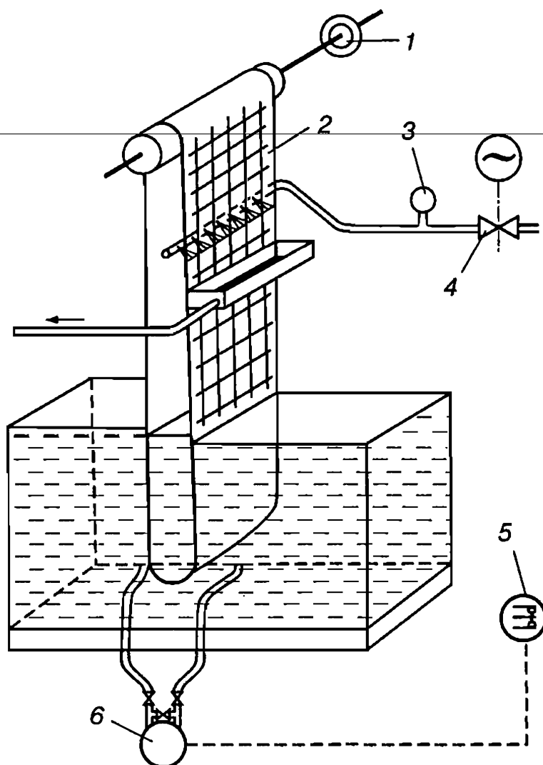
Рис. 87. Схема автоматизированной ленточной вращающейся сетки
