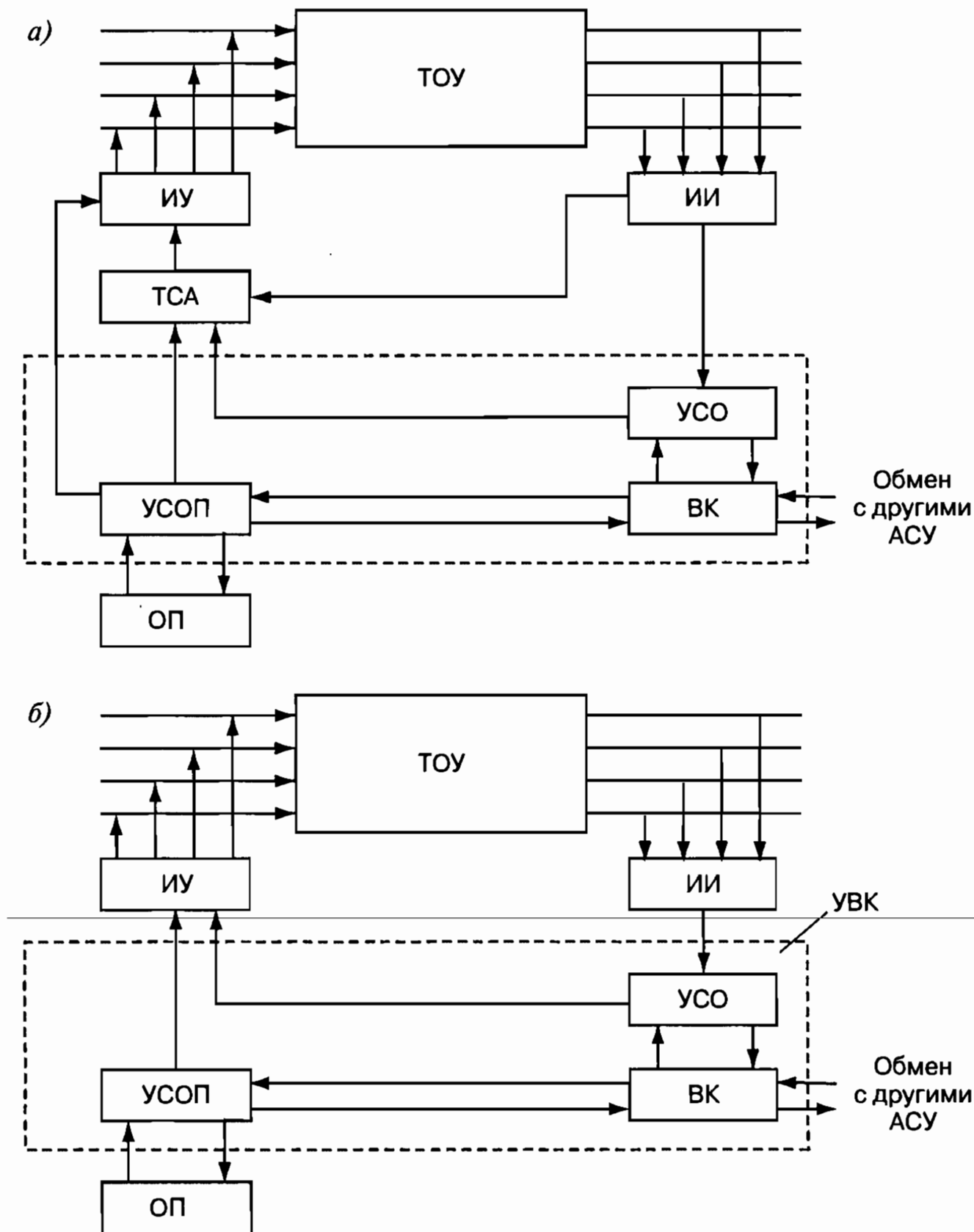
Рис. 114. Техническая структура КТС АСУ ТП:
