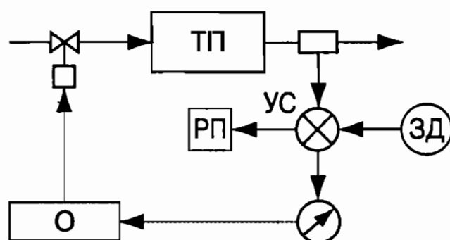
Рис. 9. Схема системы автоматического контроля
