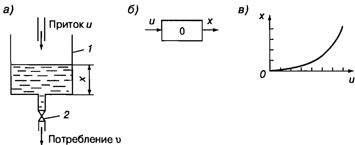
Рис. 31. Емкость как объект регулирования:
