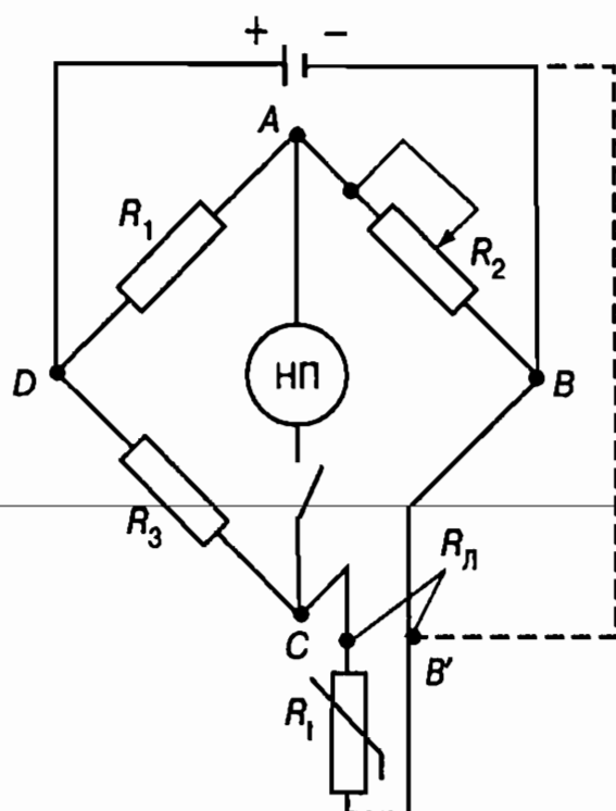
Рис. 23. Принципиальная схема уравновешенного моста с термометром сопротивления
