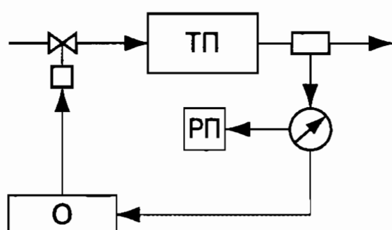
Рис. 8. Схема системы автоматической индикации
