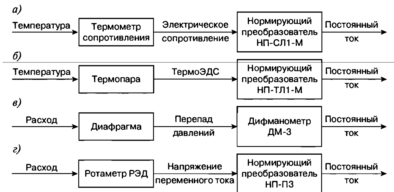
Рис. 40. Примеры измерительных цепей регулятора «Ремиконт»:
