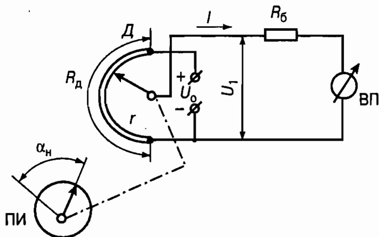
Рис. 77. Схема двухпроводной телеизмерительной системы с реостатным датчиком
