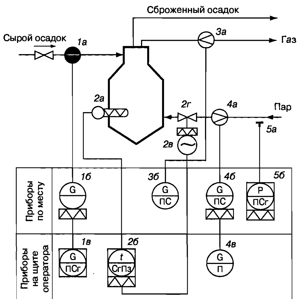
Рис. 108. Схема АСР температуры в метантенке:
