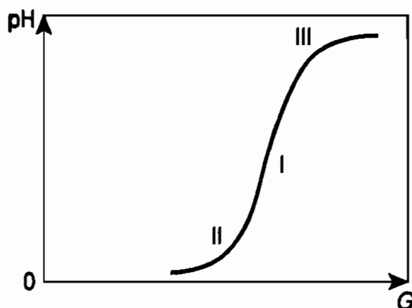
Рис. 70. Зависимость величины рН от расхода реагента
