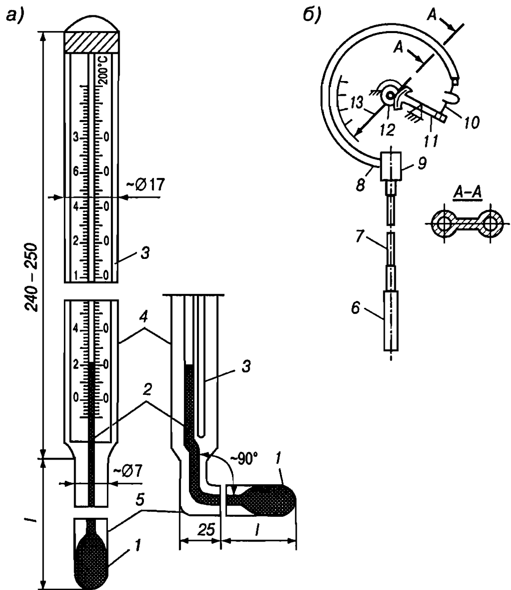
Рис. 21. Термометры расширения:
