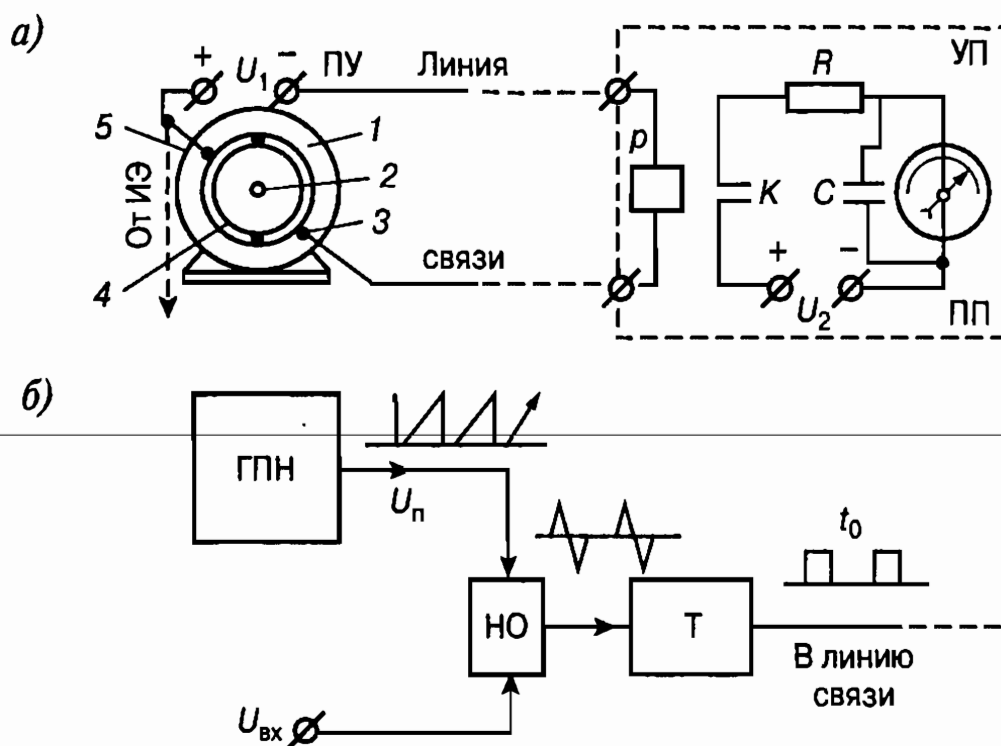
Рис. 78. Время-импульсная схема телеизмерения:
