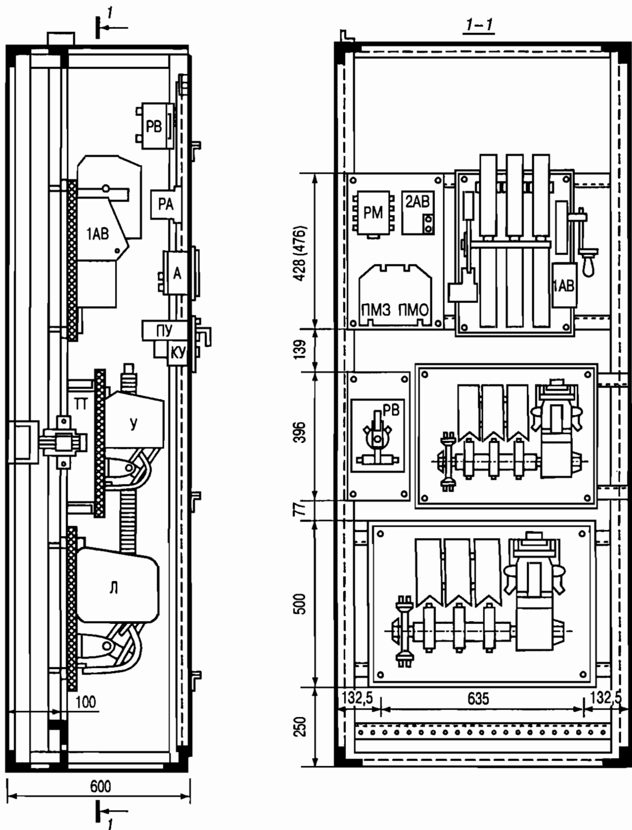
Рис. 81. Общий вид станций управления СУНО
