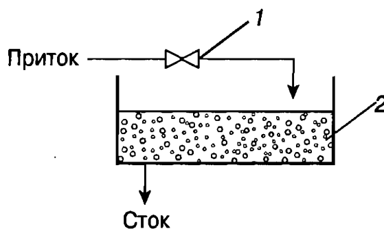
Рис. 4. Ручное регулирование уровня с притоком и стоком жидкости:
