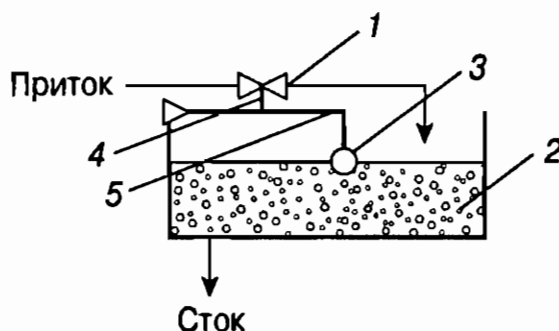
Рис. 5. Автоматическое регулирование уровня с притоком и стоком жидкости:
