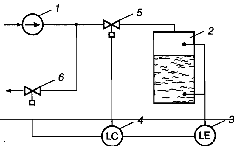
Рис. 56. Схема позиционного регулирования уровня:
