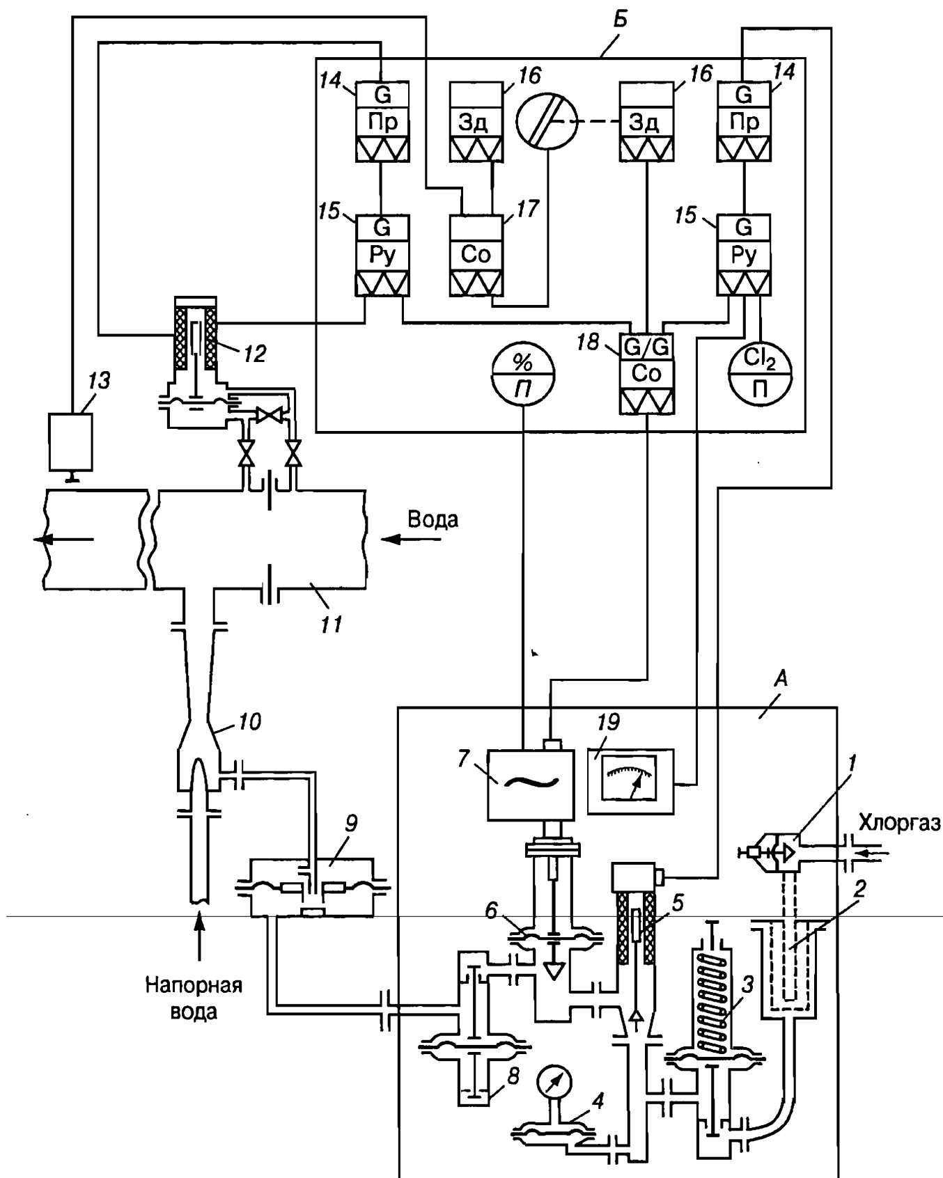
Рис. 96. Схема автоматического хлоратора:
