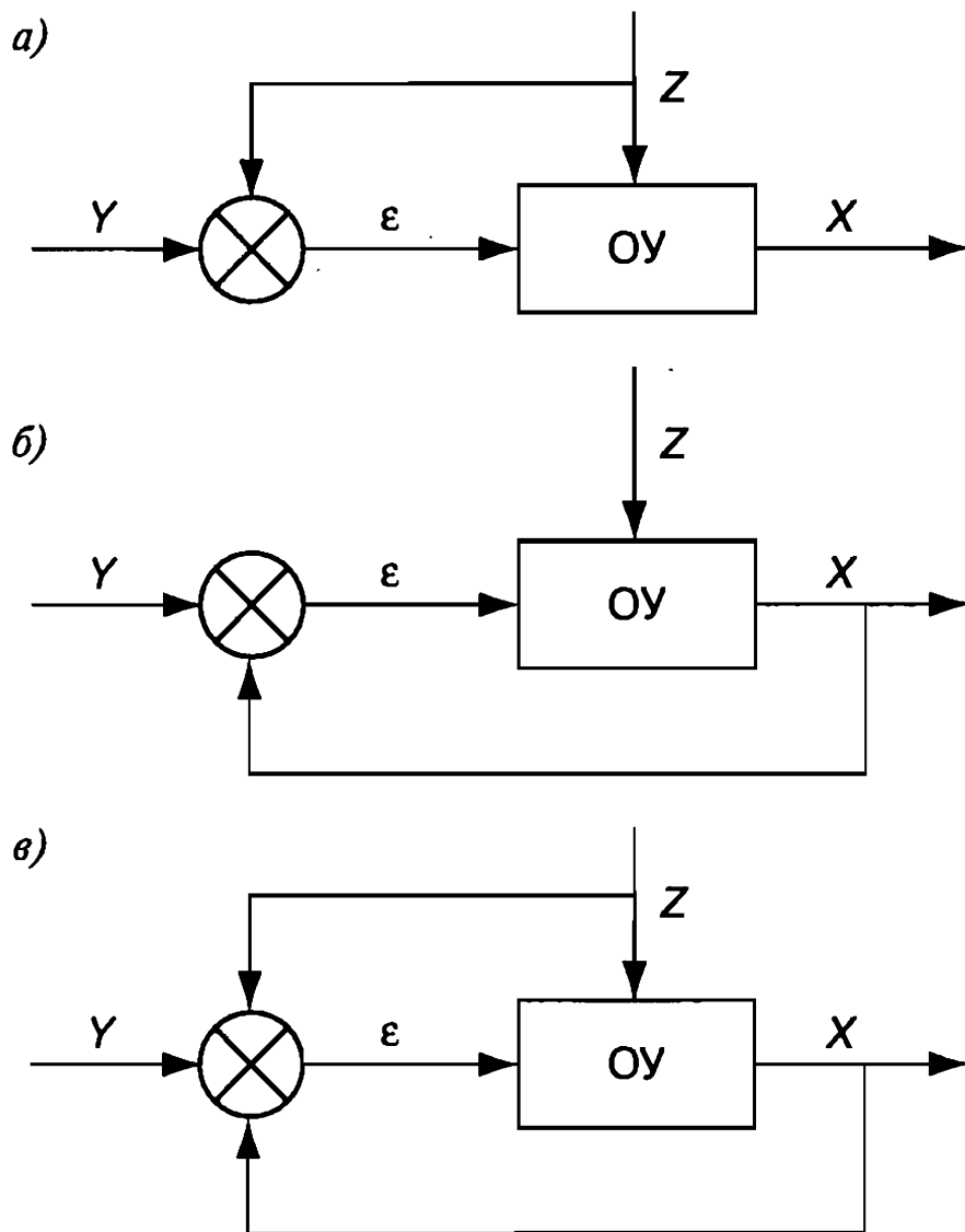
Рис. 7. Схемы регулирования по возмущению (а), отклонению (б), комбинированная (в)
