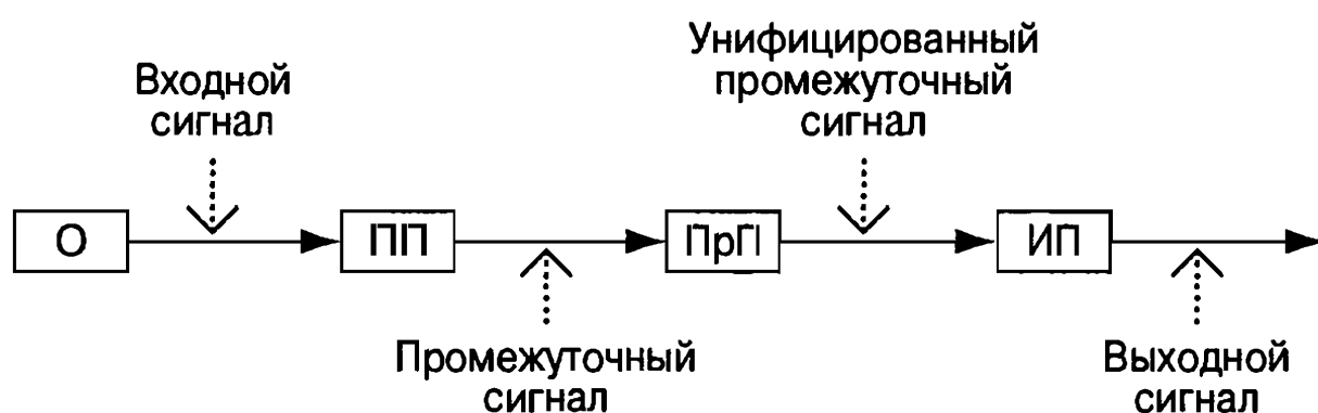
Рис. 10. Блок-схема измерительной цепи:
