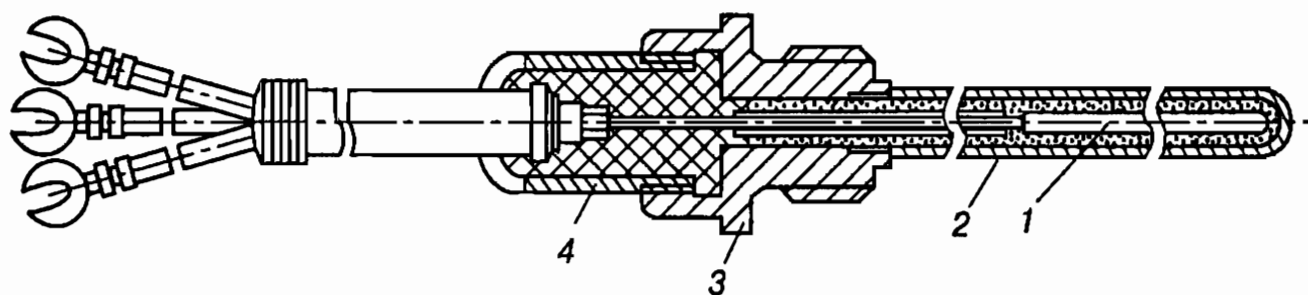
Рис. 22. Конструкция термометра сопротивления
