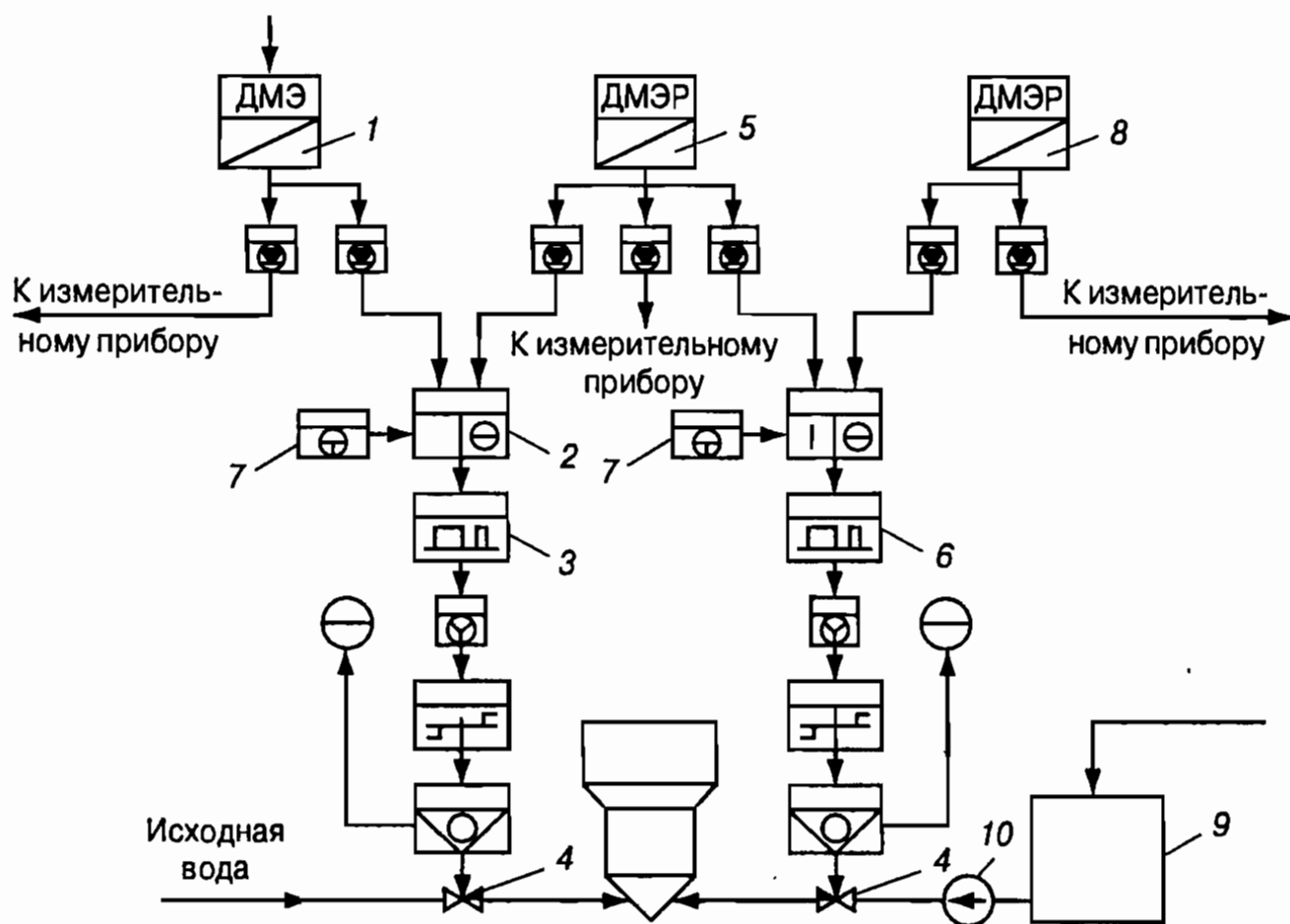
Рис. 92. Схема АСР гидравлической нагрузки на осветлитель:
