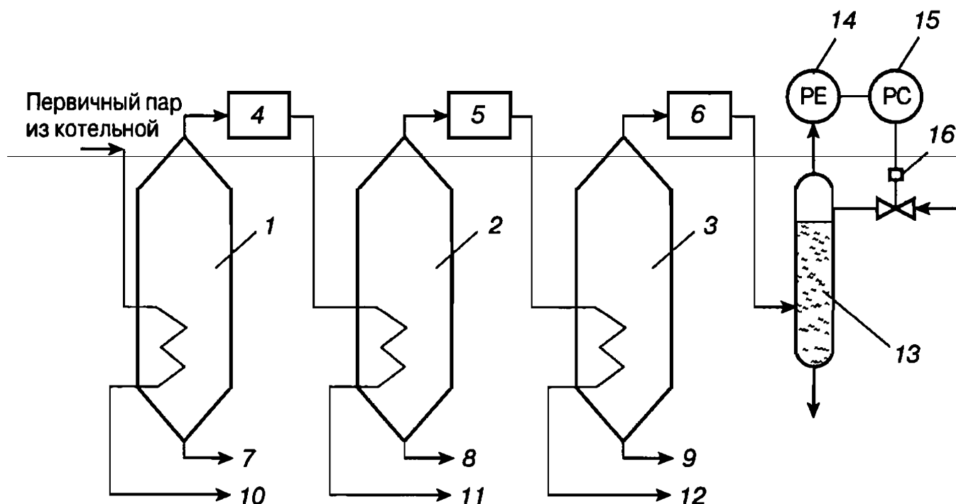
Рис. 60. Регулирование разрежения в многоступенчатой дистилляционной установке:
