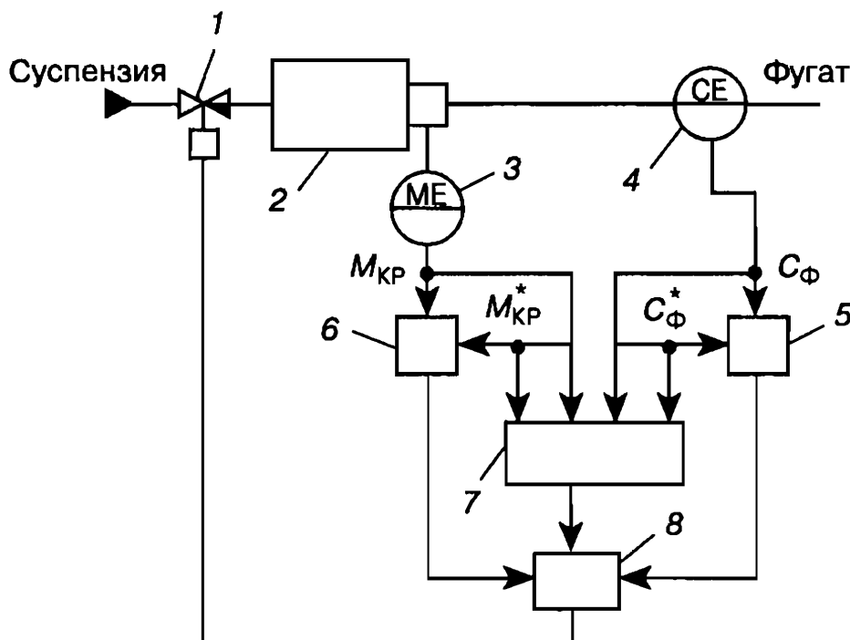
Рис. 111. Схема АСР шнековой центрифуги:
