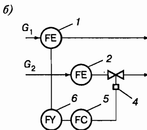
Рис. 54. Схема регулирования соотношения расходов при незаданной общей нагрузке:
