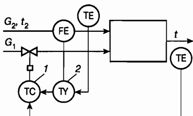
Рис. 69. Функциональная схема комбинированной АСР температуры:
