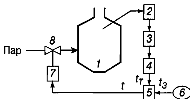
Рис. 2. Регулируемый тепловой режим сбраживания осадков сточных вод как система управления
