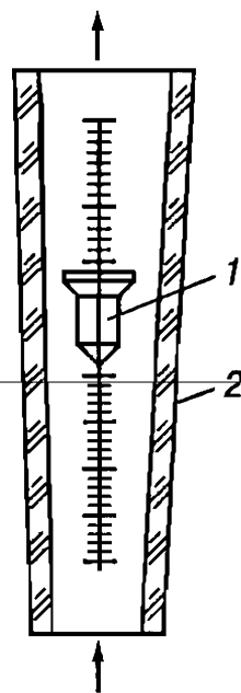
Рис. 16. Расходомер постоянного перепада давления (ротаметр)
