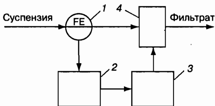
Рис. 109. Схема АСР фильтра периодического действия ФПАКМ-25:
