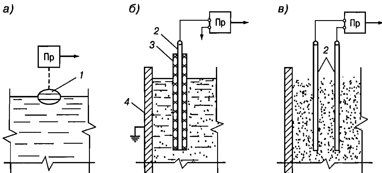
Рис. 20. Уровнемеры:
