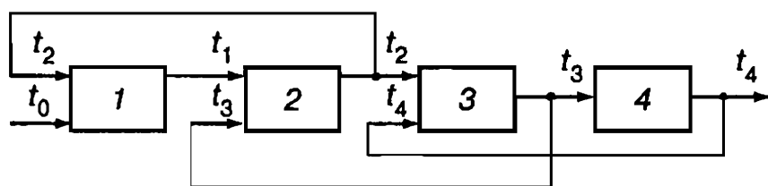
Рис. 63. Структурная схема маномерического термометра
