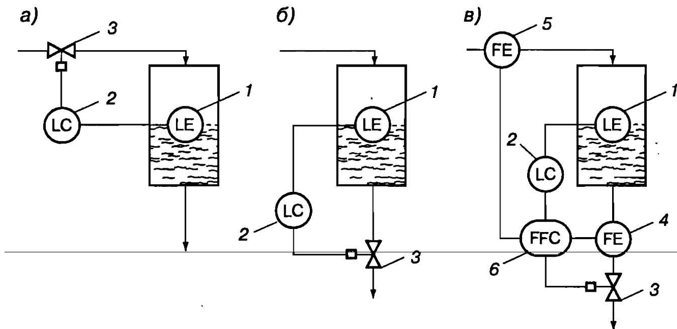
Рис. 57. Схемы непрерывного регулирования уровня:
