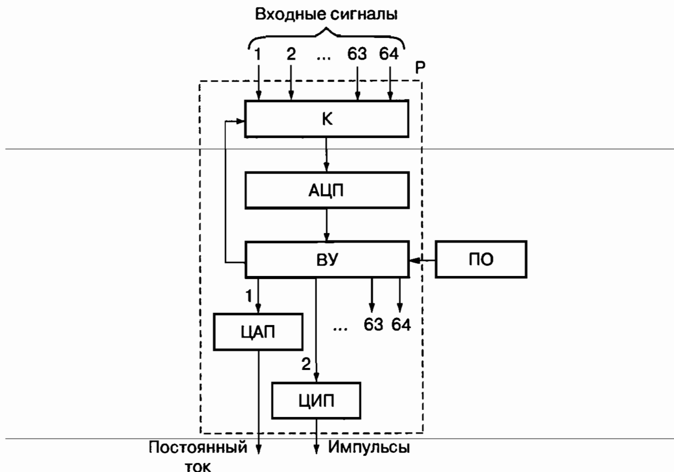
Рис. 41. Структурная схема регулятора «Ремиконт»:
