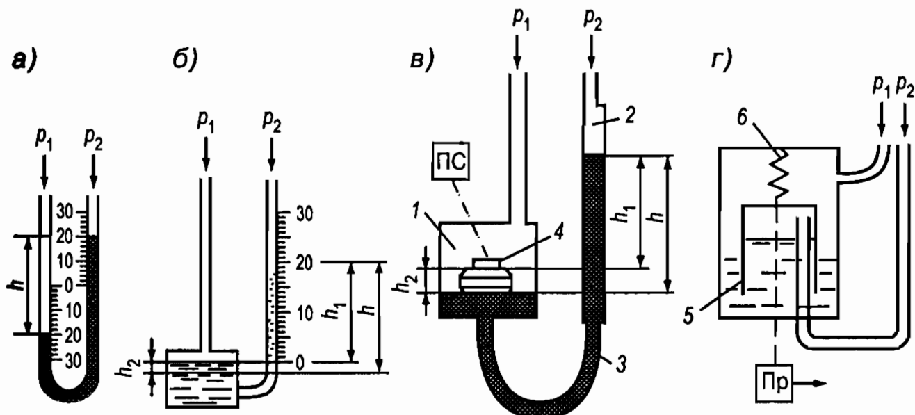
Рис. 11. Жидкостные манометры:
