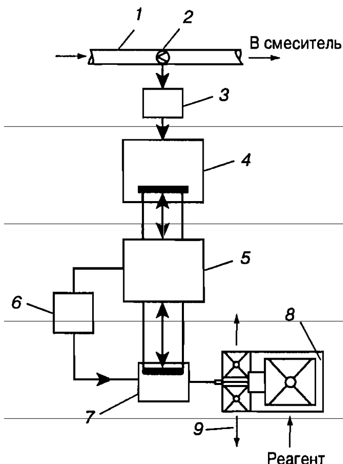
Рис. 90. Схема АСР подачи коагулянта с применением бака-дозатора:
