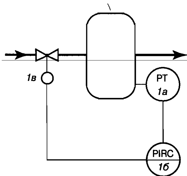
Рис. 59. Функциональная схема АСР давления
