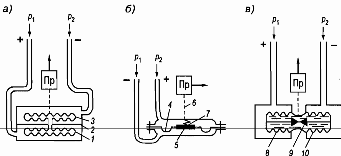
Рис. 13. Дифференциальные манометры с упругим чувствительным элементом (деформационные):
