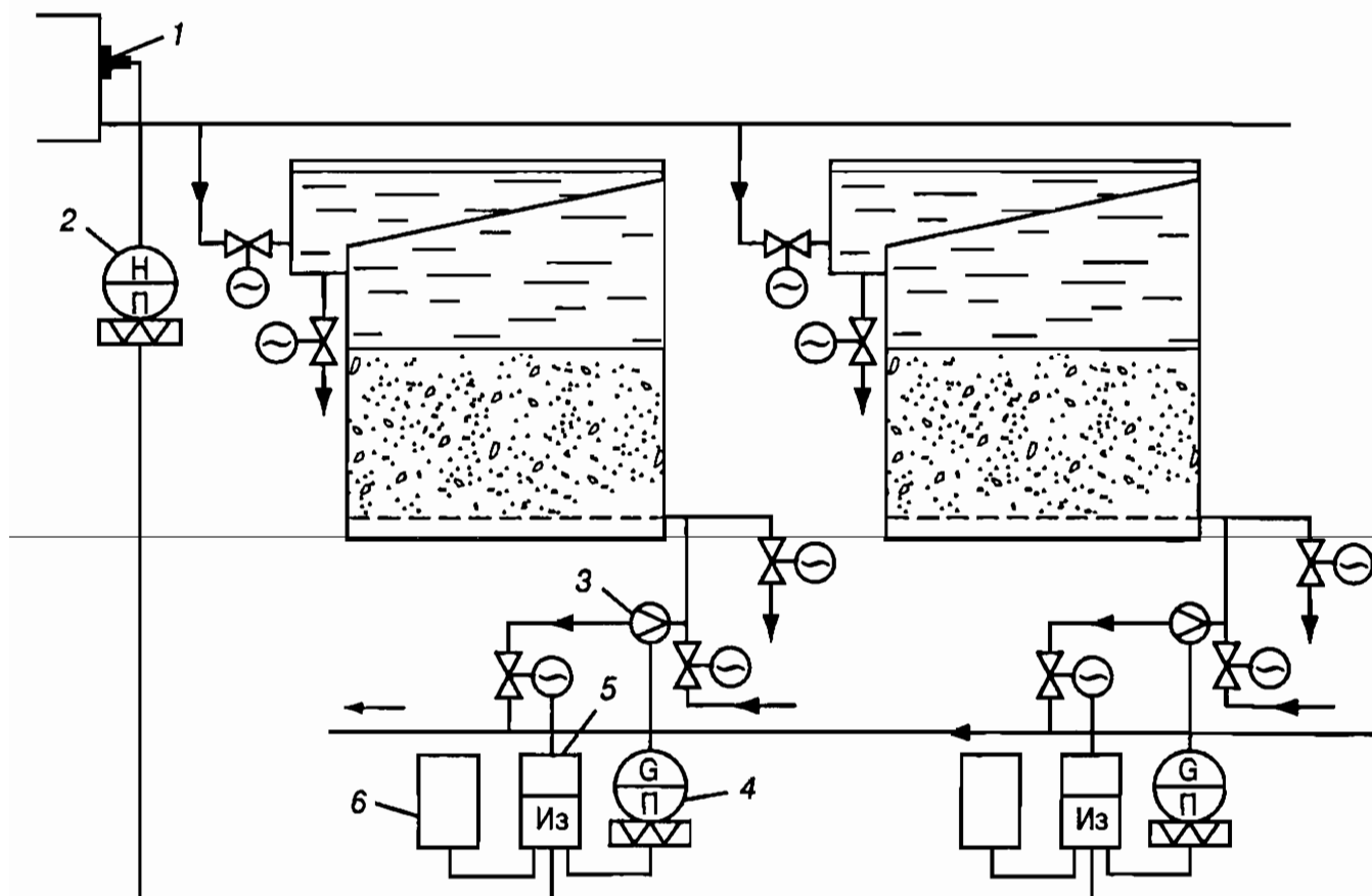
Рис. 95. Схема АСР производительности фильтров по притоку воды на станцию:
