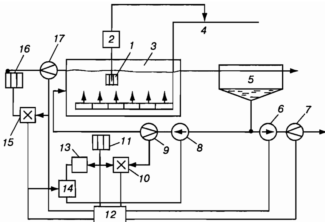
Рис. 107. Схема АСР процесса очистки сточных вод в аэротенке по ХПК исходной сточной воды и концентрации активного ила
