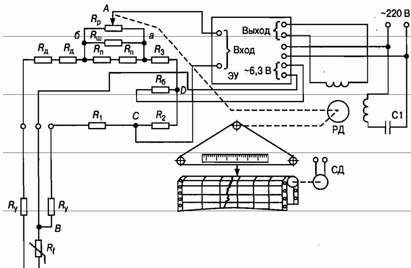
Рис. 24. Принципиальная схема автоматического электронного уравновешенного моста типа КСМ-4
