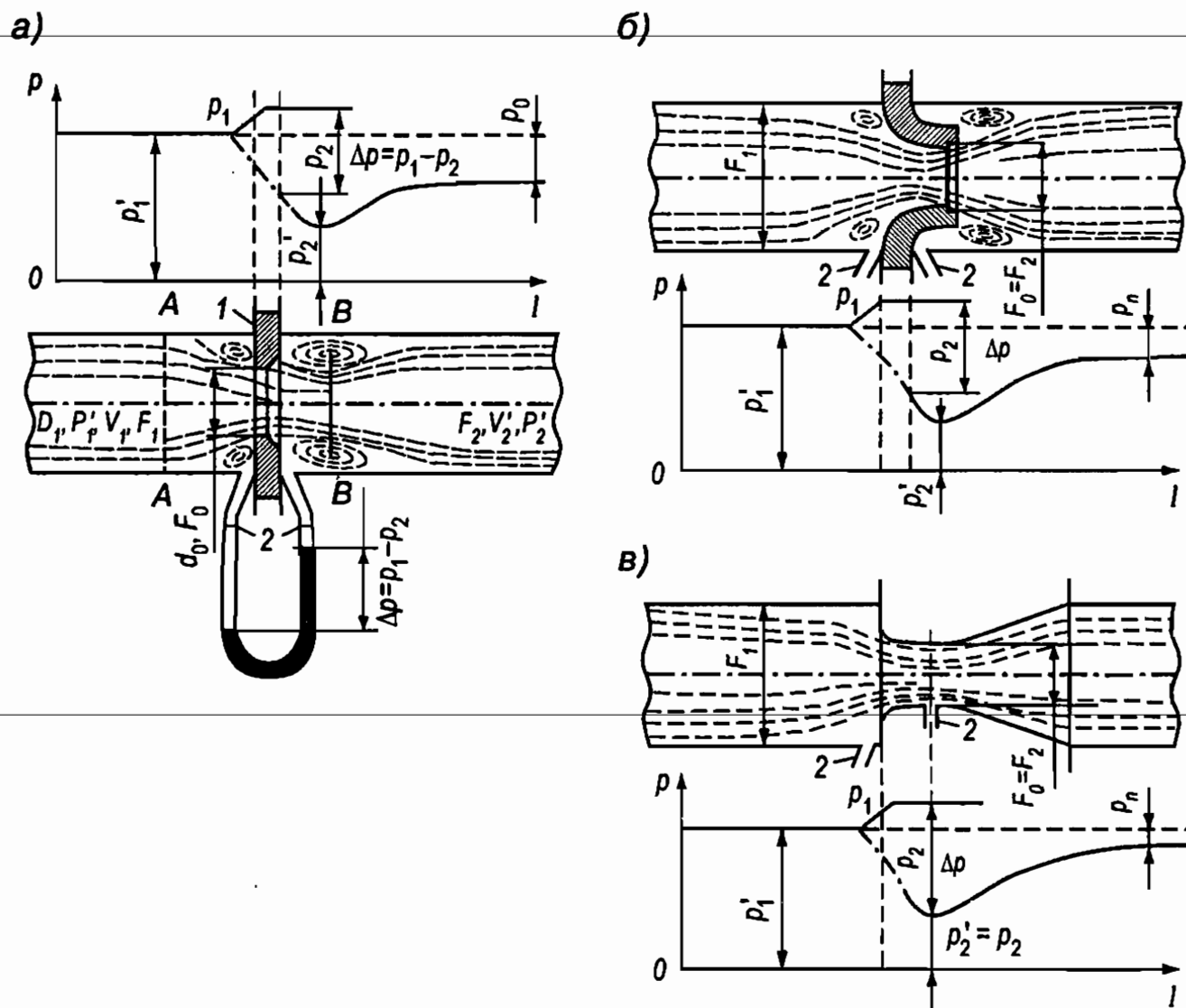
Рис. 14. Характер потока и распределения статического давления при установке в трубопроводах диафрагмы (а), сопла (б) и сопла Вентури (в)
