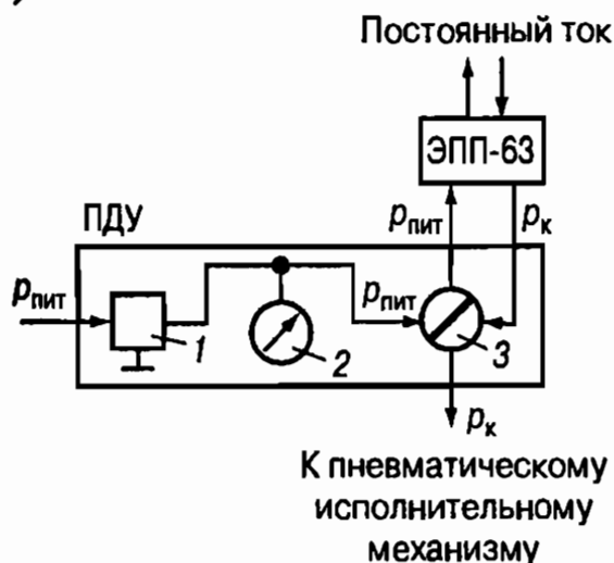
Рис. 42. Схема соединения регулятора «Ремиконт» с пневматическим исполнительным механизмом:
