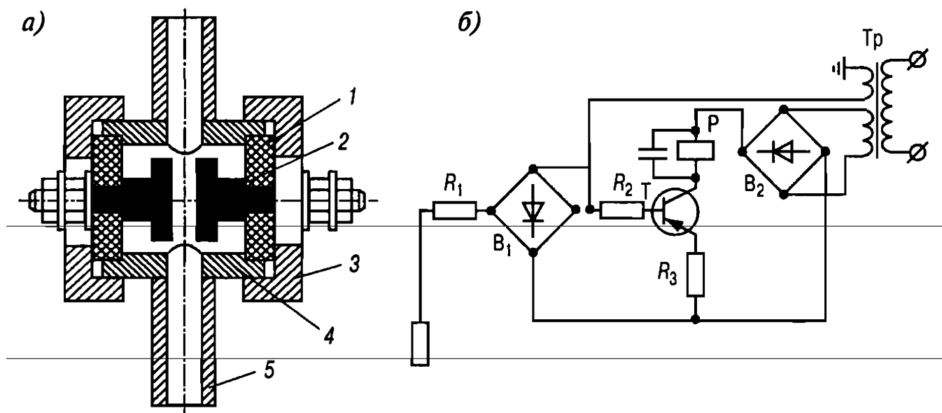
Рис. 84. Схема датчика контроля залива насоса:
