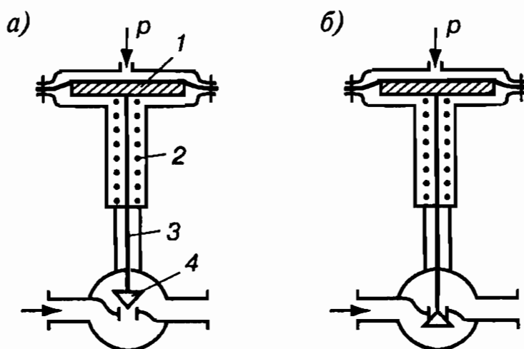
Рис. 47. Пневматический регулирующий клапан:
