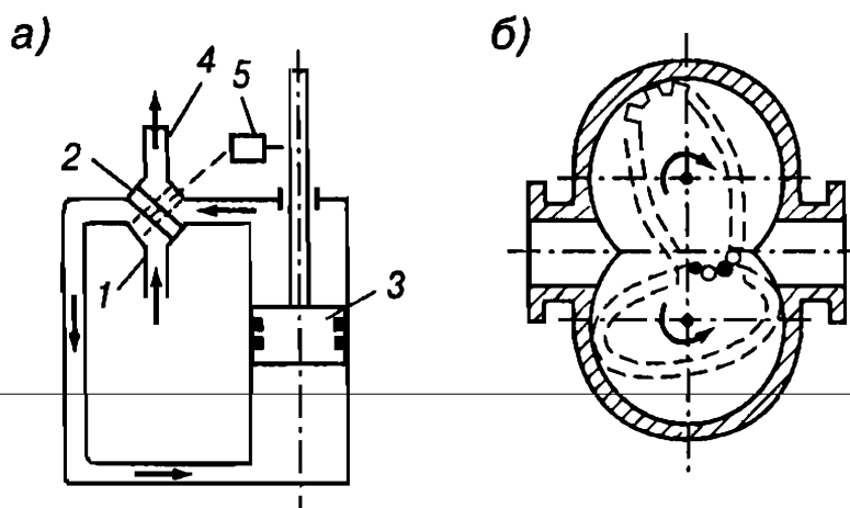
Рис. 19. Схема объемных счетчиков
