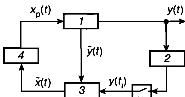
Рис. 73. Блок-схема АСР параметра качества:
