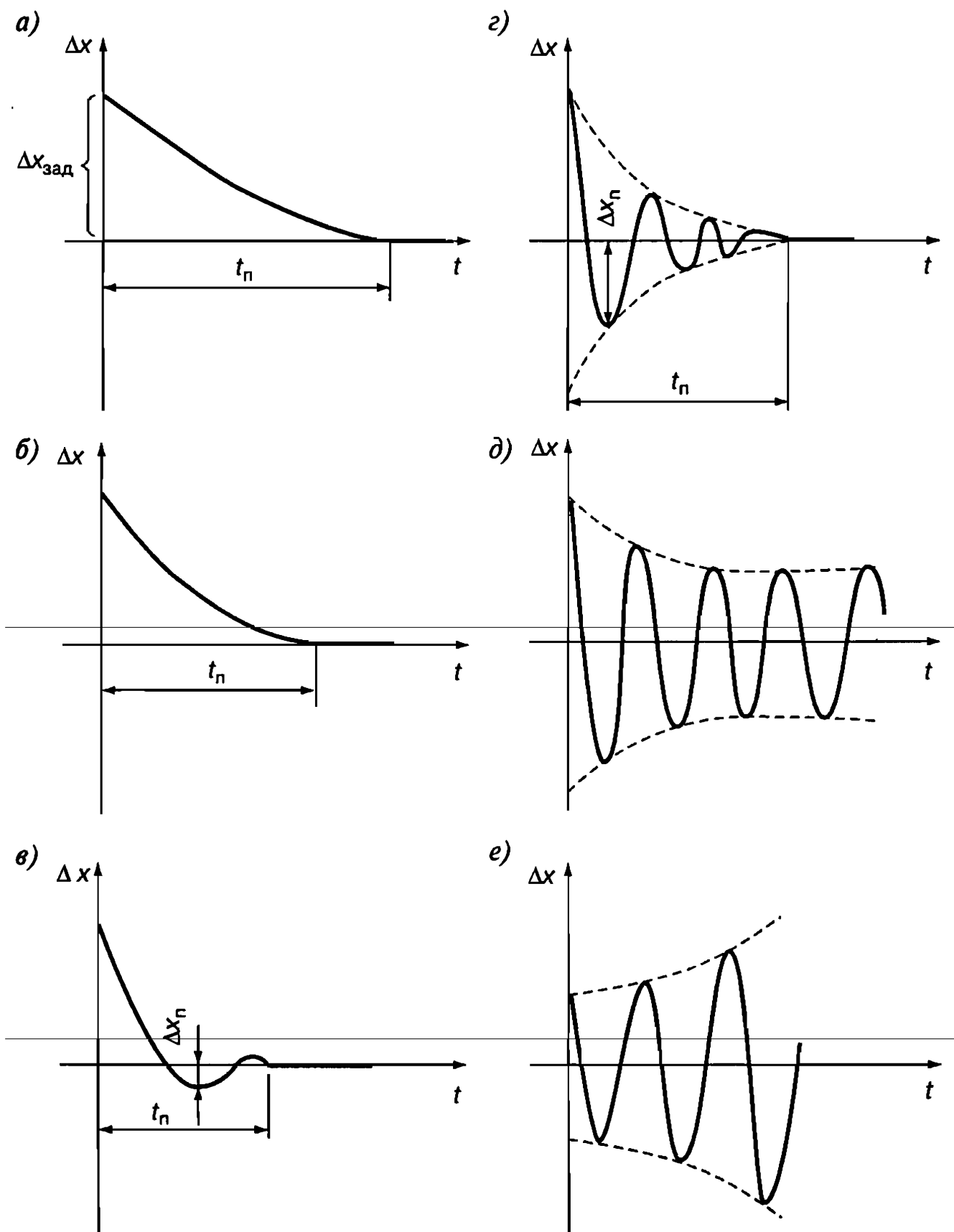
Рис. 39. Переходные процессы в замкнутой АСР при изменении параметров настройки регулятора
