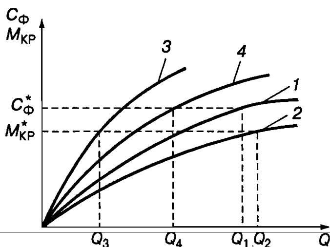
Рис. 112. Характеристики шнековой центрифуги по каналам «расход Q — крутящий момент M_{\text{кр}} » (кривые 2 и 3) и «расход Q — концентрация фугата C_{\text{ф}} » (кривые 1 и 4)
