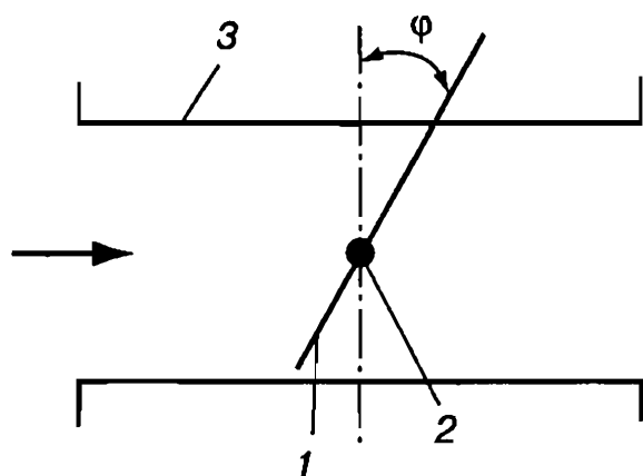
Рис. 45. Поворотная заслонка:
