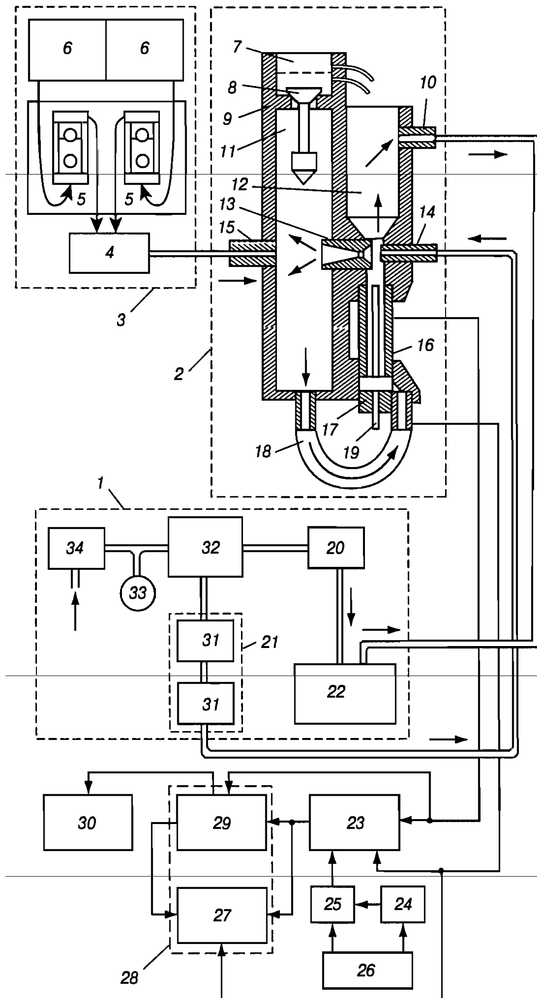
Рис. 27. Структурная схема анализатора хлора АПК-01М
