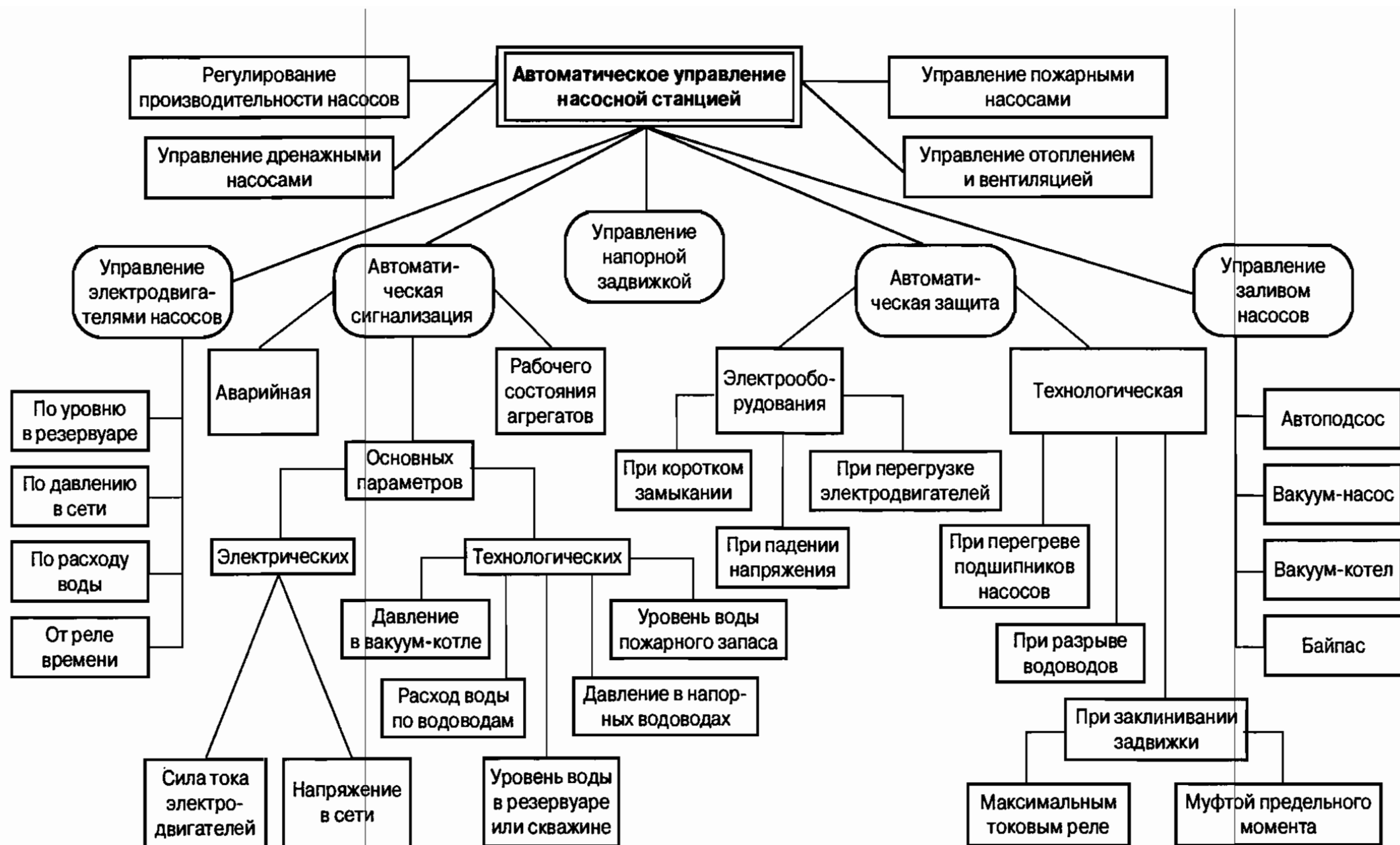
Рис. 80. Схема основных функций автоматики насосных станций
