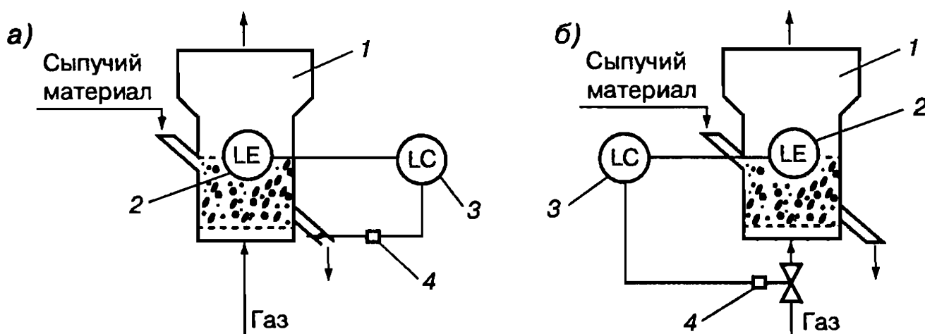
Рис. 58. Схемы регулирования уровня кипящего слоя:
