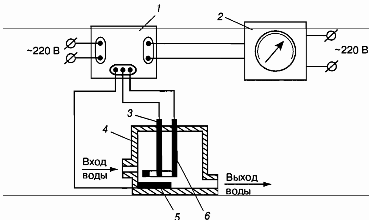
Рис. 28. Схема автоматического анализатора хлора КОХ-1:
