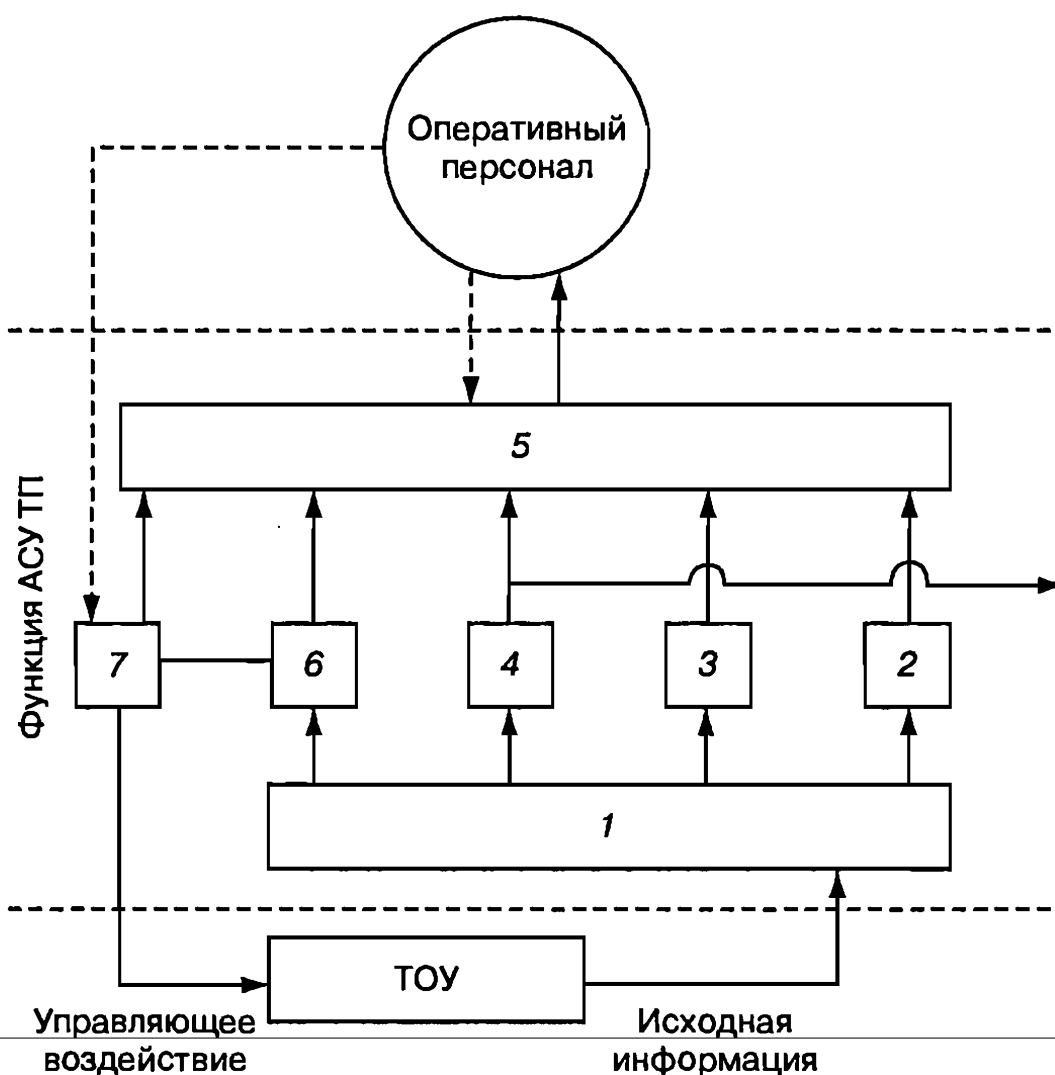
Рис. 113. Типовая функциональная структура АСУ ТП:
