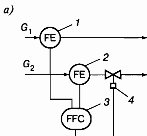
Рис. 54. Схема регулирования соотношения расходов при незаданной общей нагрузке:
