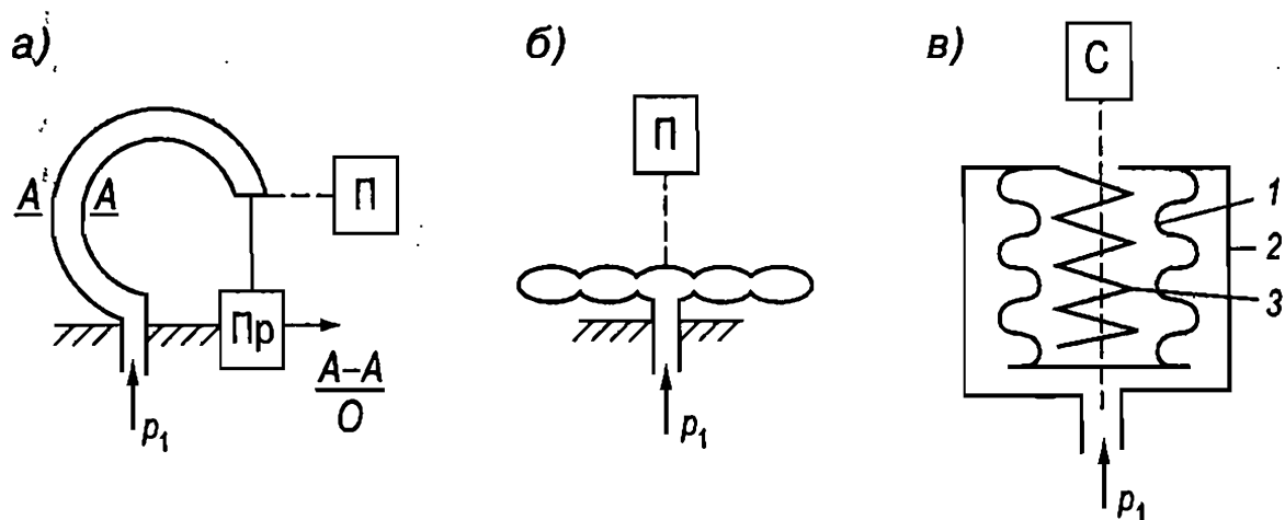
Рис. 12. Манометры с упругим чувствительным элементом (деформационные):
