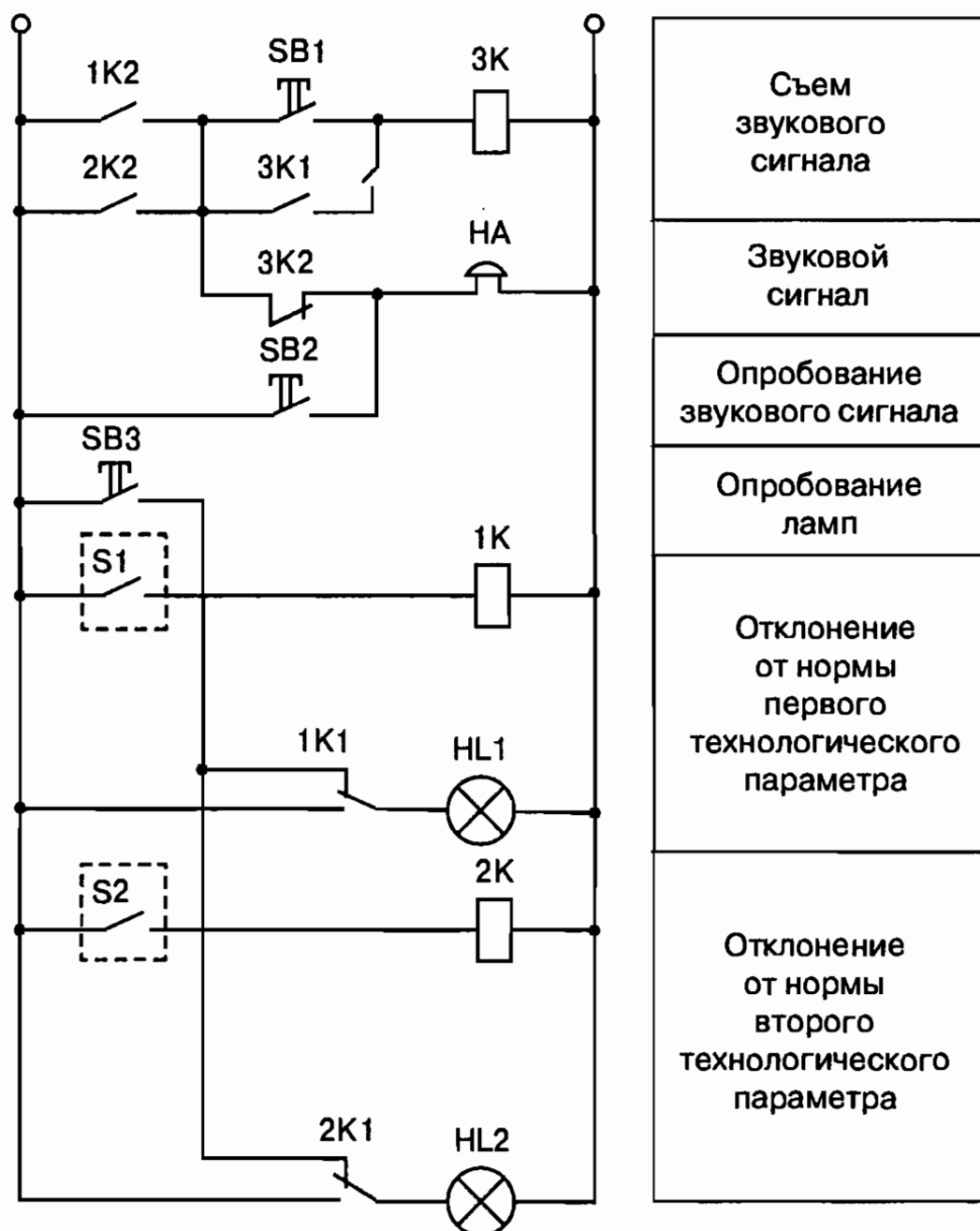
Рис. 74. Схема сигнализации
