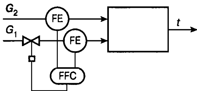
Рис. 66. Функциональная схема разомкнутой АСР температуры
