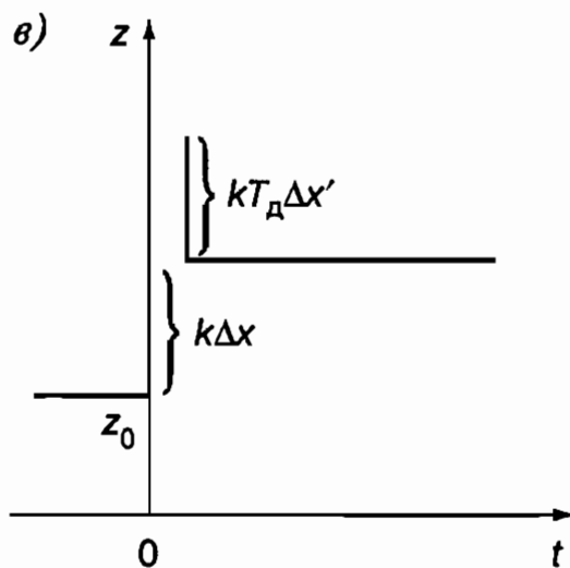
Рис. 36. Переходные процессы в регуляторе при скачкообразном входном воздействии:
