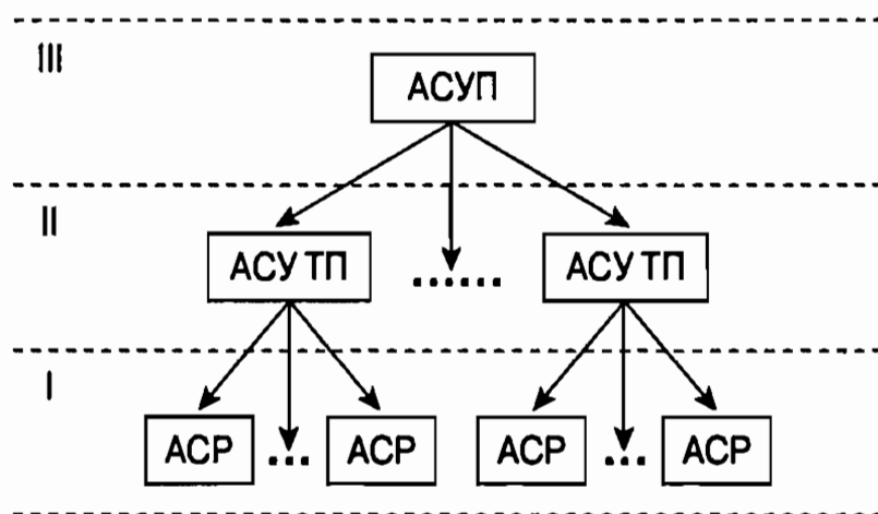
Рис. 3. Иерархия управления СВВ (предприятием водообработки)
