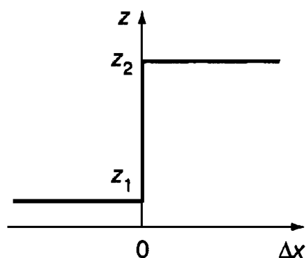
Рис. 38. График двухпозиционного закона регулирования
