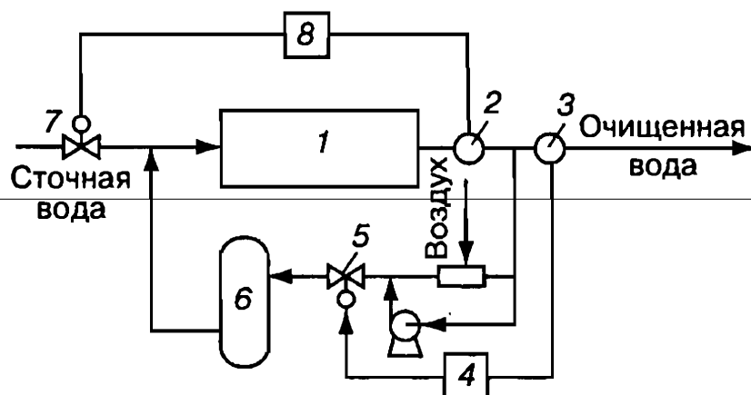
Рис. 106. Схема АСР процесса очистки сточных вод напорной флотацией
