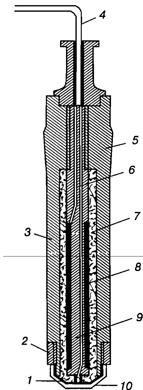
Рис. 29. Датчик для измерения концентрации растворенного кислорода
