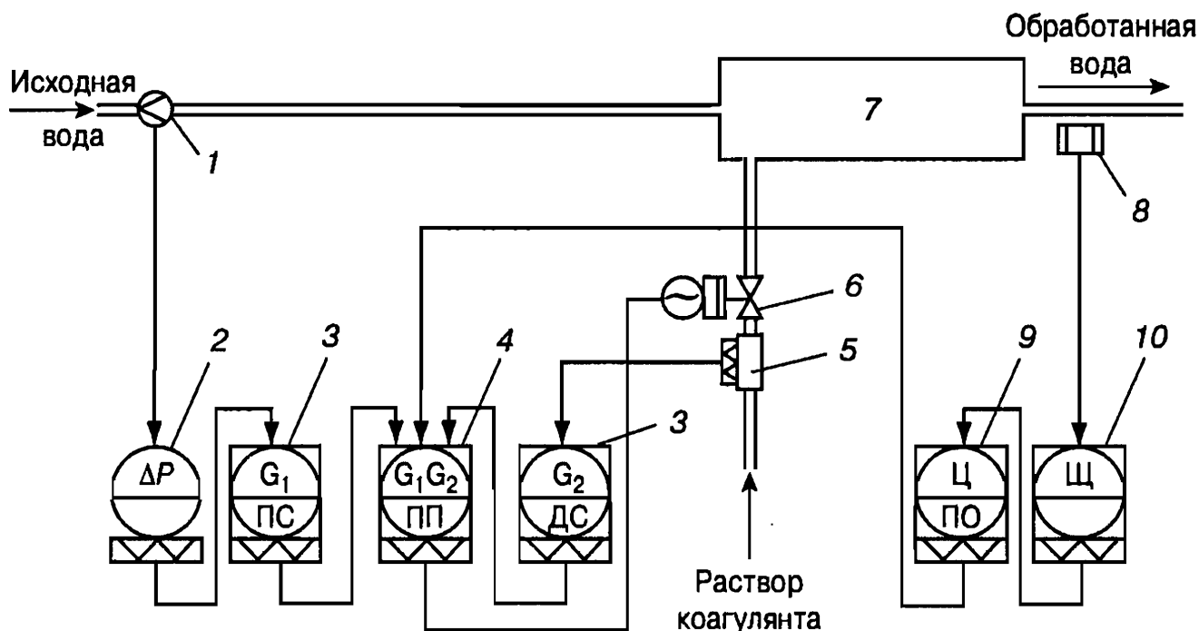
Рис. 89. Схема АСР подачи коагулянта с применением регулирующего клапана и двух расходомеров:
