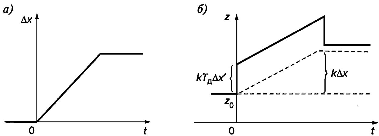
Рис. 37. Переходный процесс в ПД-регуляторе при постепенном изменении входного воздействия:
