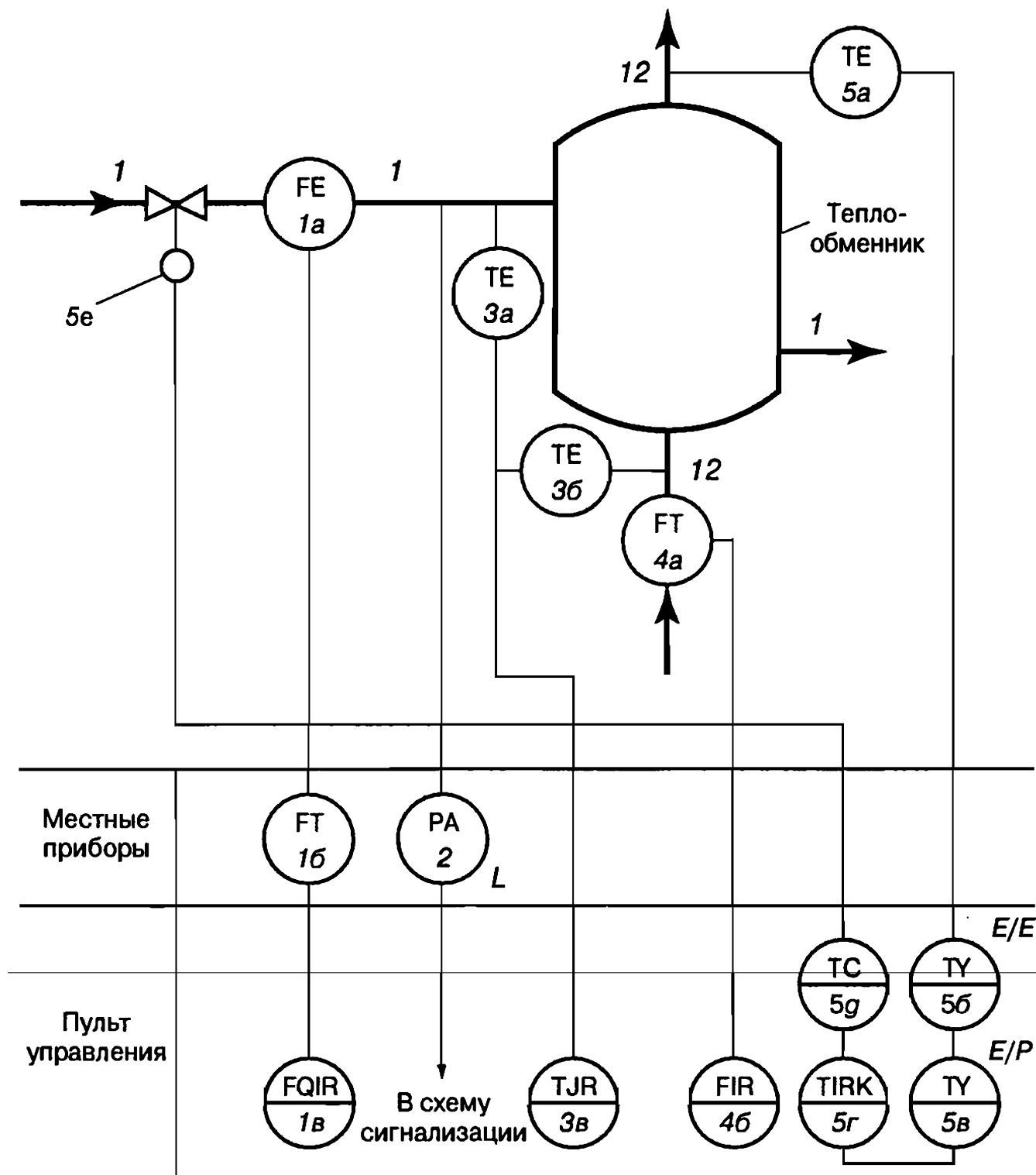
Рис. 51. Функциональная схема автоматизации процесса нагревания воды в теплообменнике
