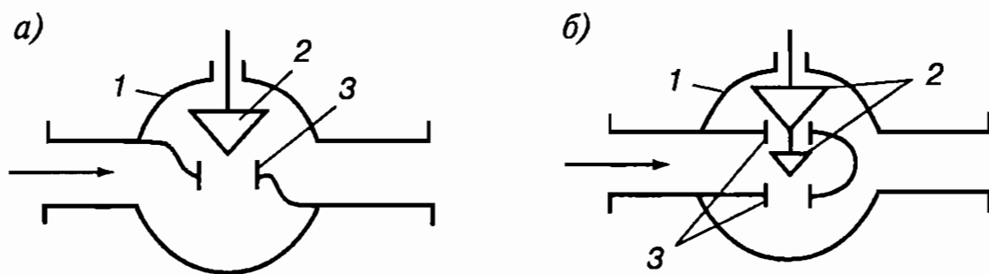
Рис. 43. Регулирующие клапаны: а — односедельный; б — двухседельный; 1 — корпус; 2 — плунжер; 3 — седло
