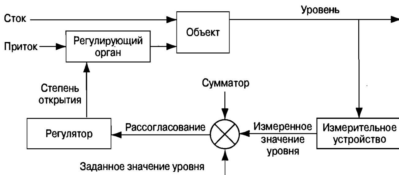
Рис. 6. Структурная схема АСР уровня в емкости
