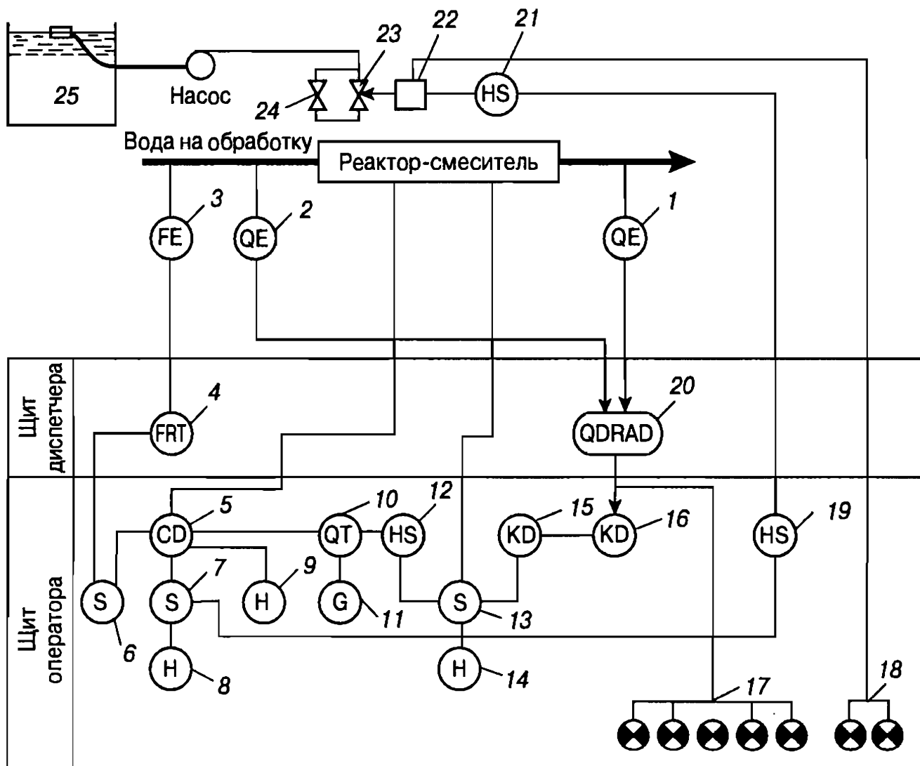
Рис. 91. Схема кондуктометрической комбинированной АСР дозирования коагулянта с импульсным регулирующим клапаном:
