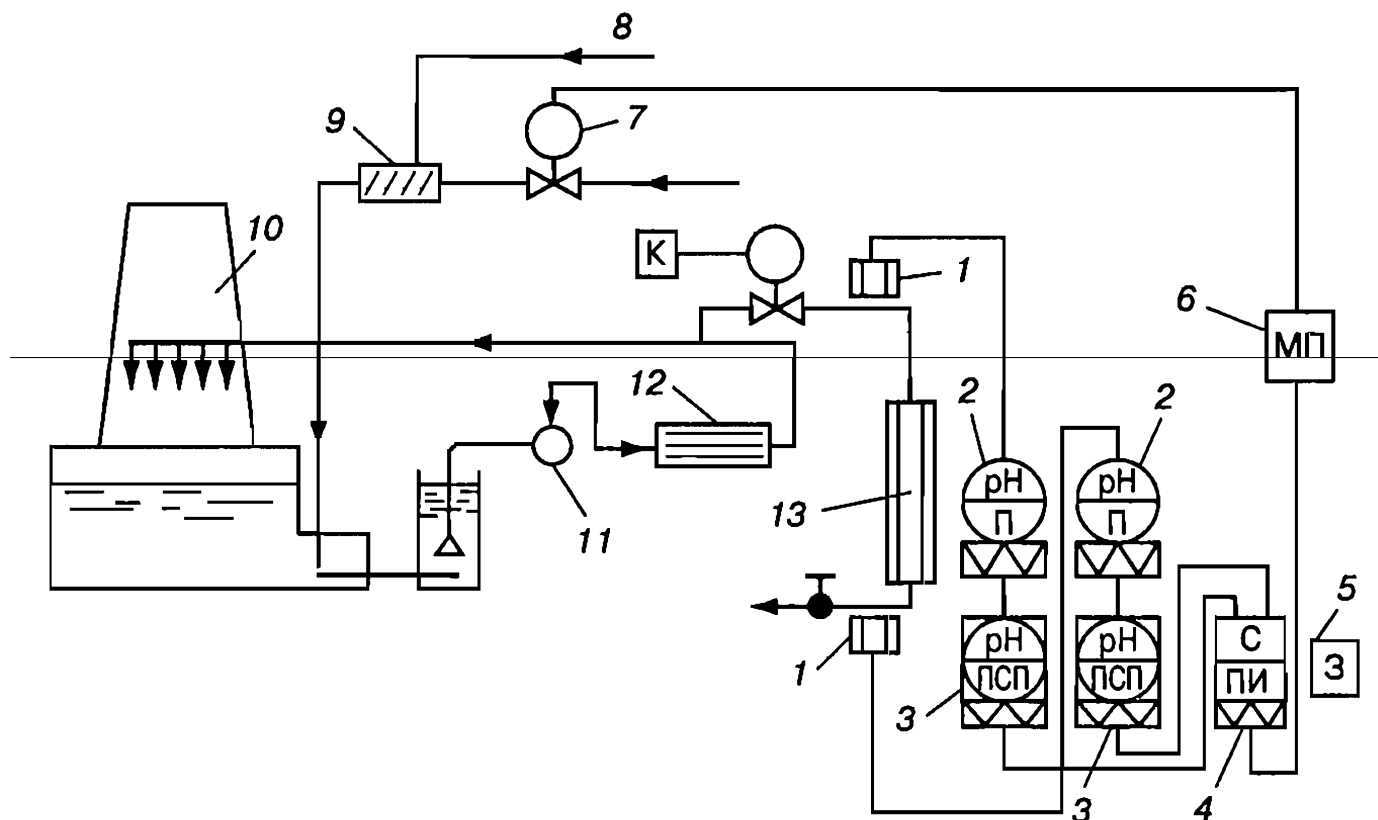
Рис. 102. Схема АСР подкисления охлаждающей воды по показателю карбонатной агрессивности:
