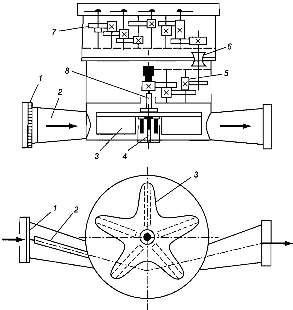
Рис. 18. Схема устройства скоростного счетчика количества жидкости с вертикальной осью вращения вертушки
