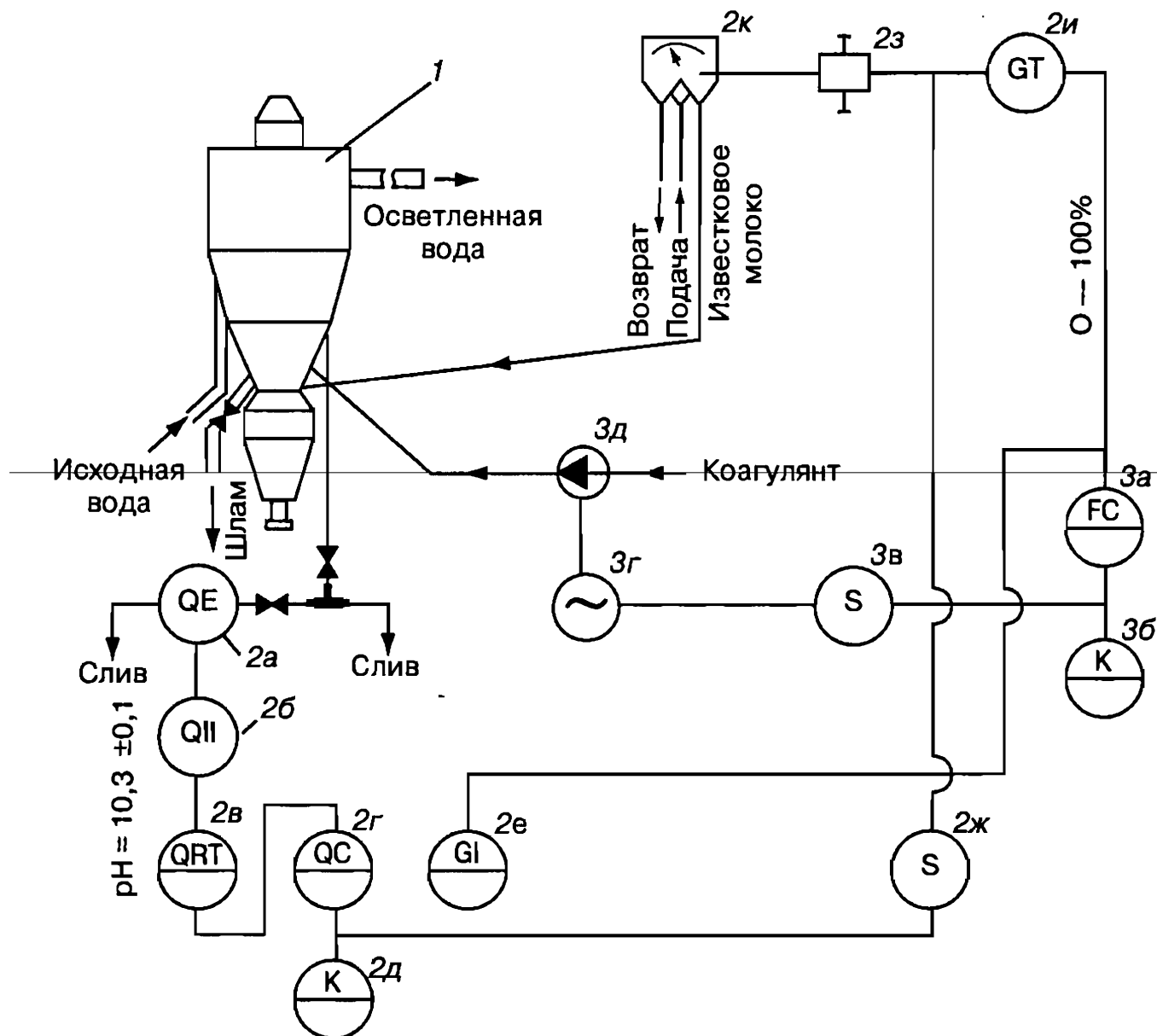
Рис. 100. Схема АСР процесса декарбонизации воды в осветлителе:
