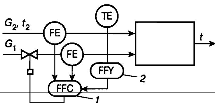
Рис. 67. Функциональная схема разомкнутой АСР температуры с компенсацией двух возмущений:
