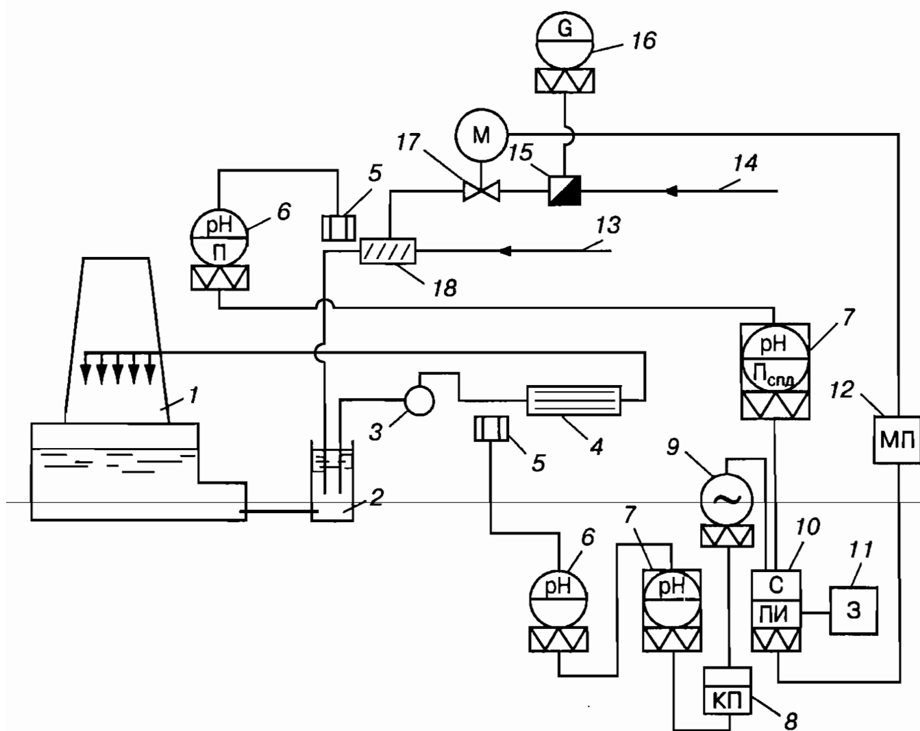
Рис. 101 Схема АСР подкисления охлаждающей воды по величине pH:
