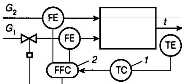
Рис. 68. Функциональная схема двухкаскадной АСР температуры:
