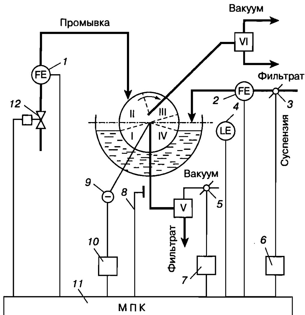
Рис. 110. Схема АСР вакуум-фильтра непрерывного действия:
