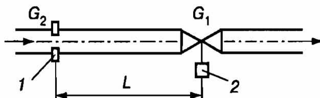
Рис. 52. Принципиальная схема объекта при регулировании расхода:
