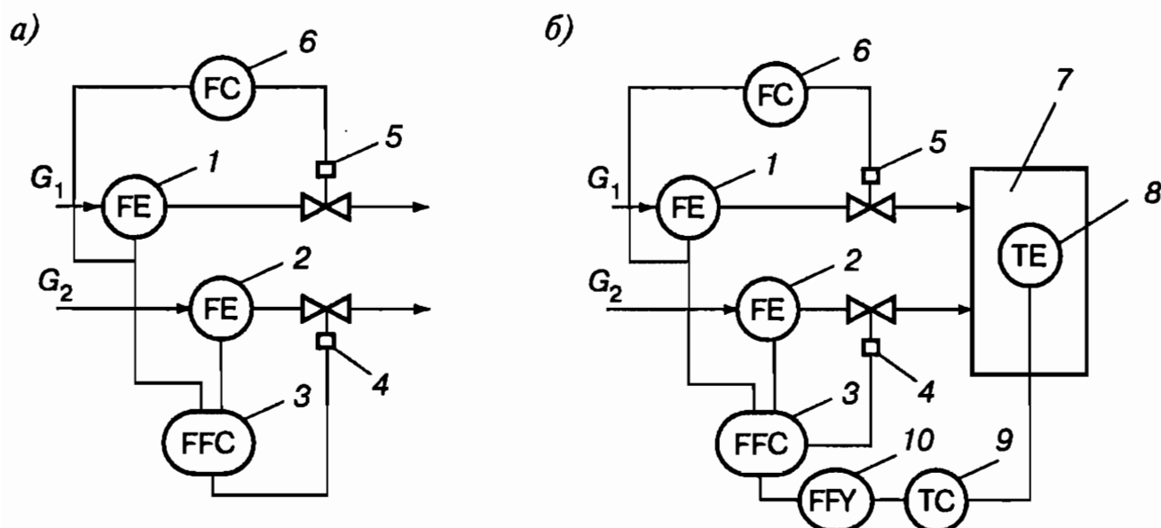
Рис. 55. Схема регулирования соотношения расходов при задании общей нагрузке (а) и коррекции коэффициента соотношения по третьему параметру (б):
